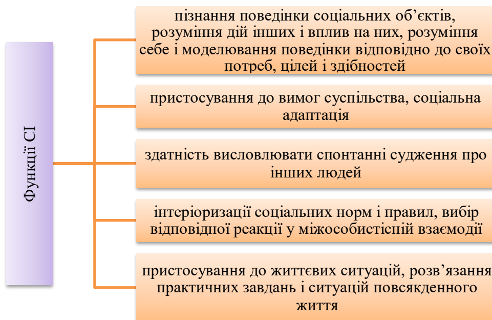
Рис. 1. Функції СІ
