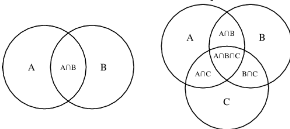
Venn diagram
