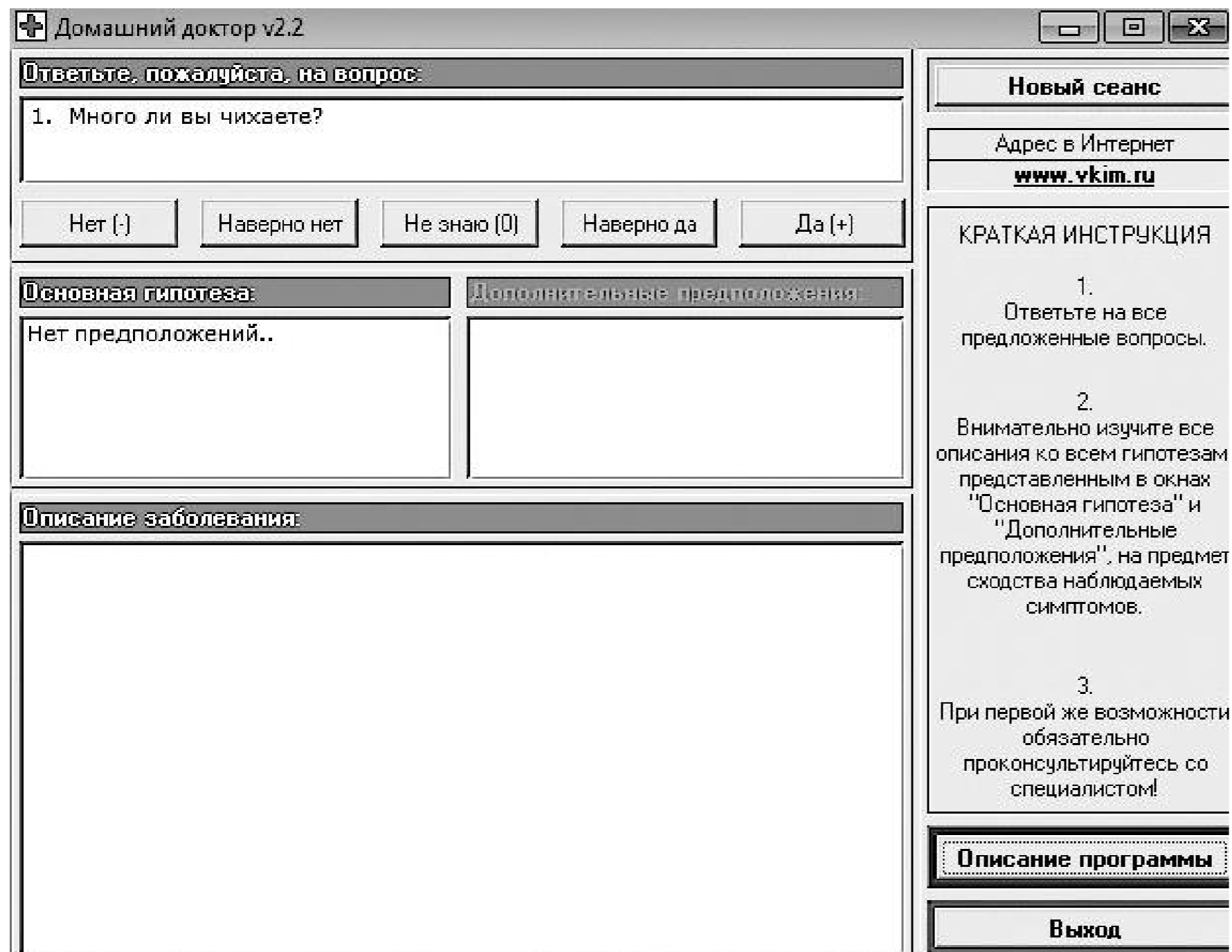
Рис. 5.31. Окно программы «Домашний доктор»
