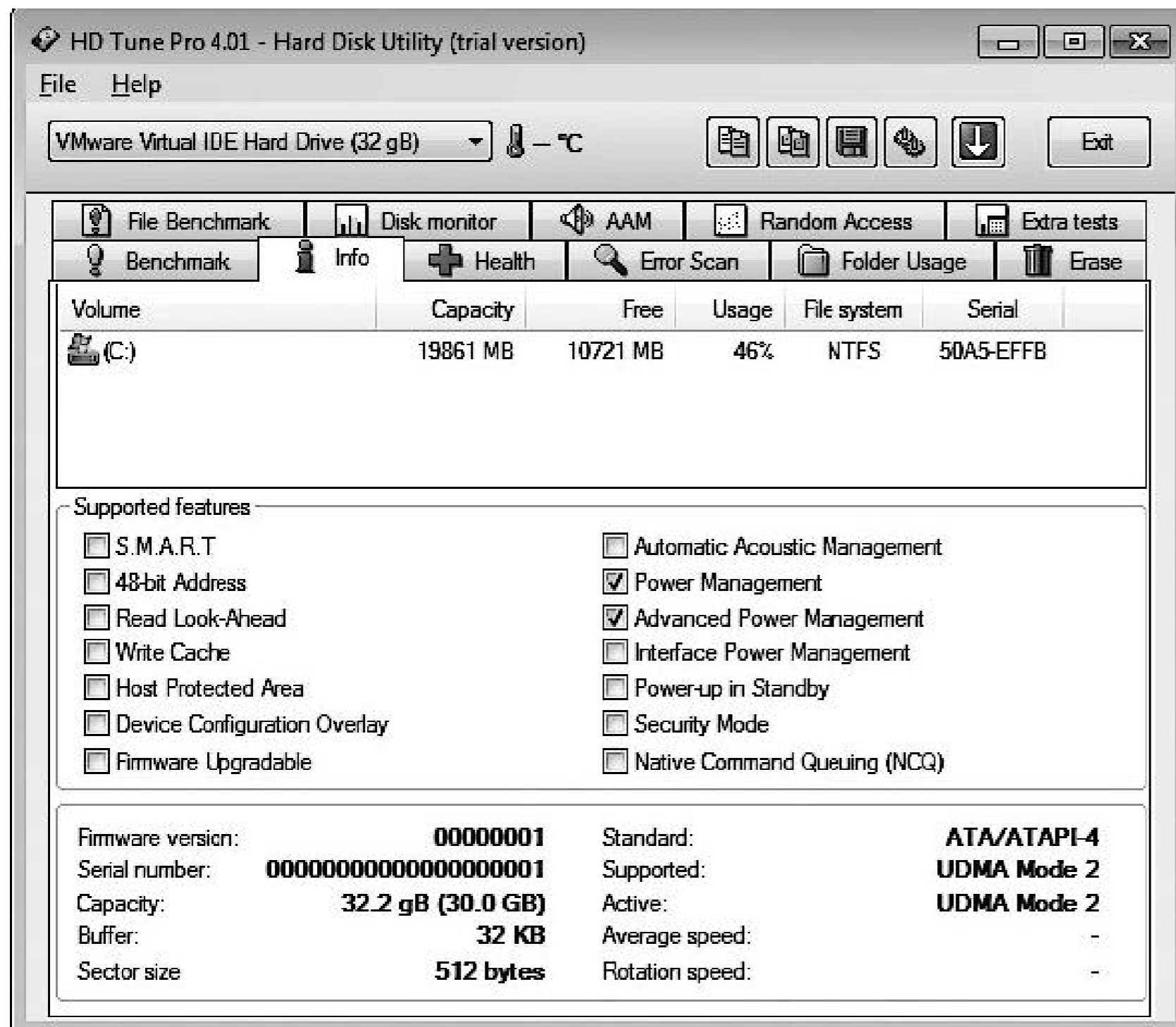
Рис. 1.27. Вкладка Info программы HD Tune Pro
