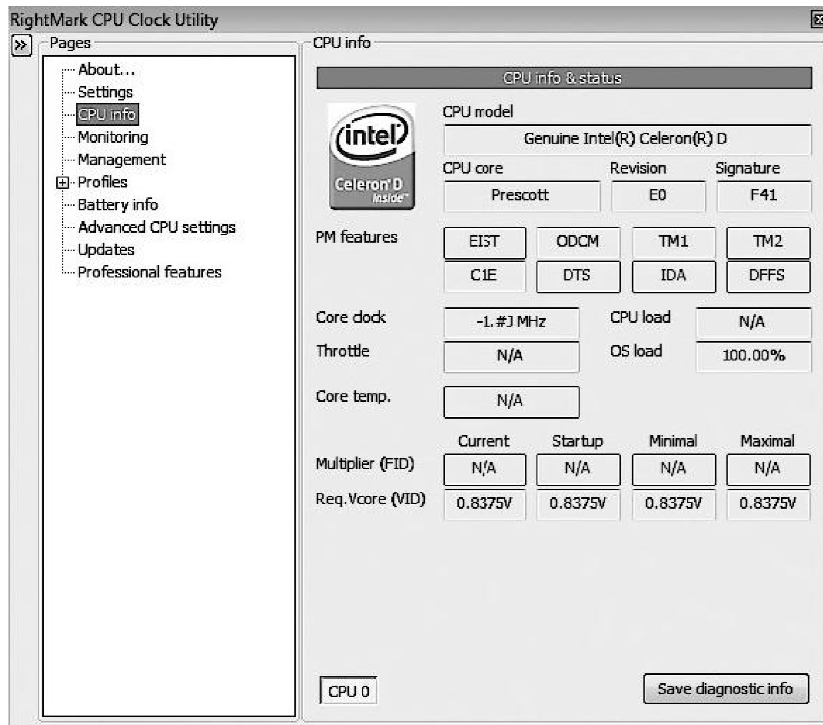
Рис. 1.3. Программа RightMark CPU Clock Utility
