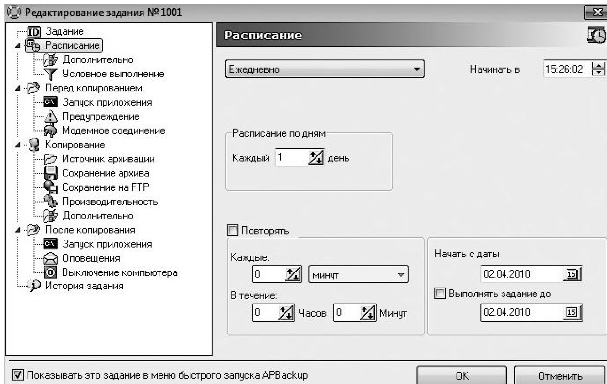
Рис. 4.7. Планировщик заданий
