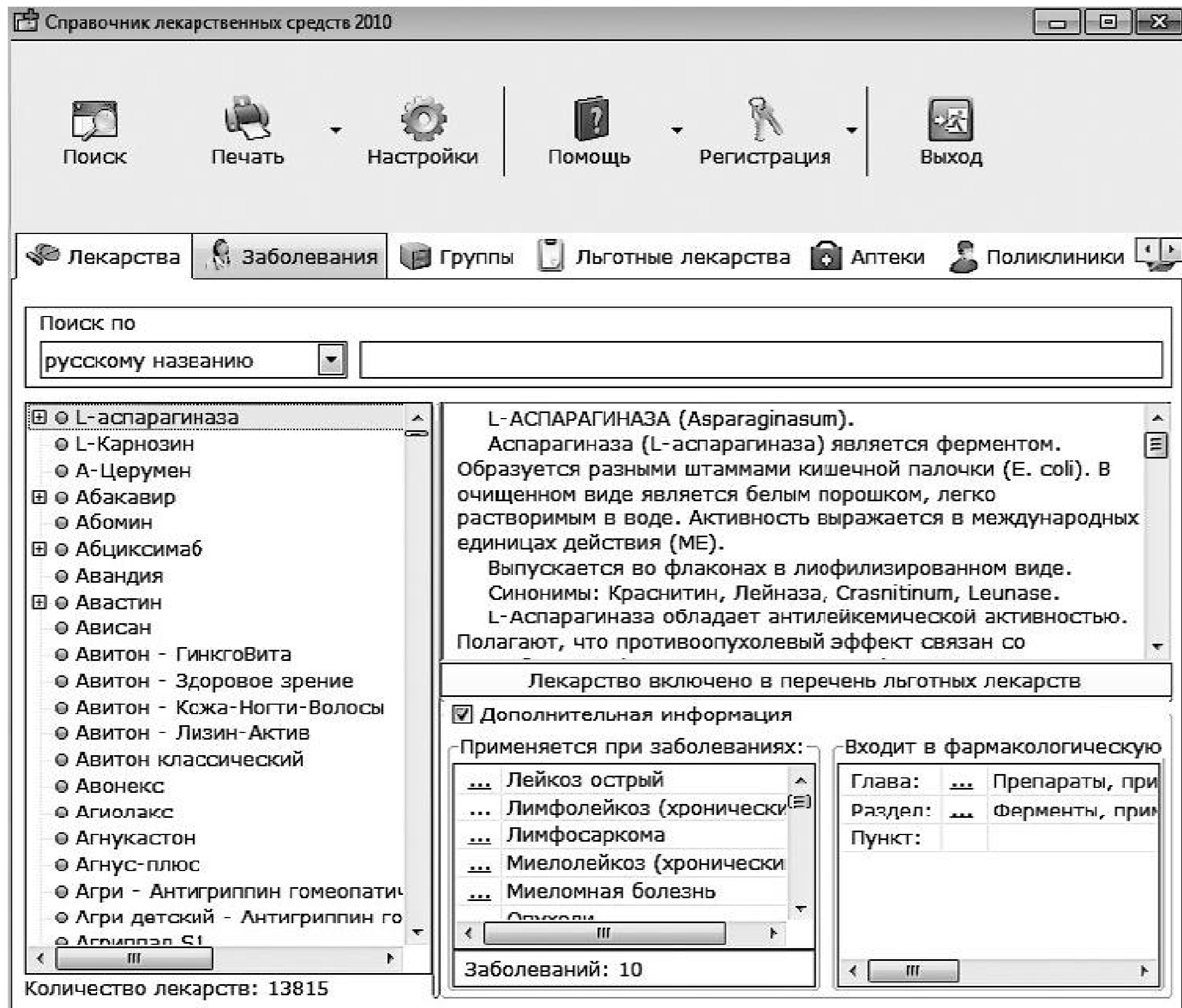
Рис. 5.32. Окно программы
