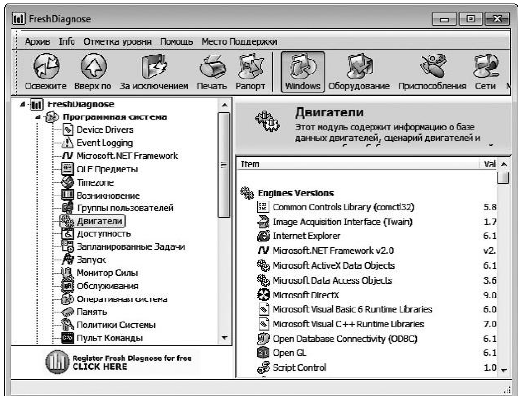
Рис. 1.2. Программа FreshDiagnose
