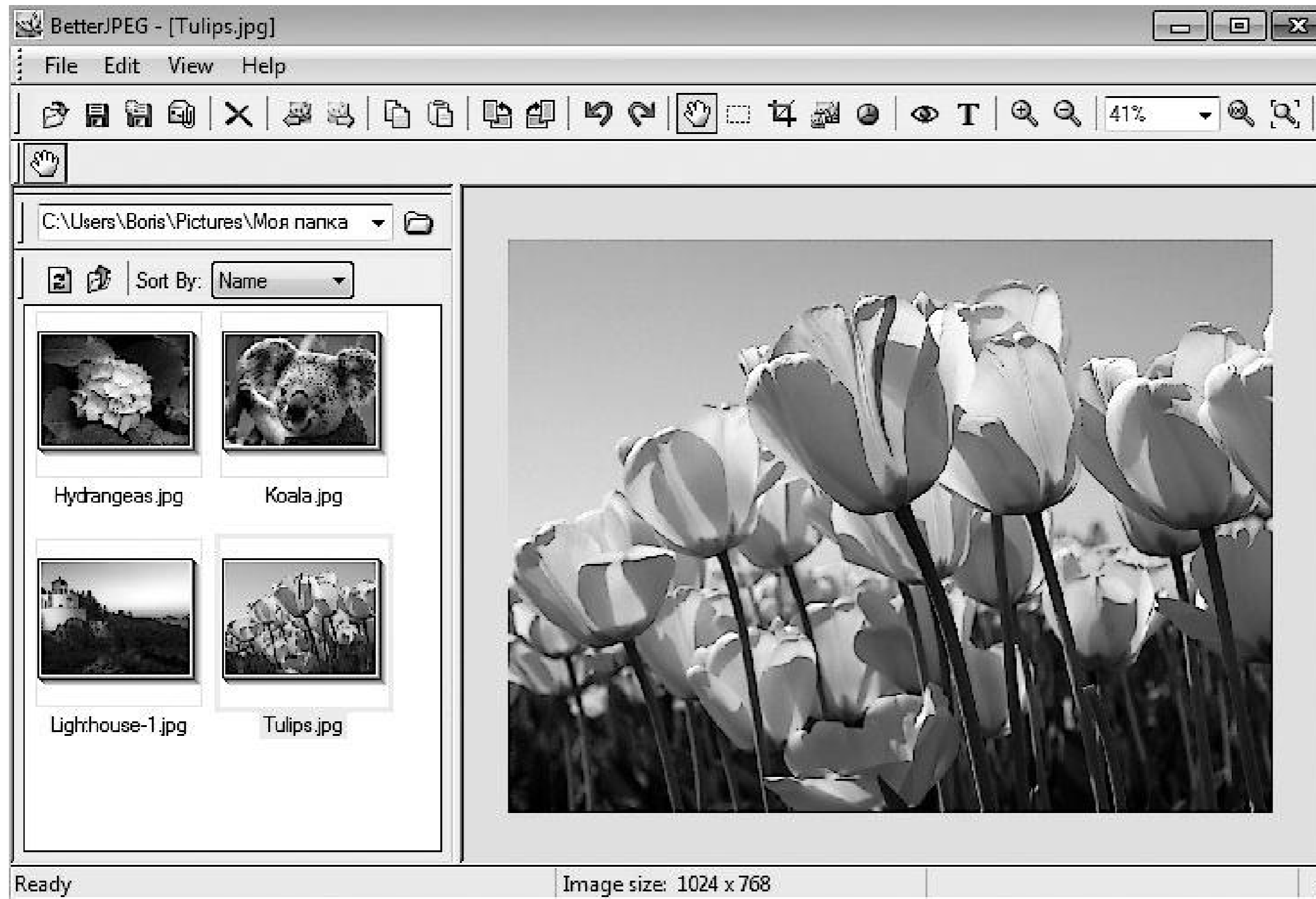
Рис. 11.6. Окно приложения
