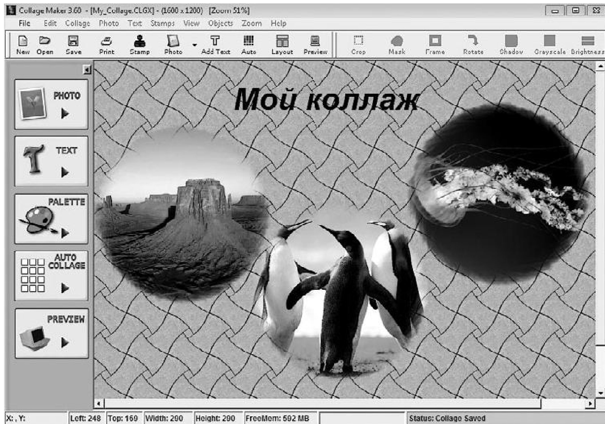
Рис. 11.8. Коллаж, созданный
