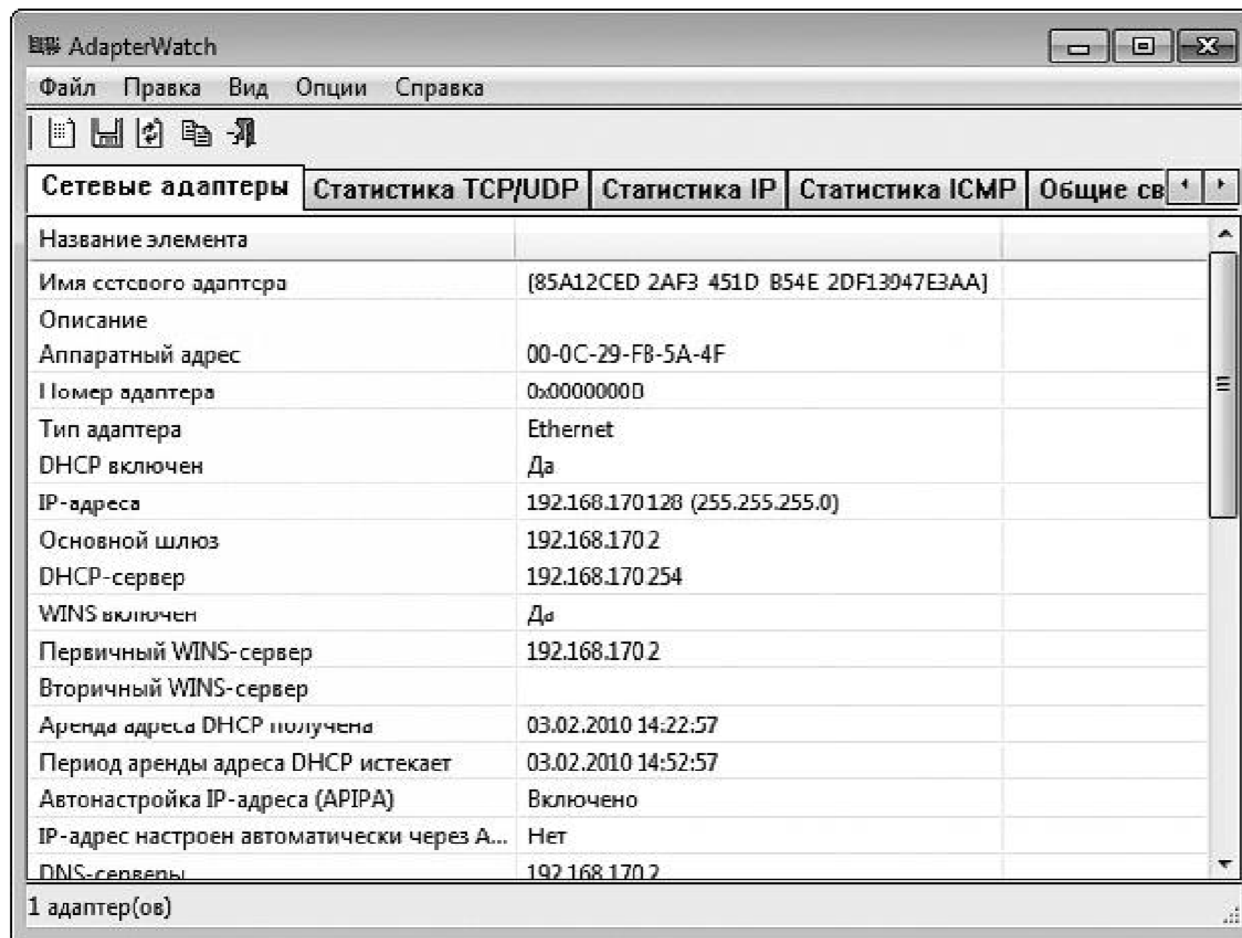
Рис. 1.1. Программа AdapterWatch
