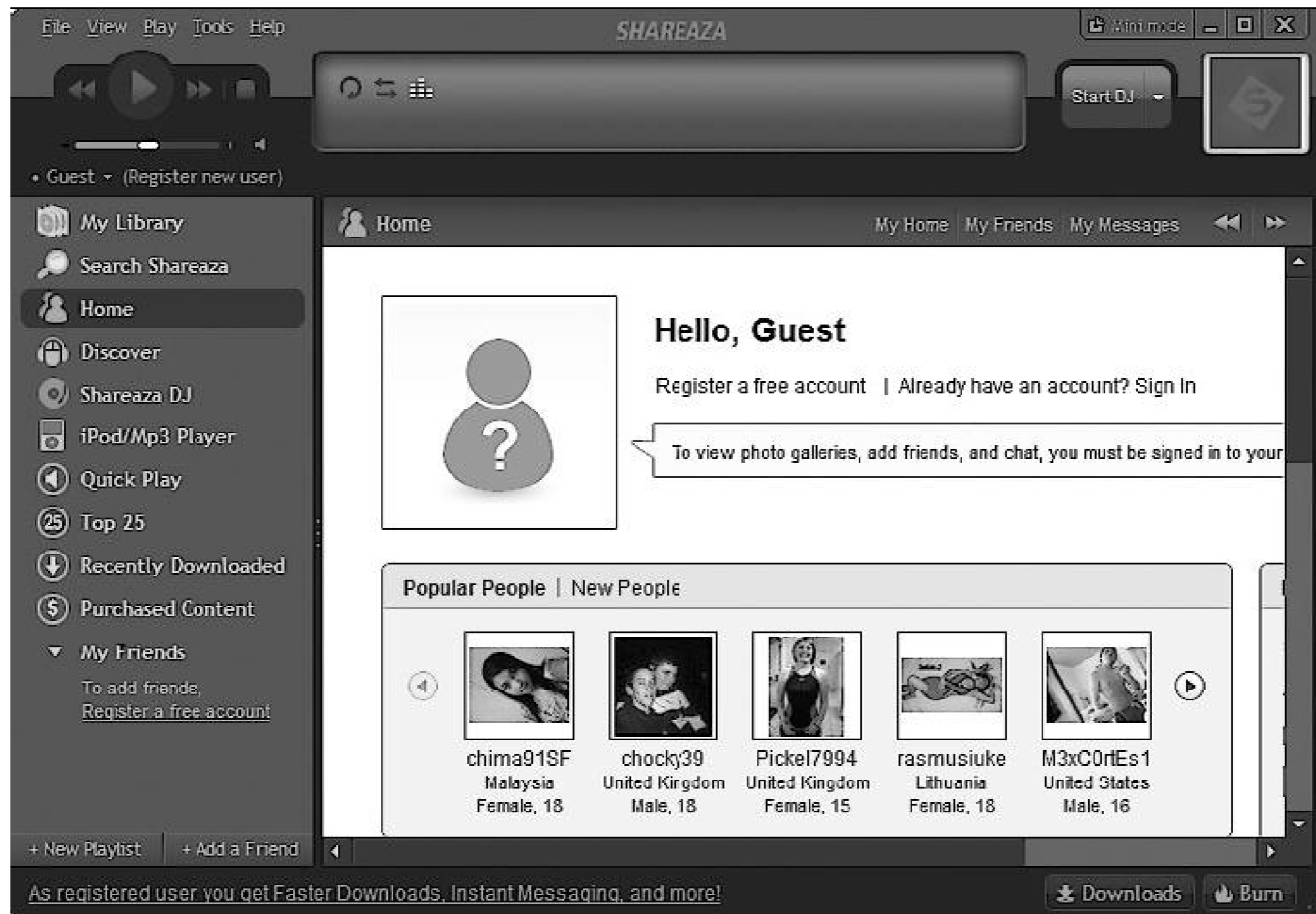
Рис. 8.8. Окно программы
