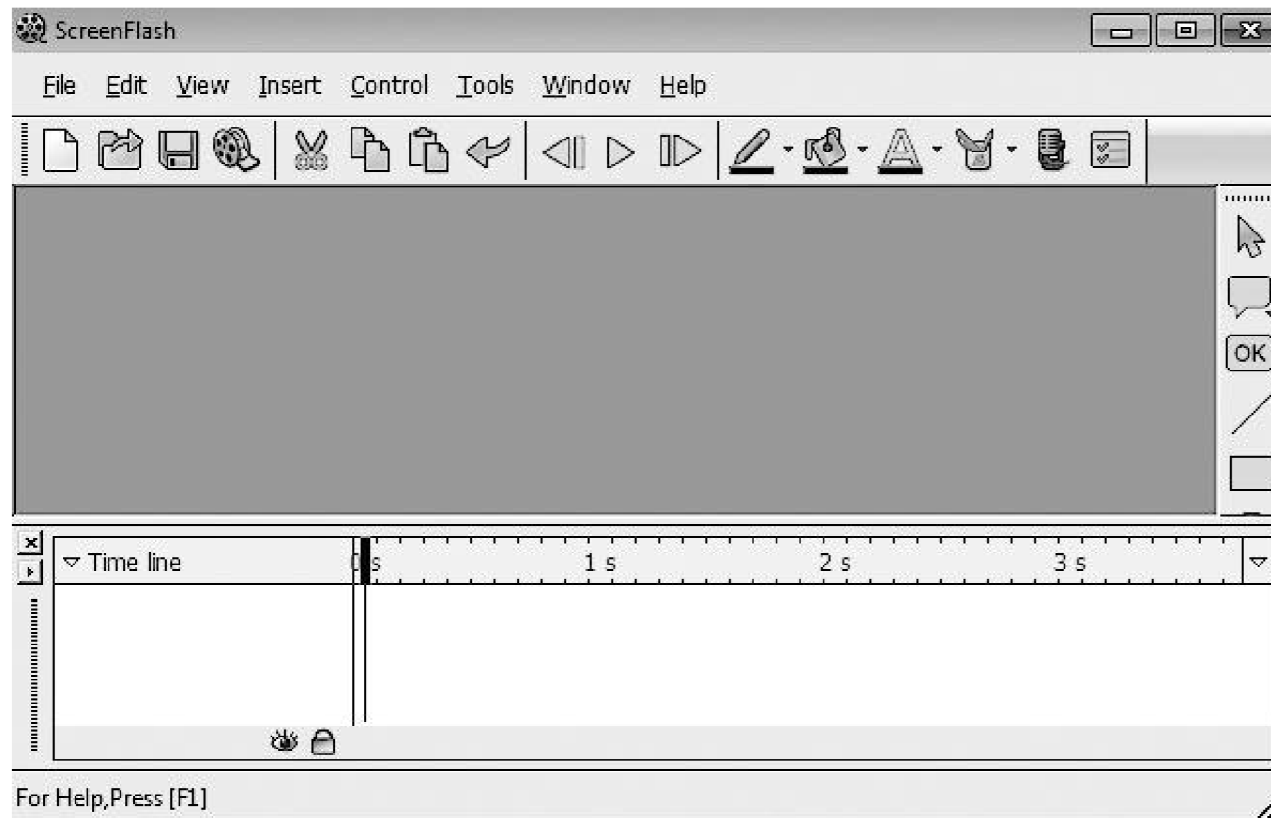
Рис. 12.16. Интерфейс программы
