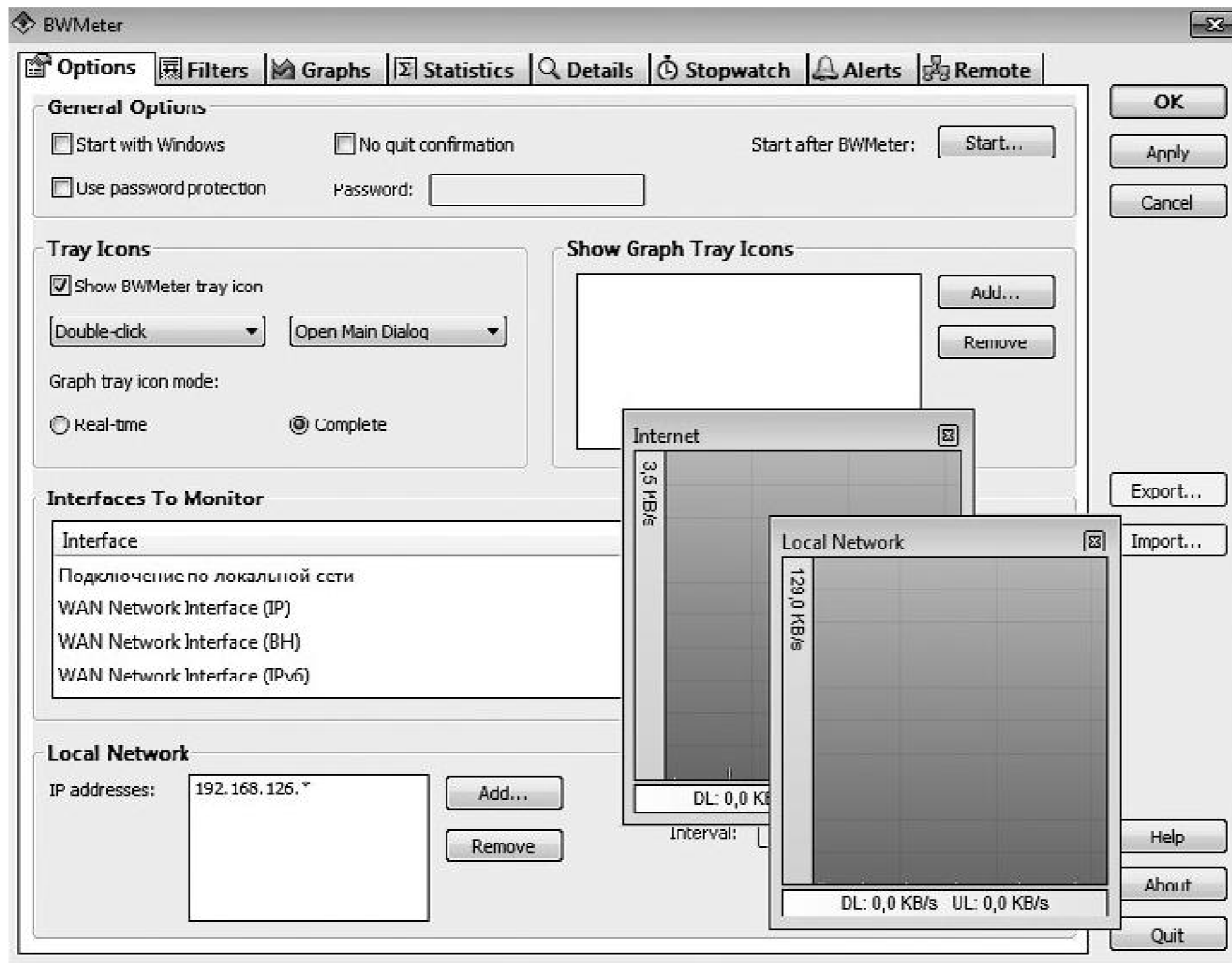
Рис. 10.7. Окно программы
