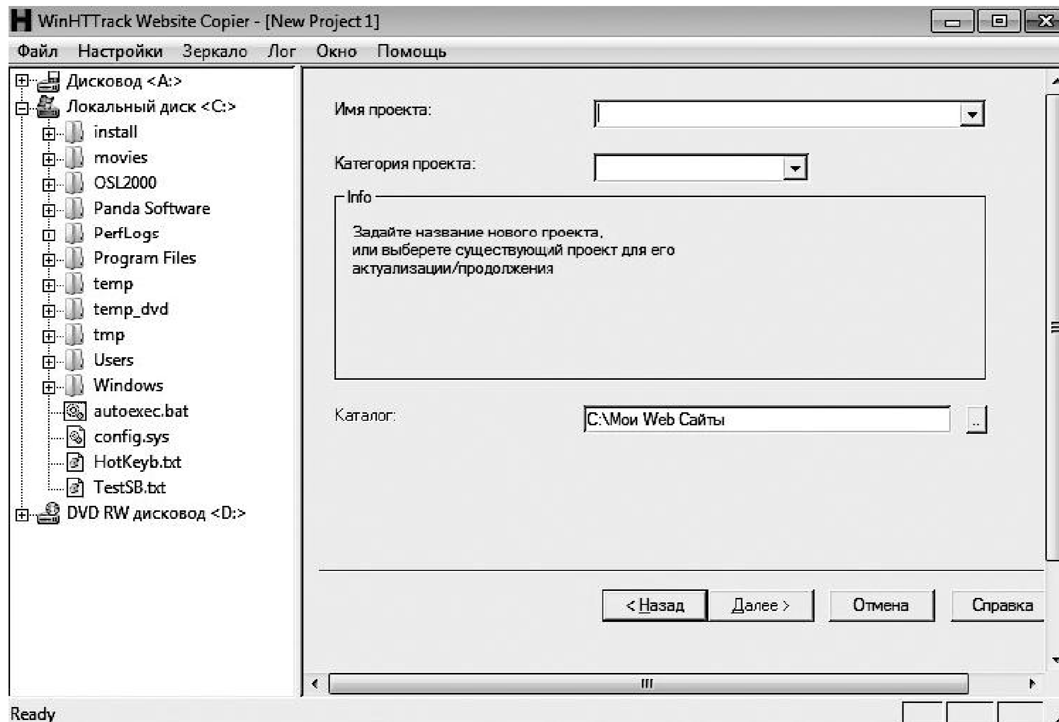
Рис. 7.8. Окно программы
