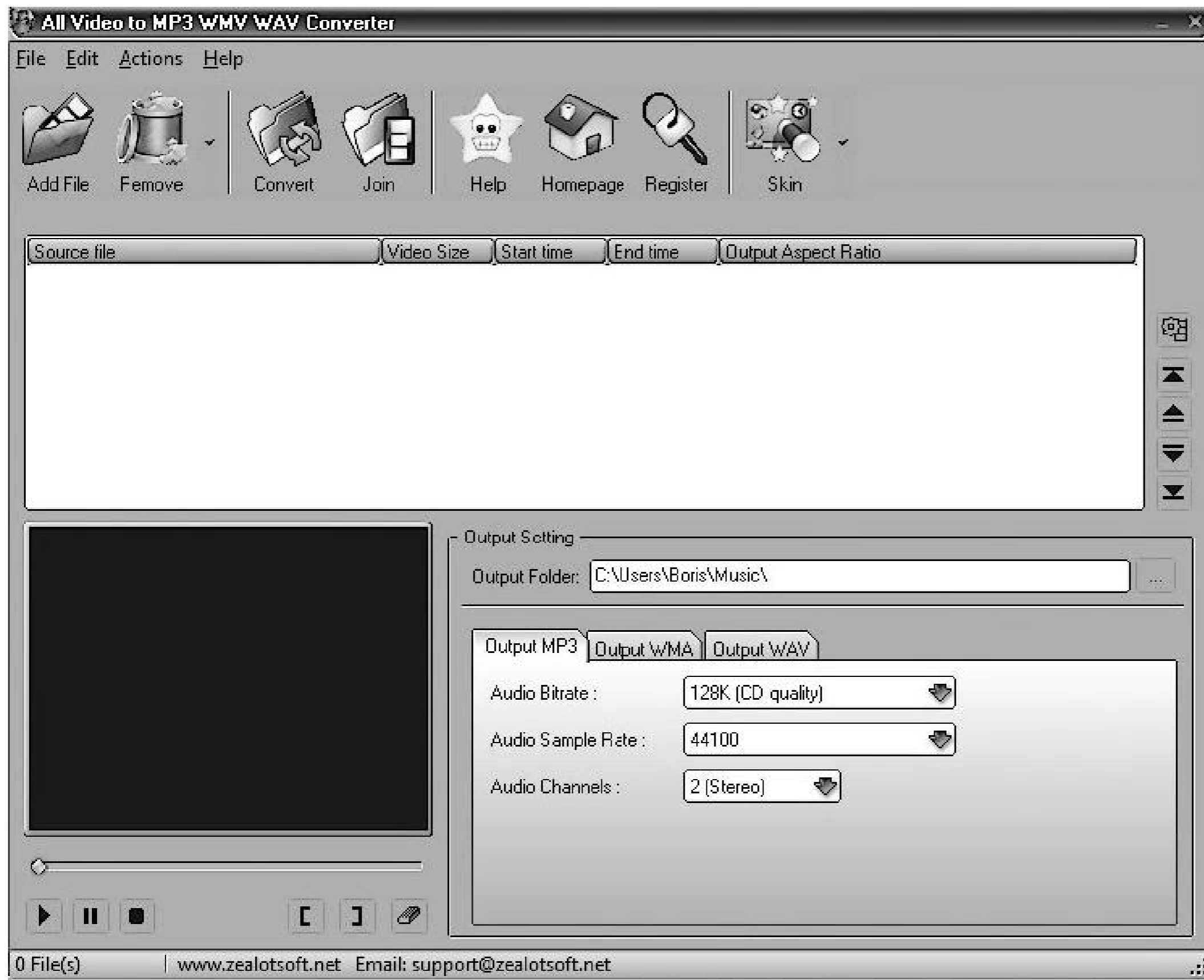
Рис. 12.20. Интерфейс
