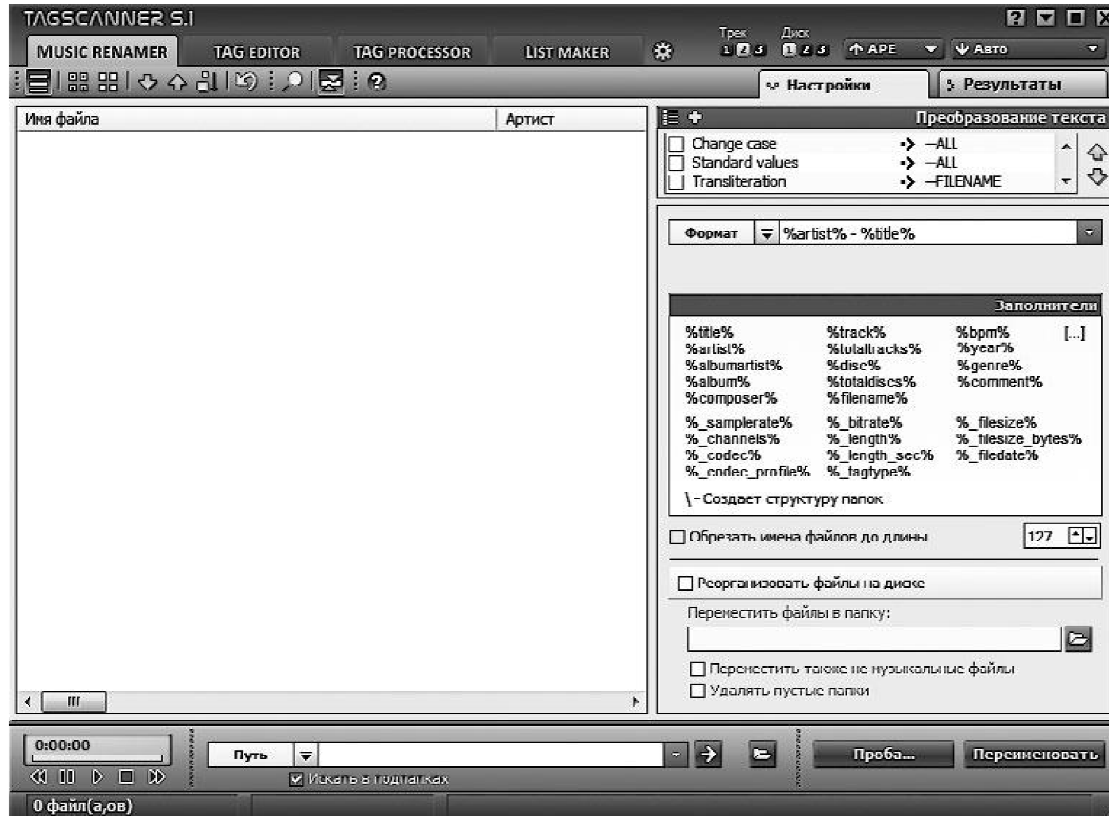
Рис. 12.13. Интерфейс
