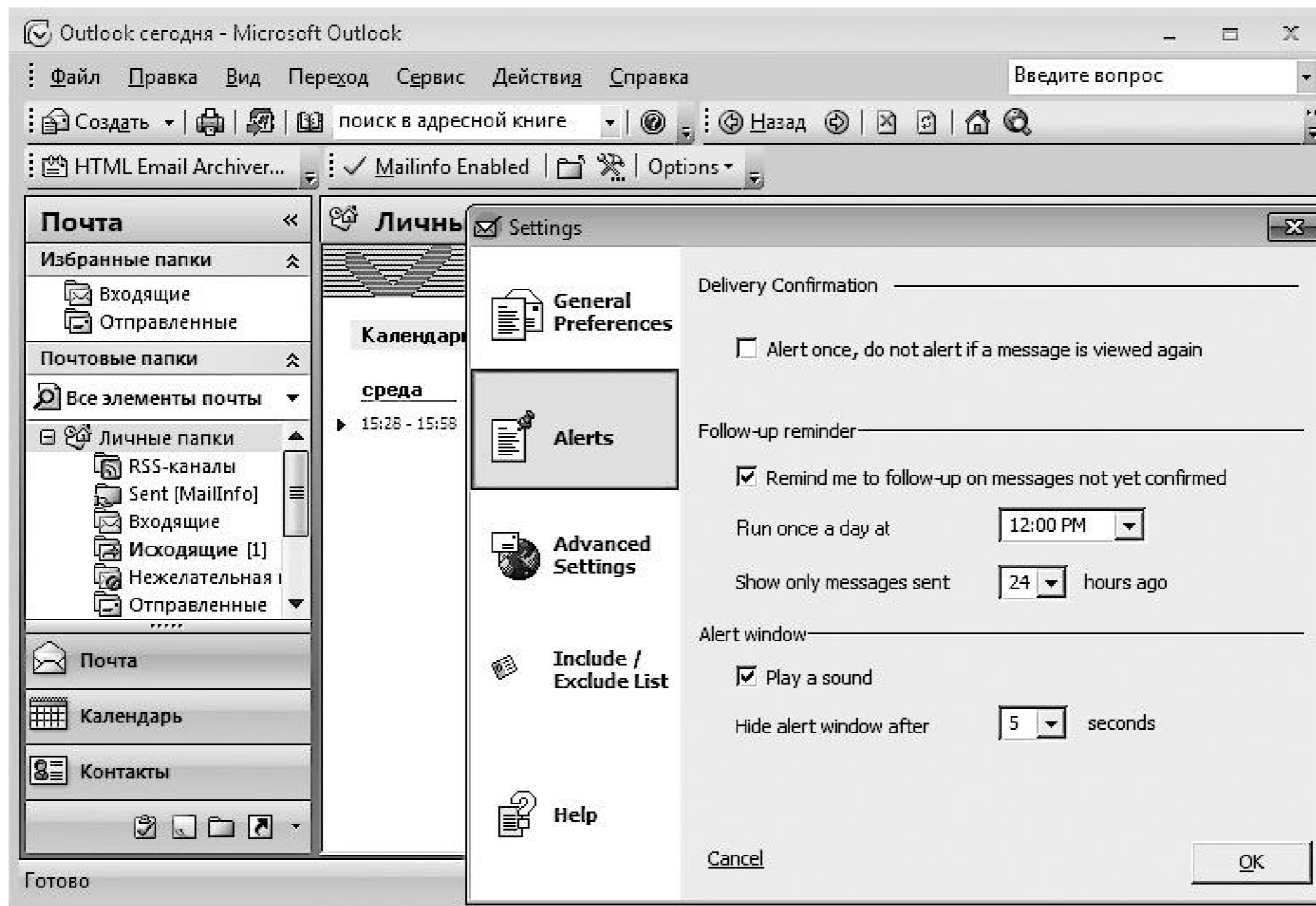
Рис. 9.8. Мастер программы
