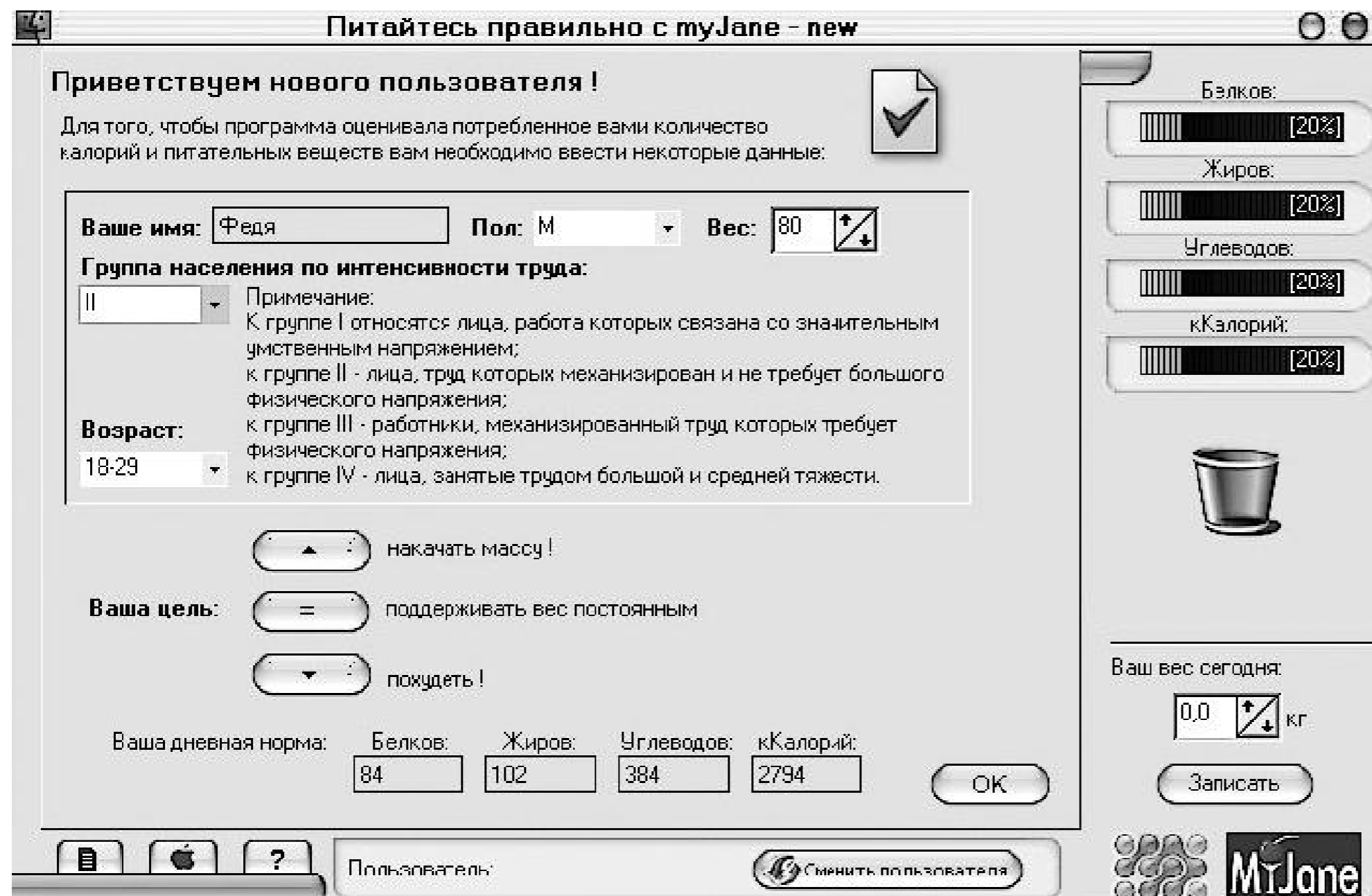
Рис. 14.5. Окно программы
