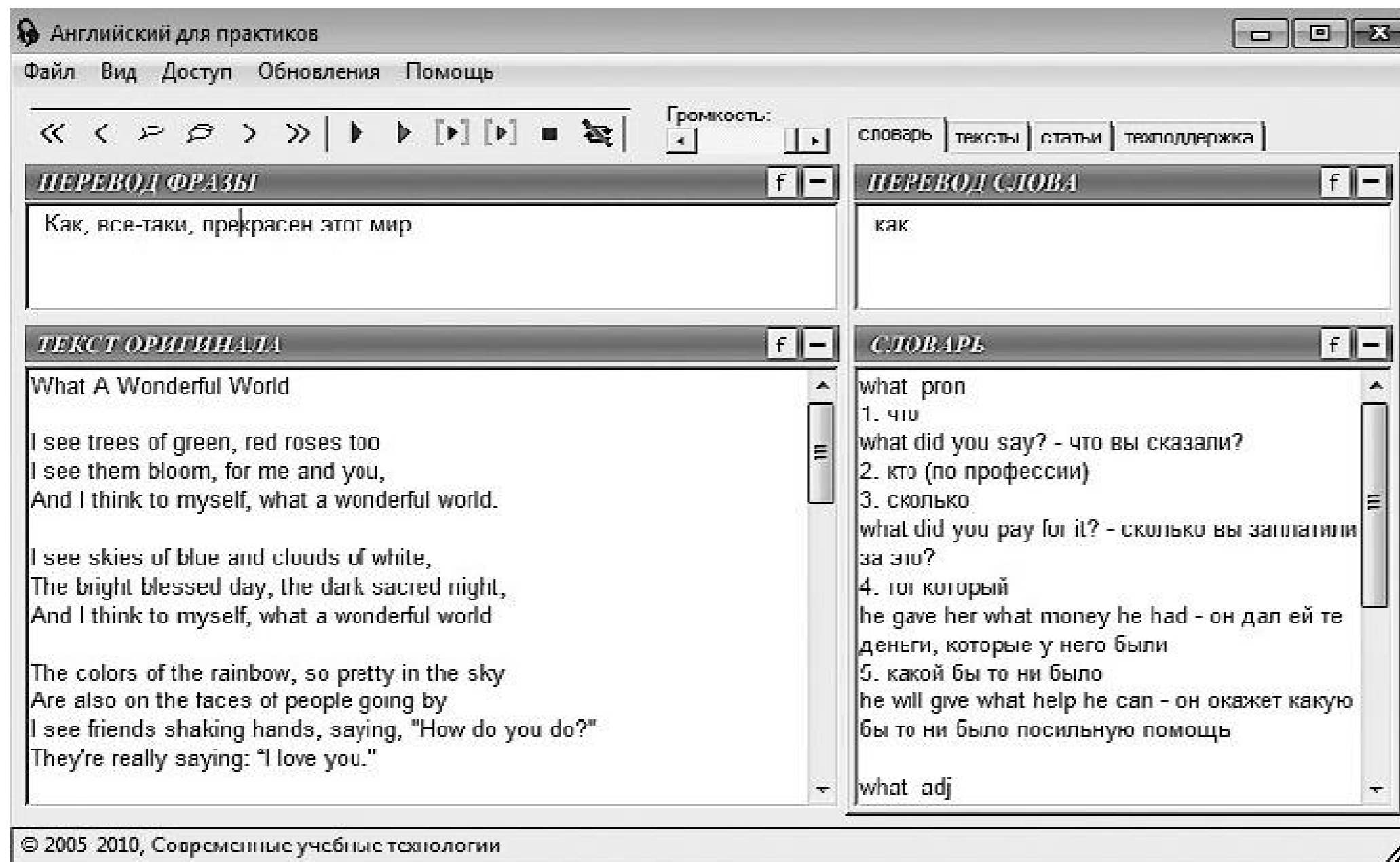
Рис. 13.4. Интерфейс
