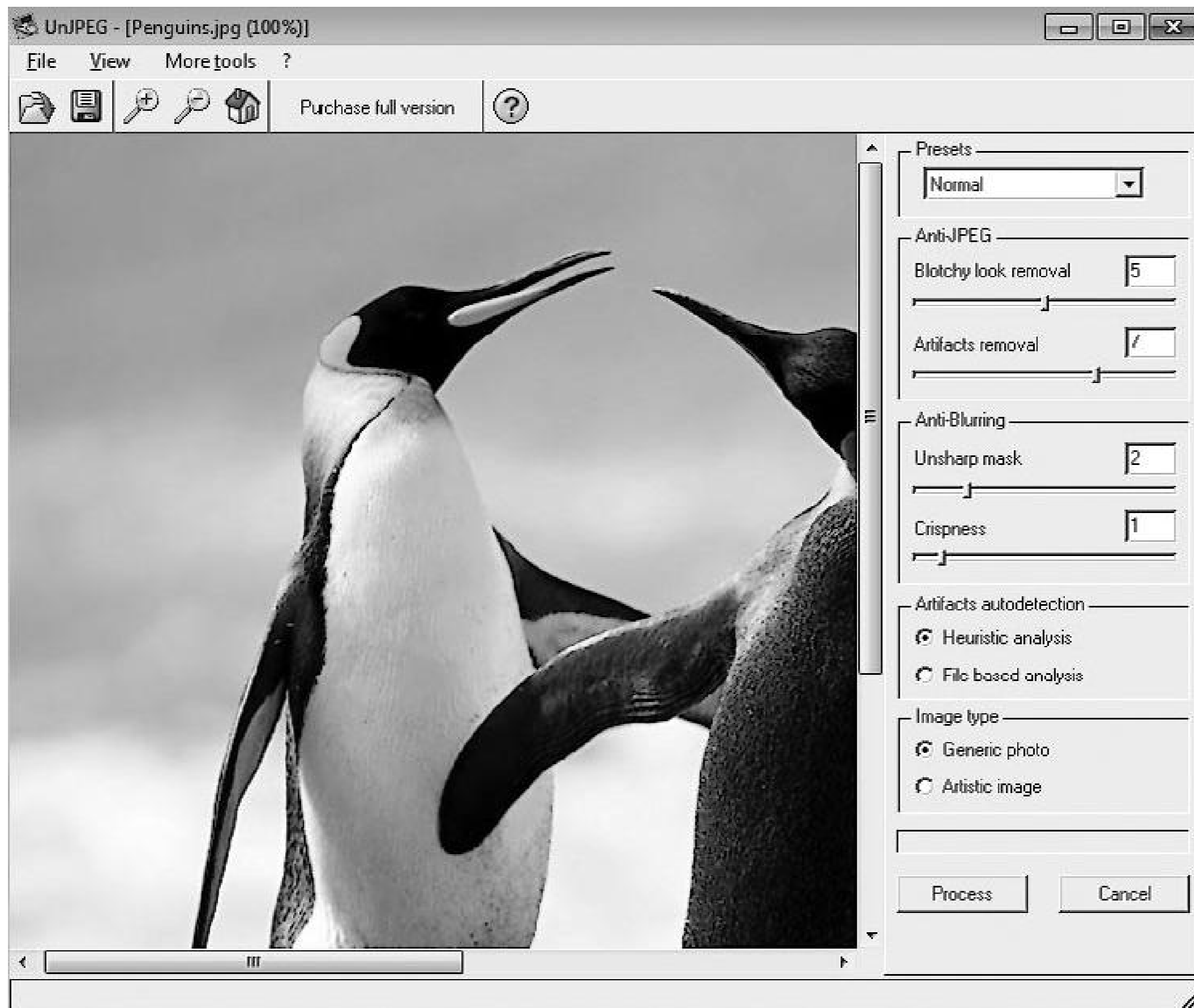
Рис. 11.14. Окно программы
