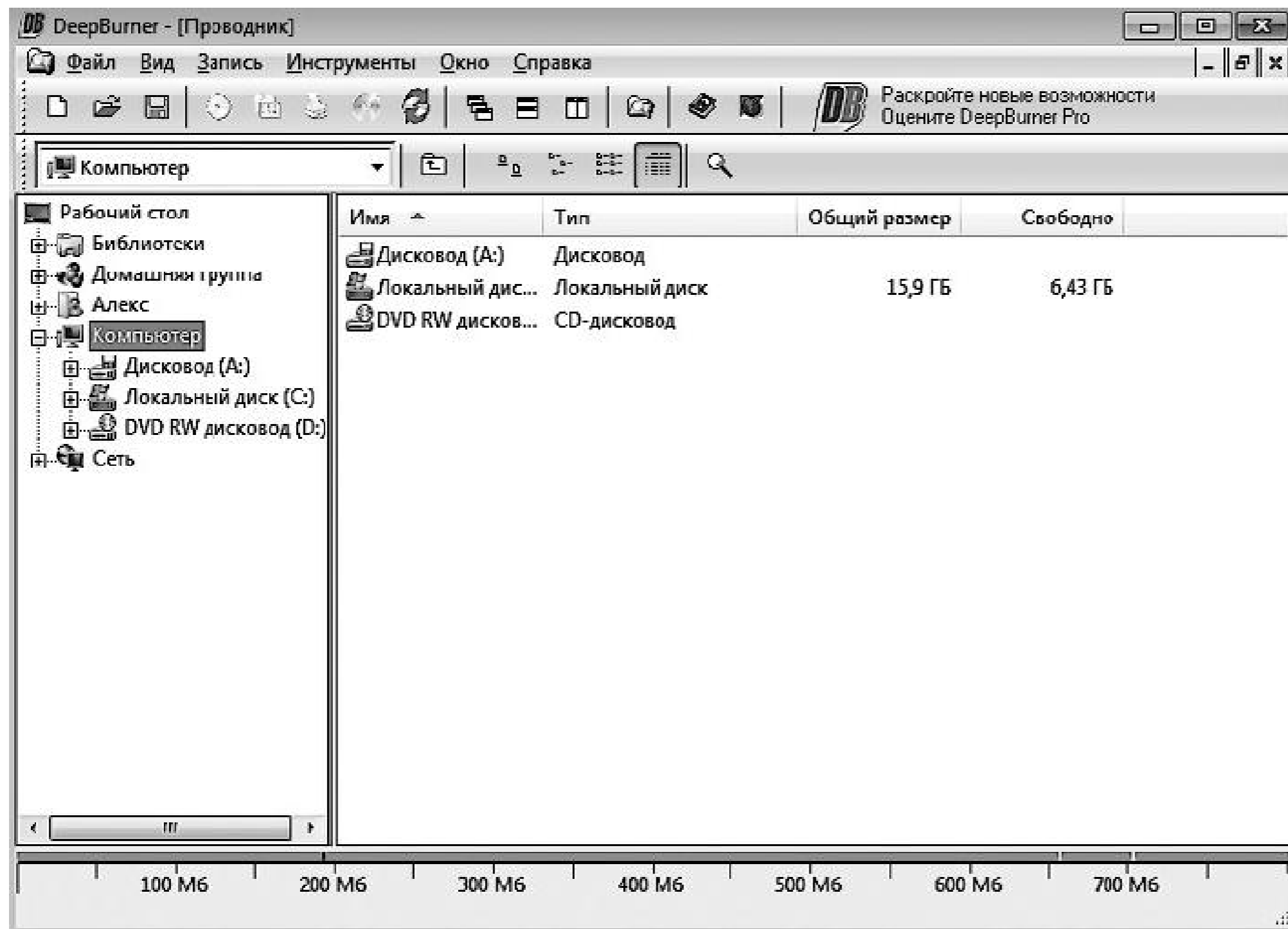
Рис. 6.4. Окно программы
