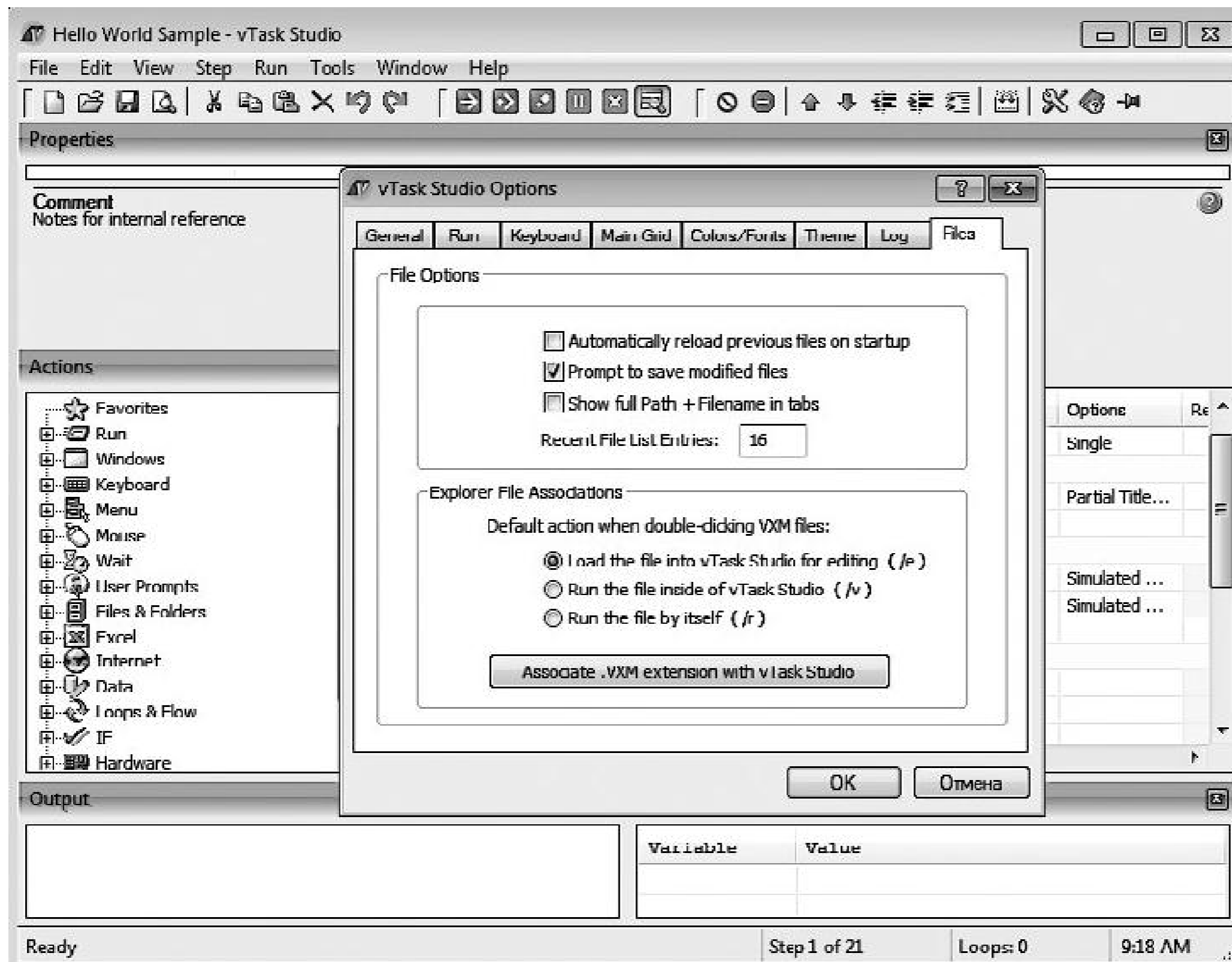
Рис. 1.35. Программа vTask
