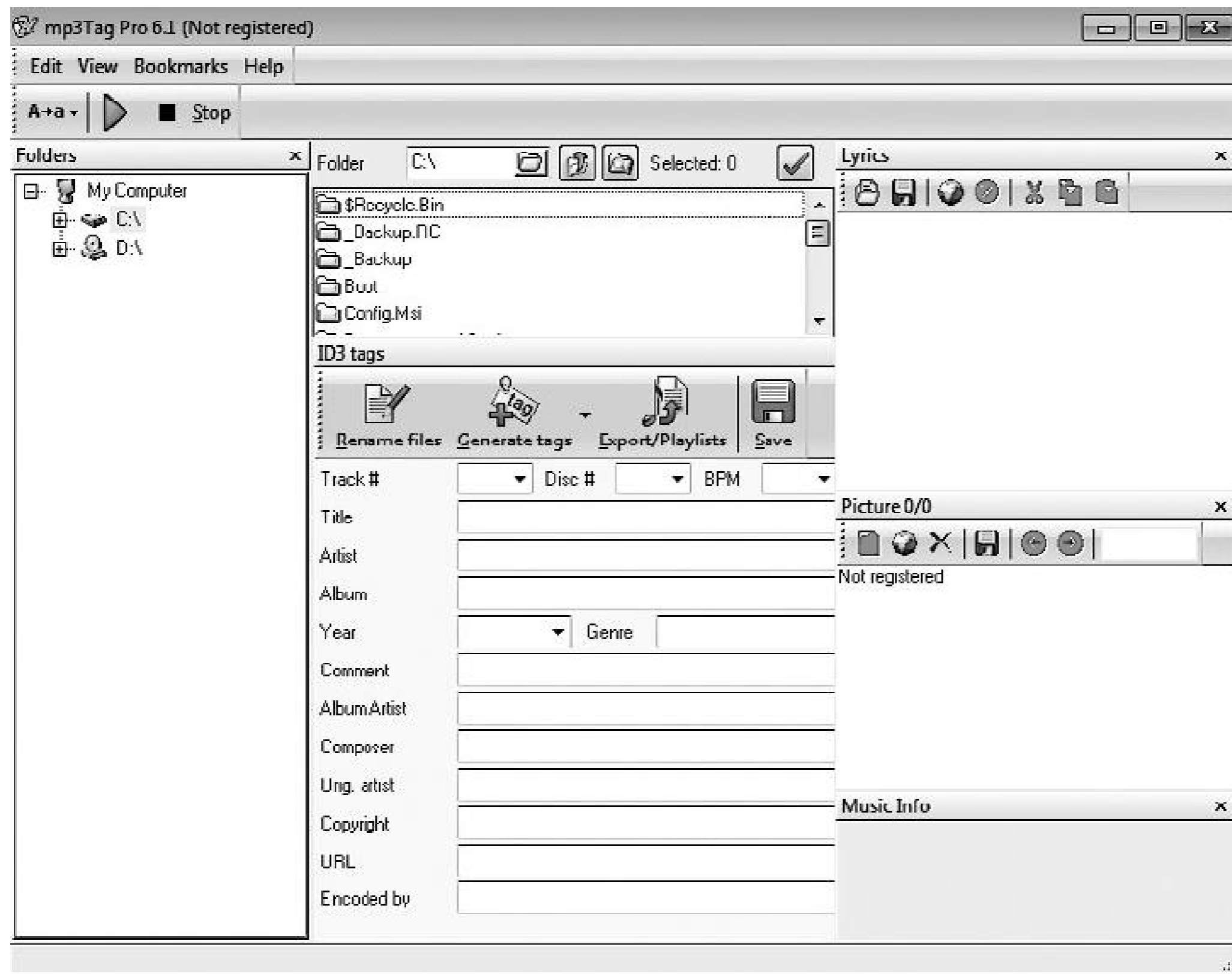
mp3Tag Pro
