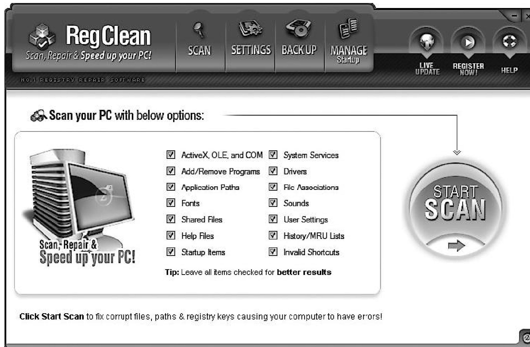
Рис. 1.21. Утилита RegClean
