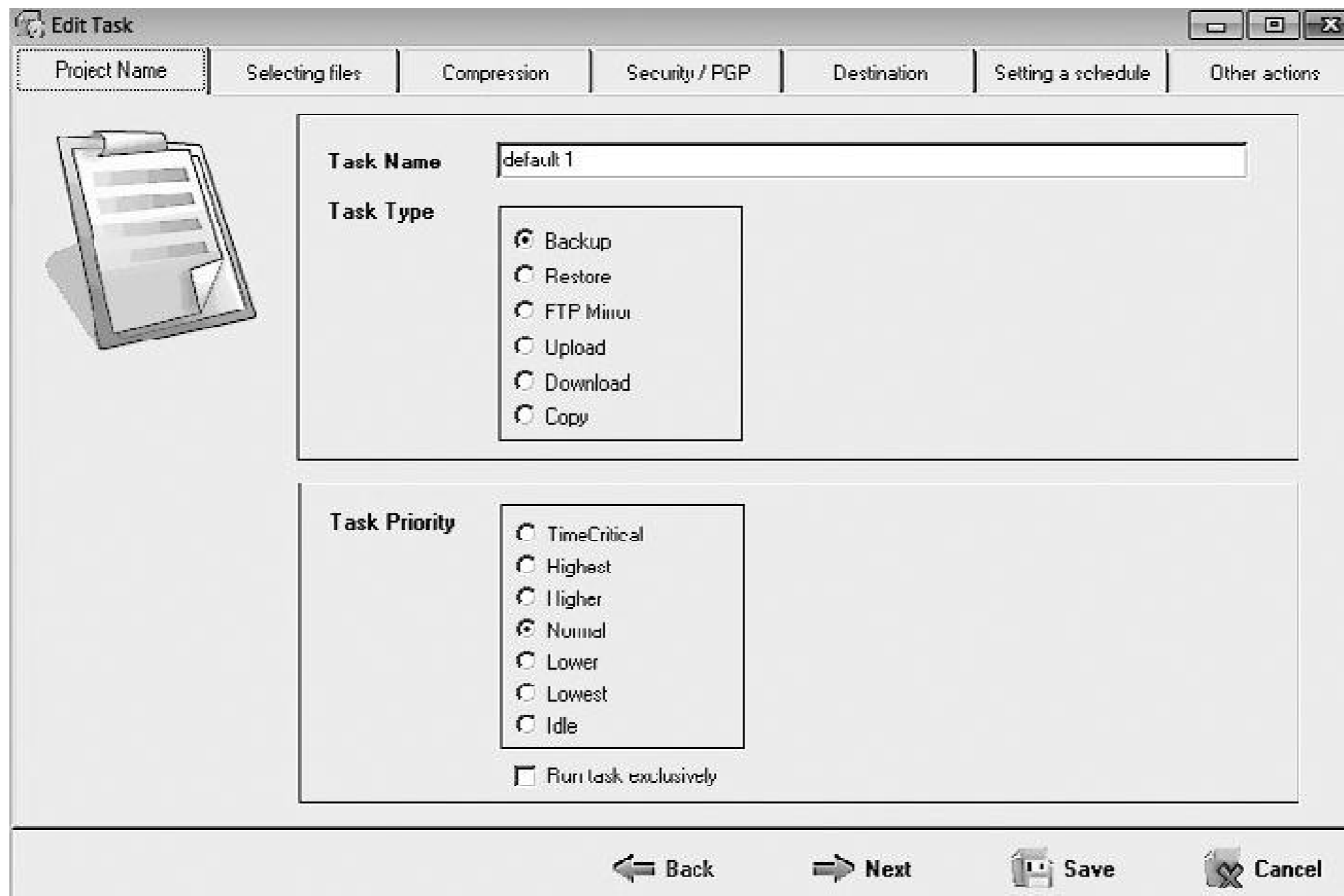
Рис. 4.6. Планировщик заданий
