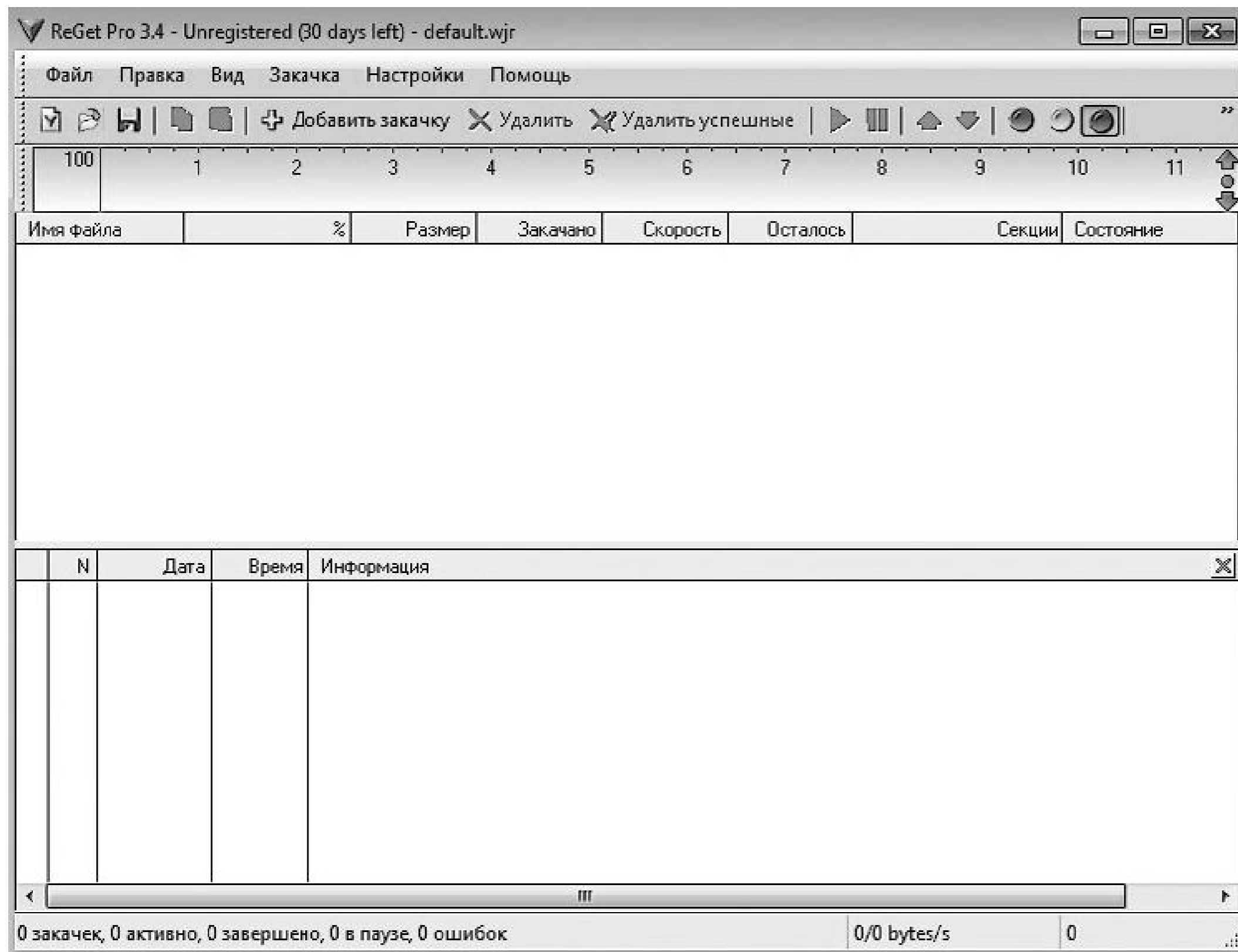
Рис. 8.5. Окно программы
