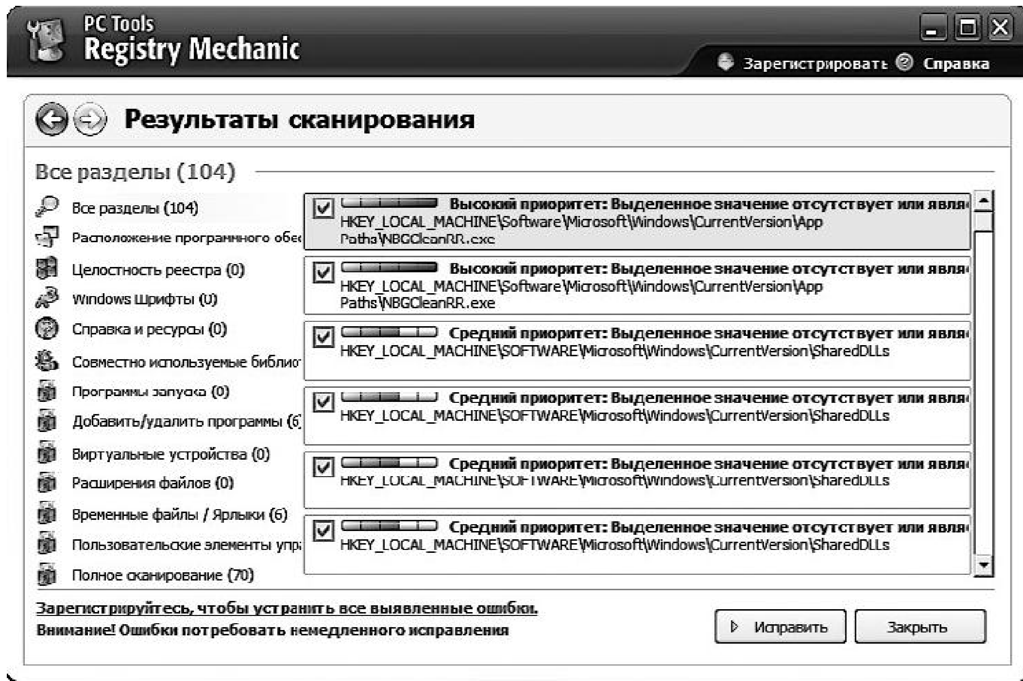
Рис. 1.22. Отчет программы
