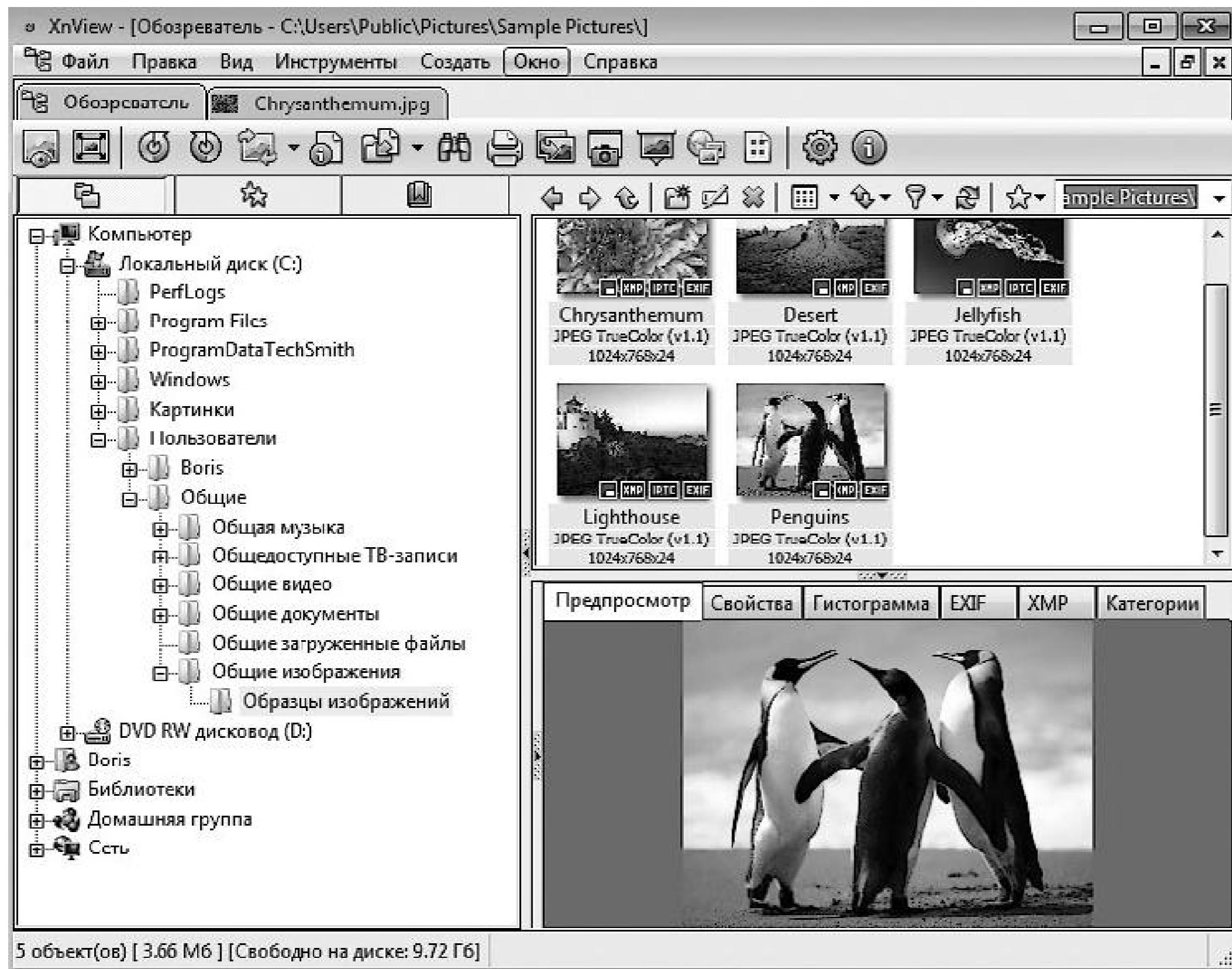
Рис. 11.5. Окно приложения
