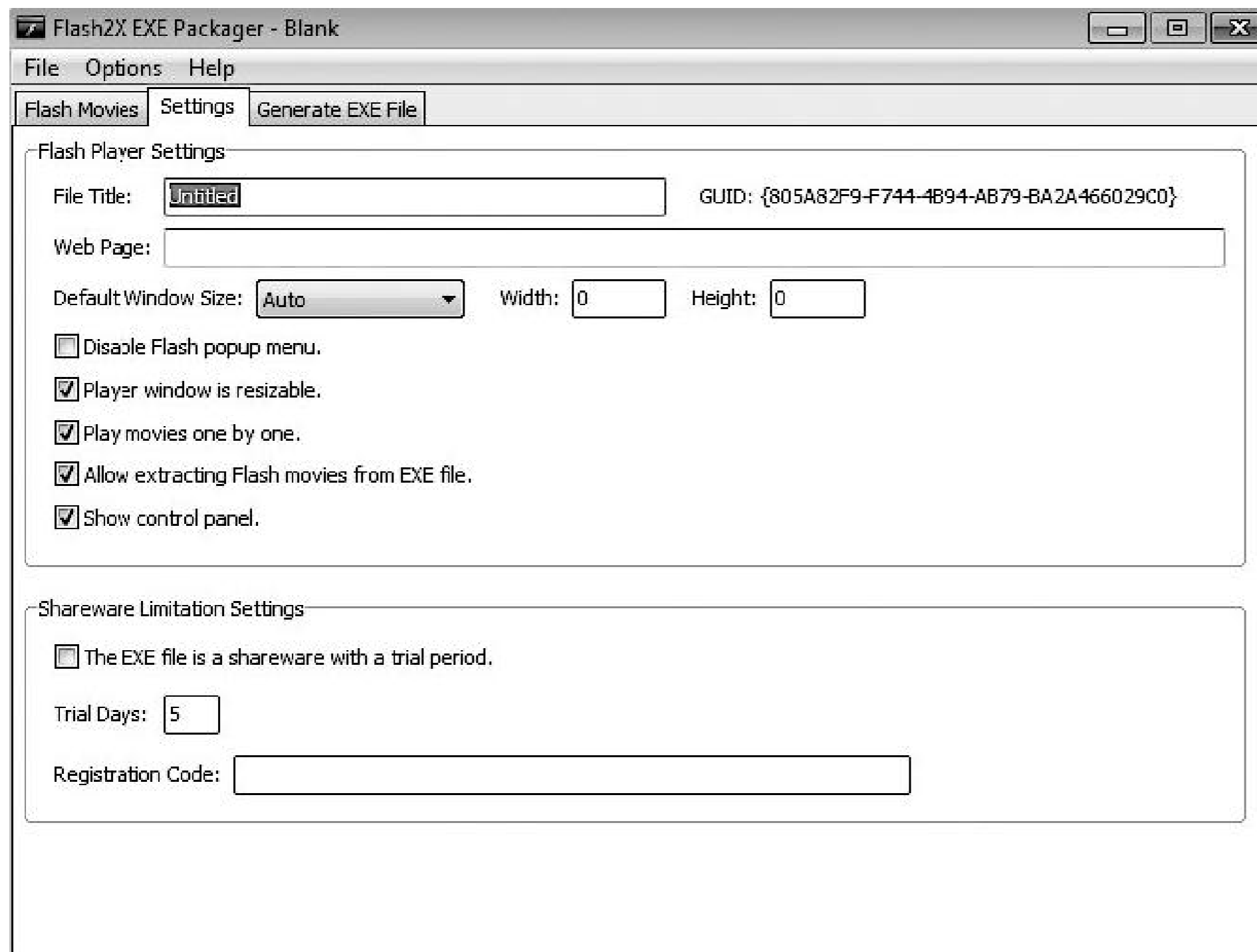
Рис. 12.14. Интерфейс программы
