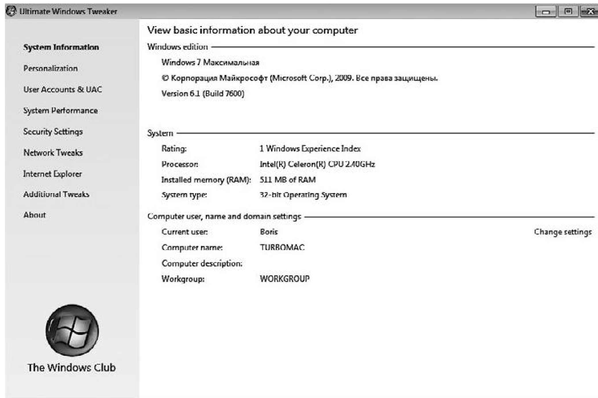
Рис. 1.17. Окно программы
