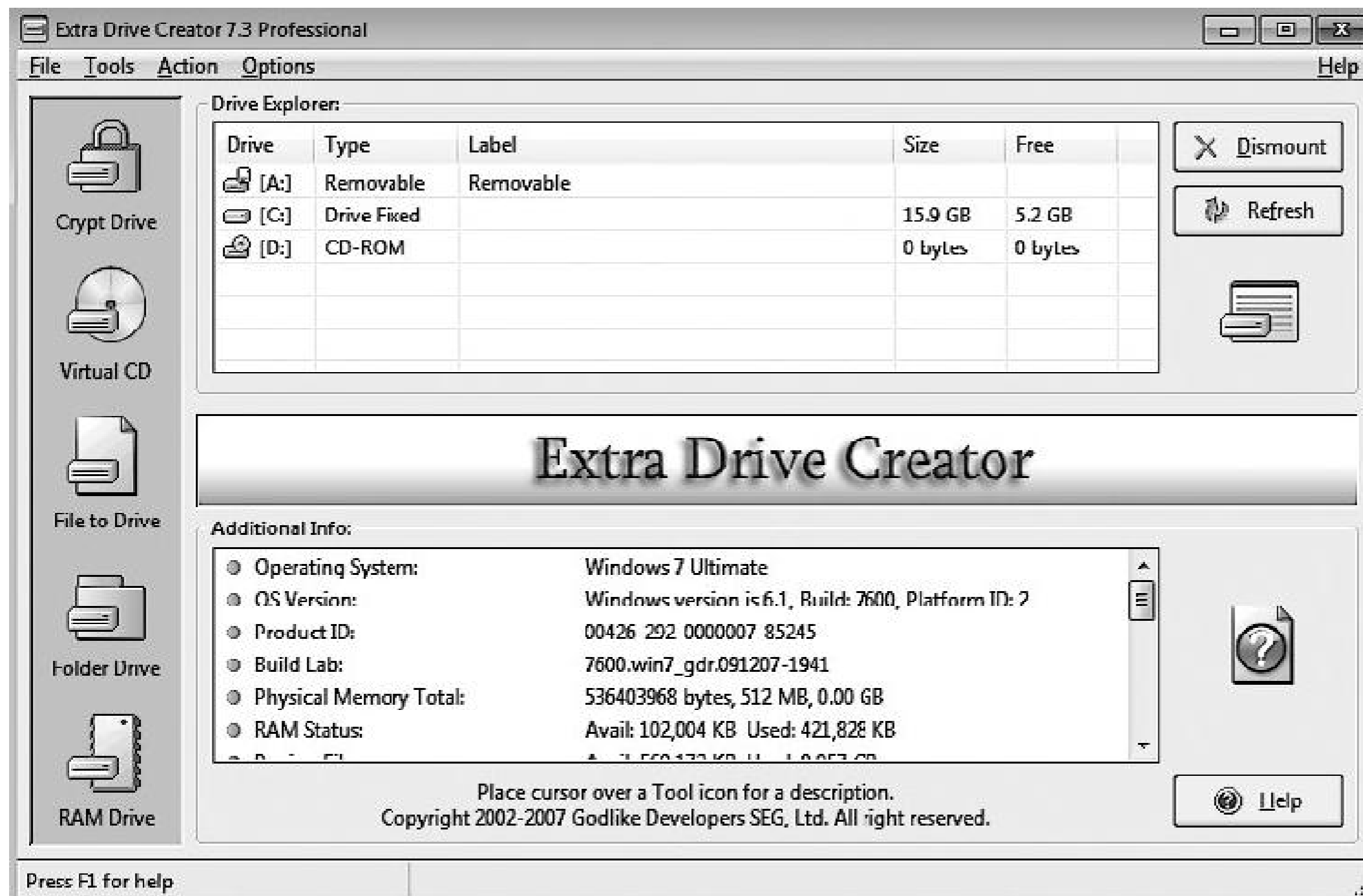
Рис. 6.1. Окно программы
