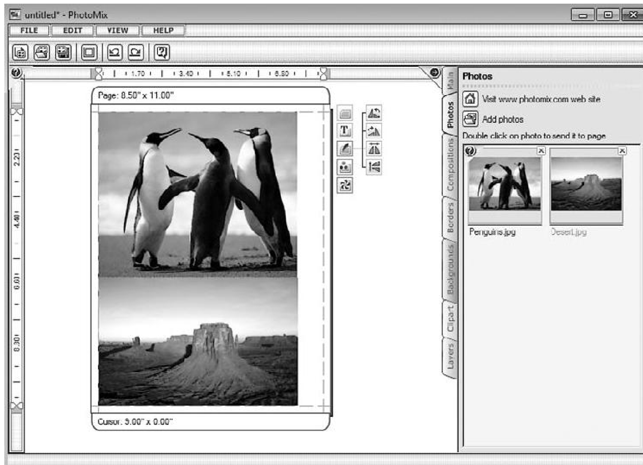
программы PhotoMix
