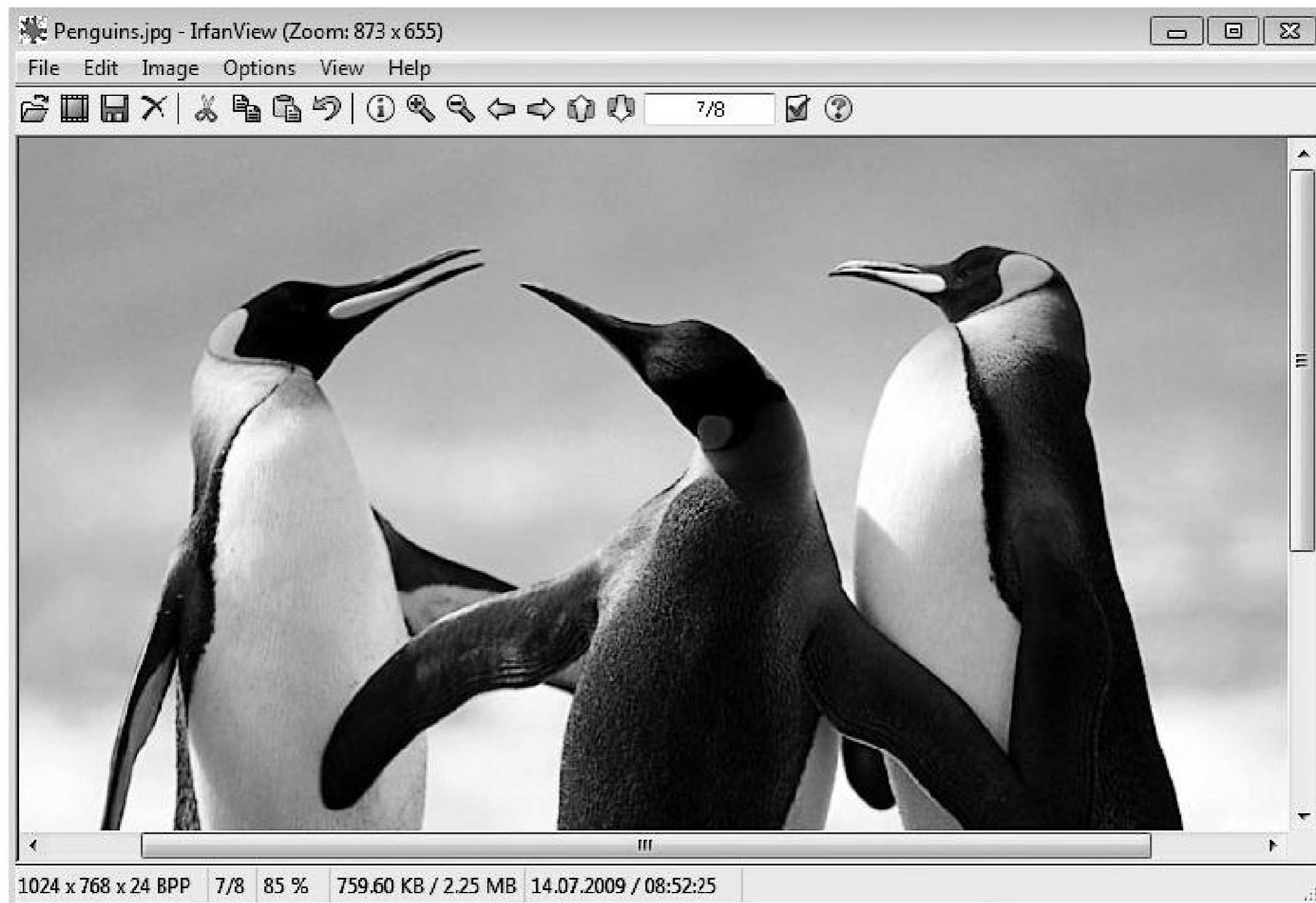
IrfanView
