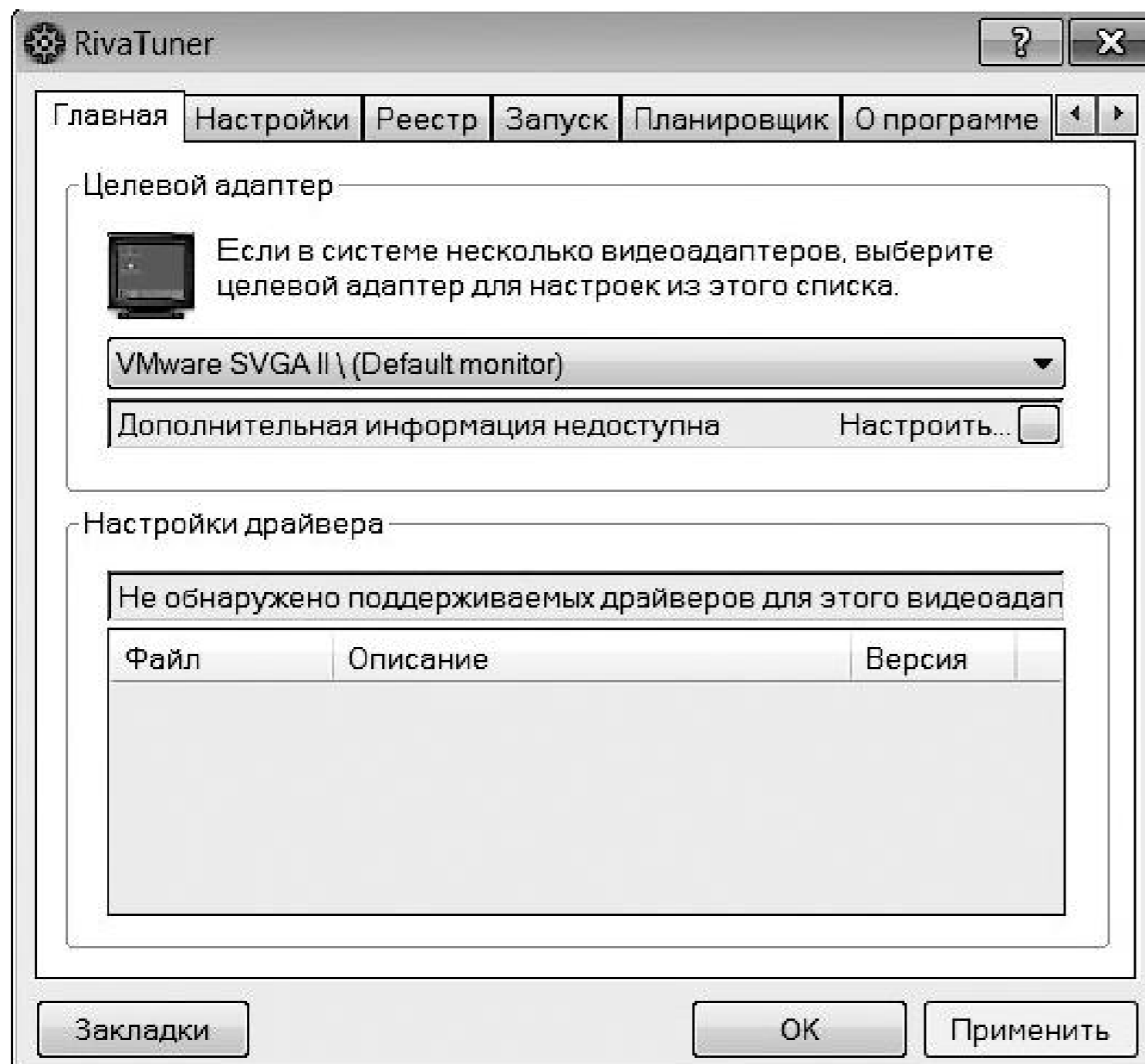
Рис. 1.12. Программа RivaTuner
