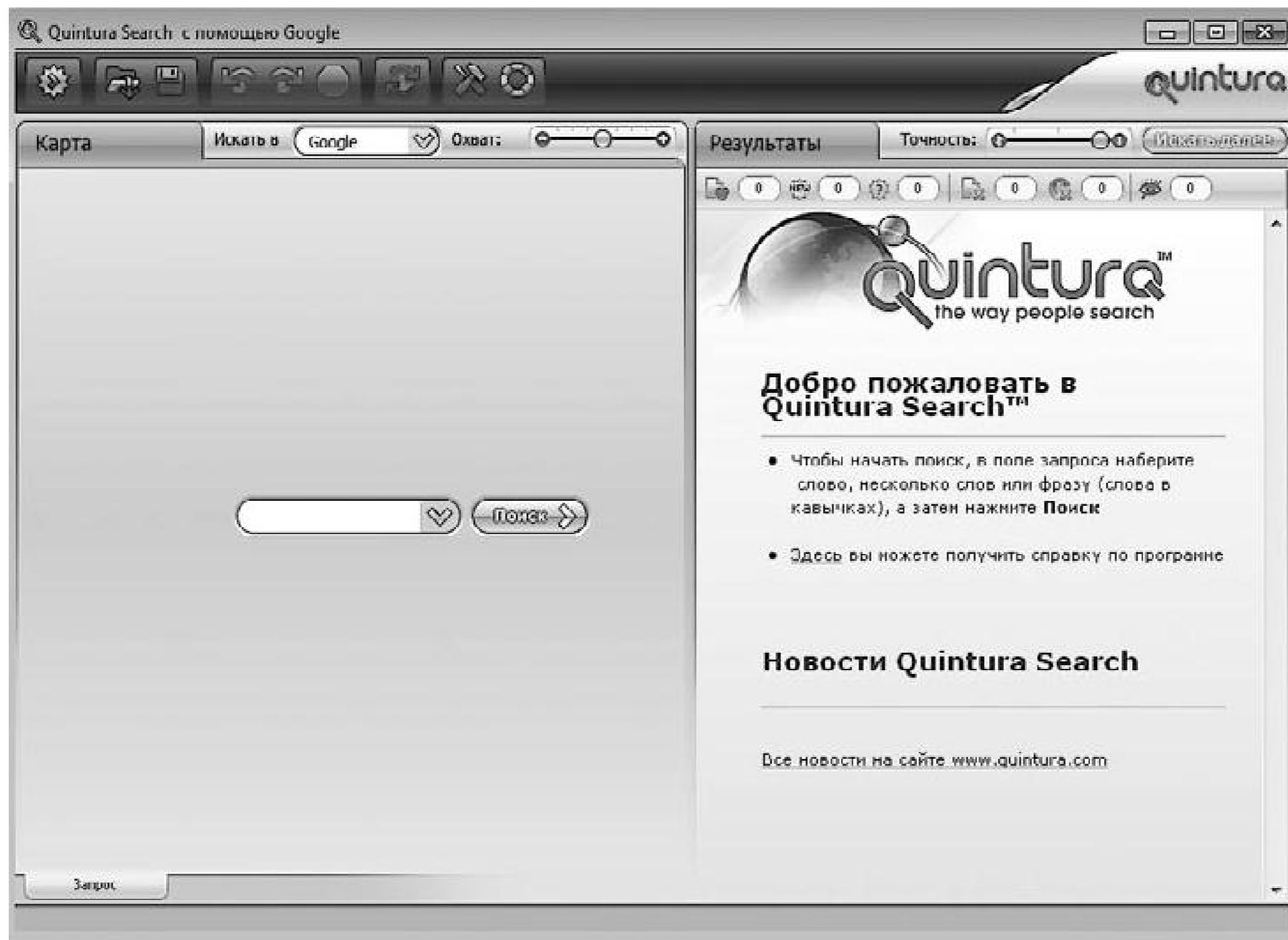
Рис. 10.3. Окно программы
