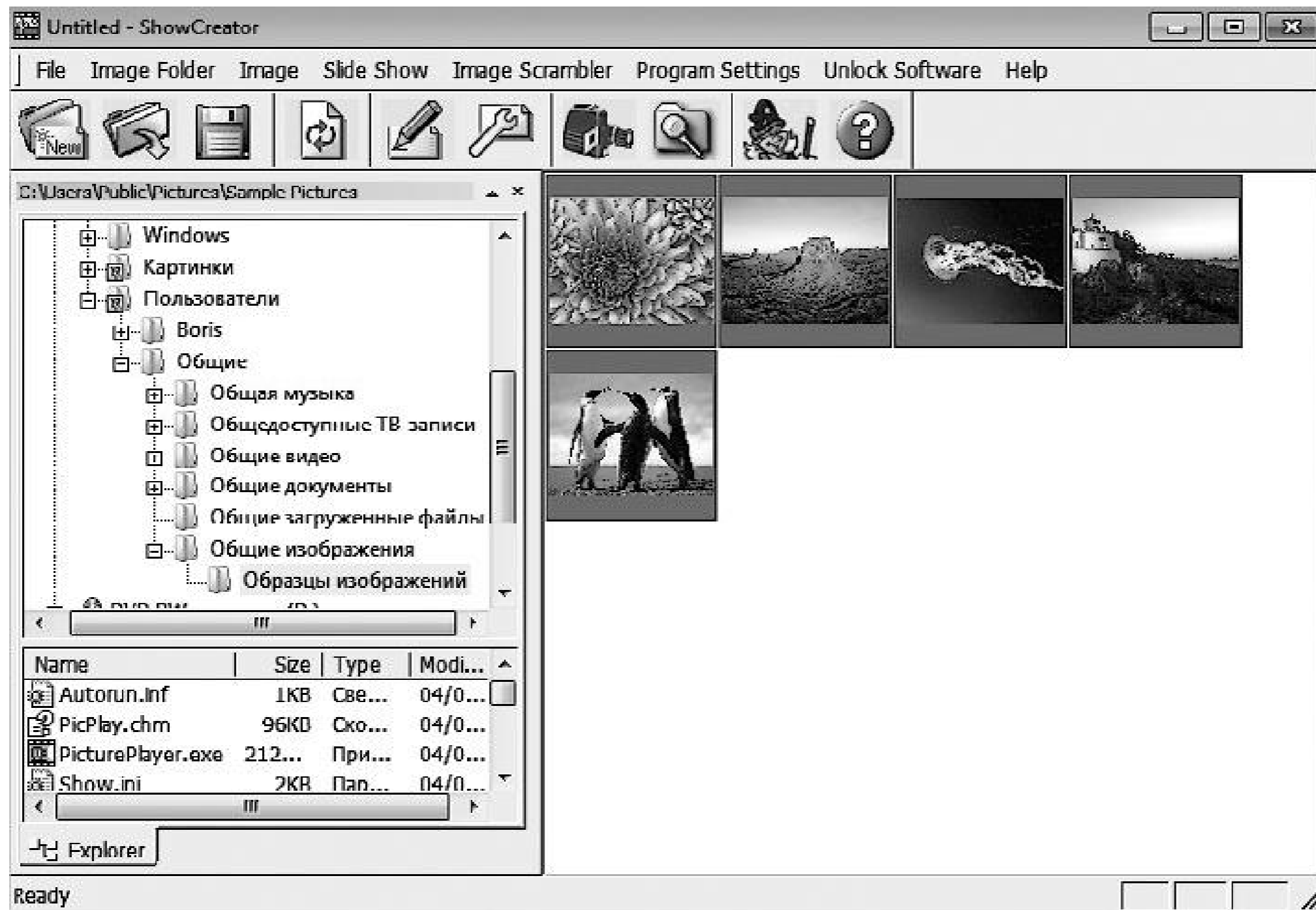
Рис. 11.19. Окно ShowCreator
