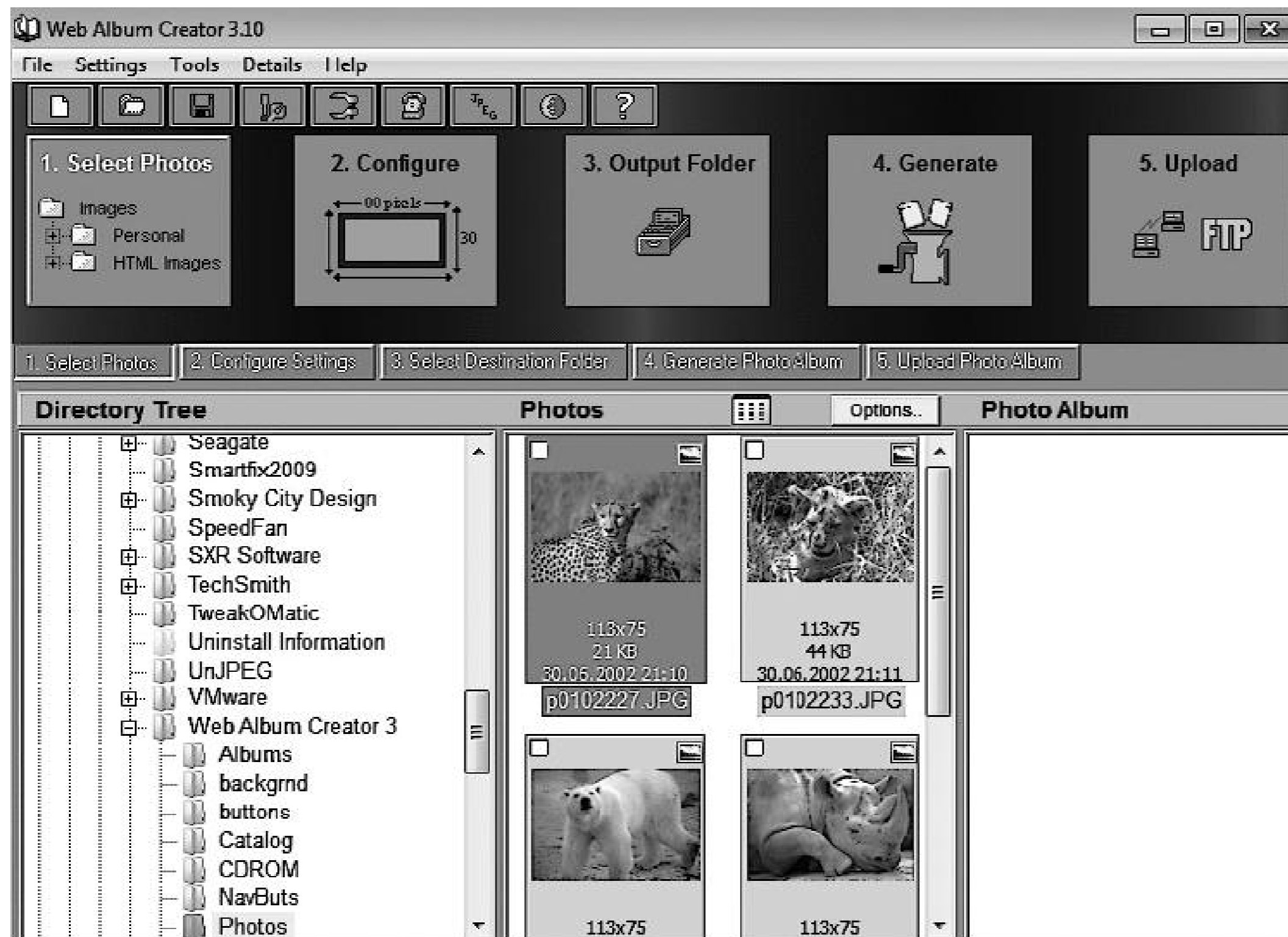
Рис. 11.25. Окно программы
