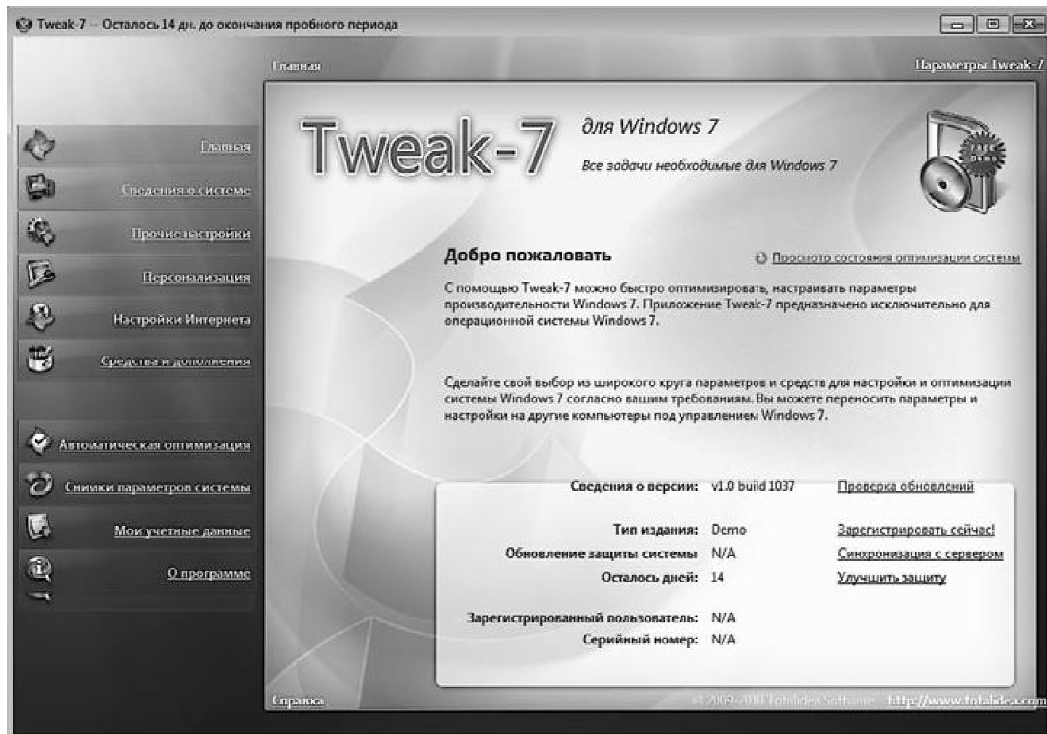
Рис. 1.18. Окно программы
