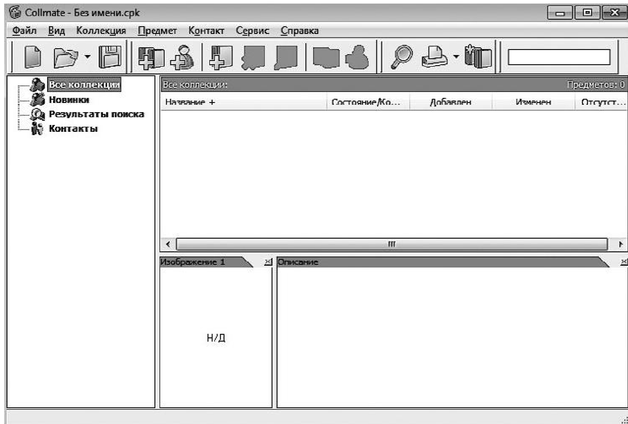
Рис. 6.14. Окно программы
