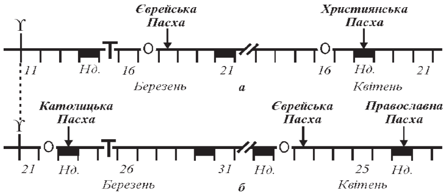
Рис. 29. Обчислення дати Пасхи за місячно-сонячним календарем у проекції на юліанський (а) і григоріанський (б) календарі наприкінці XVI ст.
