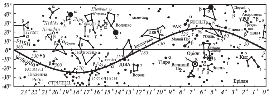
Рис 26. Карта зоряного неба з проставленими уздовж екліптики довготами
