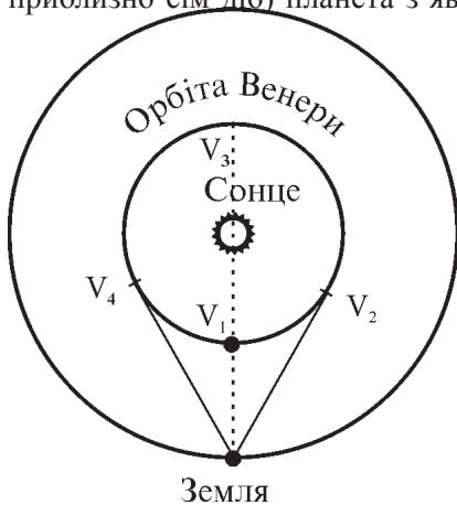
Рис. 19. Конфігурації нижньої планети
