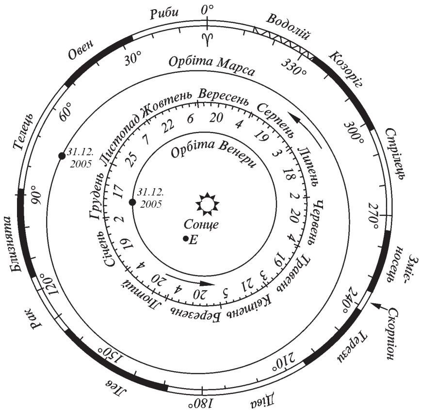
Рис 25. Орбіти Венери, Землі й Марса (вказано положення Венери і Марса на орбіті на 31 грудня 2005 р. Для більшої точності добове переміщення Марса слід вважати рівномірним відносно точки E)
