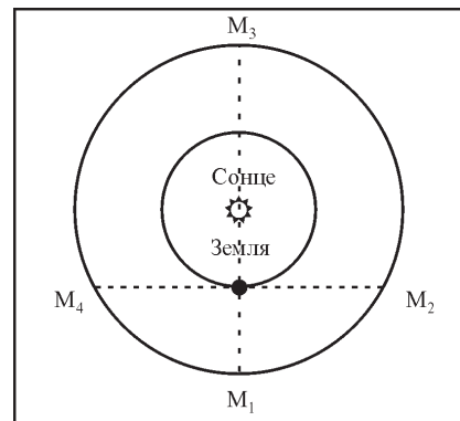
Рис. 21. Конфігурації верхньої планети
