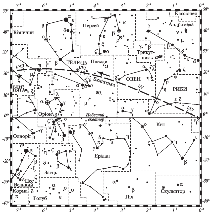
Рис. 7. Сузір'я зимового неба.
