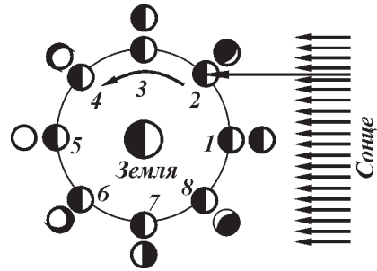
Рис. 14. Конфігурації і фази Місяця: 1 – сполучення Місяця з Сонцем (кон'юнкція), новий місяць; 3 – східна квадратура, перша чверть; 5 – протистояння Місяця і Сонця, повний Місяць (повня); 7 – західна квадратура, третя
