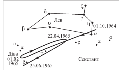
Рис. 18. Видимий рух планети Марс серед зір
