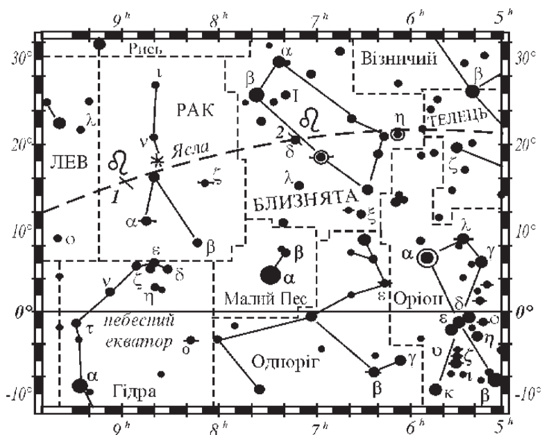
Рис. 17. Положення висхідного вузла місячної орбіти 22 січня (1)
