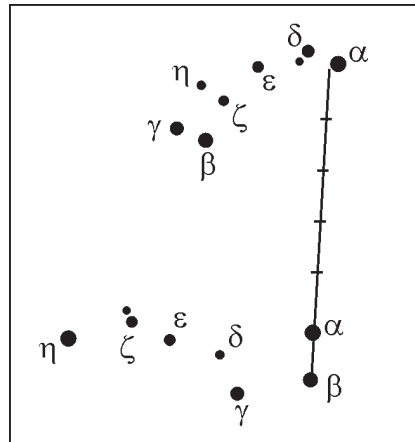
Рис. 3. Спосіб знаходження Полярної зорі
