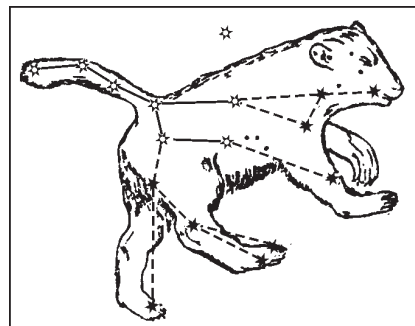
Рис. 4. Зображення Великої Ведмедиці у давньому атласі
