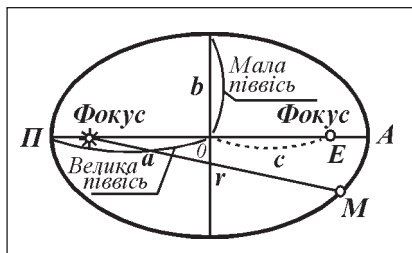
Рис. 24. Еліпс як орбіта планети: П – перигелій, А – афелій – відповідно найближча і найдалша від Сонця точки орбіти, r – радіус-вектор планети М
