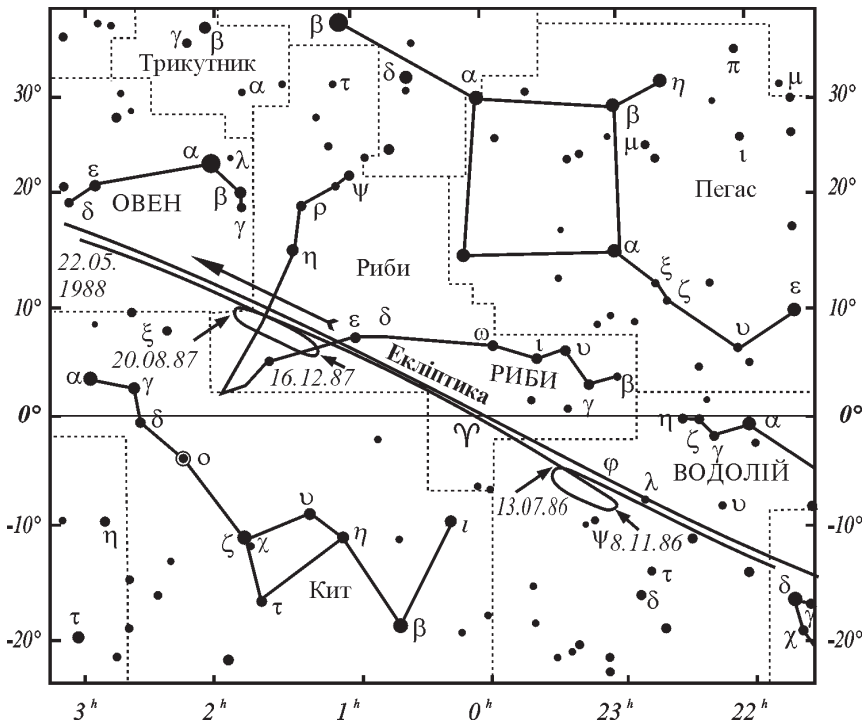
Рис. 23. Дві петлі, що їх описав Юпітер серед зір 1986–1987 рр.
