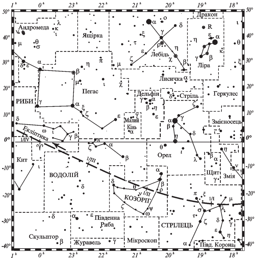
Рис. 6. Осіннє вечірнє небо
