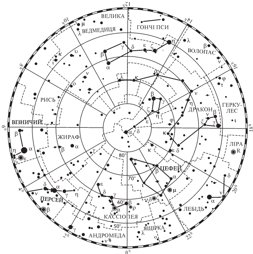
Рис. 1. В околі Північного полюса
