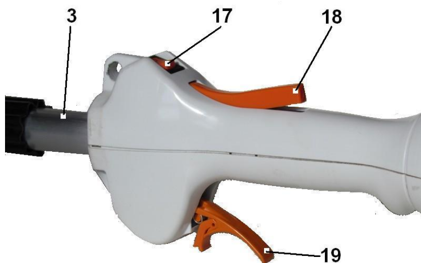
Рис. 2.1.г. Пульт управління комбідвигуном
