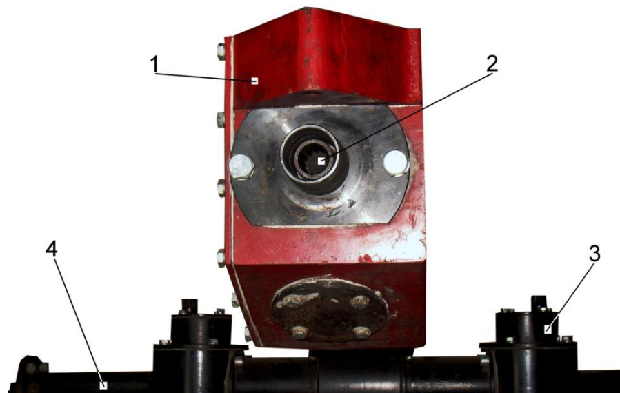
Рис. 3.12. Механізм з'єднувальний косарки роторної «Мотор Січ КРН-1С»
