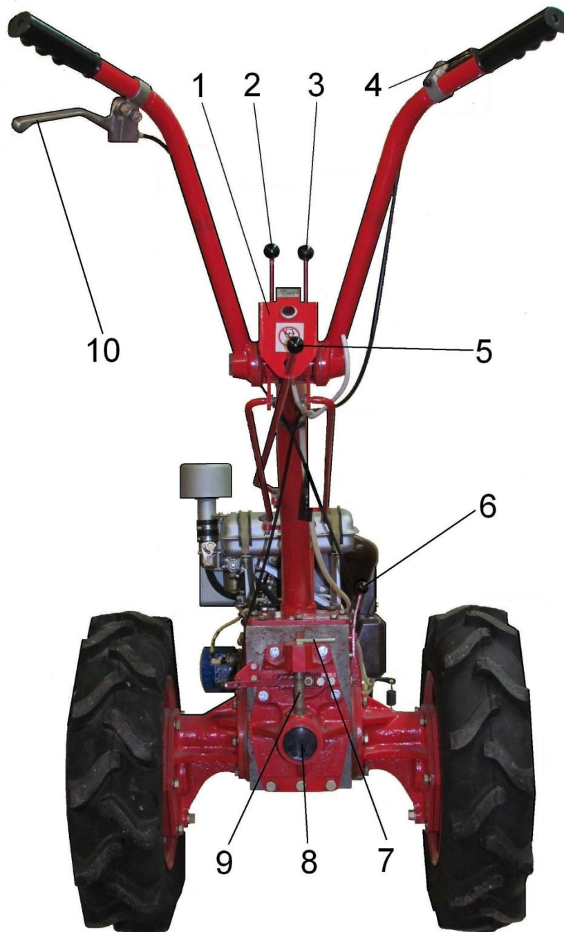
Рис. 1.2. Мотоблок «Мотор Січ МБ–4,5» (вид ззаду)
