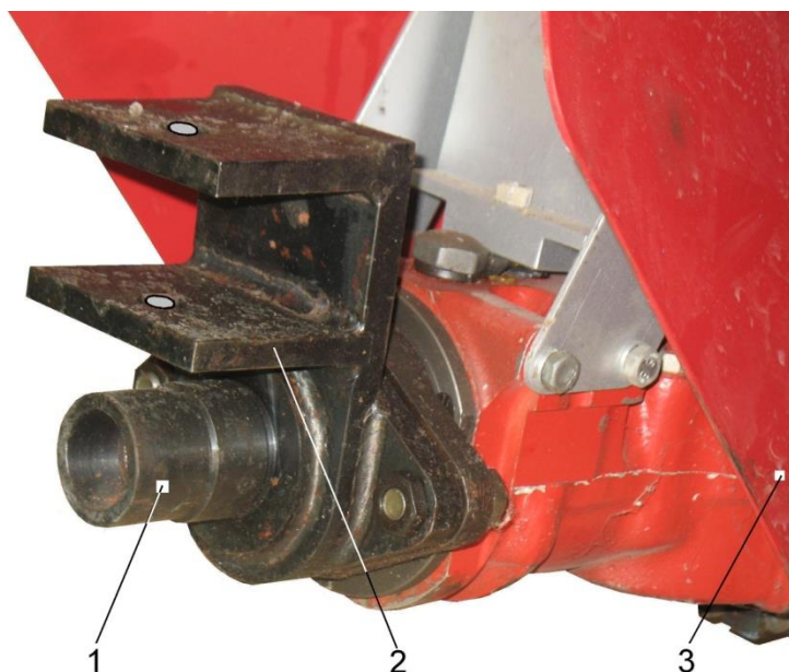
Рис. 3.7. Механізм з'єднувальний косарки сегментної
