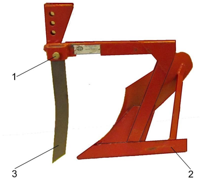
Рис. 2.6. Плуг ПН–1 (вид збоку)
