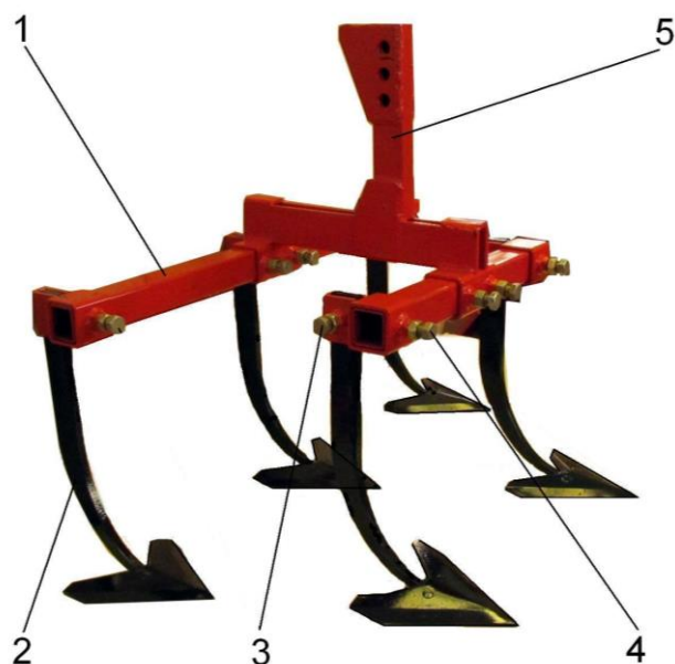
Рис. 2.14. Рама навісна універсальна «Мотор Січ РНУ-1В» із стрілочастими плоскоріжущими лапами
