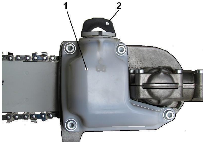
Рис. 5.12. Положення відкидного хомутика запірною бачка масляного
