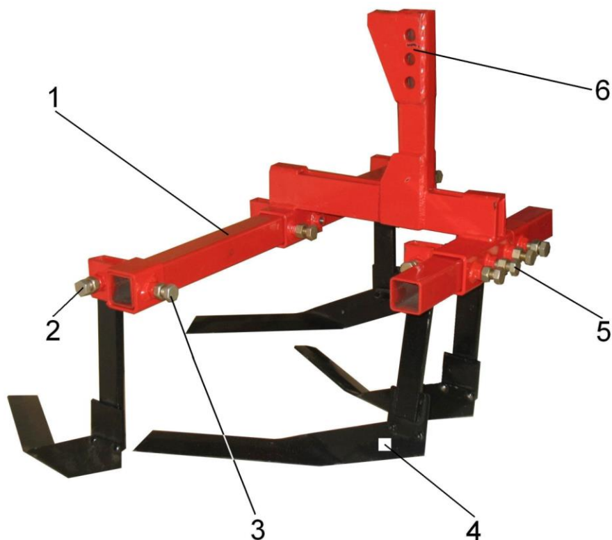
Рис. 2.16. Рама навісна універсальна «Мотор Січ РНУ–1В» із однобічними плоскоріжущими лапами
