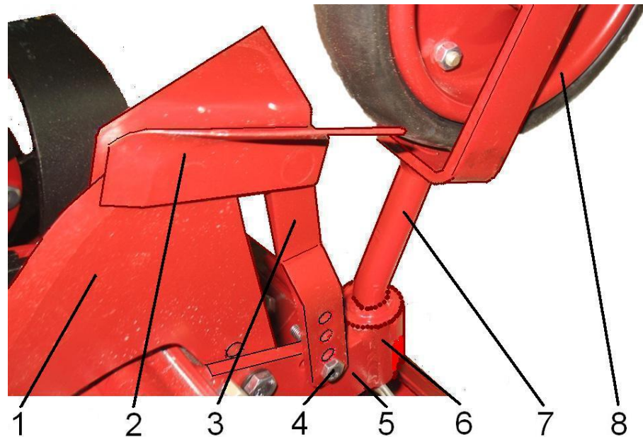
Рис. 3.3. Ніж направляючий
