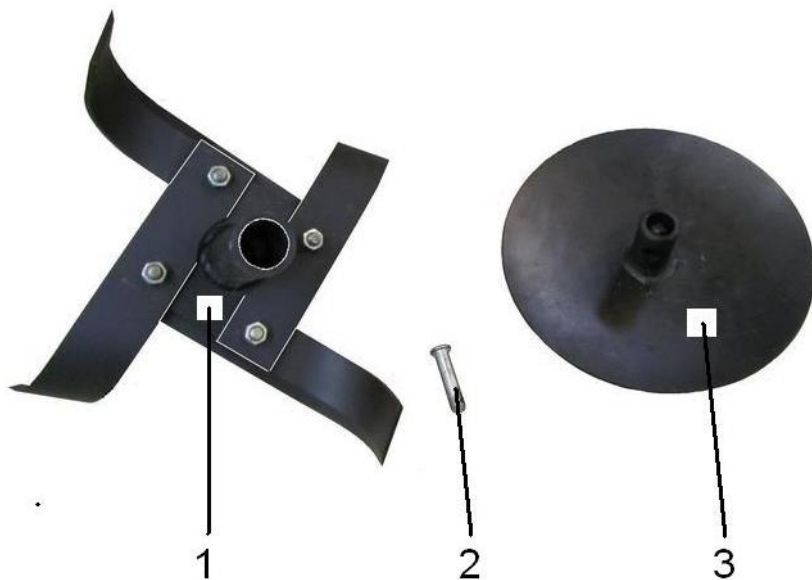
Рис. 4.4. Робочі органи мотокультиватора
