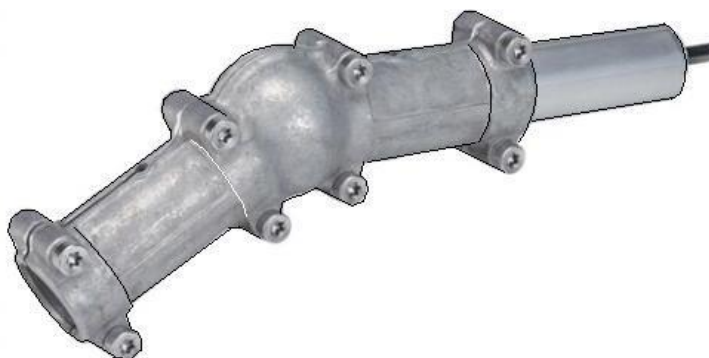
Рис. 5.21. Кутовий редуктор до висоторіза
