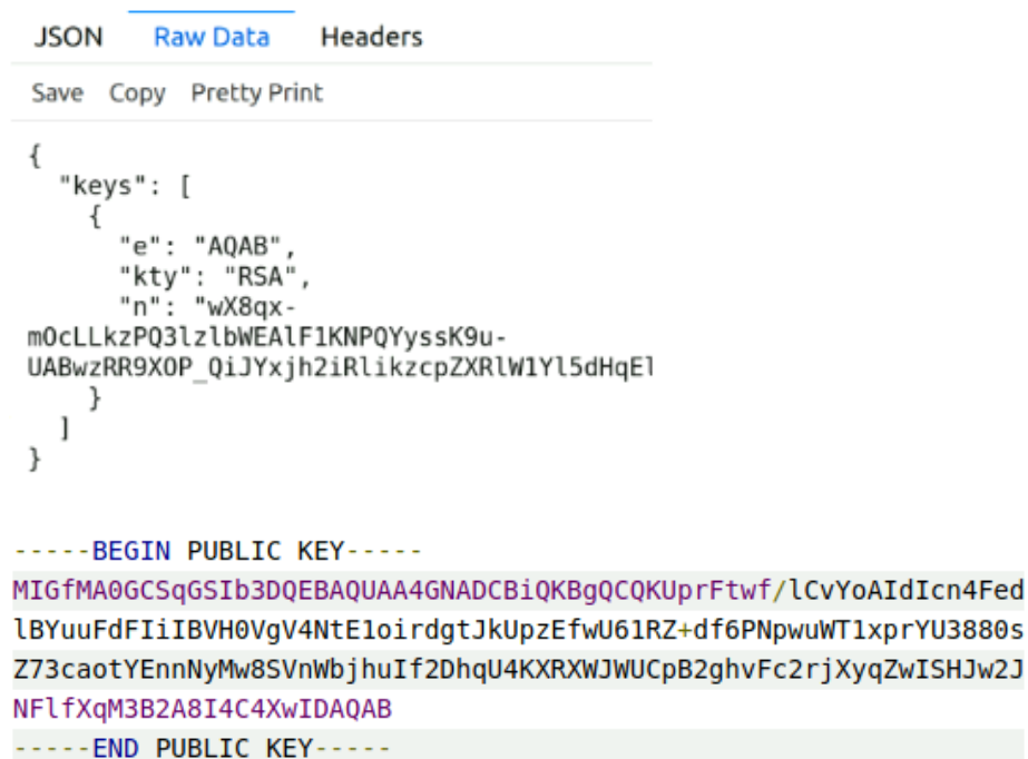
Рис. 2.4 Приклады JWK
