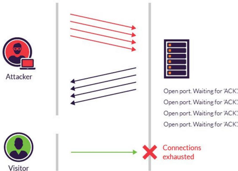
Рис. 4.6 SYN-флуд
