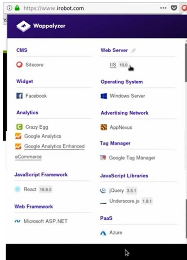
Рис. 6.6 Wappalyzer
