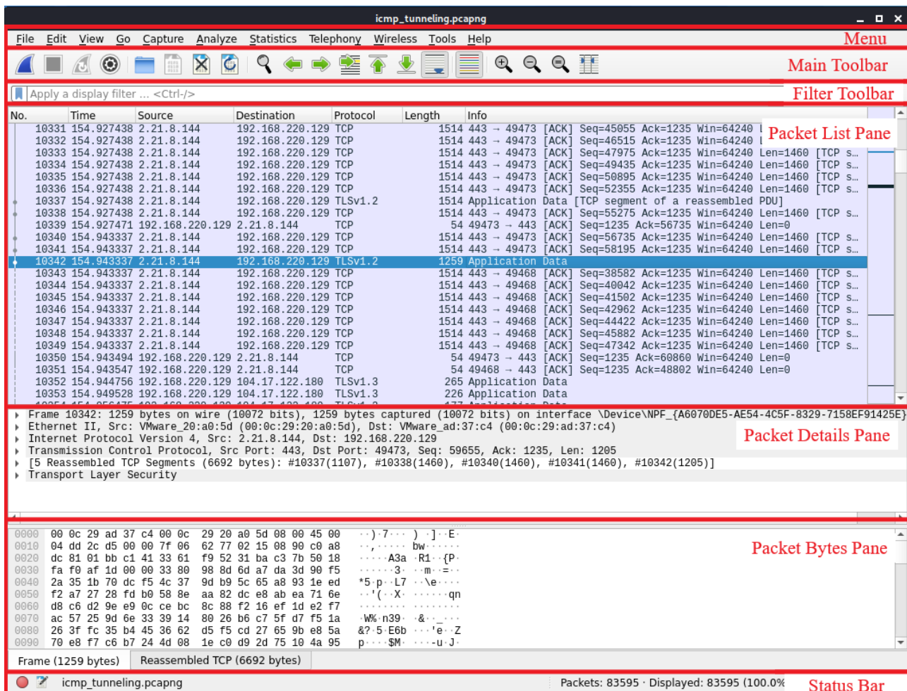
Рис. 6.39 Wireshark
