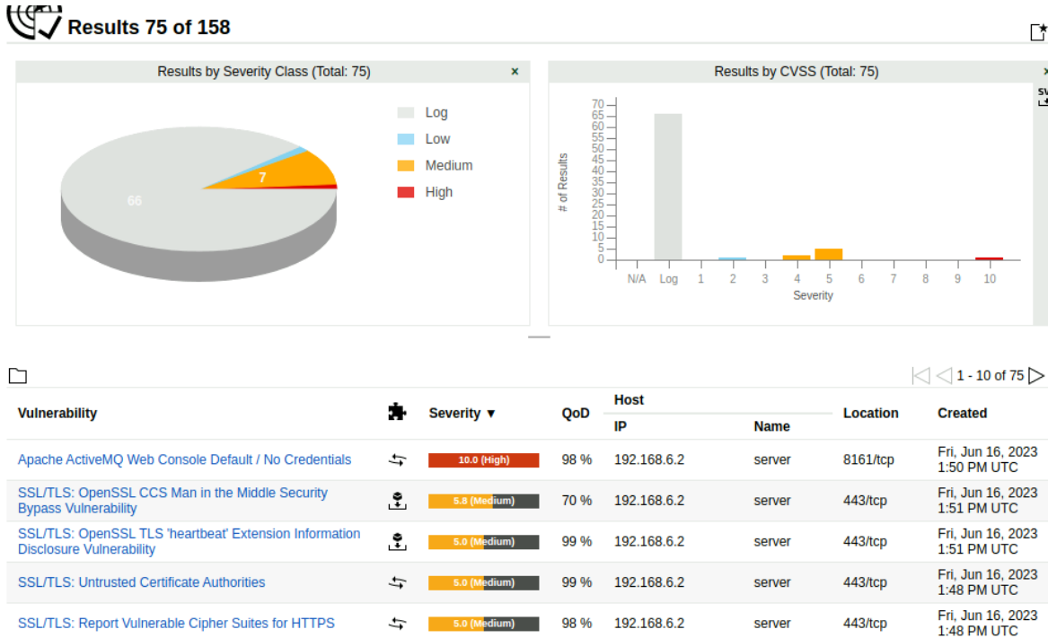
Рис. 6.18 Результати сканування в Greenbone OpenVAS
