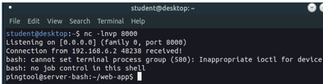
Рис. 6.45 Прослуховування порту за допомогою Netcat
