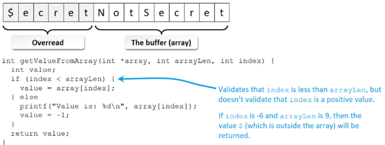
Рис. 7.12 Зчитування поза межами буфера
