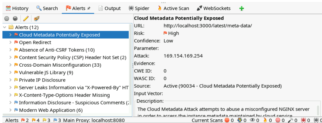
Рис. 7.16 Результати динамічного аналізу з допомогою OWASP ZAP
