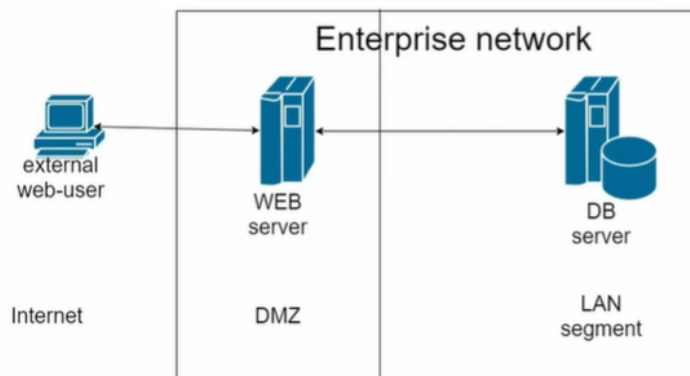
Рис. 1.1 Клієнт-серверна архітектура 1
