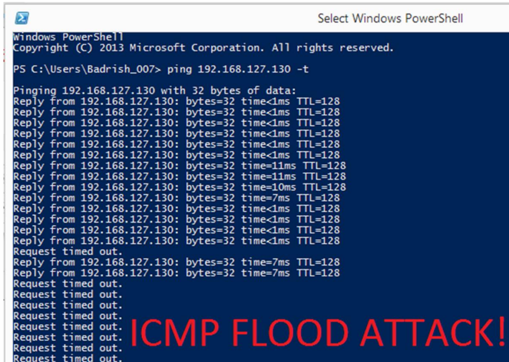
Рис. 4.2 ISMP-флуд
