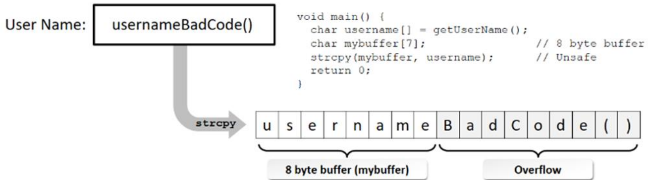
Рис. 7.11 Переповнення буфера
