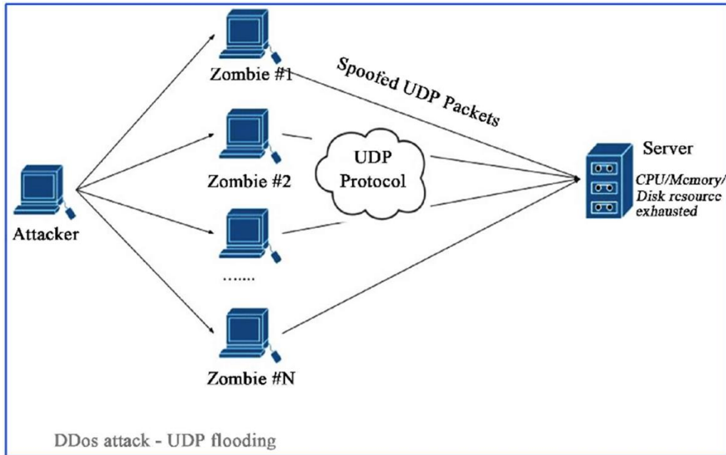
Рис. 4.4 UDP-флуд
