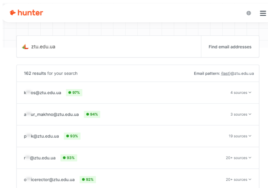
Рис. 6.4 Hunter.io
