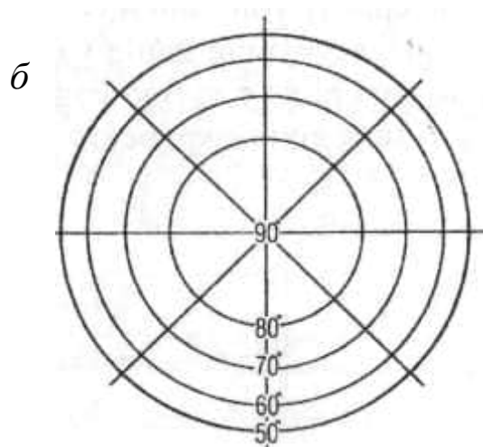
Рис. 37. Нормальні (прямі) азимутальні проекції: a – рівнопроміжна; б – рівновелика; в – рівнокутова
