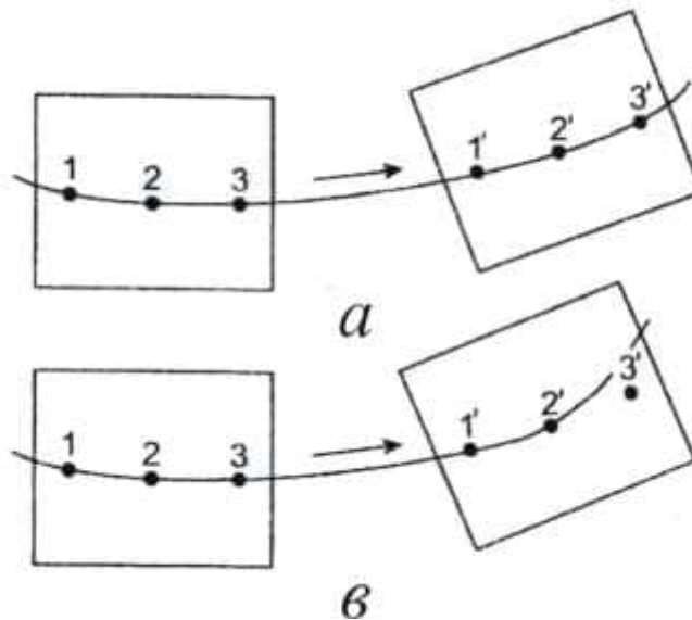
Рис. 38. Визначення вигляду лінії меридіана чи паралелі:
