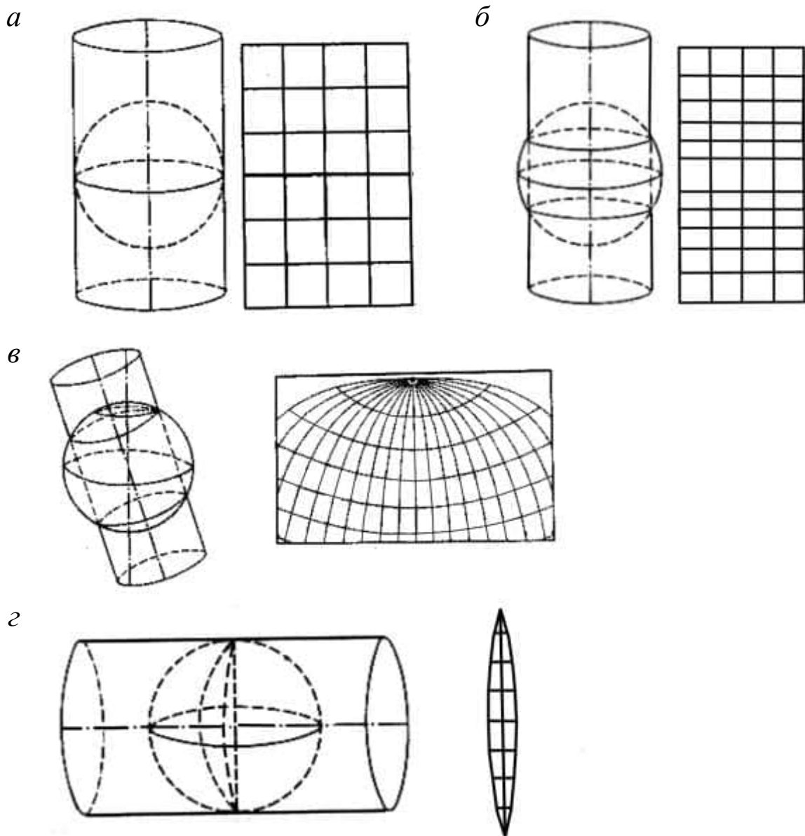
Рис. 2. Циліндричні проєкції: а – нормальна циліндрична проєкція на дотичний циліндр; б – нормальна циліндрична проєкція на січний циліндр; в – коса циліндрична проєкція на січний циліндр; г – поперечна циліндрична проєкція на дотичний циліндр
