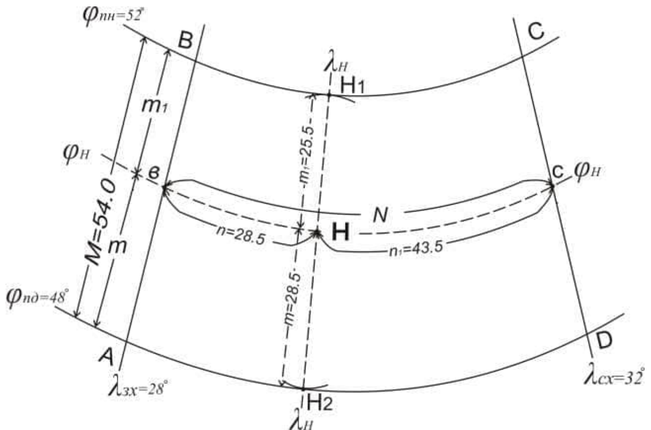
Рис. 33. Схема визначення географічних координат пункту Н
