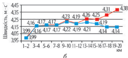
Рисунок 2.3 – Динаміка швидкості проходження дистанції у спортивній ходьбі на 20 км у чоловіків ( n = 70 ): а – чемпіонати світу 2013, 2015, 2016 рр. і кубки світу 2012, 2014 рр.; б – Ігри Олімпіад 2012 і 2016 рр. (Sovenko, 2016): —■— призери (середній результат: чемпіонати і кубки світу – 1:19.44, Ігри Олімпіад 1:19.14); —■— спортсмени, які зайняли 4–10-ті місця (середній результат: чемпіонати і кубки світу – 1:20.57, Ігри Олімпіад – 1:20.10)
