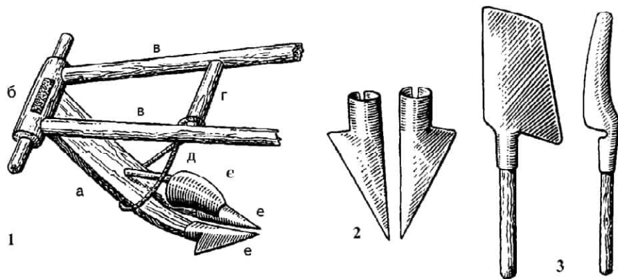
Соха російського типу:
