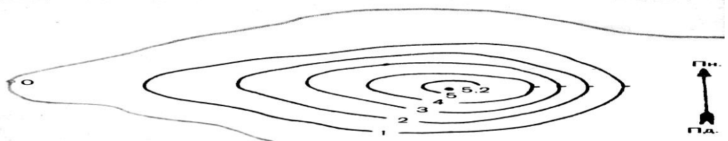
Рис. 4.12.1.Зображення горба з горизонталями і бергштрихами
