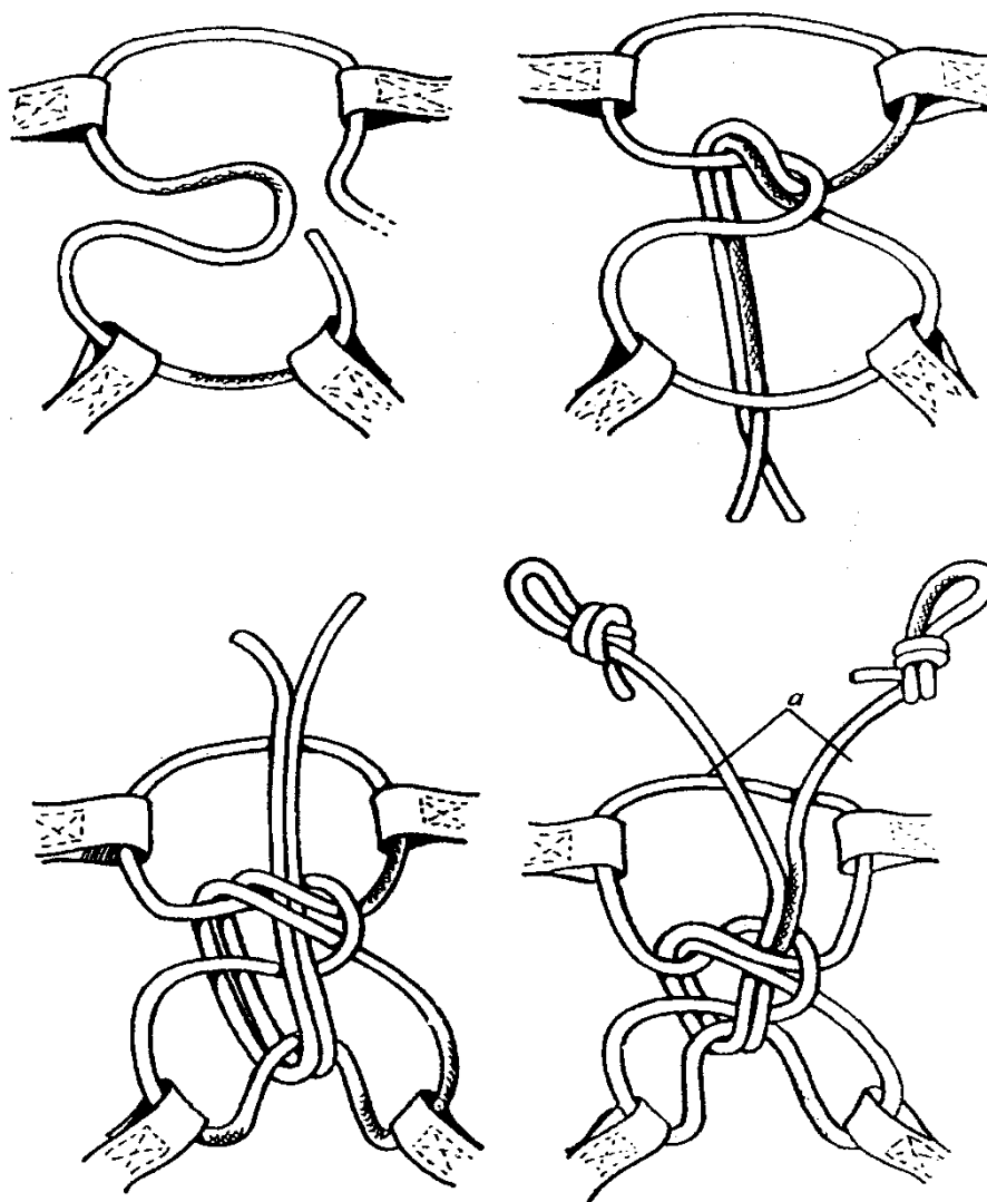
Рис. 4.11.2 Блокування страхувальної системи вузлом «подвійний булінь»; а) кінці мотузки для самострахування.
