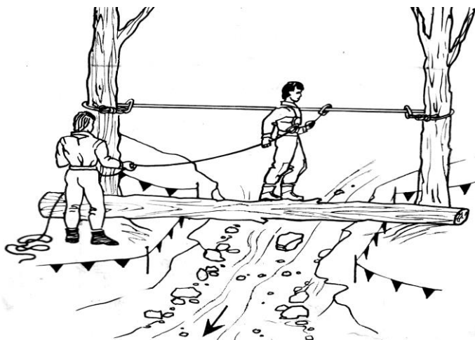
Рис. 4.11.4. Переправа по мотузці з перилами (паралельні мотузки)
