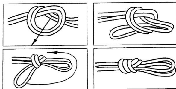
Рис. 4.8.14. В'язання подвійного провідника
