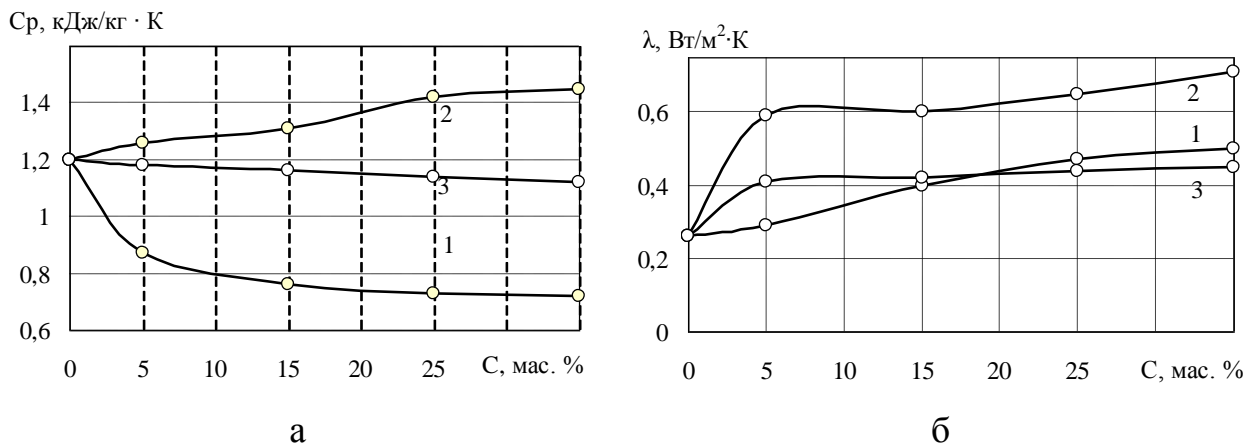
Рис. 1. Вплив вмісту вуглецевого волокна Урал (1) і органічних волокон лола (2) і терлон (3) на питому теплоємність (а) і коефіцієнт теплопровідності (б) композитів на основі пентапласту
