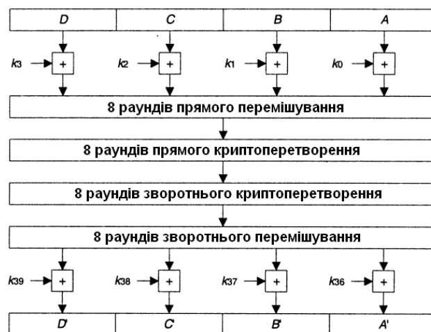
Рис. 21. Узагальнена схема алгоритму MARS
