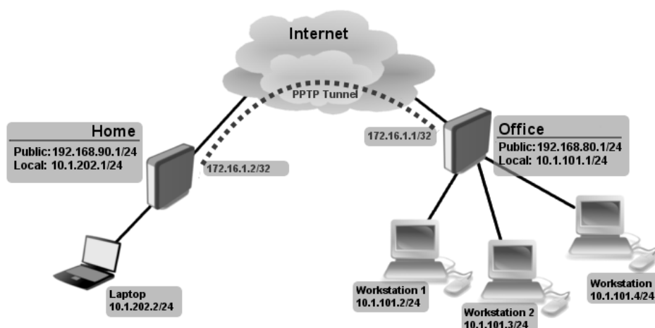
Рис. 10. Варіант побудови тунелю за протоколом PPTP
