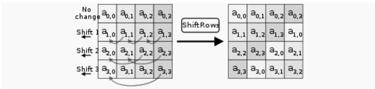
Рис. 24. Процедура ShiftRows()
