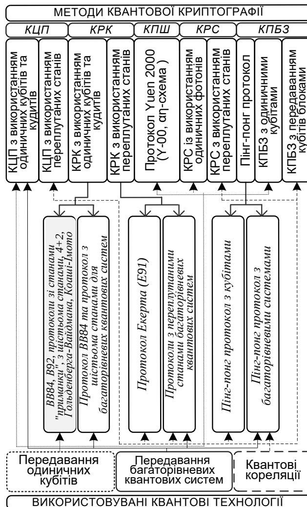
Рис. 31. Узагальнена класифікація методів квантової криптографії
