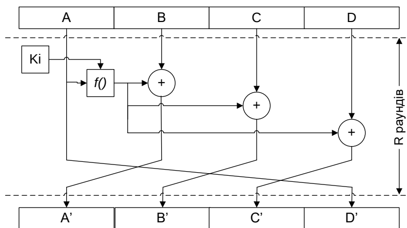
Рис. 13. Розширена мережа Фейстеля
