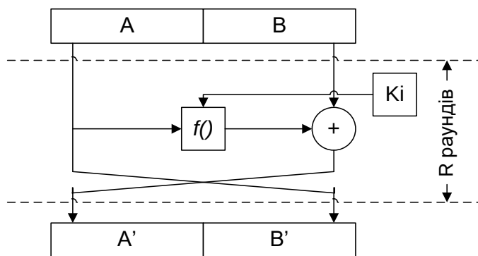
Рис. 12. Мережа Фейстеля
