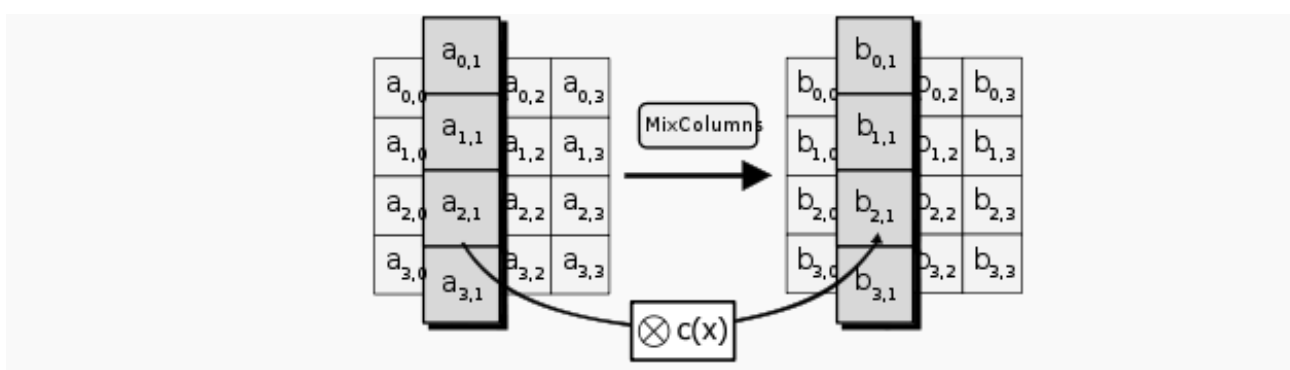
Рис. 25. Процедура MixColumns()
