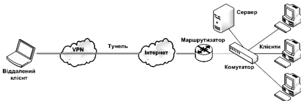
Рис. 9. VPN-тунель через мережу Інтернет
