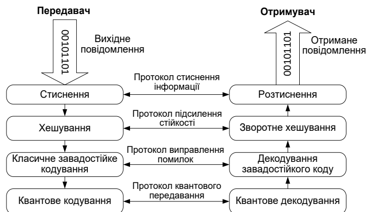
Рис. 33. Стек протоколів КПБЗ на базі пінг-понг протоколу
