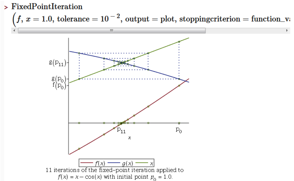
Рисунок 4 - Метод простої ітерації з графічною ілюстрацією.
