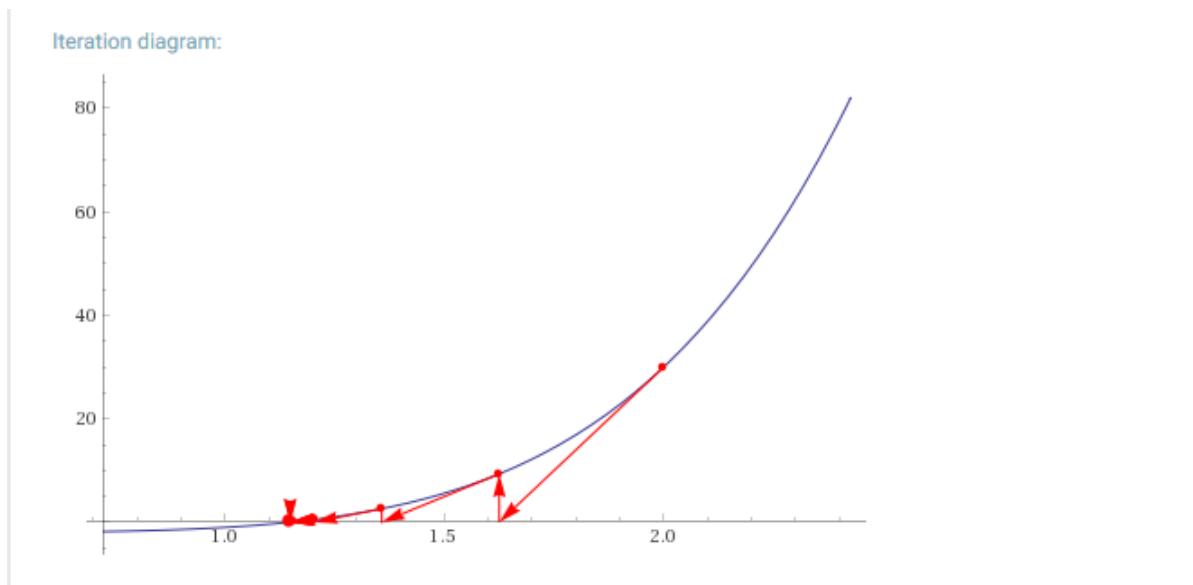
Рисунок15 – Графіка ітераційного процесу в методі Ньютона.
