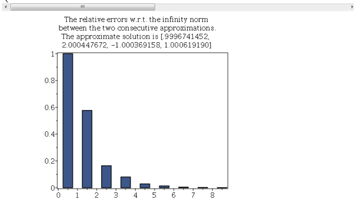
Рисунок 10 – Похибки на кожній ітерації.
