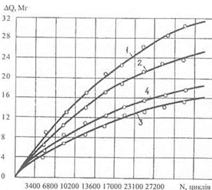
Рисунок 4.15 – Зношування титанового сплаву BT5 залежно від числа циклів: 1 – шліфування; 2 – точіння; 3 – МАП при N_i = 1,24 ; 4 – МАП при N_i = 17,5
