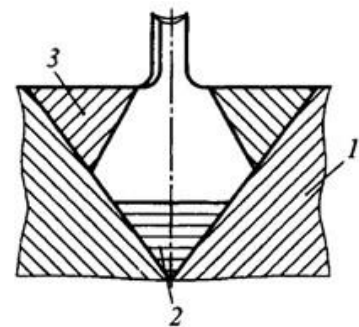
Рисунок 3.74 – Схема зрізування припуску при протягуванні хвостовиків компресорних лопаток типу "ластівчин хвіст"
