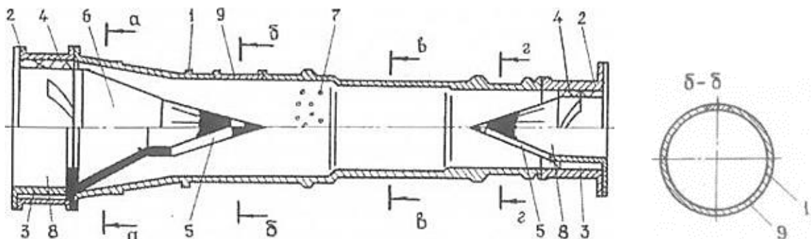
Рисунок 4.16 – Установка для пневмоімпульсної обробки валів ГТД
