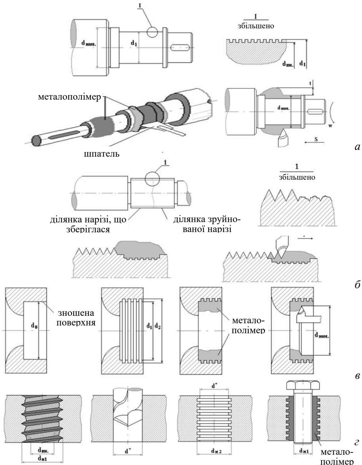
Рисунок 5.30 – Застосування металополімерних матеріалів у ремонтних роботах: відновлення зношеної цапфи валу (а), відновлення зношеної нарізі (б), відновлення зношеної внутрішньої циліндричної поверхні (в), відновлення зірваної нарізі (г)
