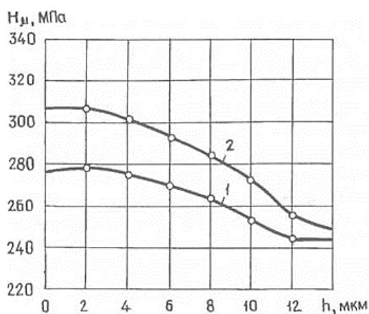
Рисунок 4.14 – Зміна мікротвердості титанового сплаву BT5: 1 – після шліфування; 2 – після МАП
