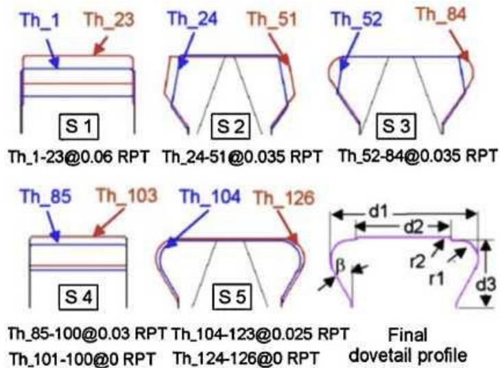
Рисунок 1.4 – Приклад поперечного перерізу п'яти сегментів протяжного інструмента для утворення профілю типу "ластівчин хвіст" (Th_ #: № зубу; RPT: підйом на зуб)
