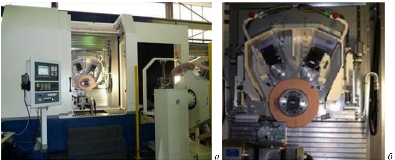
Рисунок 3.32 – П'ятиосьовий верстат ELB-SCHLIF Micro Cut4-520 (а) і його робоча зона (б)
