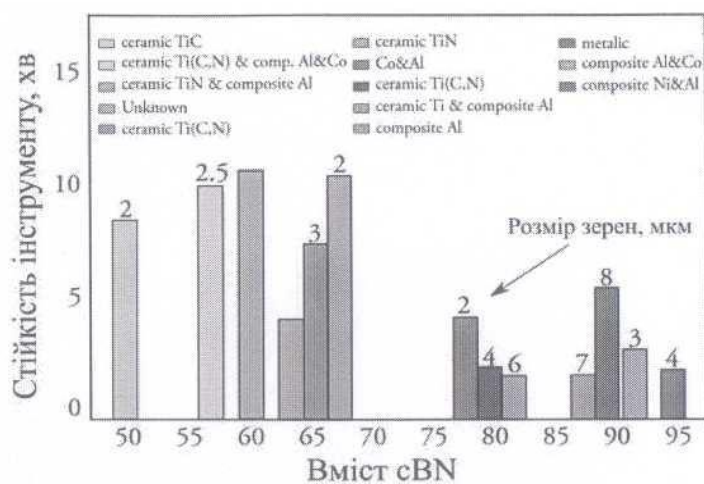
Рисунок 1.7 – Порівняння стійкості інструмента з різним вмістом CBN в умовах механічної обробки сплаву Inconel 718
