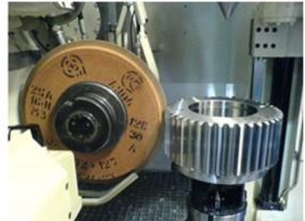
Рисунок 3.25 – Профільне шліфування прямозубого зубчастого колеса високоструктурним кругом
