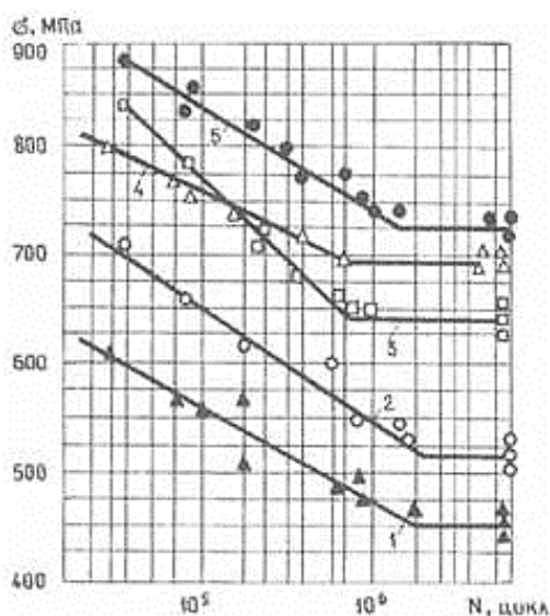
Рисунок 4.5 – Криві втомленості зразків зі сталі 13Х11Н2В2МФ-Ш:
