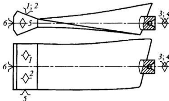
Рисунок 3.64 – Схема базування заготовки з хвостовиком типу «ластівчин хвіст» при фрезеруванні проточної частини
