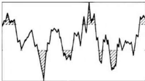
Рисунок 2.7 – Зворотний коефіцієнт зминання ареалу (X – коефіцієнт зминання ареалу S_{mc}(mr) , %; Y – висота)
