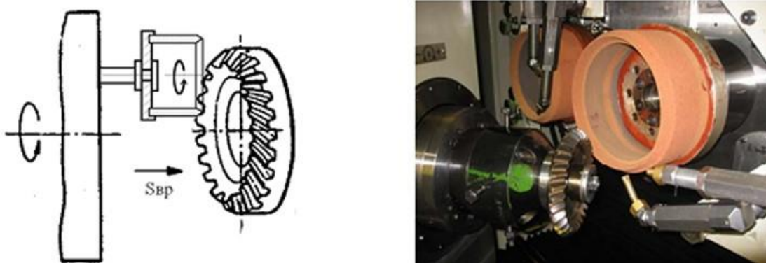
Рисунок 3.26 – Шліфування конічного зубчастого колеса за схемою періодичного обкату
