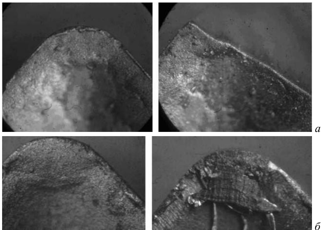
Рисунок 5.33 – Зношування різців при точінні (зліва – нова пластинка, справа – зношена): T15K6, V=157 м/хв, s = 0,1 мм/об, H = 0,2 мм, оброблюваний матеріал «Лео-Кераміка» (а), T15K6, V=157 м/хв, s = 0,1 мм/об, H = 0,2 мм, оброблюваний матеріал Сталь 45 (б)
