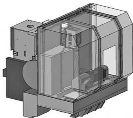
Рисунок 3.13 – 5-ти осьовий багатоопераційний ОЦ з поворотно-оберттовим столом з магазином інструментів для комплексної обробки лопаток:
