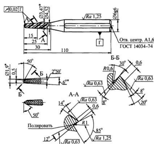
Рисунок 3.72 – Фреза кінцева для попередньої обробки складних профільних поверхонь
