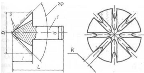
Рисунок 5.48 – Одношарова алмазна конічна зенківка: 1 – корпус зенківки; 2 – алмазовмісний робочий шар
