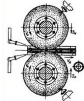
Рисунок 3.23 – Схема двостороннього профільного глибинного шліфування “ялинкового” профілю хвостовика лопатки турбіни авіаційного двигуна й високоструктурний шліфувальний круг
