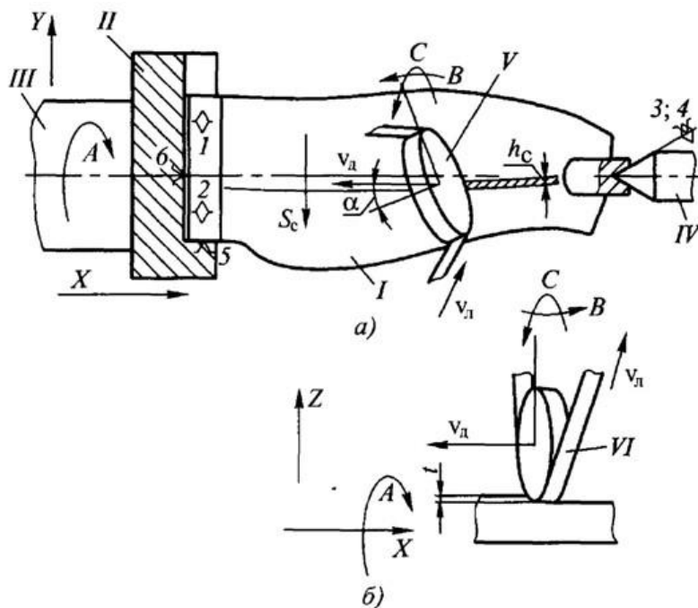
Рисунок 3.75 – Схема базування заготовки й обробки на стрічково-шліфувальному верстаті з ЧПК: a – схема базування деталі і взаємних переміщень деталі й інструмента при утворенні повздовжнього рядка шириною h_c ; б – схема зняття припуску глибиною t ; \alpha – кут розвороту притискного ролика до напрямку повздовжньої подачі деталі
