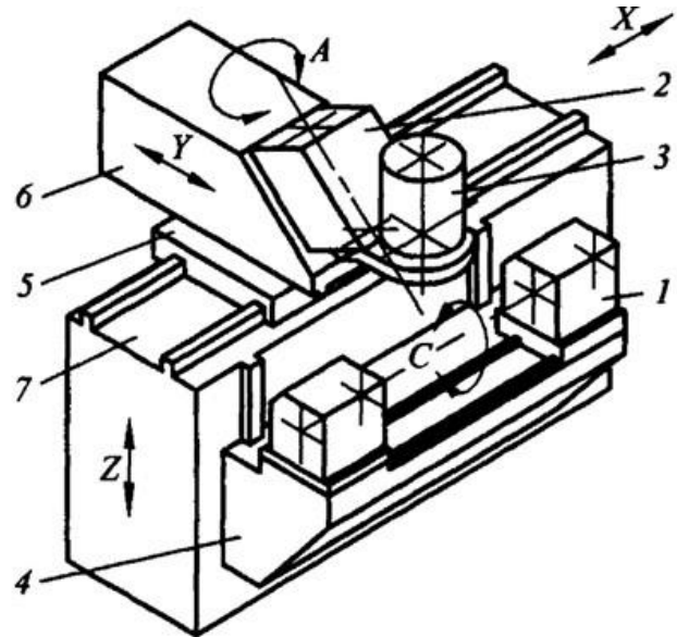
Рисунок 3.67 – Принципова схема верстата НХ-151 для кругової обробки лопатки: 1 – шпиндельні бабки кругової подачі заготовки; 2 – супорт кутового переміщення фрезерної головки; 3 – фрезерна головка; 4, 5, 6 – вертикальний, поздовжній і поперечний супорти верстату відповідно; 7 – станина
