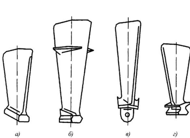
Рисунок 3.54 – Конструкції лопаток компресора: а – з хвостовиком типу "ластівчин хвіст"; б – з антивібраційними полками; в – з шарнірним хвостовиком; з – з трапецеїдальним хвостовиком
