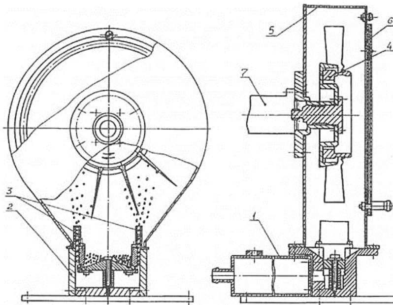
Рисунок 4.9 – Установка для пневмодробоструминного зміцнення
