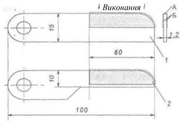
Рисунок 5.42 – Конструкції одношарових алмазних ножовочних полотен:
