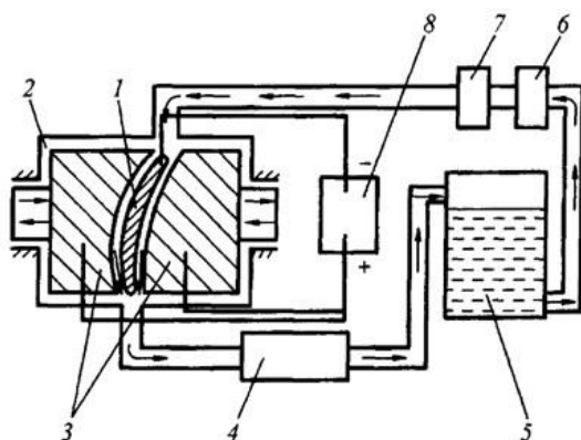
Рисунок 3.60 – Схема установки для ЕХО: 1 – робоча камера; 2 – лопатка; 3 – джерело струму; 4 – нагнітач; 5 – теплообмінник; 6 – бак з електролітом; 7 – центрифуга; 8 – електроди (інструменти)
