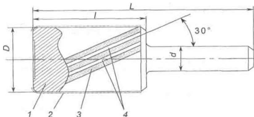
Рисунок 5.45 – Конструкція одношарової алмазної шліфувальної головки:
