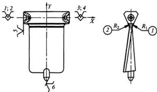
Рисунок 3.59 – Схема базування лопатки під час обробки радіусів R_1 і R_2 переходу з боку спинки й корита
