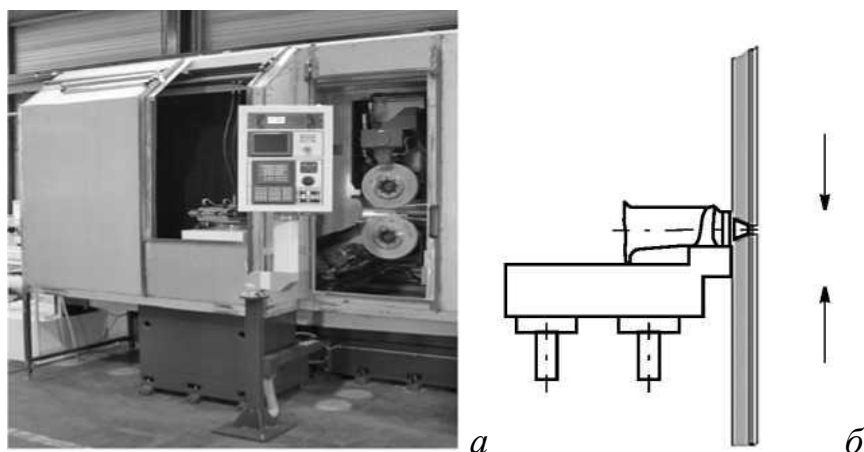
Рисунок 3.28 – Компонівка двошпиндельного верстату MICRO-CUT 4-320DS з рухомою колоною – а ; наладка операції шліфування ялинкового хвостовика – б
