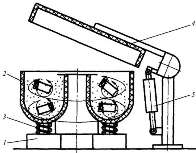
Рисунок 3.76 – Схема радіального вібратора торового типу:
