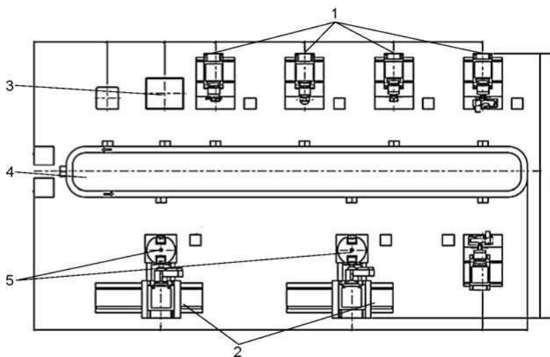
Рисунок 3.14 – Схема прямої лінії для диференційованої обробки типових поверхонь лопаток: 1 – одношпиндельні шліфувальні центри; 2 – двошпиндельні шліфувальні центри; 3 – координатно-вимірвальна машина; 4 – транспортна система; 5 – модуль обробки/завантаження
