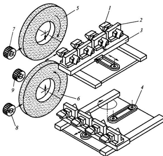
Рисунок 3.45 – Схеми роботи верстата в режимах безперервної й дискретної правки
