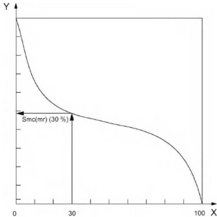
Рисунок 2.7 – Зворотний коефіцієнт зминання ареалу (X – коефіцієнт зминання ареалу S_{mc}(mr) , %; Y – висота)
