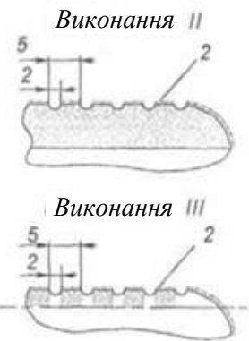
Рисунок 5.42 – Конструкції одношарових алмазних ножовочних полотен:
