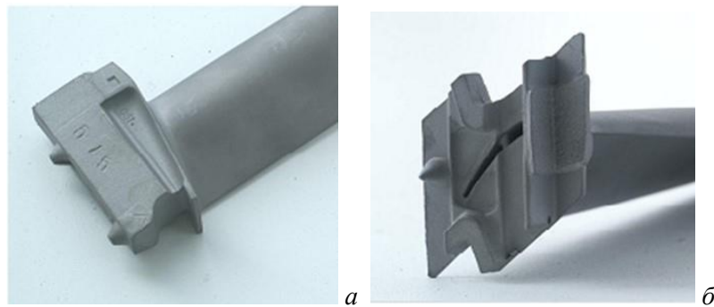
Рисунок 3.79 – Базові поверхні турбінної лопатки, виконані у виливку заготовки: а – з боку хвостовика; б – з боку бандажної полиці
