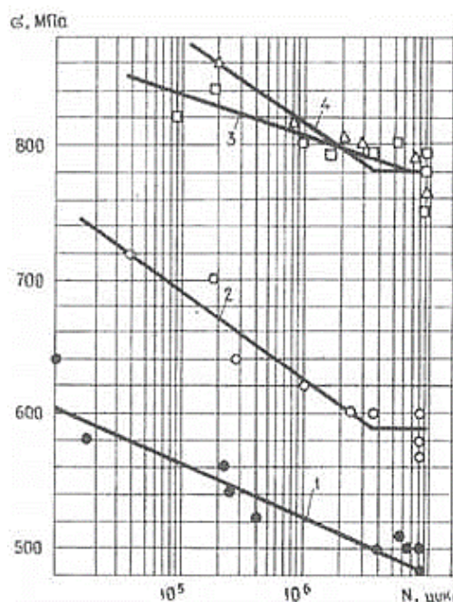
Рисунок 4.6 – Криві втомленості зразків зі сталі 40ХН2МА-Ш ( P_y = 150 Н; R_{сф} = 2 мм; s = 0,05 мм/об):
