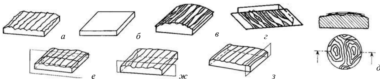
Рисунок 2.2 – Поверхня, профіль і бази відліку: реальна (а), номінальна (б), еквідистантний переріз (в), дотичний переріз плоскої номінальної поверхні (г), контурна картина поверхні (д), профіль реальної поверхні (е), поперечний профіль реальної поверхні (ж), поздовжній профіль реальної поверхні (з)
