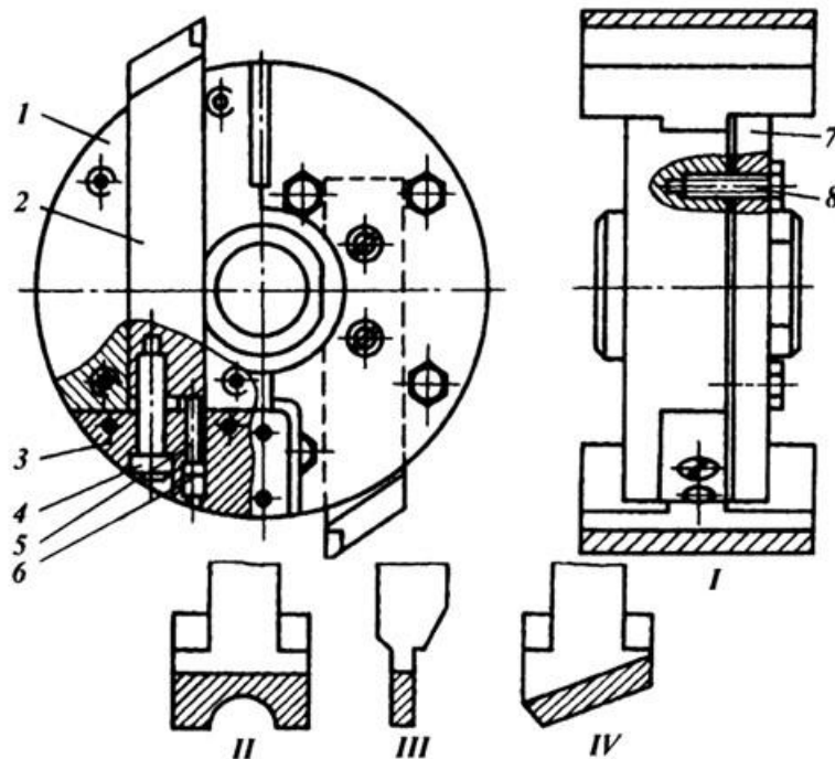
Рисунок 5.37 – Універсальна фреза: / – циліндрична; // – фасонна; /// – дискова; IV – кутова
