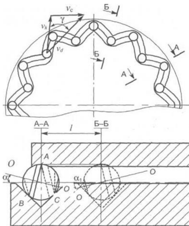
Рисунок 5.17 – Схема алмазного доведення куль у напрямних канавках зі змінною кривизною
