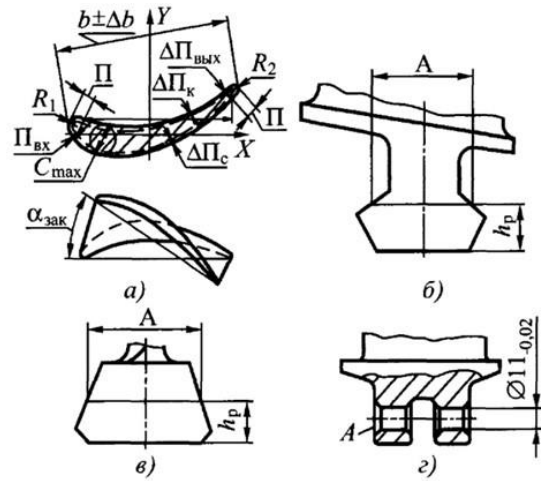
Рисунок 3.55 – Конструктивні елементи робочих лопаток компресора: а – перо лопатки; б – хвостовик типу "ластівчин хвіст"; в – кільцевий трапецеїдальний хвостовик; з – шарнірний хвостовик
