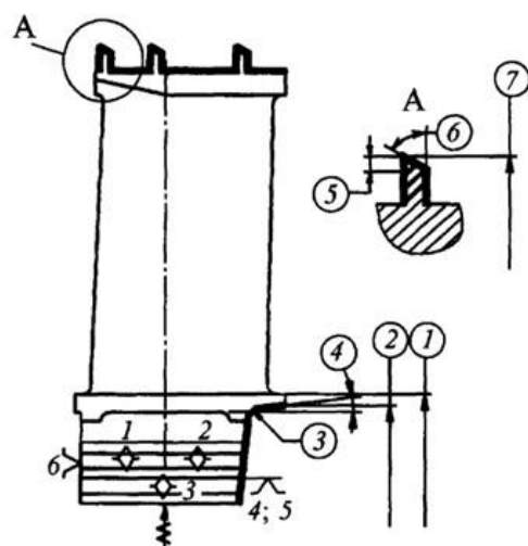
Рисунок 3.50 – Схема базування лопатки під час обробки циліндричних поверхонь
