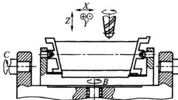
Рисунок 3.62 – Схема руху інструмента й заготовки при фрезеруванні профілю пера (варіант 1)
