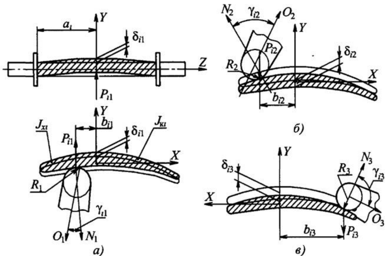
Рисунок 3.70 – Схеми до розрахунку деформації лопатки при круговому фрезеруванні
