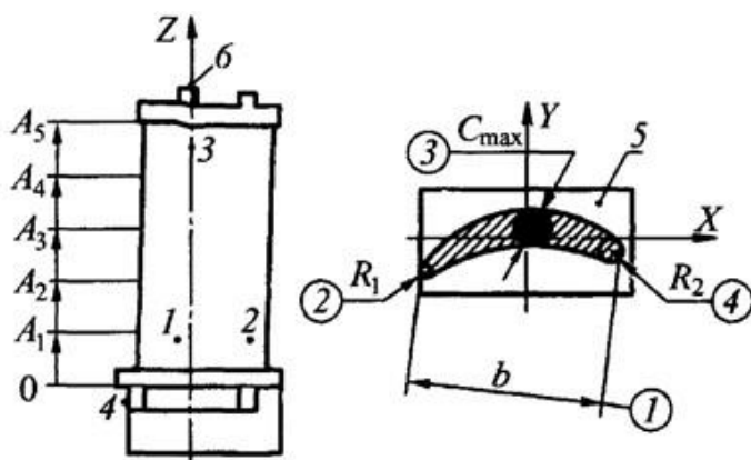
Рисунок 3.37 – схема контролю й доопрацювання заготовки на операціях вхідного контролю: 1...6 – базові точки заготовки
