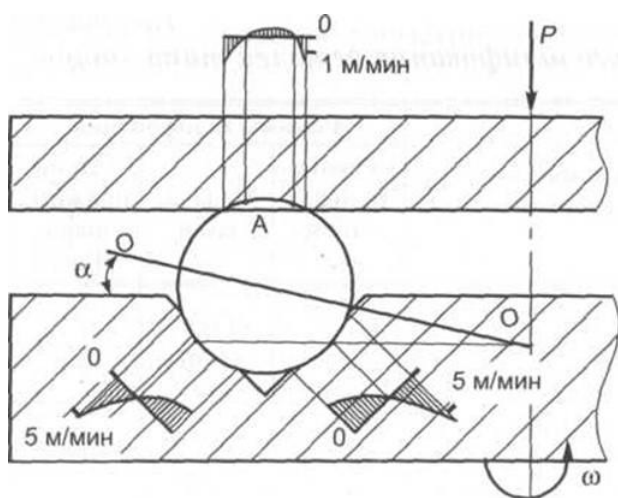
Рисунок 5.16 – Положення власної осі обертання ОО й епюра швидкостей ковзання під час доведення куль у кільцевих канавках
