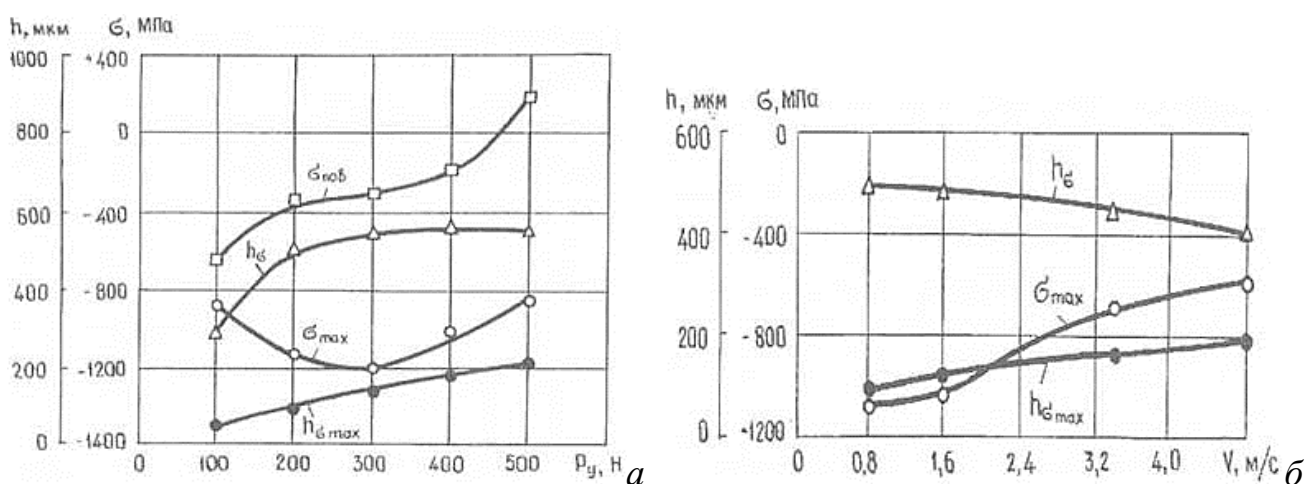
Рисунок 4.1 – Залежності глибини залягання тангенціальних залишкових напружень та їхнього рівня ( v = 1,3 м/с) від сили (а) і швидкості вигладжування ( P_y = 400 Н) валу зі сталі 13Х11Н2В2МФШ (б)
