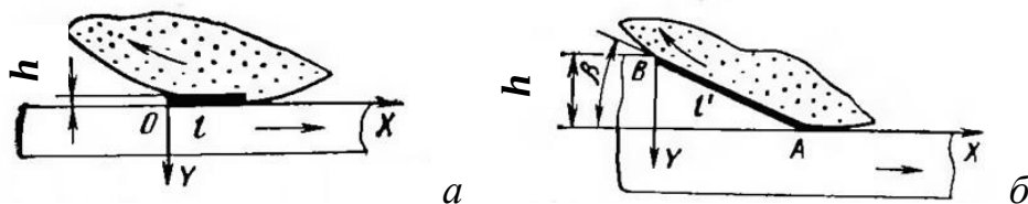
Рисунок 3.20 – Схеми звичайного ( а ) й глибинного ( б ) врізного шліфування: а – шліфування з великими відносними швидкостями деталі й малою глибиною різання; б – шліфування з невеликими відносними швидкостями деталі й великою глибиною різання
