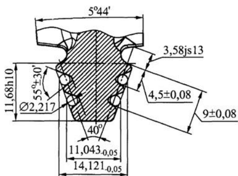
Рисунок 3.46 – Конструкція поперечного перерізу хвостовика лопатки турбіни
