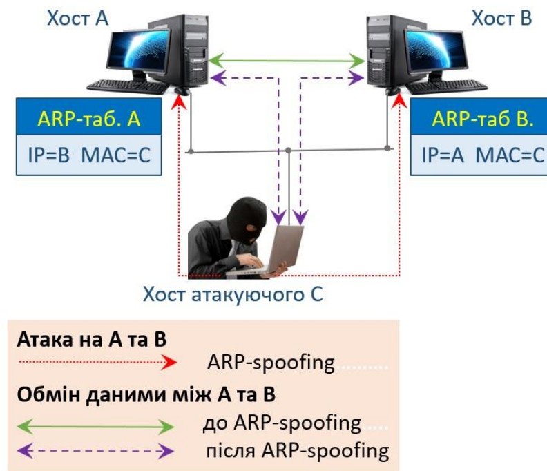
Рисунок 3.6. Схема атаки «ARP-spoofing»
