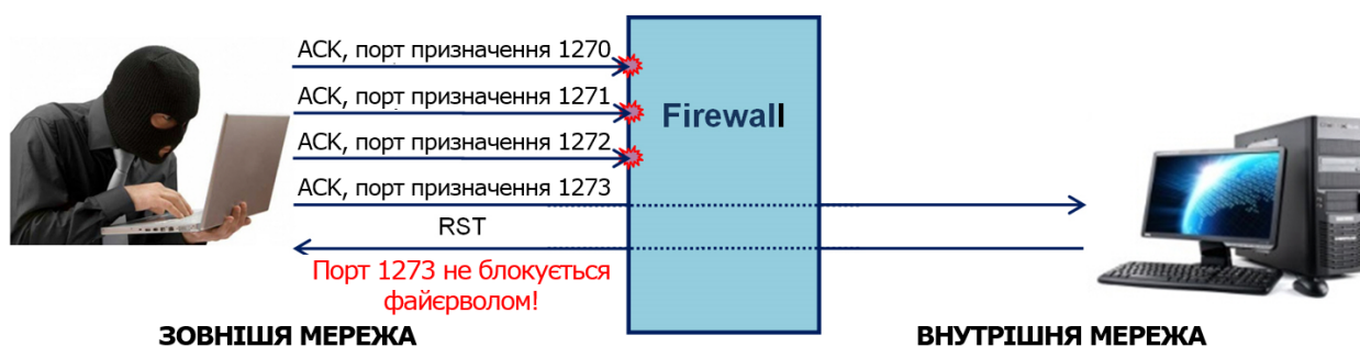
Рисунок 3.13. ACK-сканування
