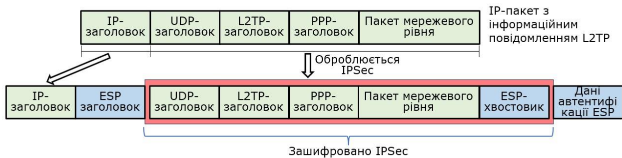
Рисунок 7.21. Приклад використання протоколу L2TP поверх IPsec
