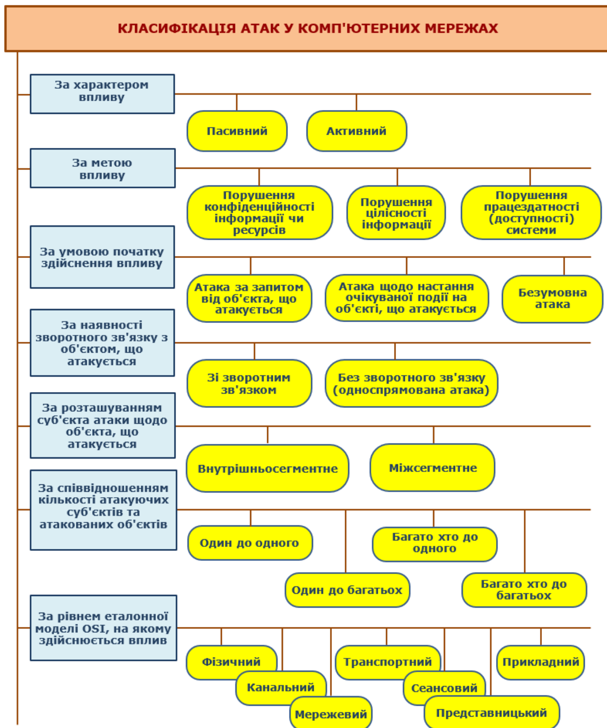
Рисунок 1.1. Класифікація атак у комп'ютерних мережах
