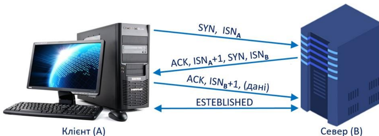
Рисунок 2.1. У процесі створення TCP-з'єднання сторони обмінюються рядом службових повідомлень
