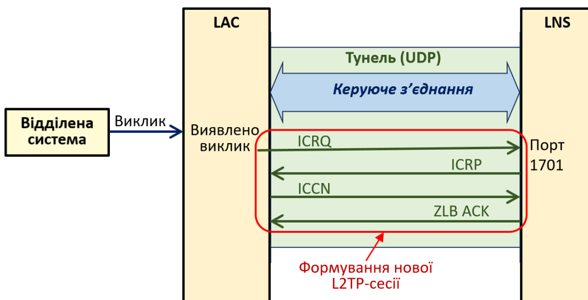
Рисунок 7.19. Обмін керуючими повідомленнями для формування індивідуальної L2TP-сесії за ініціативою LAC
