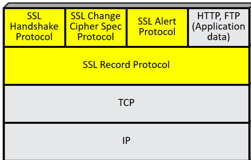
Рисунок 6.3. Архітектура протоколу SSL/TLS
