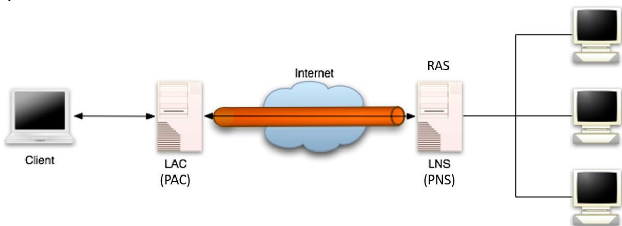
Рисунок 7.2. Можлива схема криптиотунелю з використанням протоколів PPTP та L2TP
