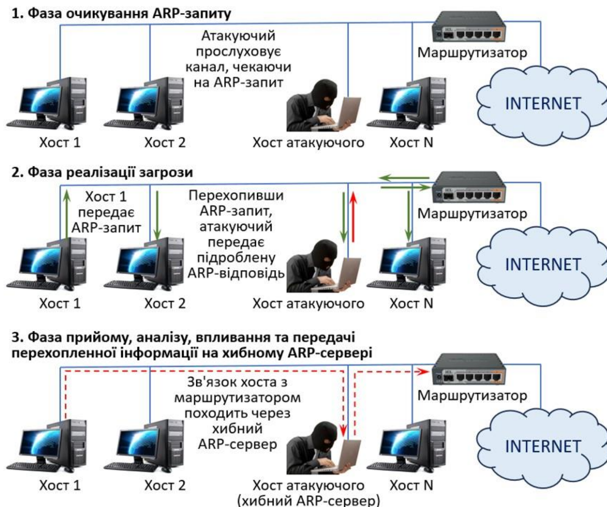
Рисунок 3.5. Атака «Помилковий ARP-сервер» з перехопленням ARP-запиту
