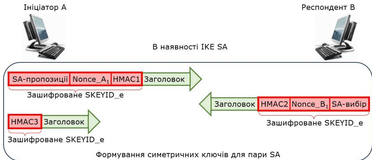
Рисунок 8.11. Швидкий режим фази 2
