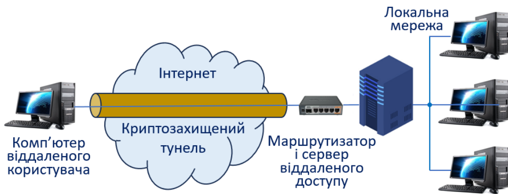
Рисунок 7.13. Схема тунелювання під час прямого підключення комп'ютера віддаленого користувача до Internet
