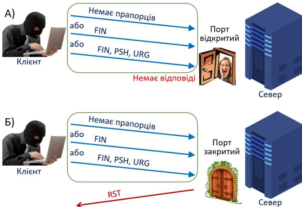
Рисунок 3.11. Сканування TCP-FIN, Xmas Tree, TCP-Null
