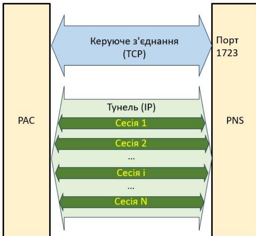
Рисунок 7.11. Компоненти протоколу PPTP, що працюють між PAC та PNS
