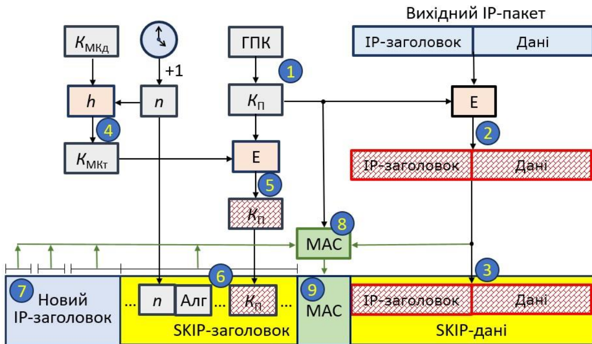
Рисунок 8.1. Схема формування захищеного SKIP-пакета
