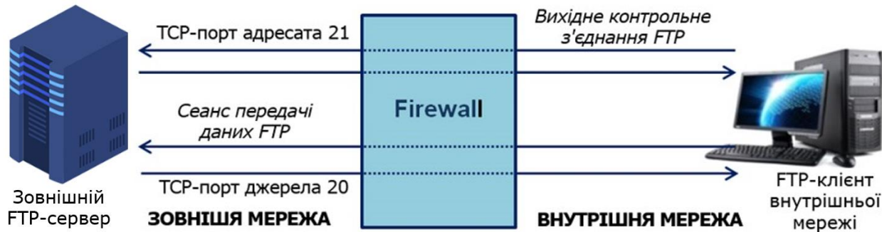
Рисунок 3.14. Стандартні з'єднання FTP (контрольна та безпосередня передача даних)
