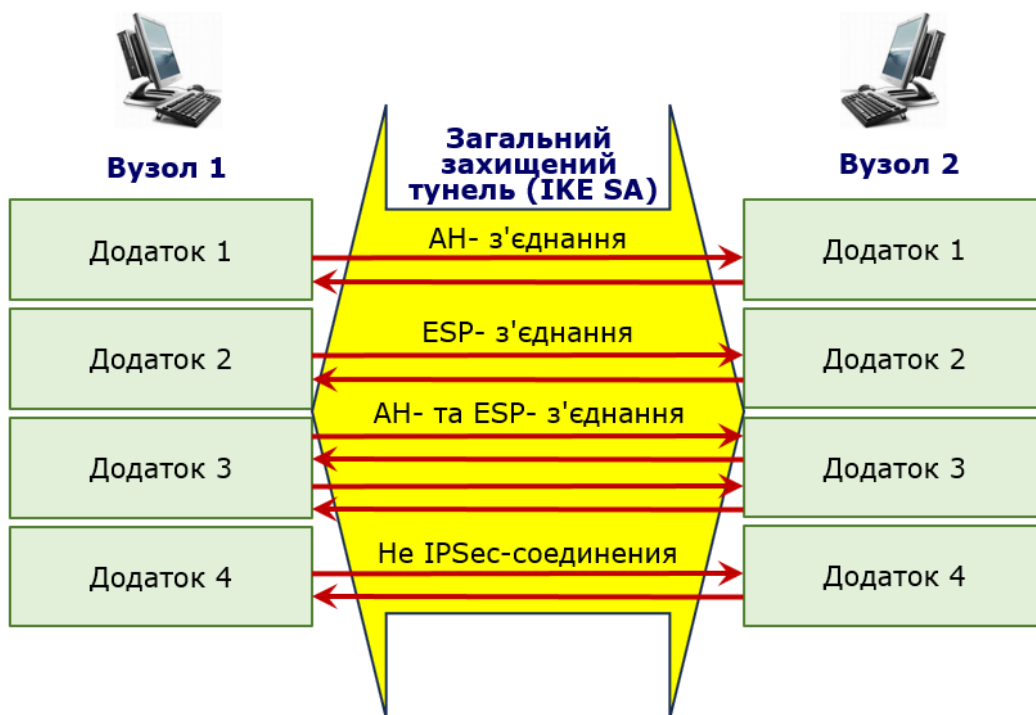
Рисунок 8.8. Формування захищених з'єднань протоколом IKE
