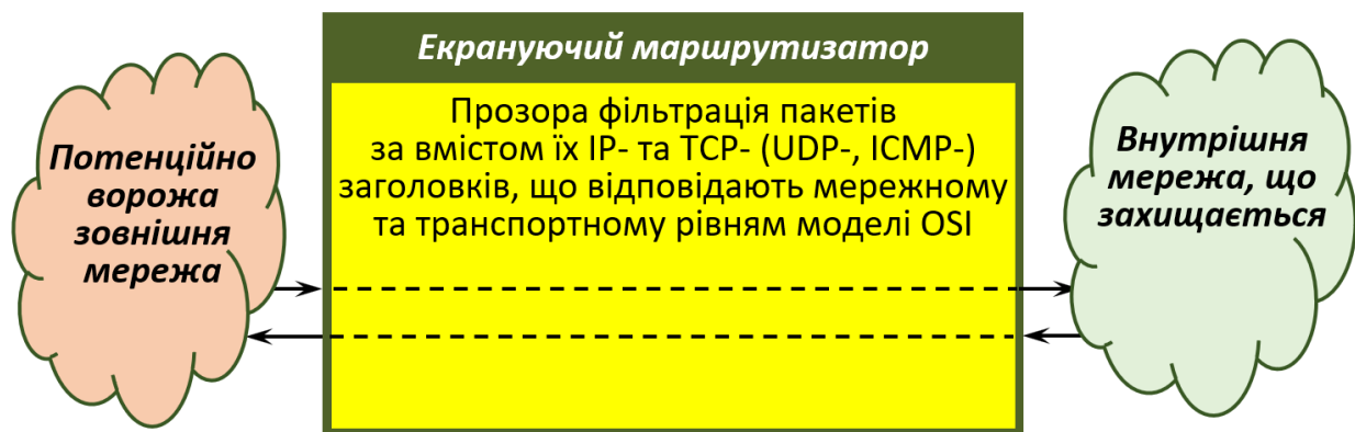
Рисунок 4.5. Схема функціонування пакетного фільтра
