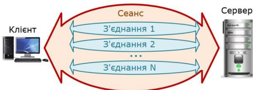
Рисунок 6.2. Сеанс та з'єднання SSL/TLS
