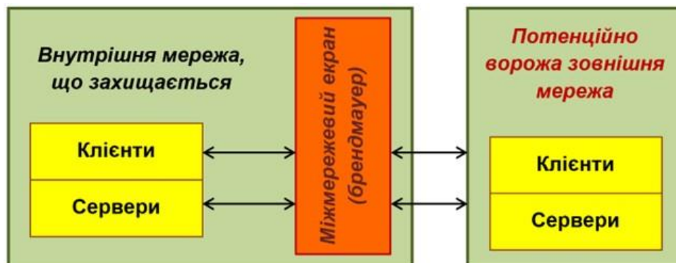
Рисунок 4.1. Схема підключення міжмережевого екрану
