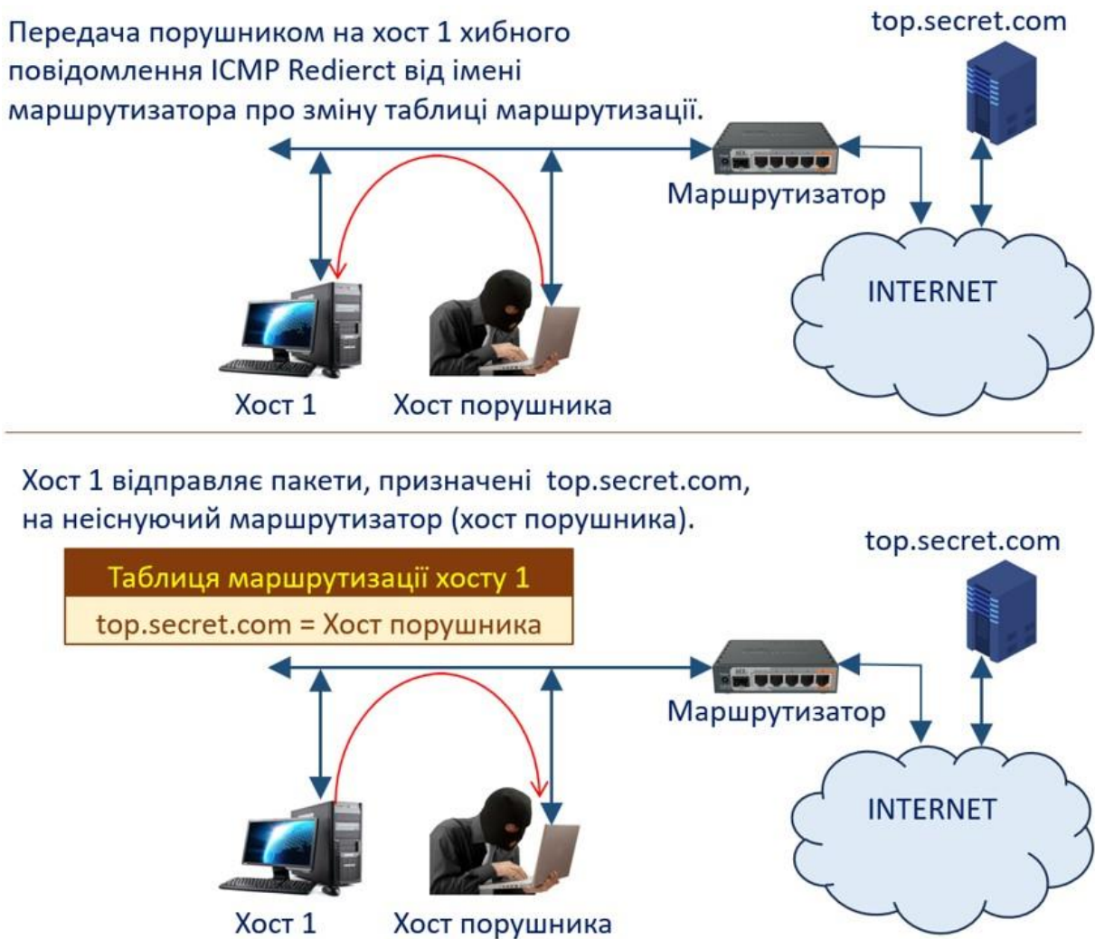
Рисунок 2.5. Атака «Помилковий DNS-сервер»
