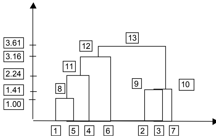
Рисунок 9.1 – Дендрограма
