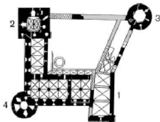
План замку магістра Лівонського ордену в Цесисі:
