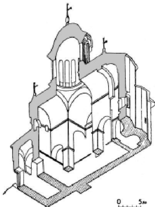
Церква Св. Миколая в Куртя де Арджеш. Аксометричний розріз
