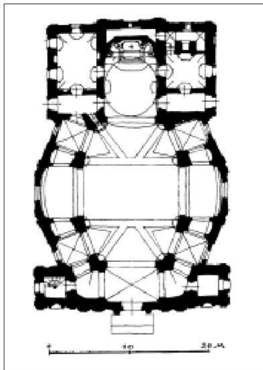
План костелу Св. Анни в Любартові
