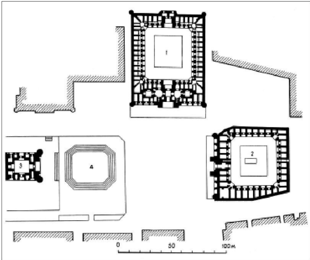
План ансамблю Лябі-хауз у Бухарі:
