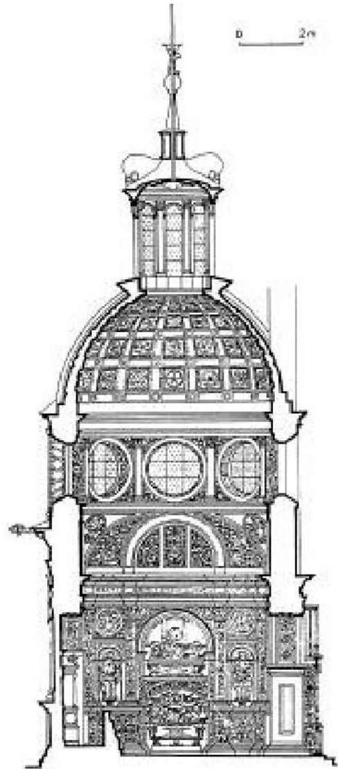
Поздовжній розріз капели короля Сігізмунда I при кафедральному костелі на Вавелі в Кракові
