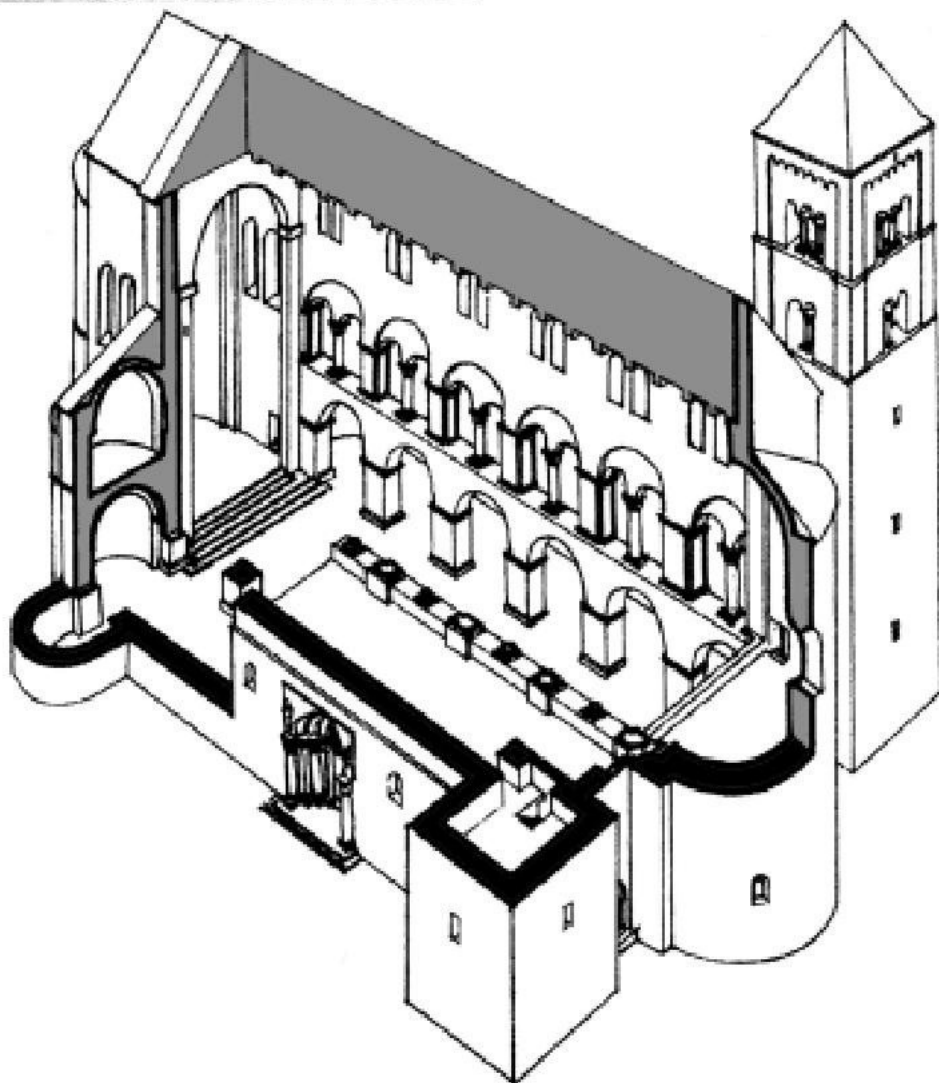
Аксометричний розріз костелу в Тумі
