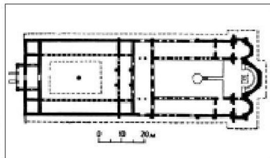
План «Великої базиліки» в Плисці
