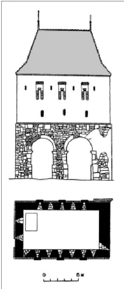
Кравецька надбрамна башта міських murів Сігішоари. Фасад і план третього ярусу
