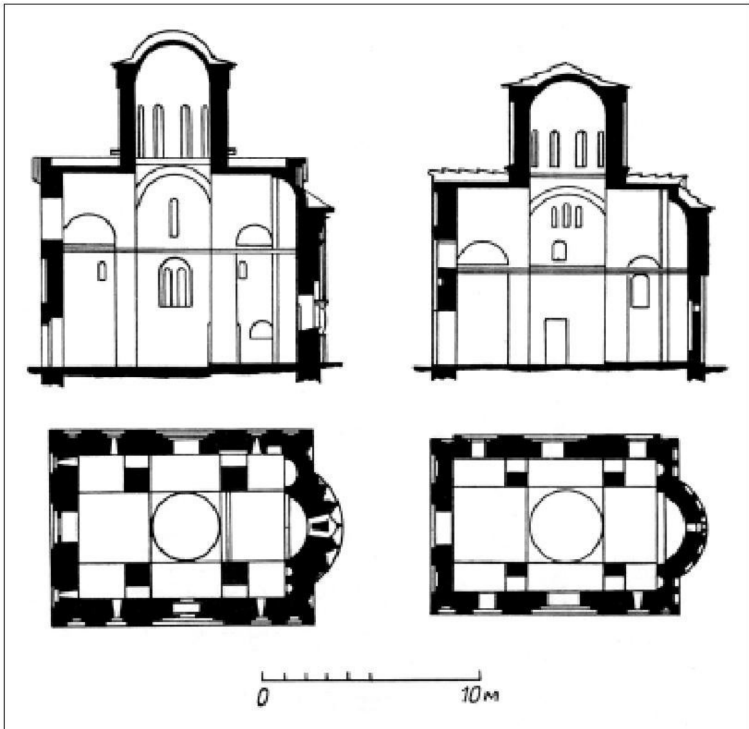
Плани й поздовжні розрізи церков Македонської і Косовсько-Метохійської школи: Архангелів у монастирі Лісново; Архангелів у Штупі
