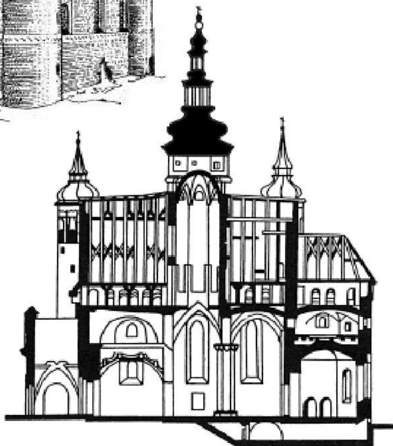
Благовіщенська церква у Супраслі. Поздовжній розріз
