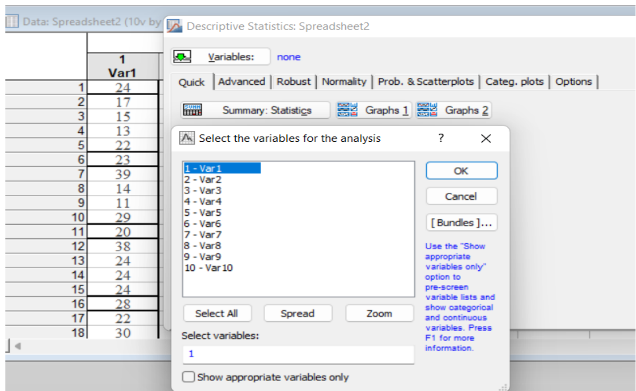
Рис. 4.32. Вибір Graphs 1 та даних
