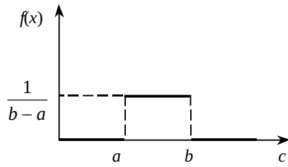
Рис. 2.17. Щільність розподілу ймовірності
