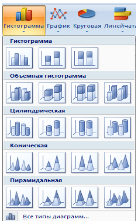
Рис. 3.3. Діалогове вікно майстра гістограм
