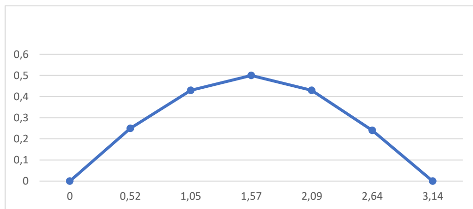
Рис. 2.10. Диференціальна функція
