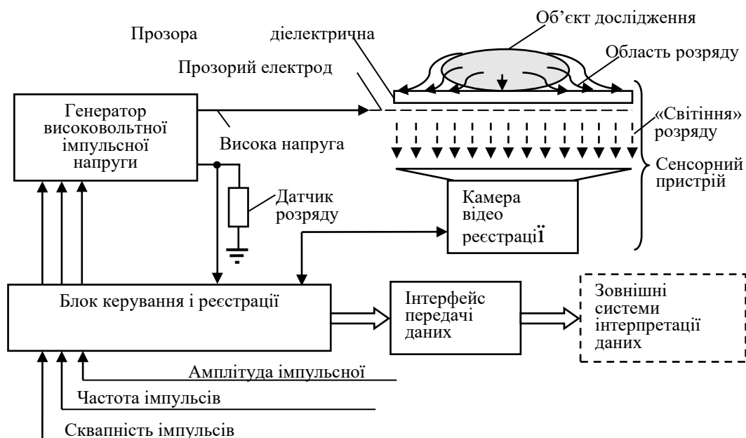
Рис. 2. Структурна схема пристрою з додатковими параметрами ГРВ досліджень
