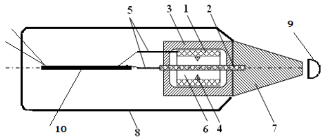
Рис. 1. Коаксіальний іскровий розрядник: 1 - металева трубка 2 - центральний стрижень; 3 - діелектричний циліндр; 4 - металеві виступи; 5 - вводи електродів; 6 - порожнина іскрового розряду; 7 - діелектрична антена; 8 - металевий екран (корпус), 9 - аплікатор, 10 - друкована плата.
