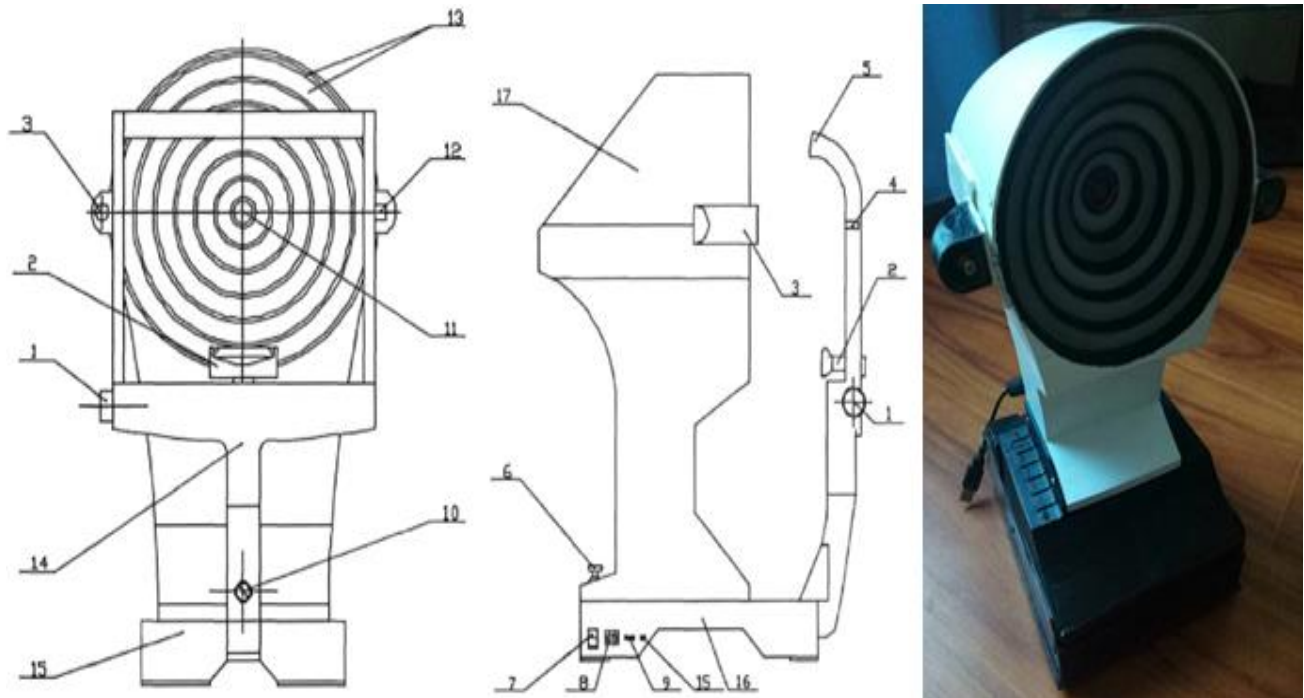
Рис.1. Автофотокератометр:
