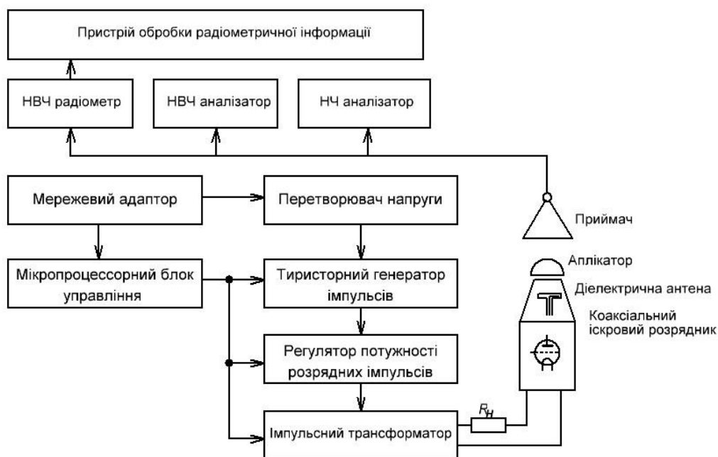
Рис. 1. Макет імпульсного генератора іскрових розрядів
