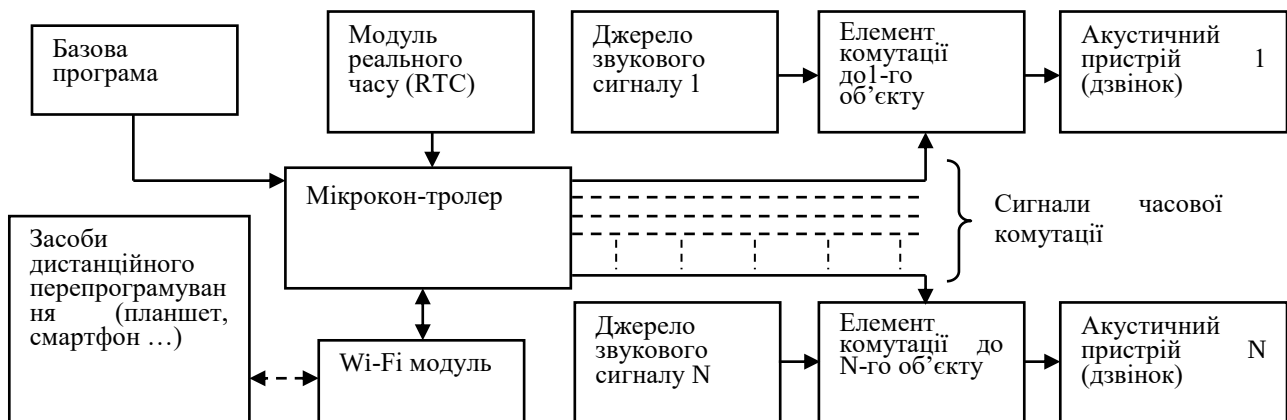
Рис.1. Структура адаптивної системи
