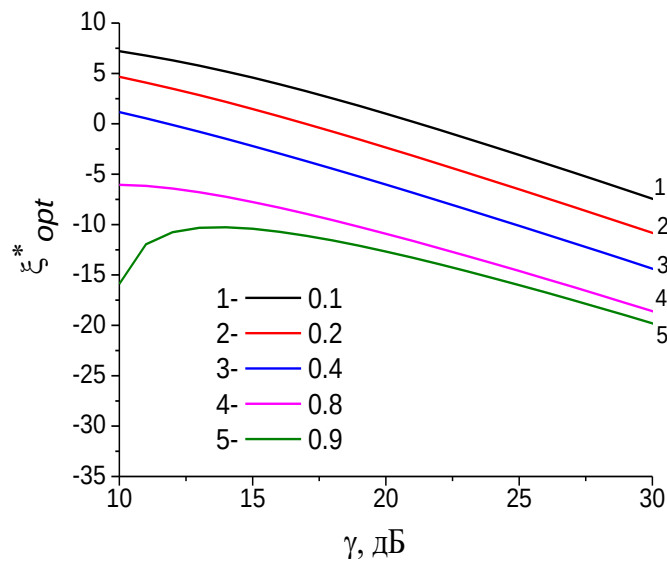
Рис. 1. Залежність оптимального порогу від співвідношення інтенсивності компонент і ймовірності викидів P при нормуванні порога на сумарну дисперсію \xi_{opt}^* (1- P=0,1 , 2- P=0,2 , 3- P=0,4 , 4- P=0,8 )
