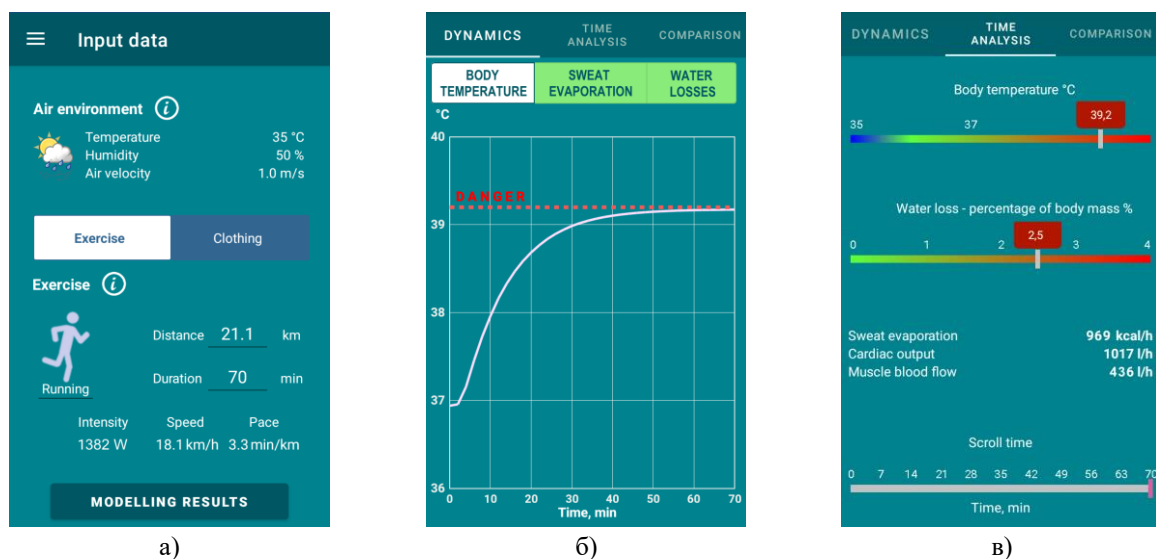
Рис. 1. Інтерфейс приложения для смартфона
