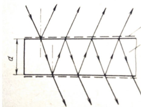
Рис.2. Многолучевая интерференция
