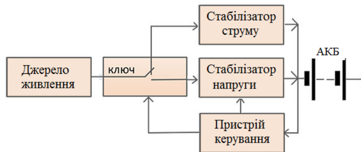
Рис. 1. Структурна схема двоступеневого зарядного пристрою
