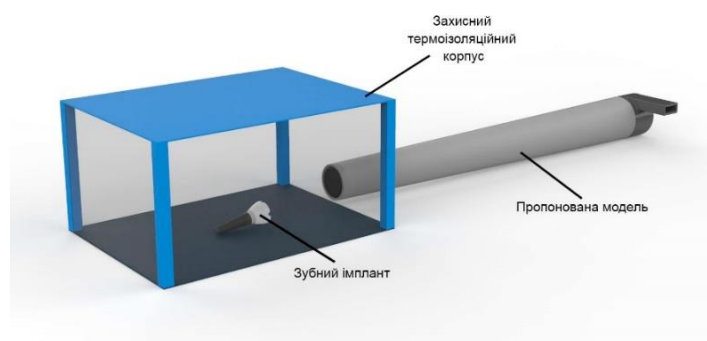
Рис. 1. 3Д модель запропонованої конструкції апарату
