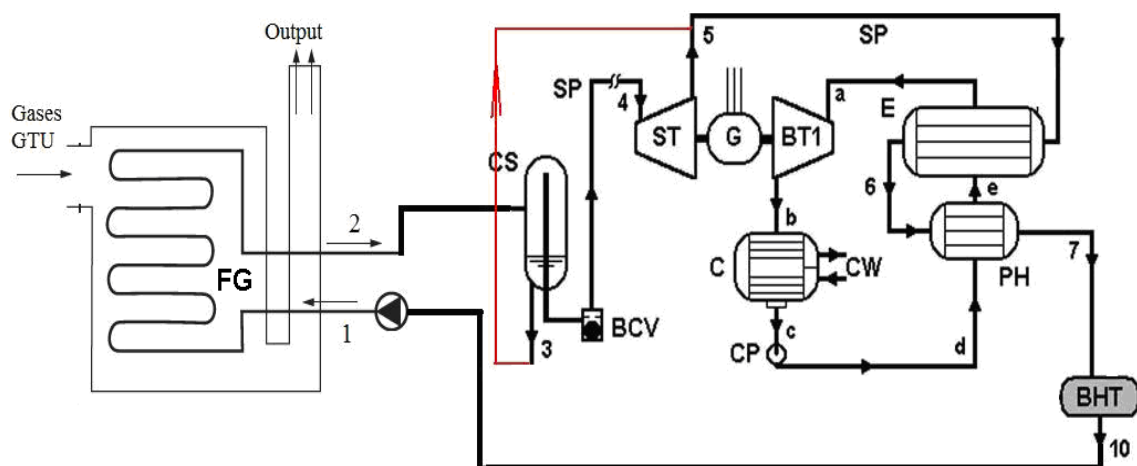
Рис. 1. Теплова схема
