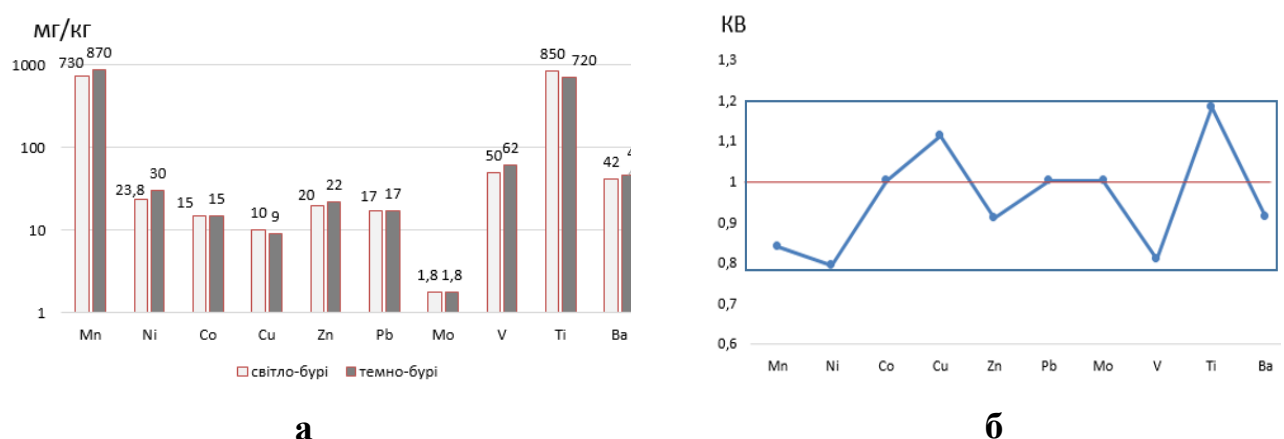
Рис. 4. Діаграма розподілу хімічних елементів у світло-бурих (Кузийський масив) та темно-бурих ґрунтах Мармароського масиву (а) та значення коефіцієнту відношення (KB) (б), де ґрунтоутвірними породами є карбонатні
