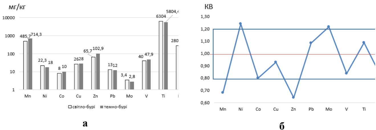
Рис. 2. Діаграма розподілу хімічних елементів у світло-бурих та темно-бурих ґрунтах Мармароського масиву (а) та значення коефіцієнту відношення (KB) (б), де ґрунотвірними породами є кристалічні сланці
