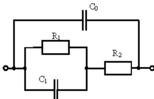
Рис. 2 – Еквівалентна схема вимірювальної комірки із власною ємністю комірки C_0 , ємністю за рахунок діелектричної проникливості рідини C_1 та відповідними активними опорами R_1 та R_2
