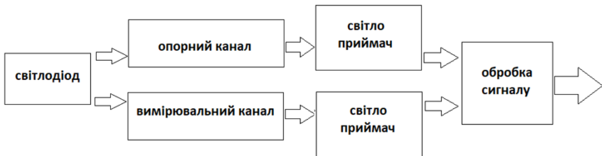
Рисунок 1. 2 - Оптична система детектора
