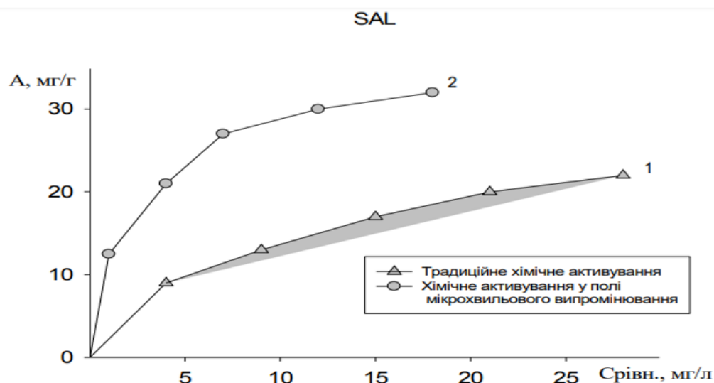
Рисунок 1 - Ізотерма адсорбції саліцилової кислоти зразками активованого вугілля, отриманими при традиційній та мікрохвильовій хімічній активації
