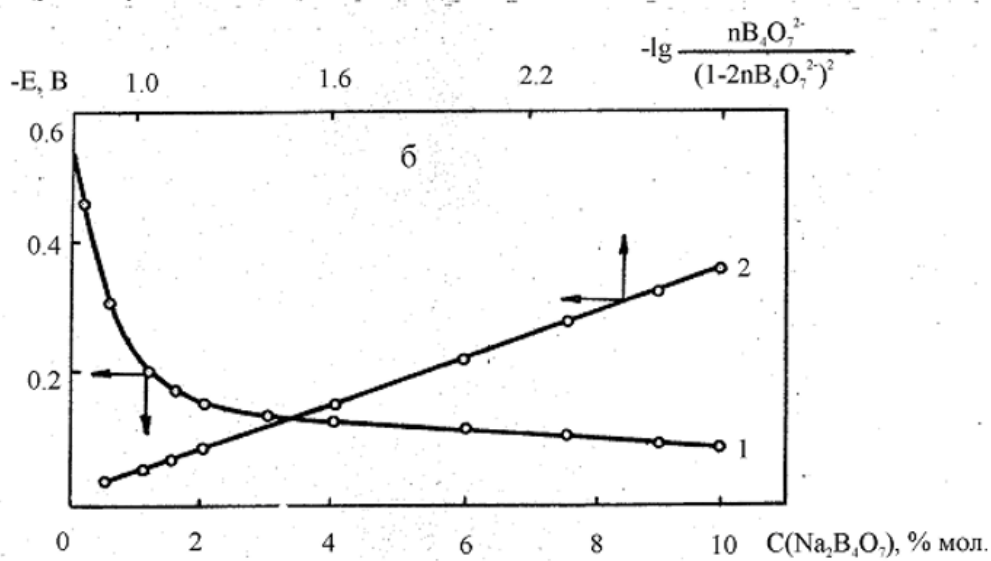
Рисунок 1 - Залежність потенціалів платино-кисневого електрода від концентрації \text{B}_2\text{O}_3 (а) та \text{Na}_2\text{B}_4\text{O}_7 (б) і її аналіз у логарифмічних координатах
