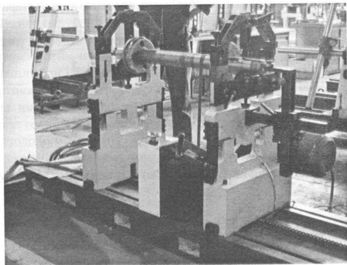
Рисунок 3.11 Балансувальний верстат ВТ1000
