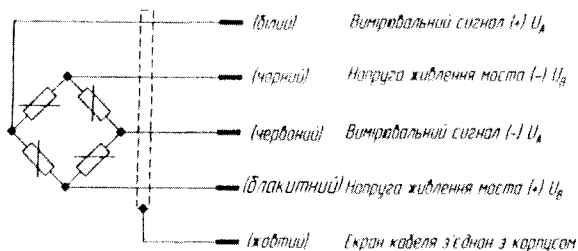
Рисунок 4.4 Вимірювання зусиль натягу в канатах ме- ханізму підйому елек- тродугової печі
