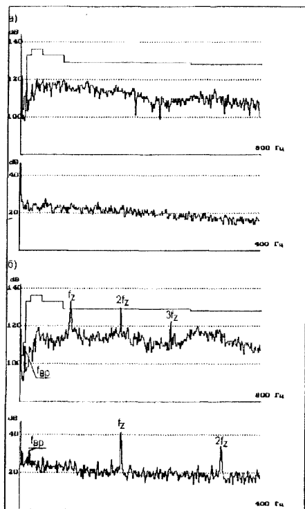
а — бездефектний редуктор; б — редуктор з дефектом зчеплення шестерней
