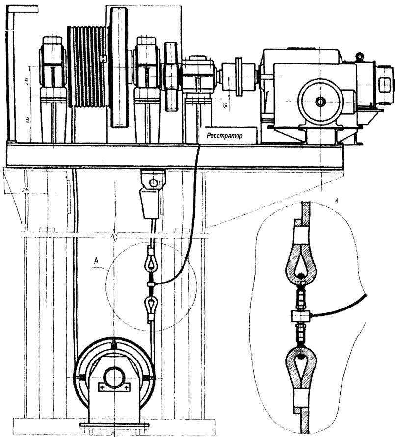
Рисунок 4.4 Вимірювання зусиль натягу в канатах ме- ханізму підйому елек- тродугової печі
