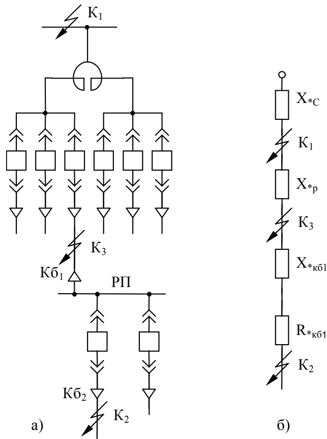
Рисунок 2.5 – Груповий здвосний реактор (а) і заступна схема (б)
