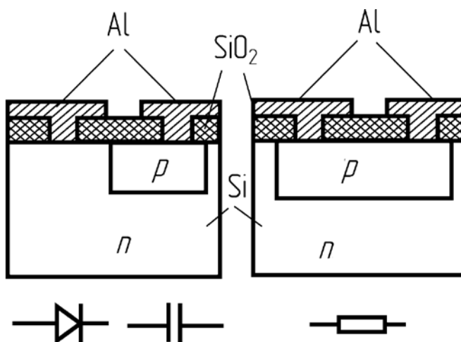
Рис. 3. Планарні структури діода (ліворуч) і резистора (праворуч)
