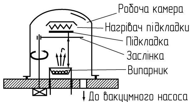
Рис. 22. Схема установки для термовакuumного осадження плівок
