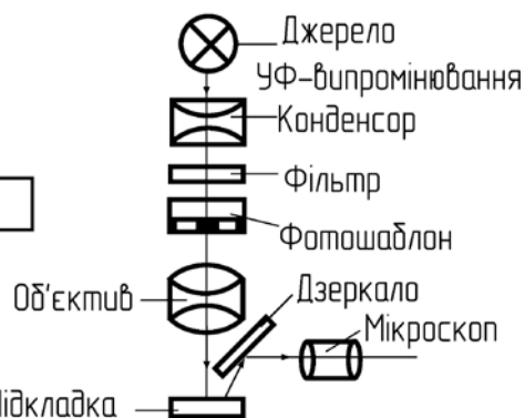
Рис. 11. Схема експонування у проєкційний фотолітографії
