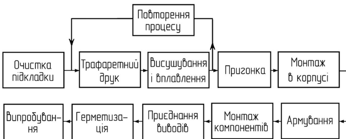
Рис. 35. Схема технологічного процесу виготовлення товстоплівкових ГІС
