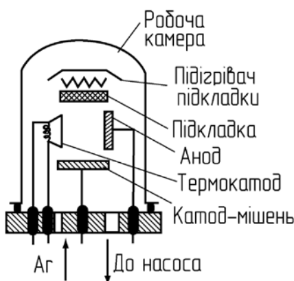
Рис. 27. Система для розпилення в несамостійному газовому розряді
