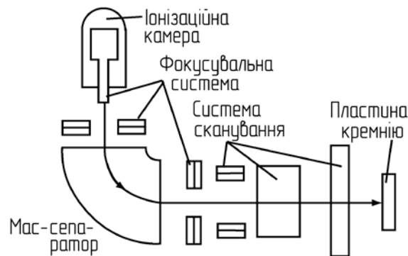
Рис. 15. Схема установки для іонного легування
