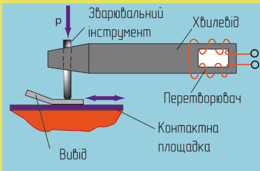
УЛЬТРАЗВУКОВЕ ЗВАРЮВАННЯ
