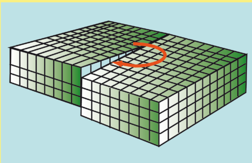
ГВИНТОВА ДИСЛОКАЦІЯ
