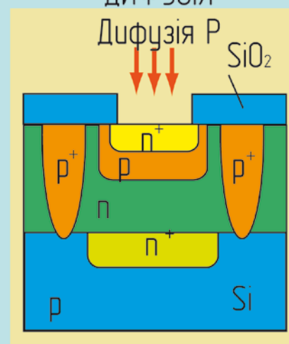
ВИГОТОВЛЕННЯ ЕМІТЕРА
