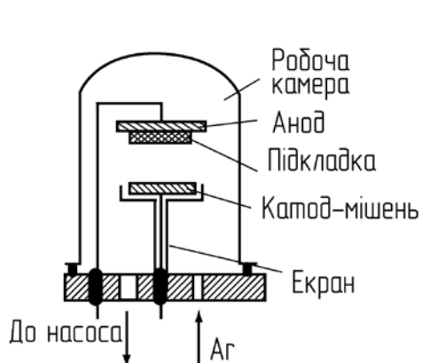
Рис. 26. Система для катодного розпилення у тліюному розряді
