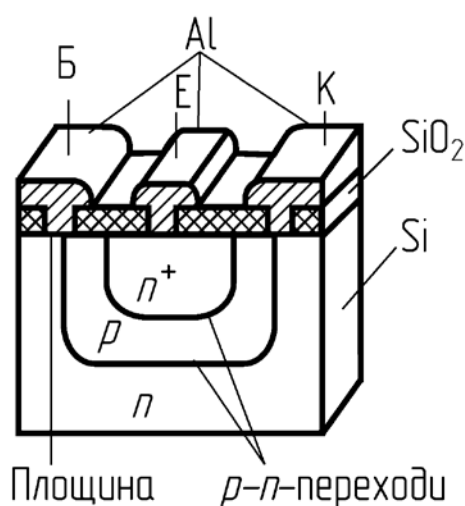
Рис. 2. Структура планарного n-p-n -транзистора
