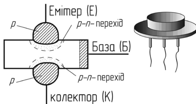
Рис. 1. Ліворуч – спрощена схема конструкції перших сплавних транзисторів, у яких металеві контакти емітера і колектора (з акцепторною p -типу домішкою) сплавлені з електронною n -напівпровідниковою базою ; праворуч – загальний вид транзистора у металічному корпусі
