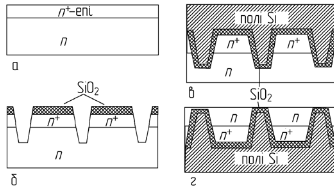
Рис. 20. Схема формування структури з діелектричною ізоляцією
