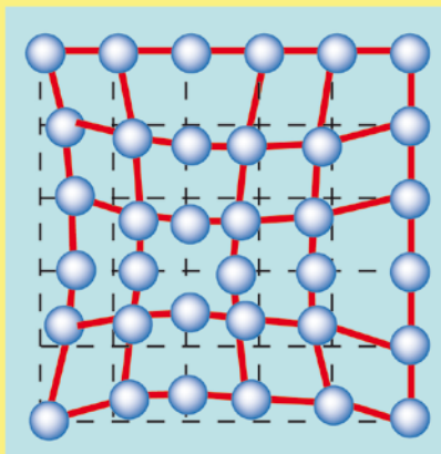
ВАКАНСІЯ
