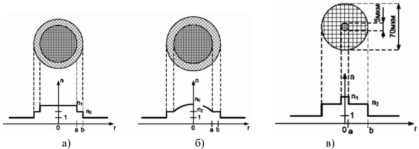
Рисунок 15 – Профіль розподілу показника заломлення та поперечний переріз різних типів оптичних волокон: а) багатомодове східчасте оптоволокно, б) багатомодове градієнтне оптоволокно, в) одномодове оптоволокно
