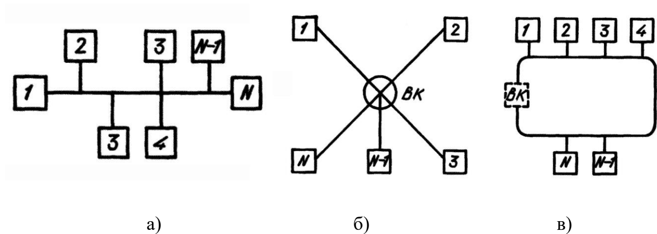
Рисунок 21 – Різновиди базових топологій мереж ВОСПІ: топологія “шина” (а), топологія “зірка” (б), топологія “кільце” (в)
