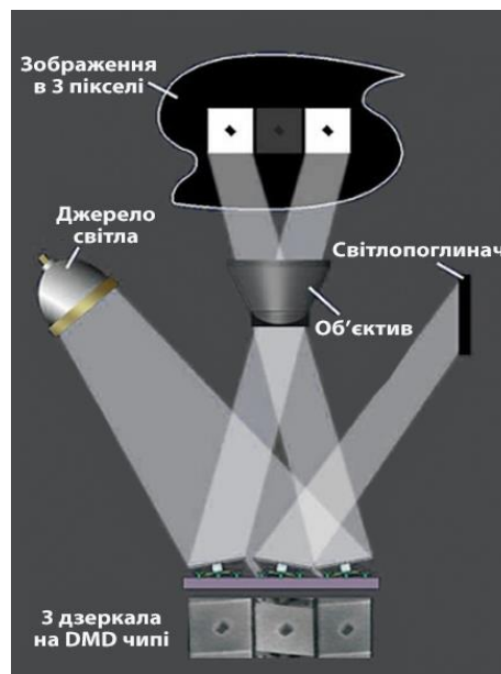
Рисунок 47 – Ілюстрація принципу дії DMD чіпу
