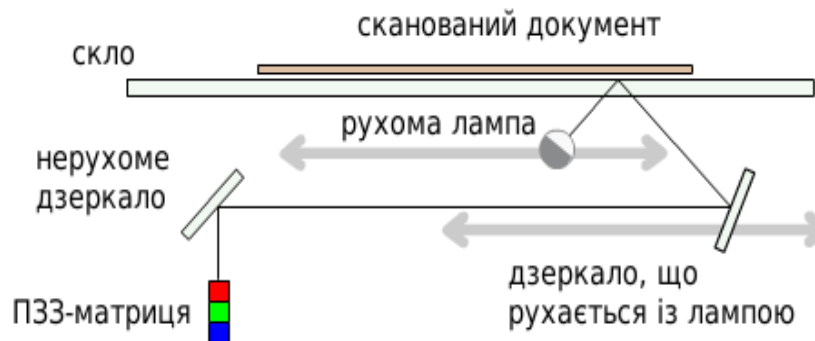
Рисунок 31 – Структурна схема планшетного сканера
