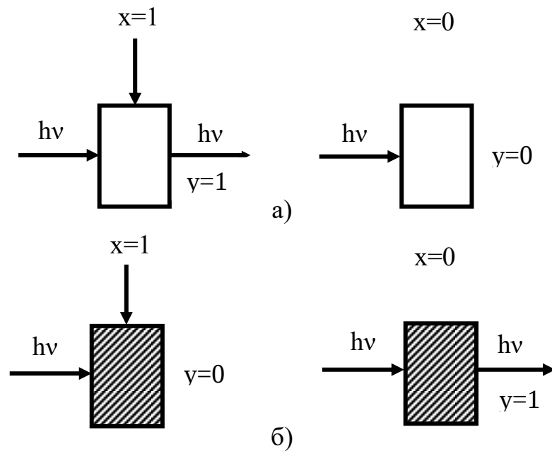
Рисунок 25 – Різновиди найпростіших оптичних логічних елементів:
