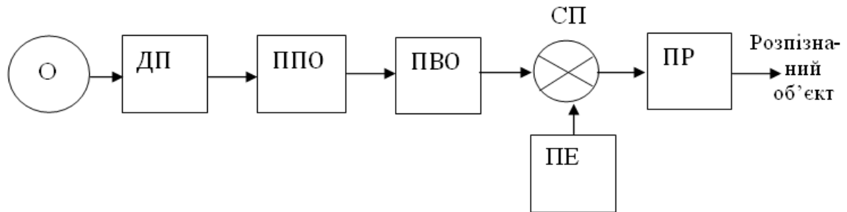
Рисунок 30 – Узагальнена структурна схема системи розпізнавання образів: О – об'єкт; ДП – детектор параметрів об'єкта; ППО – пристрій попередньої обробки параметрів об'єкта; ПВО – пристрій виділення ознак; СП – схема порівняння; ПЕ – пам'ять еталонів; ПР – схема прийняття рішень на розпізнавання
