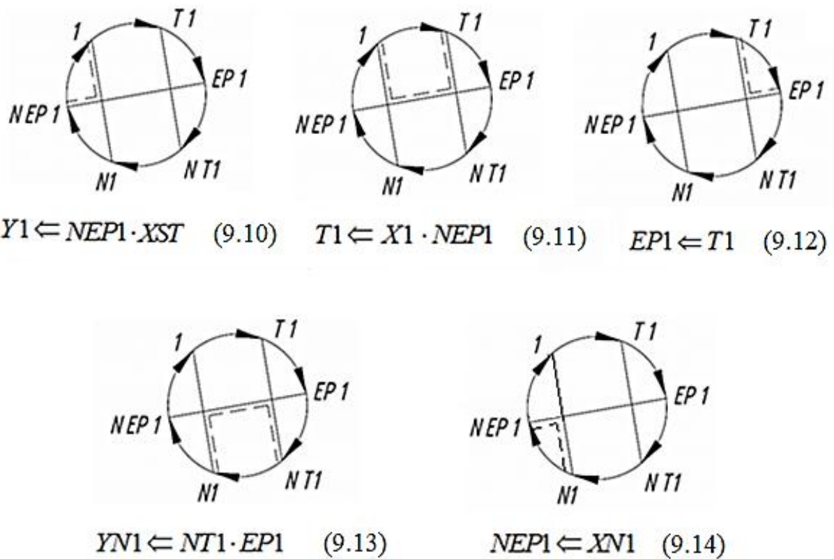
Рис. 9.24. Фрагменти графу при використанні ліній зв'язку (пунктир) для побудови логічних команд керування циклу 1 - 5c - \bar{1}
