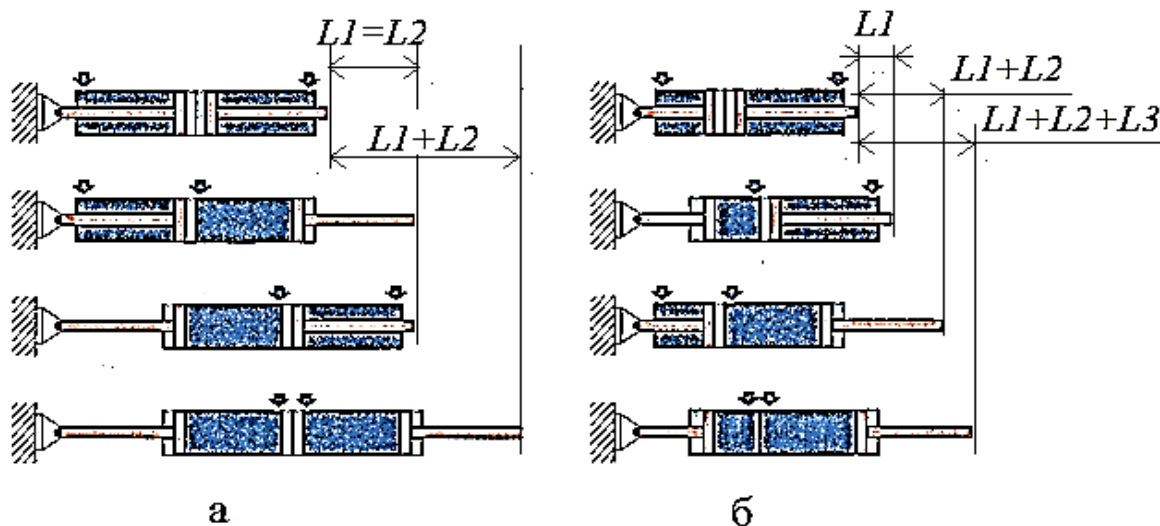
Рис. 6.8. Принципові схеми роботи опозитних циліндрів: а – три позиції штоку, якщо стикуються циліндри з однаковим ходом поршнів ( L1 = L2 ); б – чотири позиції штоку, якщо стикуються циліндри з різним ходом поршнів ( L1 \neq L2 )
