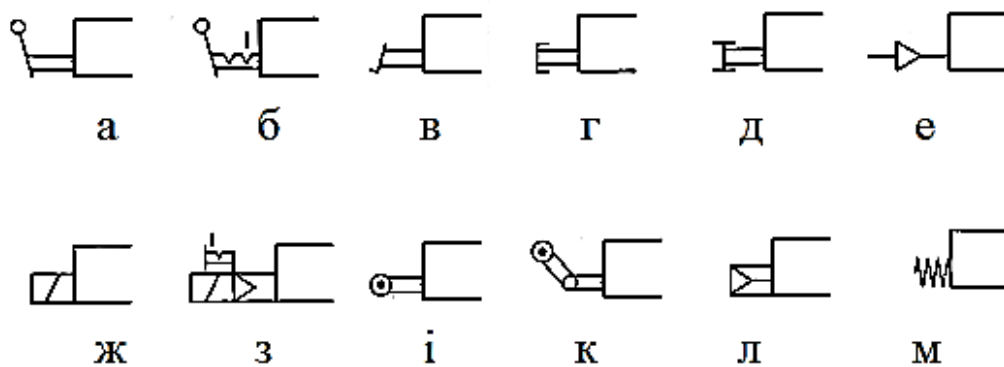
Рис. 1.25. Умовні позначення елементів керування і елементів контролю в схемах типу ПЗ: а – тумблер без фіксації положення; б – тумблер з фіксацією положення; в – педаль; г – кнопка; д – кнопка з фіксацією; е – пневматичне керування; ж – електромагнітне керування; з – електропневматичне керування з ручним дублюванням включення; і – механічне керування з роликовим штовхачем; к – механічне керування з роликовим штовхачем-важелем; л – повернення за допомогою пневматичної пружини; м – повернення за допомогою механічної пружини.
