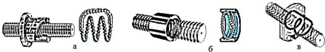
Рис. 5.15. Типи рециркуляції (системи ротації) сталевих кульок кульково-гвинтових передач: а – зовнішня ( тип 1 ); б – внутрішня ( тип 2 ); в – з кінцевою системою повернення ( тип 3 )
