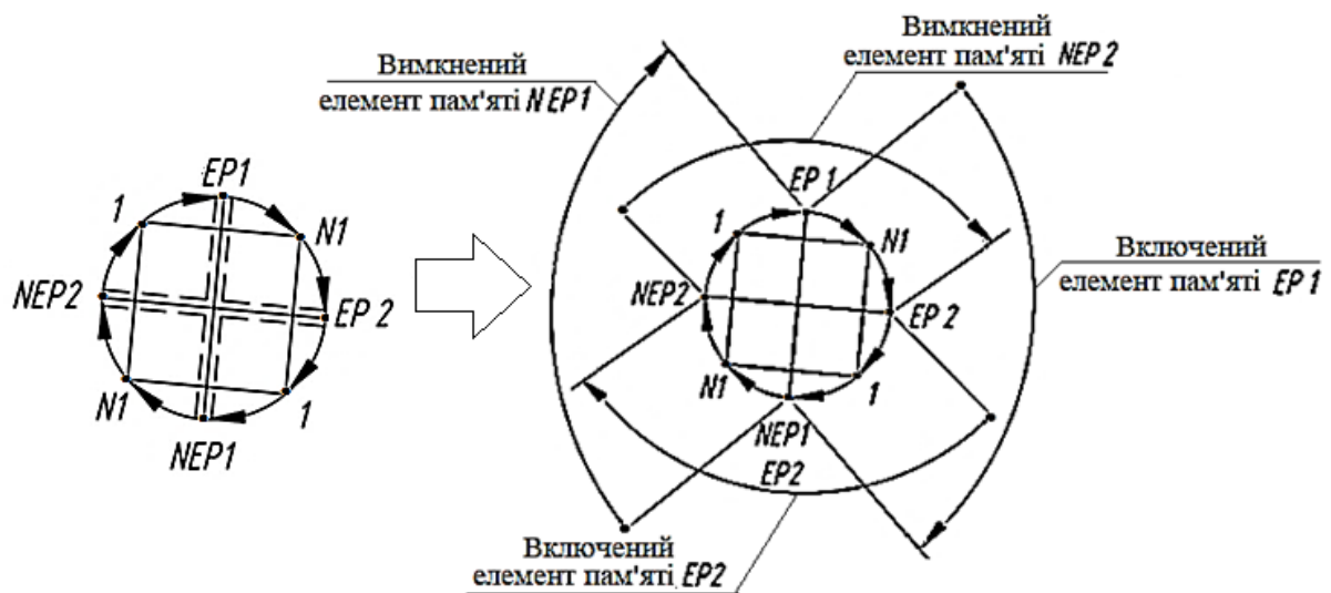
Рис. 9. 39. Граф циклу 1 \rightarrow EP1 \rightarrow N1 \rightarrow EP2 \rightarrow 1 \rightarrow NEP1 \rightarrow N1 \rightarrow \rightarrow NEP2 із зонами існування сигналів включеного ( EP1 та EP2 ) стану і вимкненого ( NEP1 та NEP2 ) стану елементів пам'яті
