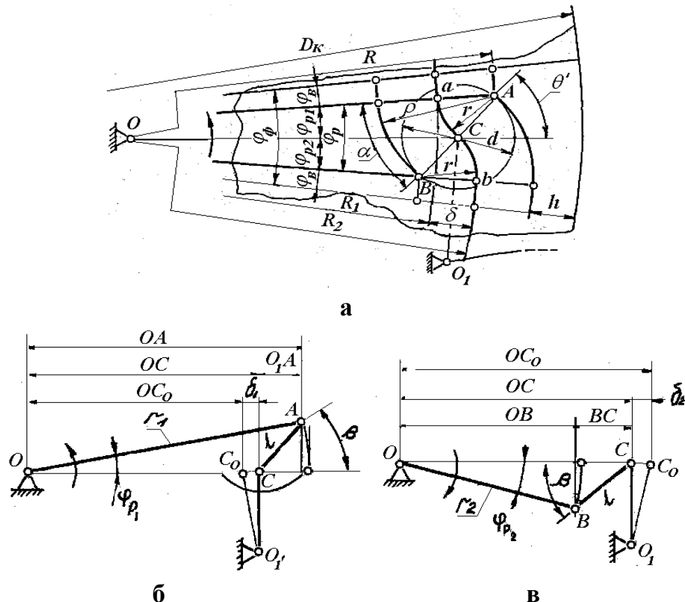
Рис. 2.6. Схема (а) типового фазового кута – кроку кулачкового програмоносія та еквівалентні замінюючи механізми: б - механізм еквівалентний увігнутої частині «аС» профілю «аСb» програмоносія; в - механізм еквівалентний опуклої частини профілю «Сb» профілю «аСb» програмоносія
