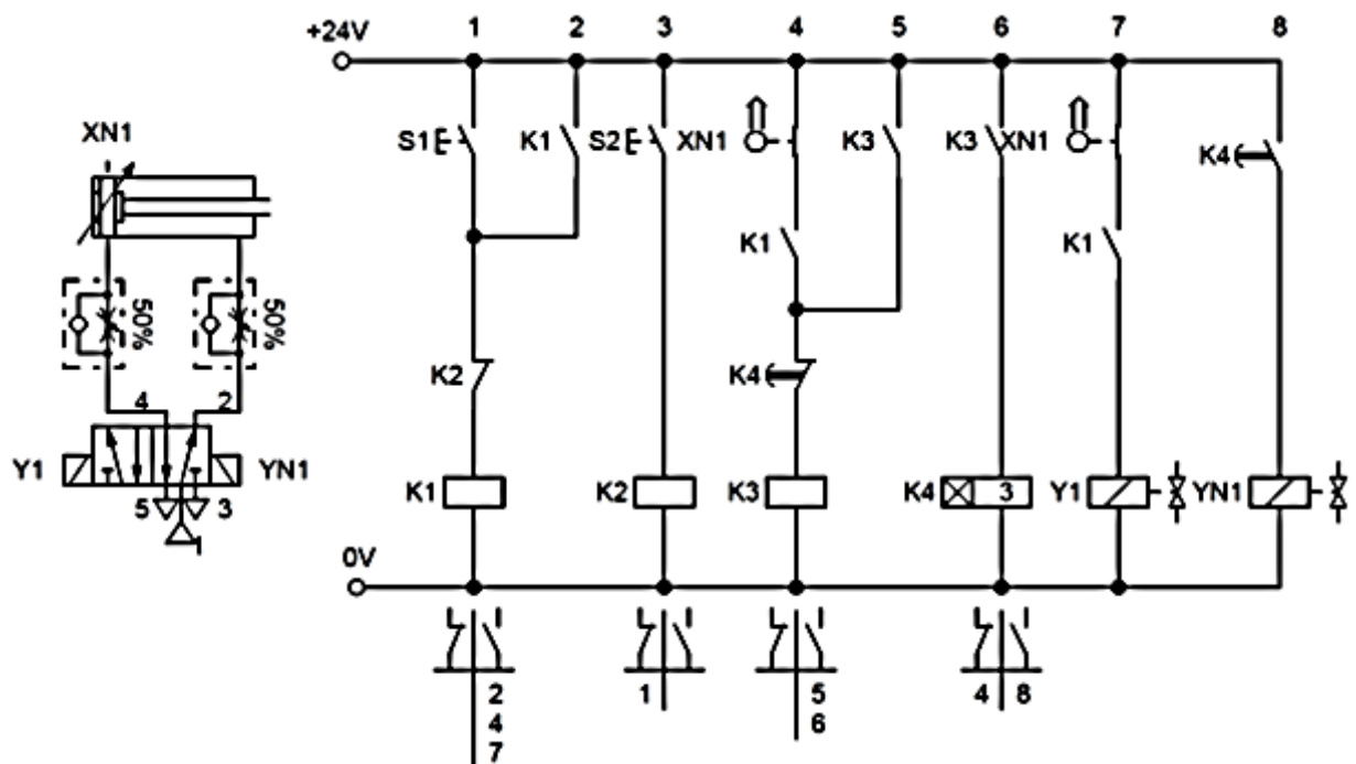
Рис. 9.9. Комбінована схема без контролера для виконання циклу 1 - \bar{1} з Бістабільним керуванням та одним кінцевим вимикачем
