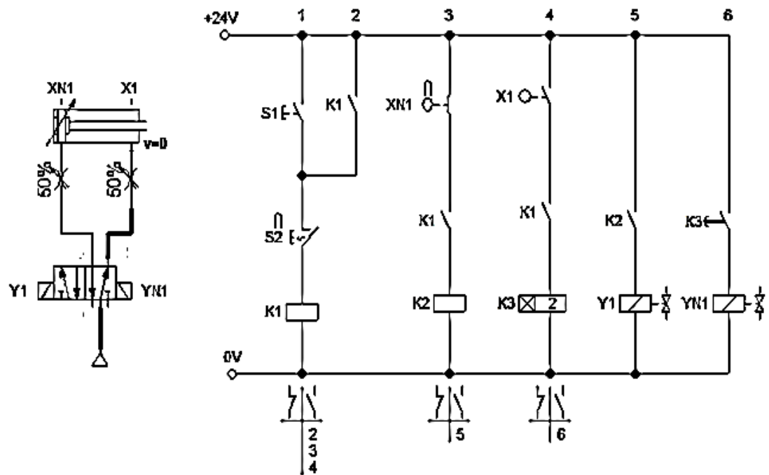
Рис. 8.34. Комбінована схема циклу «1–N1» з Бістабільним керуванням, двома кінцевими вимикачами та реле часу
