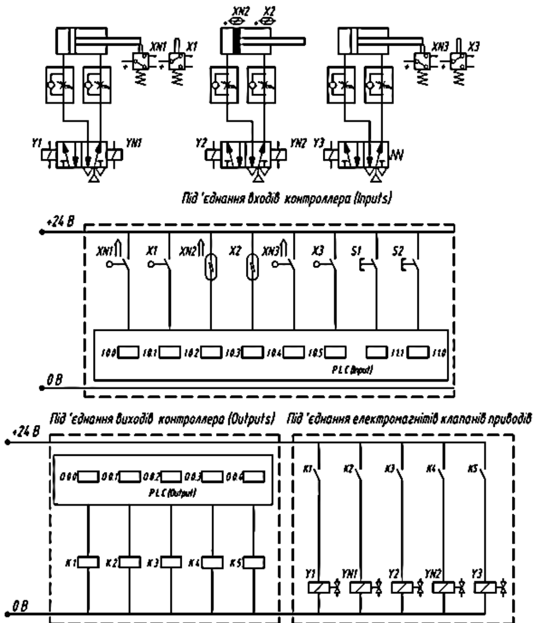
Рис. 9.43. Схема СЗ з контролером для виконання циклу
