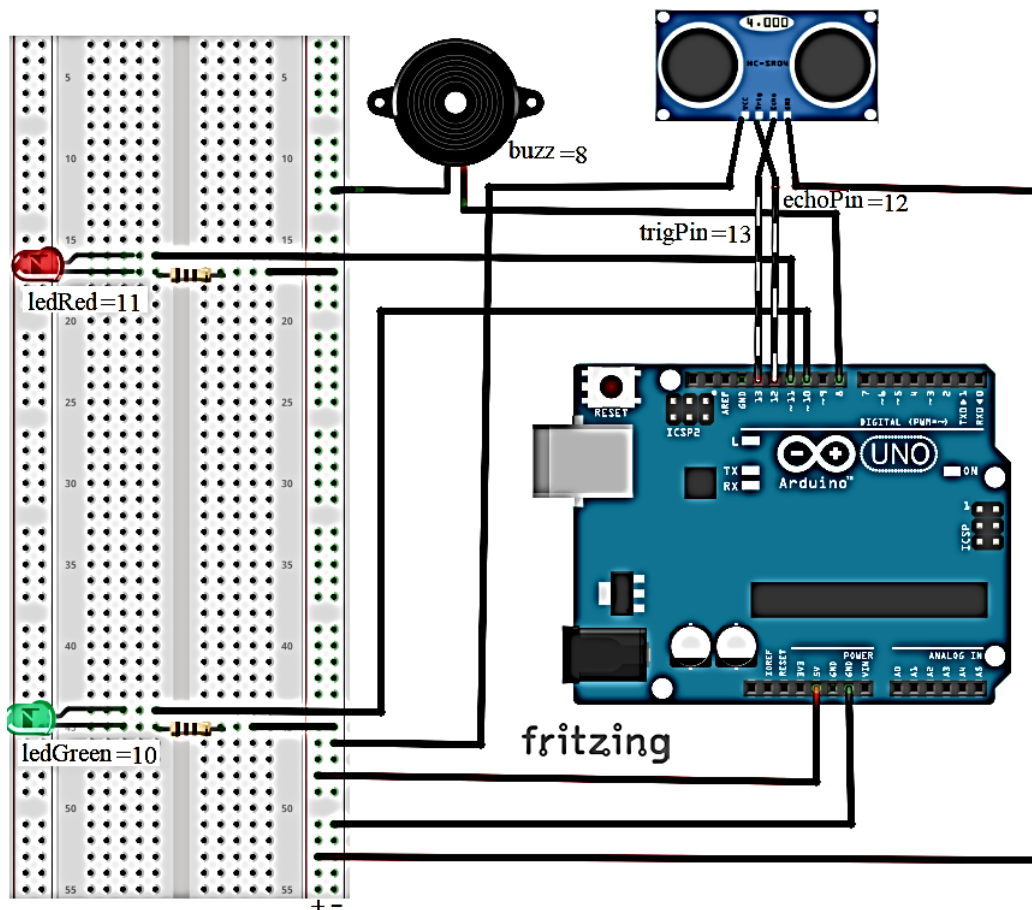
Рис. 7.26. Монтажна схема підключення ультразвукового датчика HC-SR04 до контролера Arduino UNO
