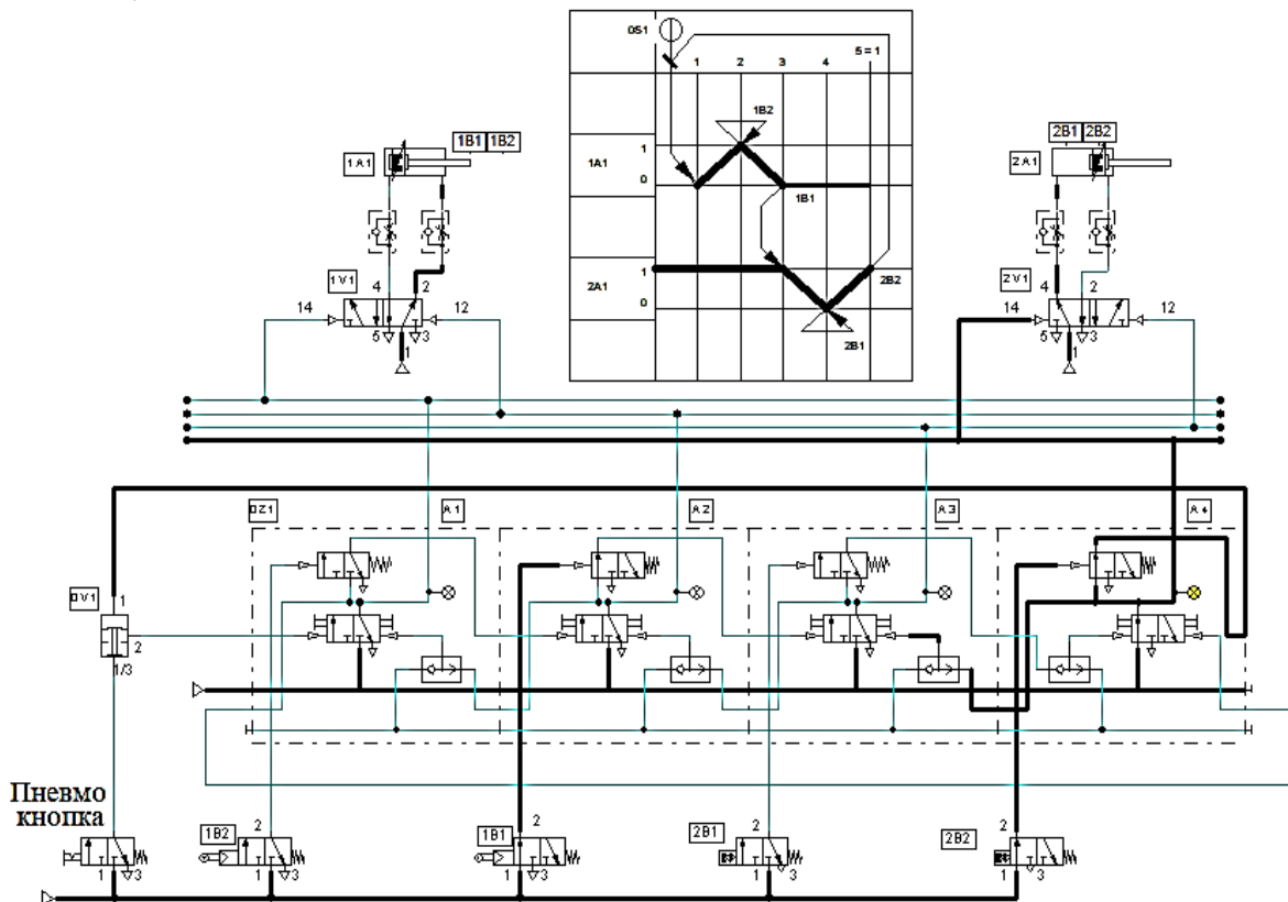
На рис. 8.52 наведена функціонально-адекватна пневматична схема (тип ПЗ) циклу 1 \rightarrow \bar{1} \rightarrow \bar{2} \rightarrow 2 при включеному компресорі і не натиснутої пневмокнопки.
