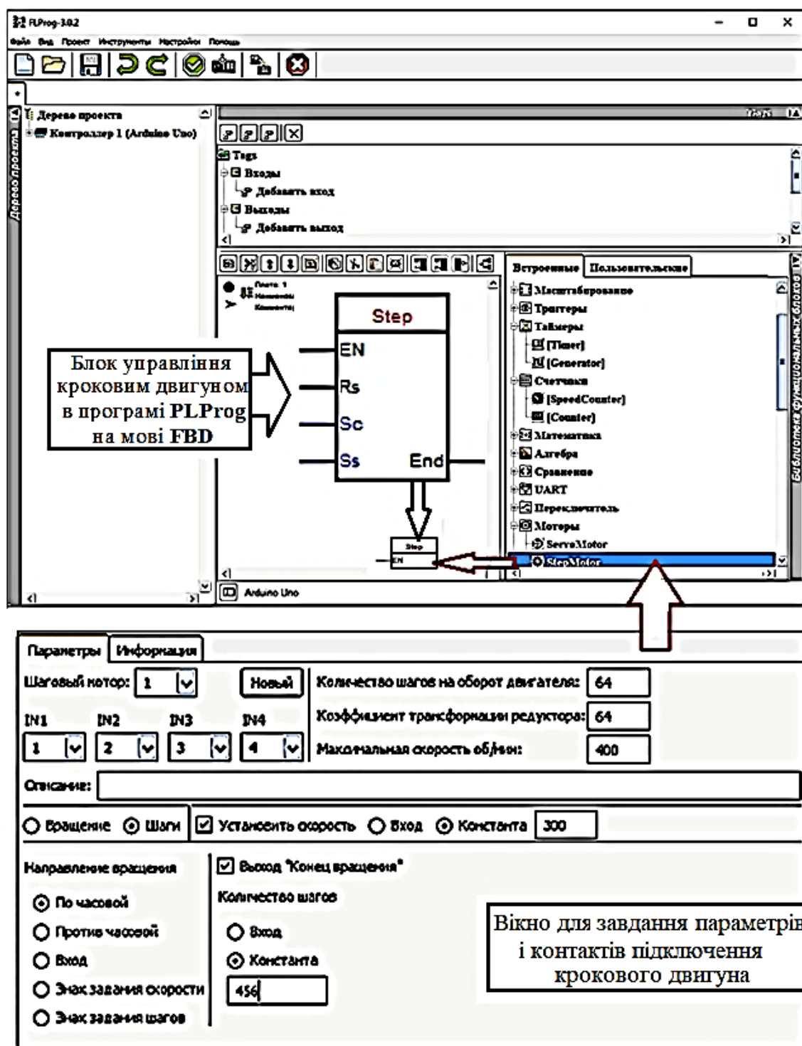
Рис. 4.30. Фрагменти рабочего поля проекта для програмування крокового двигуна в програмі FLProg на мові FBD для наступної компіляції програми на мові Arduino C
