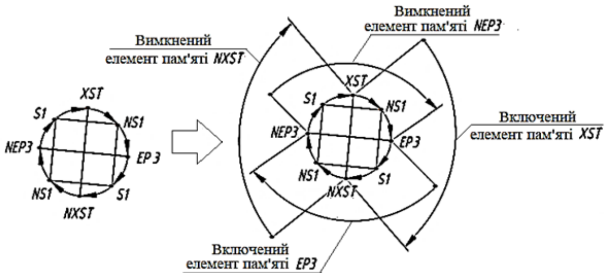
Рис. 9.40. Функціональний граф циклу натиснення кнопки (а) і зон обов'язкового існування сигналів включеного ( XST та EP3 ) і вимкненого ( NXST та NEP3 ) стану додаткових елементів пам'яті
