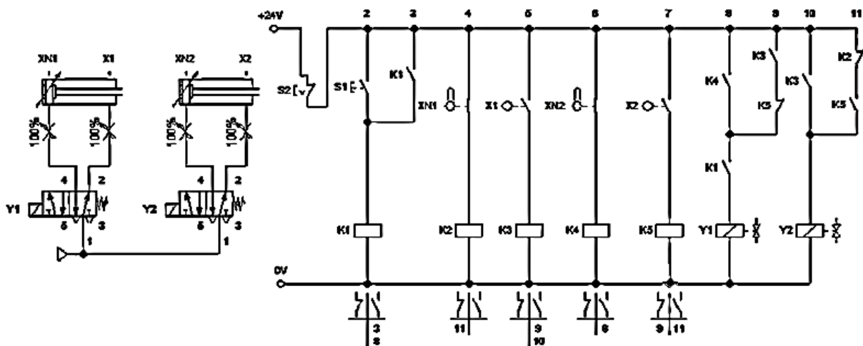
Рис. 8.43. Комбінована схема циклу (тип СЗ) 1 \rightarrow 2 \rightarrow \bar{1} \rightarrow \bar{2} з МОНОстабільним керуванням та чотирма кінцевими вимикачами
