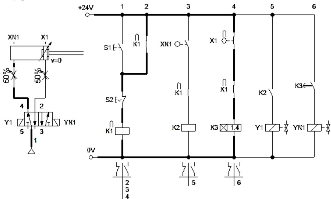
Рис. 8.35. Скриншот анімації циклу «1–N1» з Бістабільним керуванням з двома кінцевими вимикачами та реле часу
