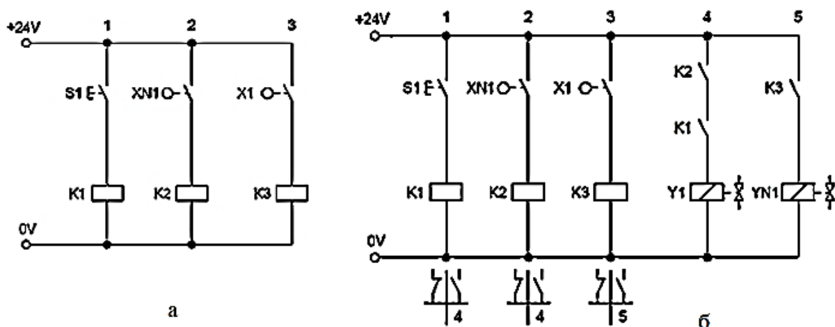
Рис. 8.6. Фрагменти електричної схеми (тип Е3) для входних сигналів - кнопки пуск S1 і кінцевих вимикачів XN1 та XN1: а – прямого включення електромагнітів Y1 і YN1; б – непрямого включення електромагнітів Y1 і YN1
