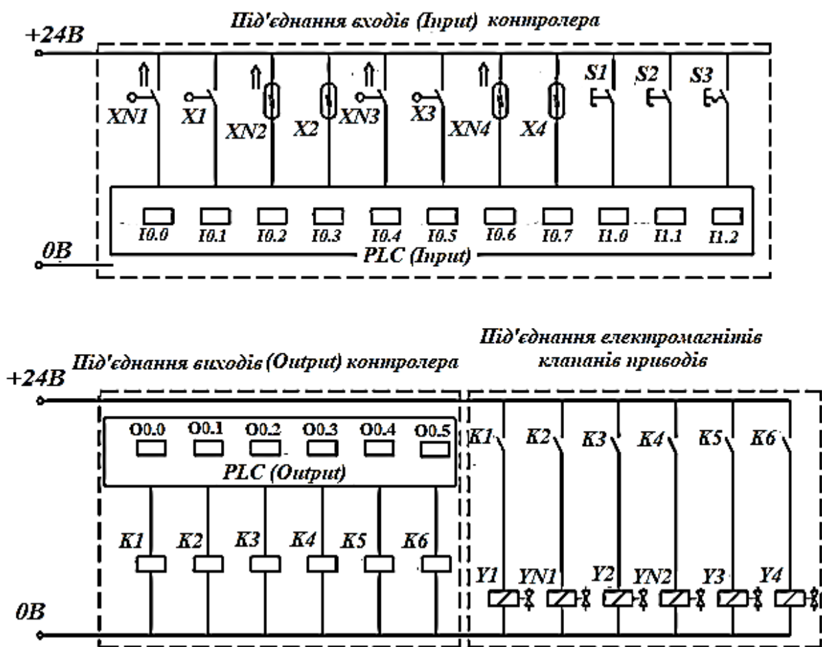
Рис. 9.3. Приклад підключення датчиків, реле, електромагнітів пневматичних розподільників до шини входів (Input), шини виходів (Output) та джерела живлення
