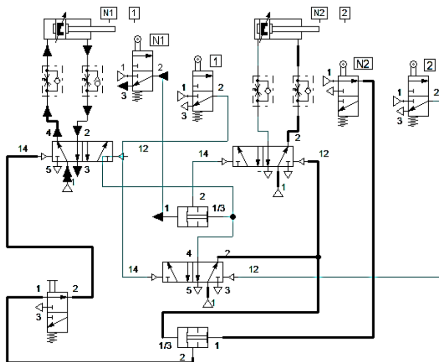
Рис. 8.55. Пневматична схема циклу 1 – N1– 2 – N2 (крок 1) – натиснута пневмокнопка і початок руху поршня першого пневмоцилінду
