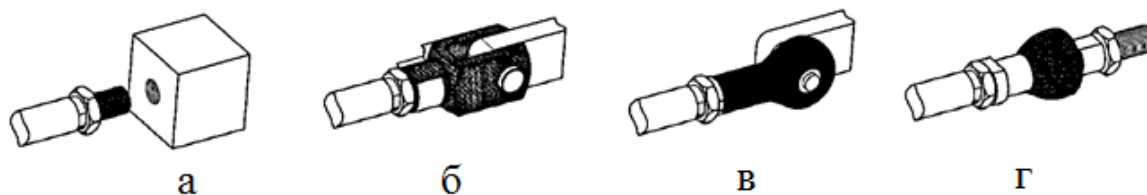
Рис. 6.21. Варіанти з'єднань штоку поршня з веденою ланкою передавальних механізмів: а – різьбове; б – вільчасте; в – сферичною кінематичною парою; г –кульовим шарніром
