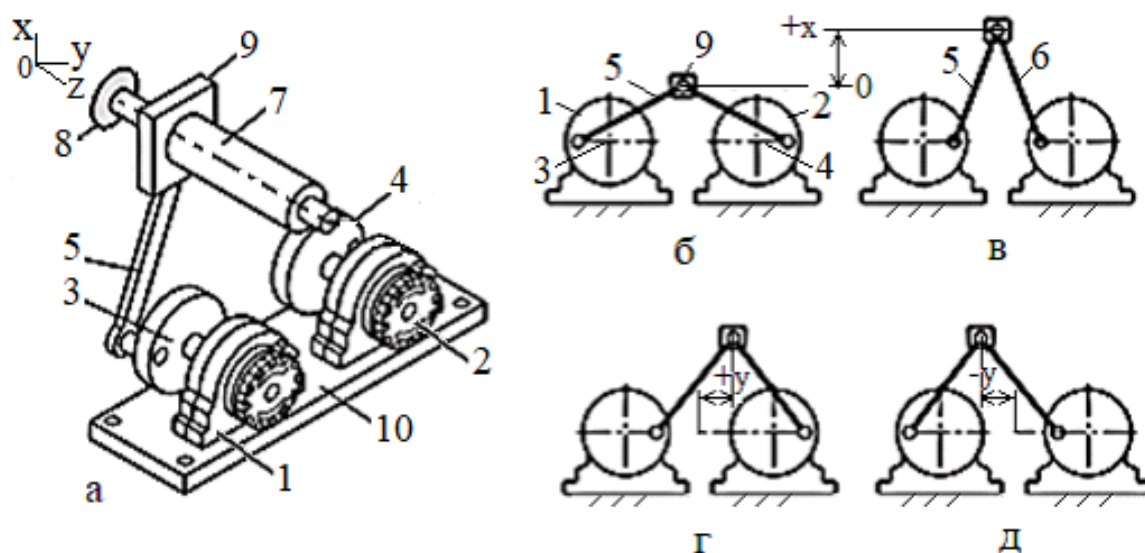
Рис. 6.23. Двукоромисловий чотири позиційний 3D-механізм з програмованими пневмоприводами: а – конструктивне-кінематична схема; б і в – програмовані переміщення робочого органу по осі 0X; г і д – програмовані переміщення робочого органу по осі 0Y
