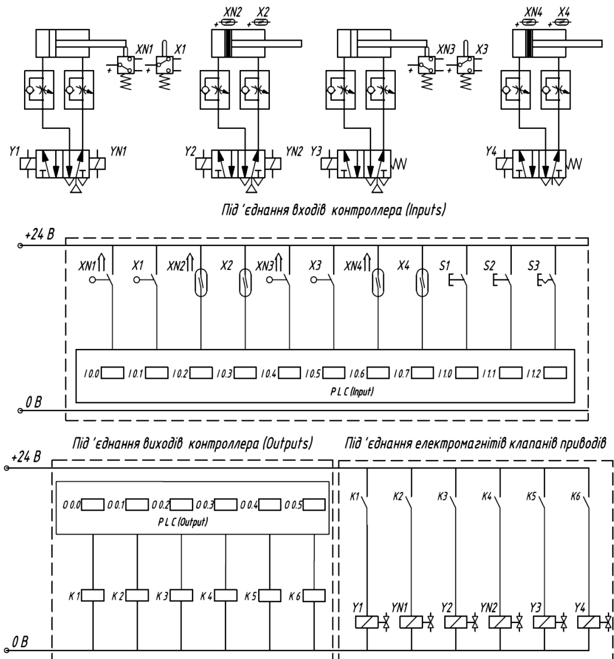
Рис. 9.47. Комбінована схема з контролером для виконання циклової мехатронної системи з двома альтернативними циклами: циклом 1, 2 – 3 – 4 – \bar{1} – \bar{2} – \bar{3} – \bar{4} та циклом 1 – 2 – 3 – \bar{2} – \bar{3} – 2 – \bar{1} – 4 – \bar{2} – \bar{4}
