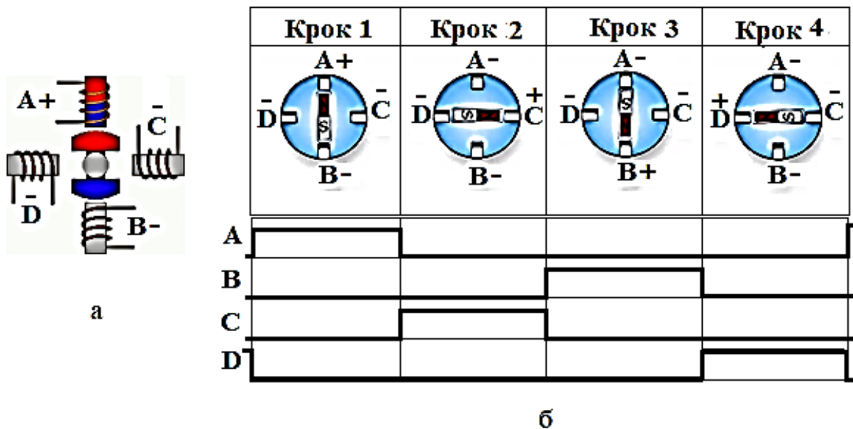
Рис. 4.8. Повно кроковий режим роботи біполярного крокового двигуна ( варіант 1 ): а – живлення котушки А для кроку 1; б – положення ротора (постійних магнітів) для чотирьох тактів (чотири кроку) A \rightarrow C \rightarrow B \rightarrow D програмного почергового перемикавання по одній фазі статора для одного циклу обороту ротора
