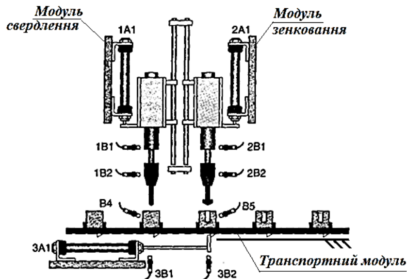
Рис. 2.11. Приклад застосування циклового програмного керування (ЦПК) в свердлильно-фрезерувальні верстаті
