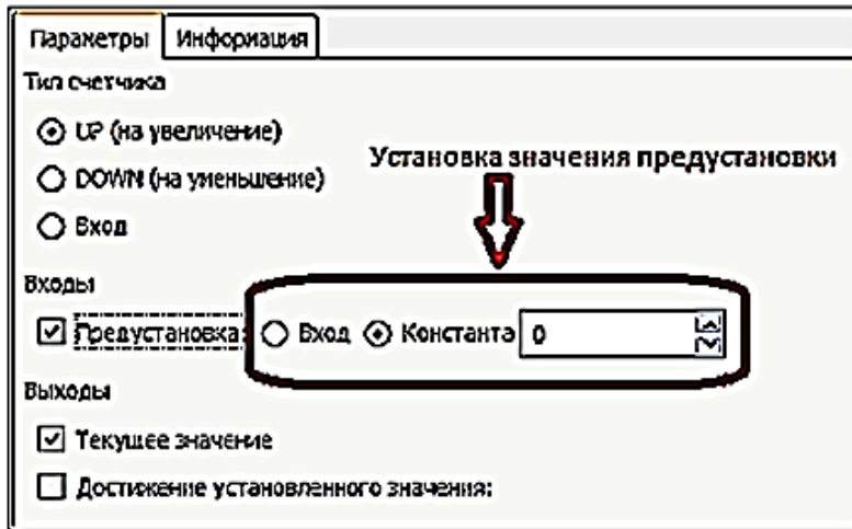
Рис.7.22. Вікно активного стану опції «Попередня установка» параметрів входу лічильника
