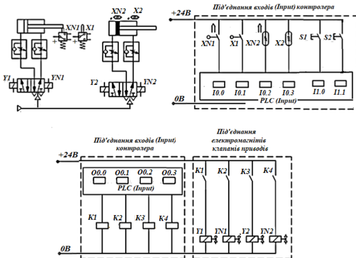
Рис. 9.26. Комбінована схема з контролером для виконання циклу 1 \rightarrow 2 \rightarrow \bar{1} \rightarrow \bar{2} з Бістабільним керуванням
