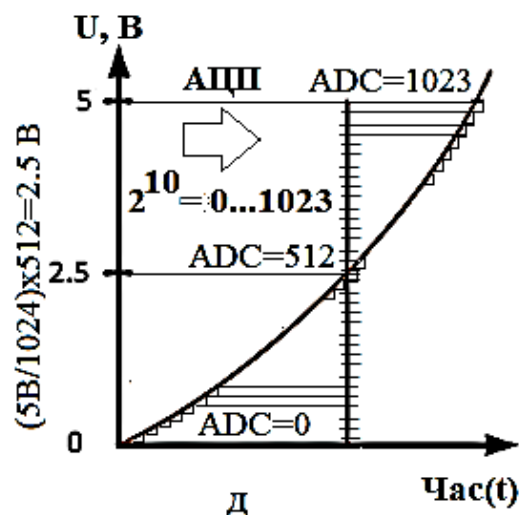
Рис. 7.1. Принципові схеми перетворення аналогового сигналу датчика у дискретний (цифровий сигнал) UNO: а – аналоговий сигнал датчика і цифрові сигнали після аналого-цифрового перетворення ; б – при
