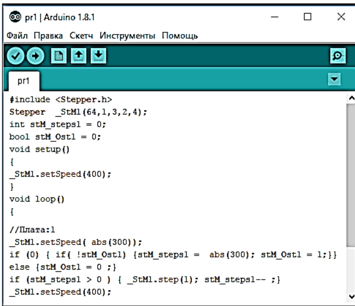
Рис. 4.31. Програма на мові Arduino_C після компіляції програми FLProg на мові FBD
