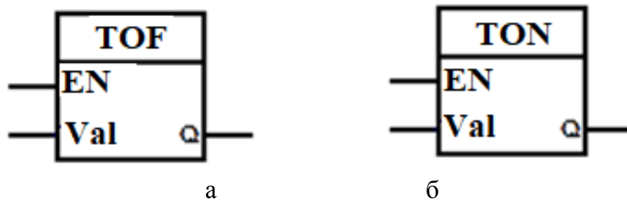
Рис. 7.14. Програмні блоки програми FLProg : а – таймер типу TOF (Timer O ff-delay) із затримкою вклучення , який формує затримку часу по переднього фронту імпульсу (рис. 7.15,а), що подаються на вхід «EN» (від. E nable - увімкнути); б – таймер типу TON (Timer O n-delay) із затримкою вимкнення , який формує затримку часу по заднього фронту імпульсу (рис. 7.15,б), що також подаються на вхід «EN»
