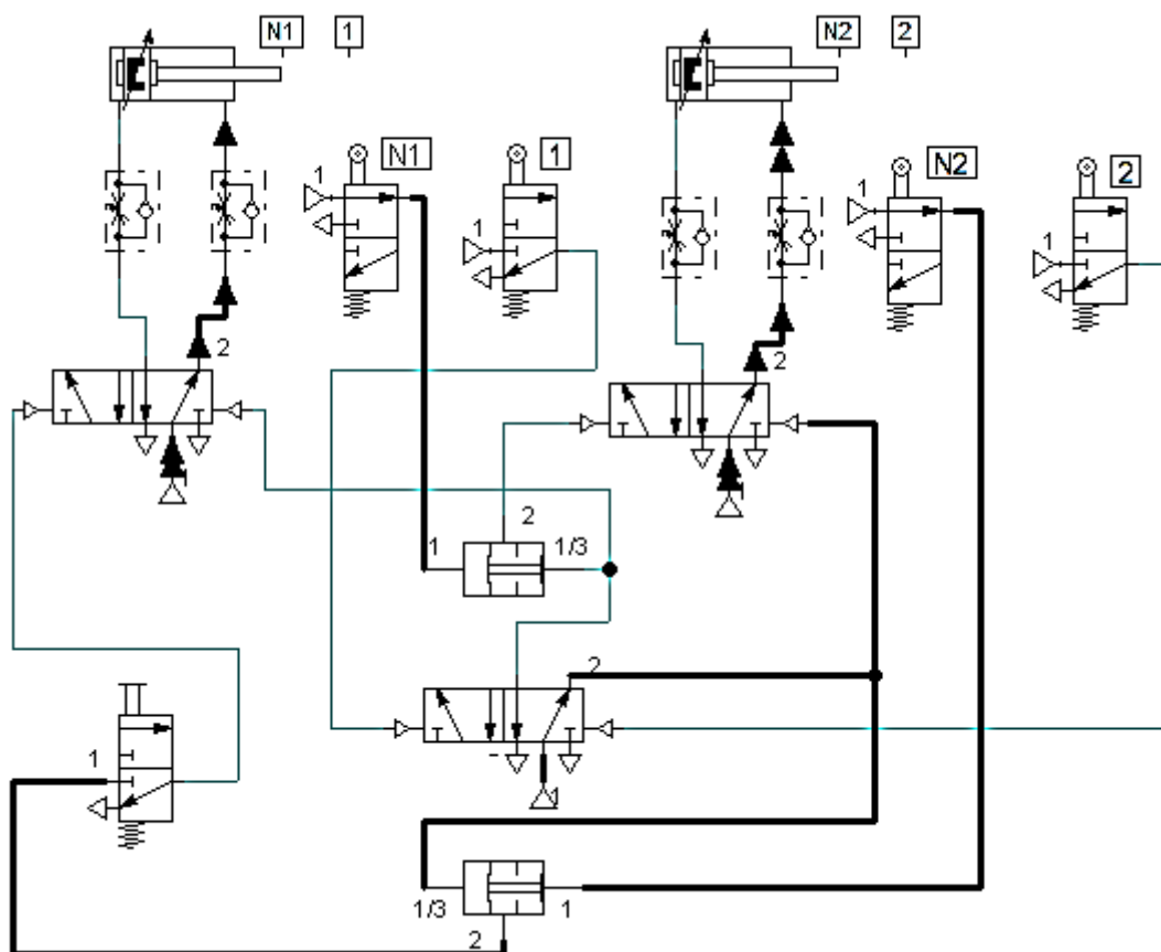
Рис. 8.60. Пневматична схема циклу 1 – N1 – 2 – N2 (крок 6) – повернення виконавчих механізмів в початковий стан (закінчення циклу)
