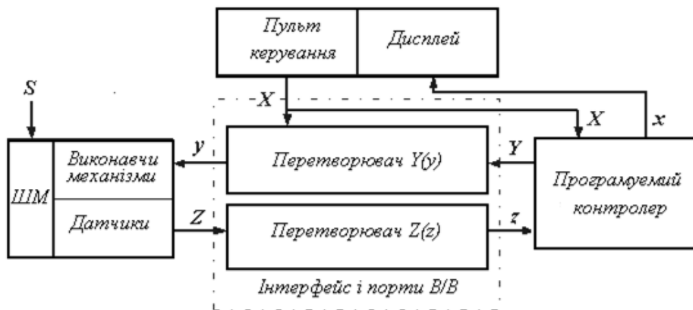
Рис. 2.2. Інтерфейс програмуючого контролера в блок-схемі комп'ютерно-інтегрованої швейної машини з цифровим керуванням
