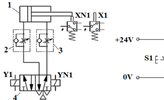
Рис. 8.5. Схема типового мехатронного модуля з Бістабільним керуванням
