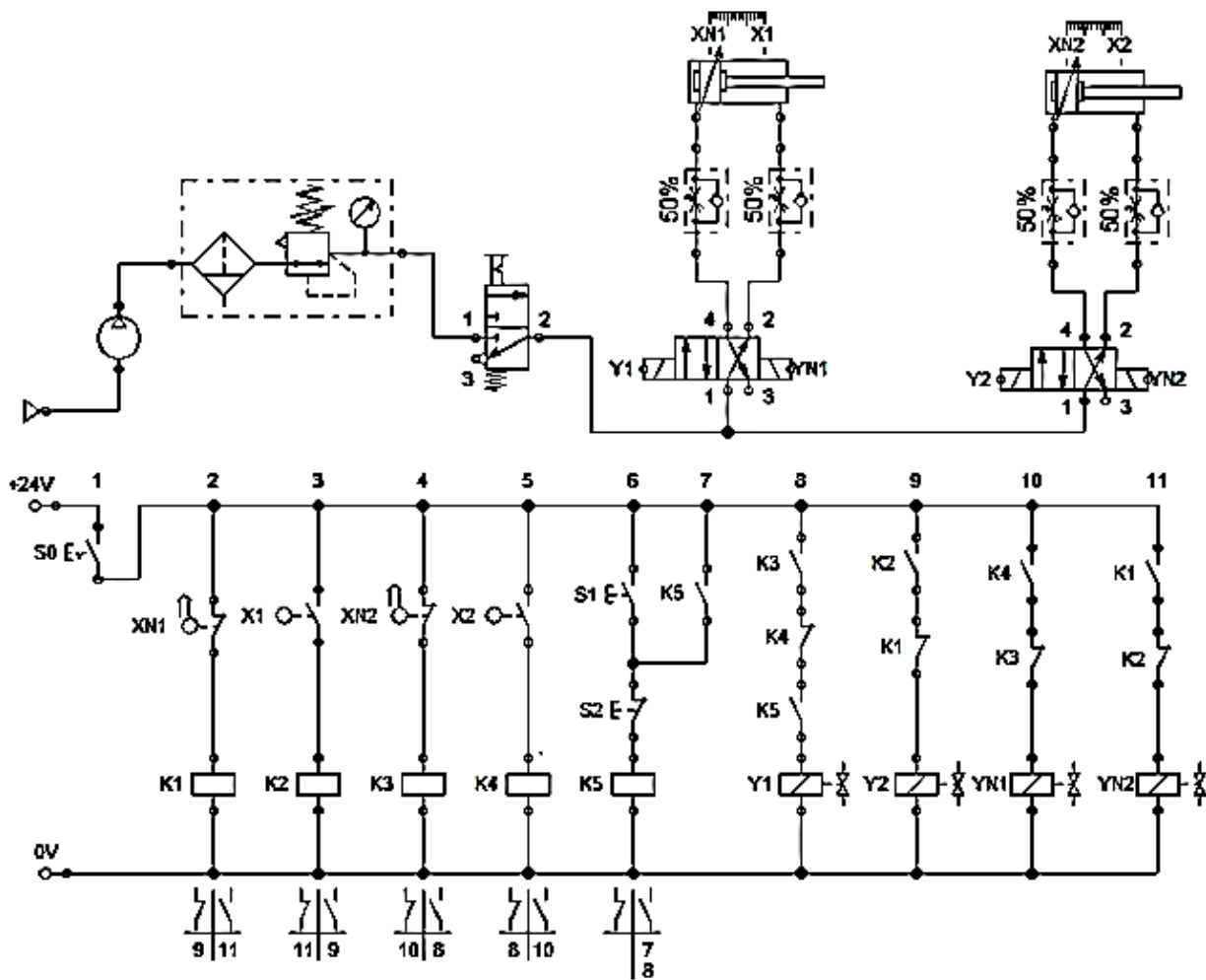
Рис. 8. 38. Комбінована схема циклу \Rightarrow 1 \rightarrow 2 \rightarrow \bar{1} \rightarrow \bar{2} з Бістабільним керуванням двома виконавчими механізмами
