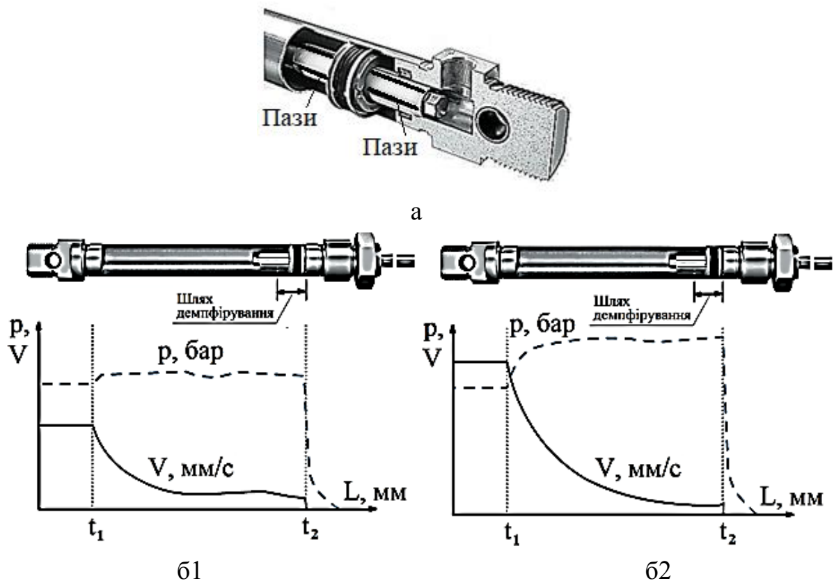
Рис. 6.3. Якісні характеристики поршня з подовженою довжиною демпфера з використанням поздовжніх пазів у демпфіруючій частині поршня (тип PPS демпфірування): а - 3D-схема конструкції; б – графіки динаміки роботи при малої (б1) і великої (б2) швидкості
