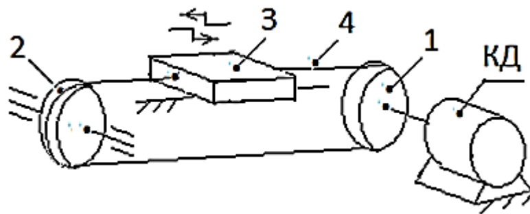
Рис. 5.1. Кінематична 3D-схема модуля програмованих переміщень з тросової передачею
