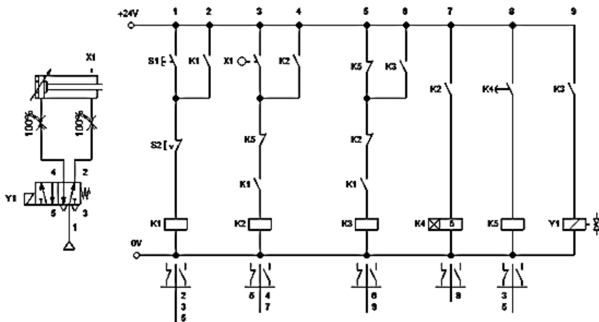
Рис. 8.20. Комбінована схема циклу «1–N1» з МОНОстабільним керуванням з одним кінцевим вимикачем для виконання та затримкою в часі 5 с при втягнутому положенні поршня для реалізації циклу «1–N1» з МОНОстабільним керуванням та з одним кінцевим вимикачем
