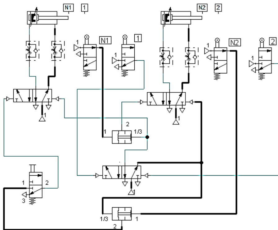
Рис. 8.54. Початковий стан схеми на рис. 8.53 після включення компресора і не натисканній пневмокнопки «Start» S1
