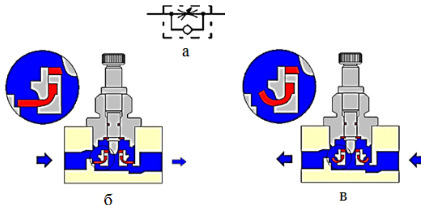
Рис. 1.9. Дросель зі зворотнім клапаном: а – умовне позначення на схемах типу ПЗ; б – конструктивна схема для стану при регулювання витрати повітря у прямому напрямку; в – конструктивна схема для стану при вільному пропусканні повітря у зворотному напрямку
