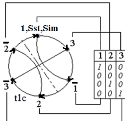
Рис. 3.8. Функціональний граф і таблиця відповідності:
