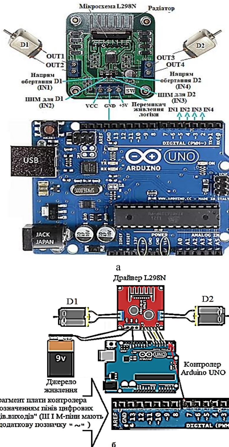
Рис. 4.26. Приклад монтажної схеми підключення до контролера Arduino UNO драйвера на мікросхемі L298N непрямого керування двома двигунами D1 і D2 постійного струму: а – без підключеного джерела живлення; б – з підключеним джерелом живлення і фрагментом плати контролера
