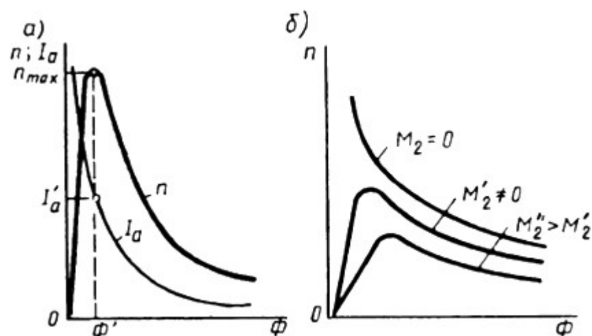
Рисунок 42.1 – Регулювальні характеристики двигуна паралельного збудження
