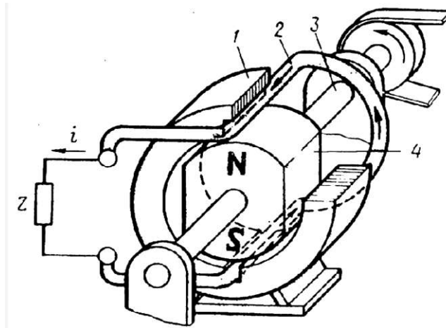
Рисунок 8.1 – Спрощена модель синхронного генератора
