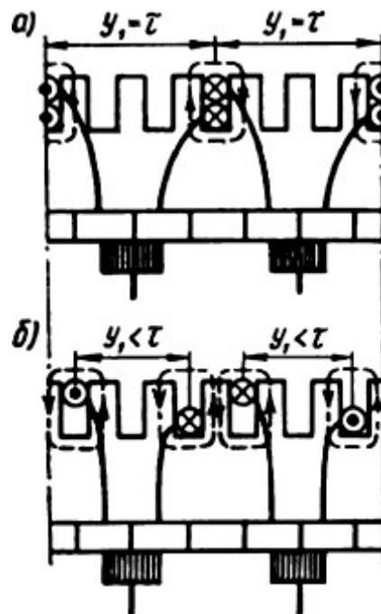
Рисунок 39.2 – Магнітний зв'язок одночасно комутуючих секціях: а – при повному кроці; б – при вкороченому кроці обмотки якоря
