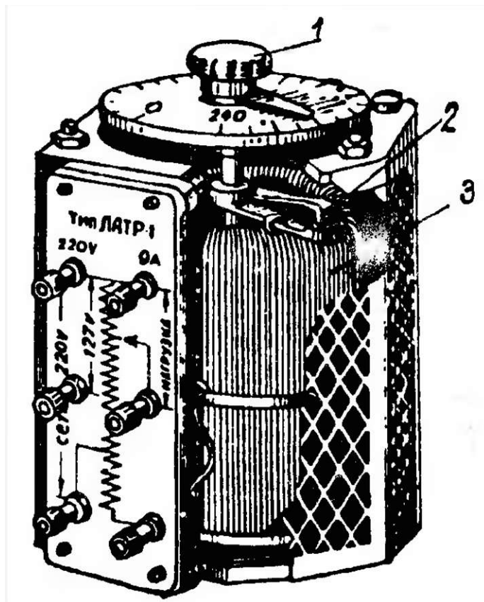
Рисунок 6.5 – Регульовальний однофазний автотрансформатор:
