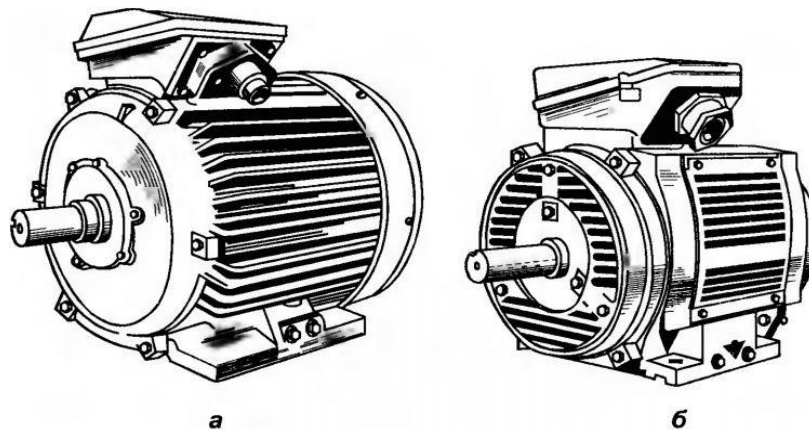
Рисунок 23.1 – Асинхронні двигуни серії 4А: а – закритого виконання, що обдувається; б – захищеного виконання
