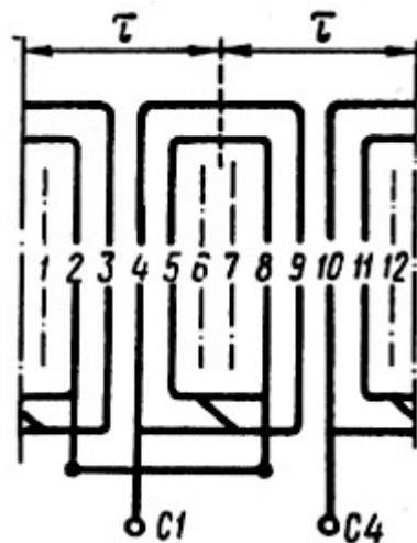
Рисунок 12.3 – Однофазна одношарова обмотка статора: 2p=2 ; Z_1 = 12 ; q_1 =
