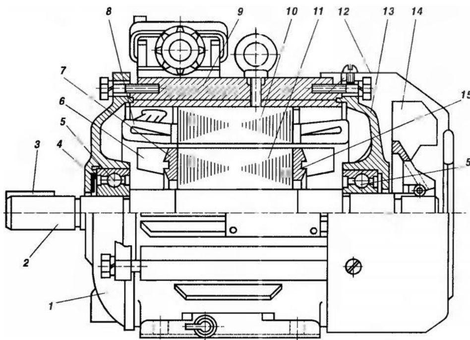
Рисунок 23.2 – Асинхронний електродвигун єдиної серії 4А: 1,13 – передній і задній щити; 2 – вал; 3 – шпонка; 4 – настановна пружина; 5 – підшипник; 6 – крильчатка; 7-11 – сердечники статора й ротора; 12 – кожух вентилятора; 14 – вентилятор; 15 – балансувальний грузик
