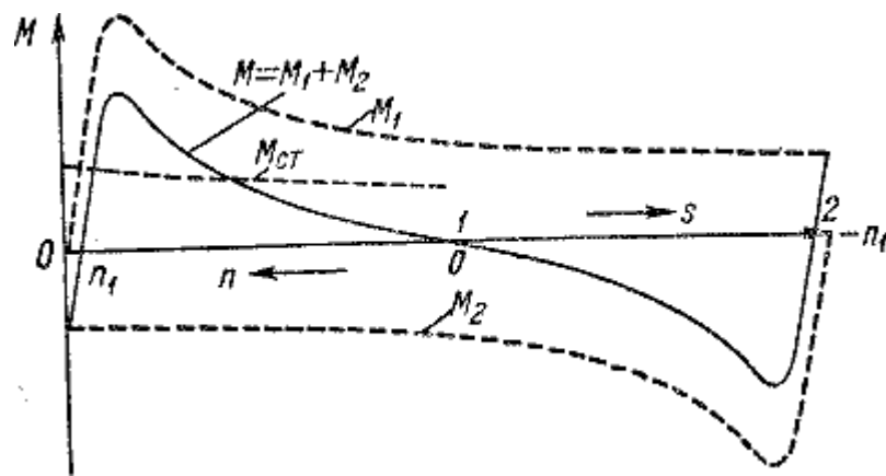
Рисунок 20.2 – Криві моментів однофазного двигуна
