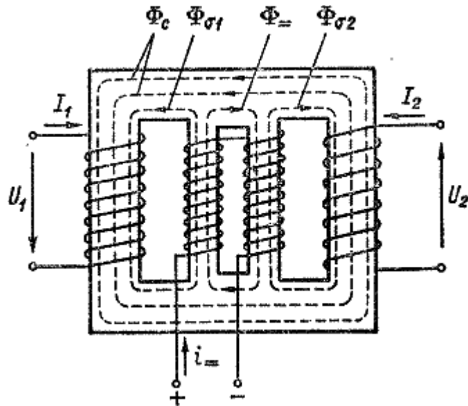
Рисунок 7.3 – Однофазний трансформатор з підмагнічуючим шунтом
