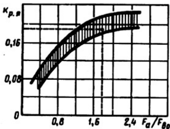
Рисунок 37.1 – Графік залежності k_{p.я.} = f(F_a / F_{a0})
