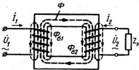
Рисунок 3.1 – Магнітні потоки в однофазному трансформаторі
