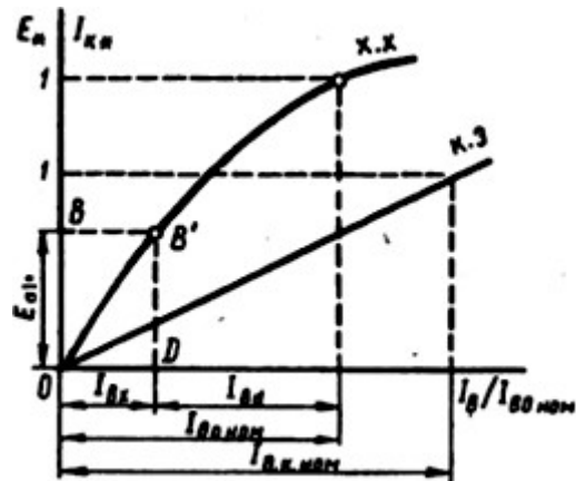
Рисунок 29.3 – Визначення складових струму короткого замикання
