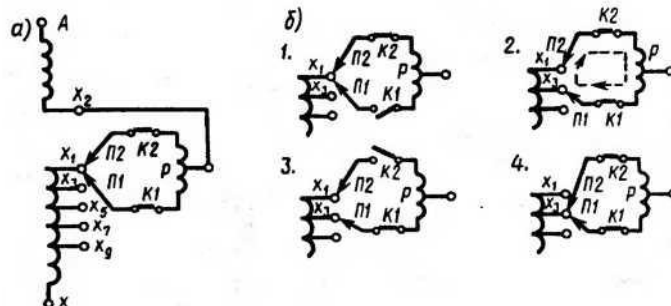
Рисунок 5.5 – Послідовність перемикання контактів під навантаженням
