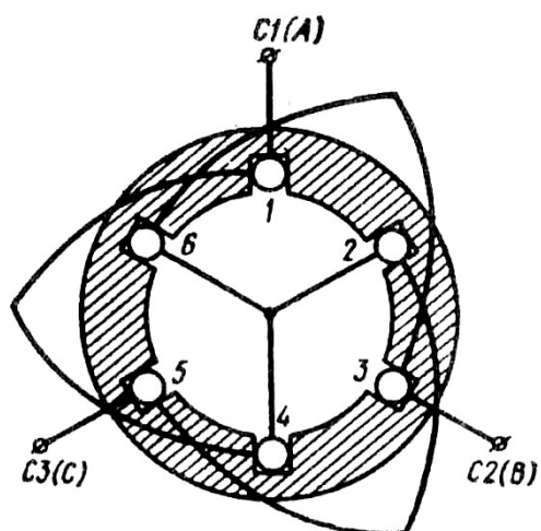
Рисунок 15.2 – Статор з трифазною обмоткою
