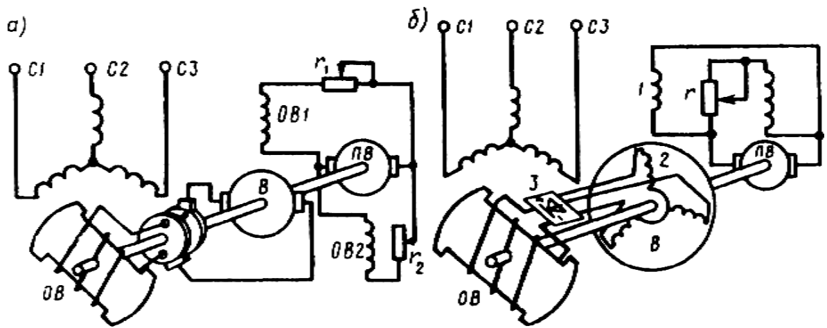
Рисунок 26.1 – Контактна (а) і безконтактна (б) системи електромагнітного збудження синхронних генераторів
