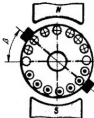
Рисунок 36.2 – Наведення ЕРС в обмотці якоря при зсуві щіток з
