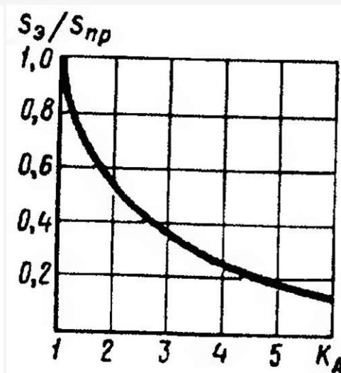
Рисунок 6.3 – Залежність S_e/S_{нр} від коефіцієнта трансформації автотрансформатора
