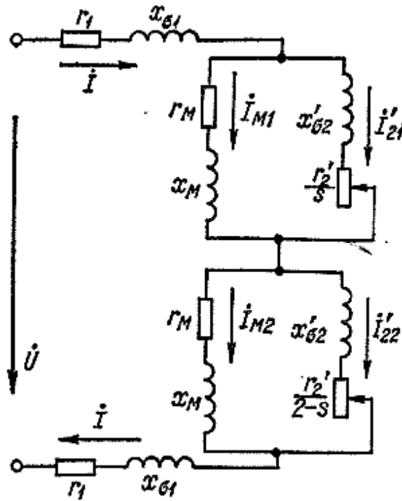
Рисунок 20.3 – Схема заміщення однофазного асинхронного двигуна
