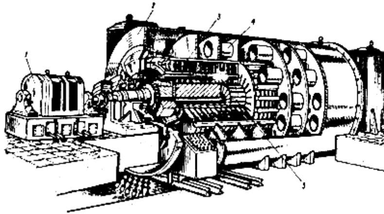
Рисунок 26.5 – Турбогенератор:
