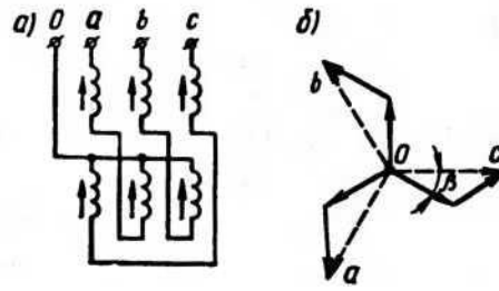
Рисунок 4.3 – З'єднання обмоток в зигзаг
