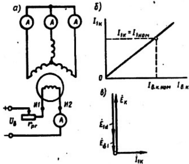
Рисунок 29.2 – Дослід короткого замикання синхронного генератора
