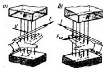
Рисунок 1.2 – Правила «правої руки» й «лівої руки»
