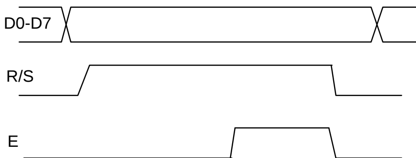
Рисунок 5.12 – Тимчасові діаграми сигналів при виводі символу на РКІ
