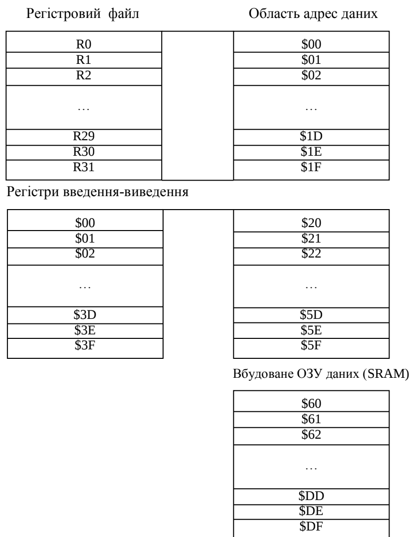
Рисунок 4.17 – Організація пам’яті даних у мікроконтролері AT90S2313
