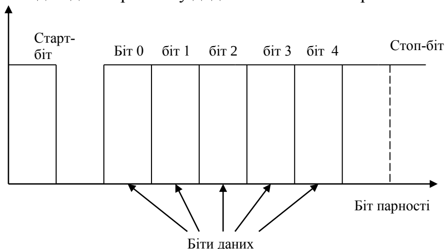
Рисунок 2.28 – Асинхронне послідовне передавання даних
