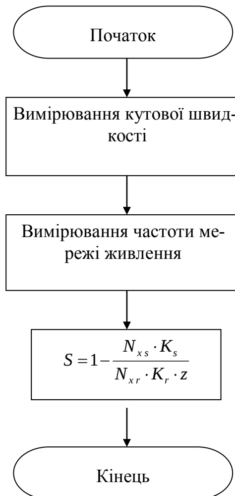
Рисунок 6.17 – Алгоритм роботи мікропроцесорного вимірювача ковзання
