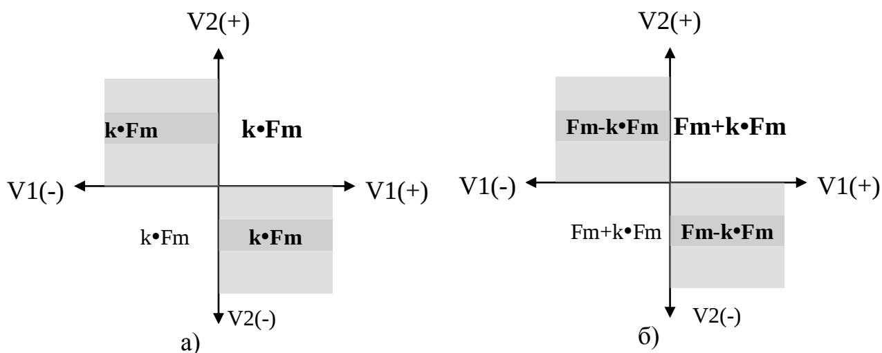
Рисунок 6.11 – Залежність вихідних сигналів від різниці фаз струму і напруги для двоквадрантного (а) і чотириквадрантного (б) вимірювання потужності
