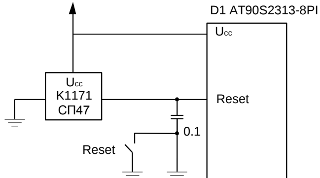
Рисунок 5.4 – Схема підключення супервайзера живлення
