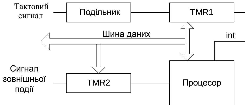
Рисунок 2.21 – Реалізація тахометра
