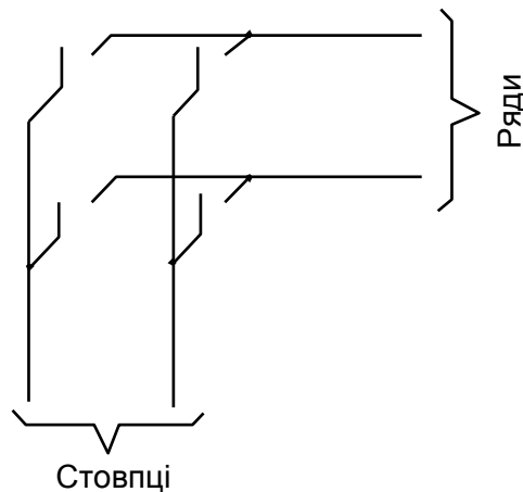
Рисунок 5.10 – З'єднання ключів в матричній клавіатурі
