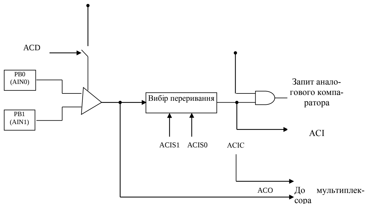
Рисунок 4.45 – Структурна схема аналогового компаратора
