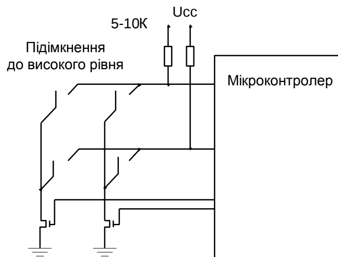
Рисунок 5.11 – Підключення до мікроконтролера матричної клавіатури
