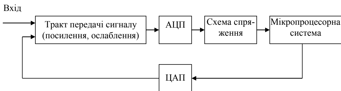
Рисунок 1.2 – До пояснення принципу корекції систематичної похибки
