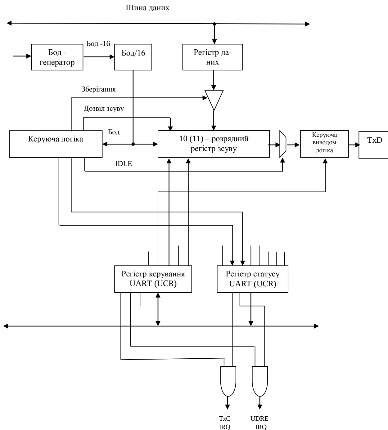
Рисунок 4.39 – Структурна схема вузла передавання даних UART
