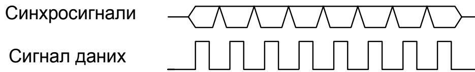
Рисунок 2.31 – Форма сигналів при синхронному передаванні даних
