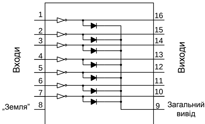
Рисунок 5.16 – Набір вихідних драйверів в мікросхемі ULN2003A
