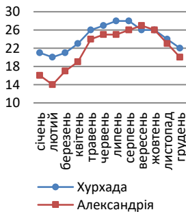
Рис. 2. 75. Пересічна температура води в районі Хурхада й Александрії
