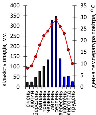
Рис. 2. 34. Кліматична діаграма Пусану
