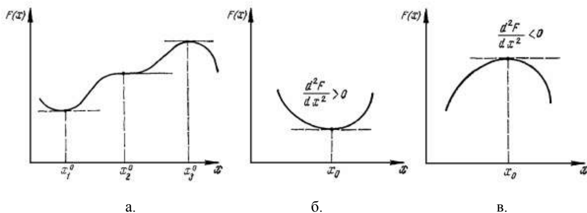
Рис. 5.3 Приклади екстремумів цільових функцій
