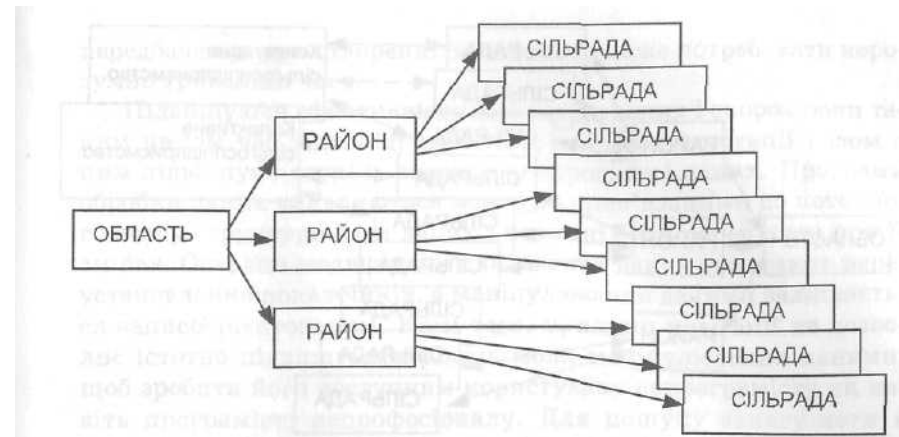
Рис. 3.2. Схема відношень між об'єктами в ієрархічній базі даних
