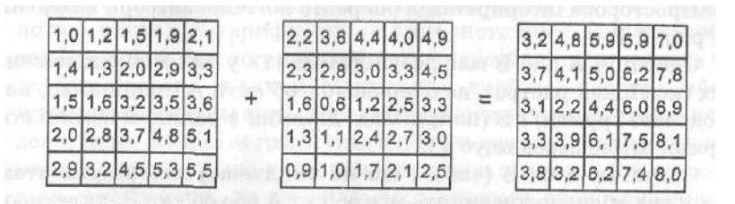
Рис. 7.2. Приклад локальної операції картографічної алгебри (операції додавання)
