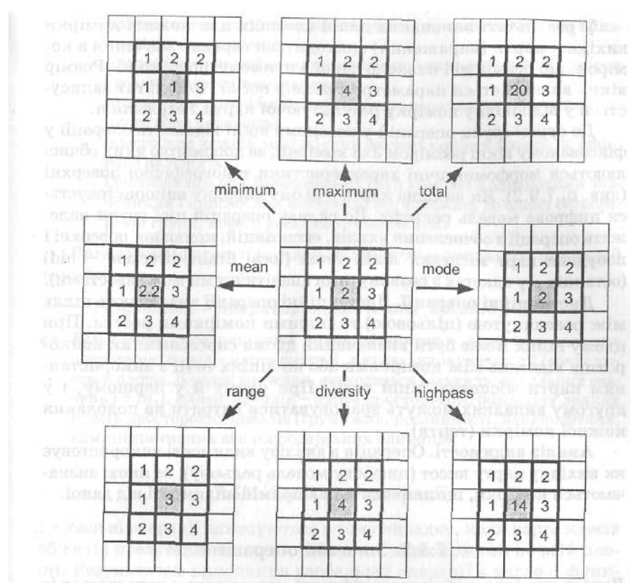
Рис. 7.4. Операції в ковзному вікні розміром 3x3 комірки
