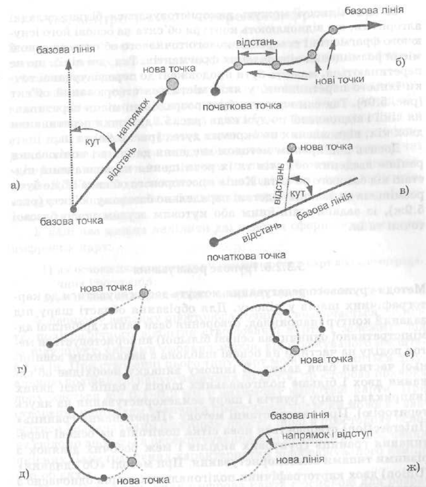
Рис. 5.9. Введення і редагування з використанням існуючих графічних об'єктів
