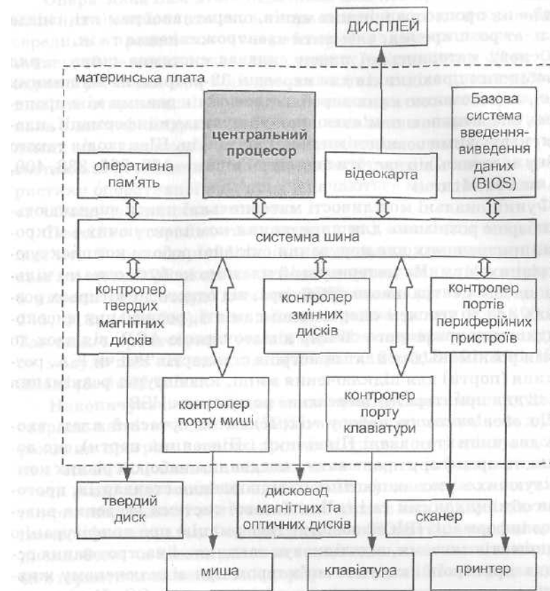
Рис. 2.3. Конфігурація й основні компоненти персонального комп'ютера
