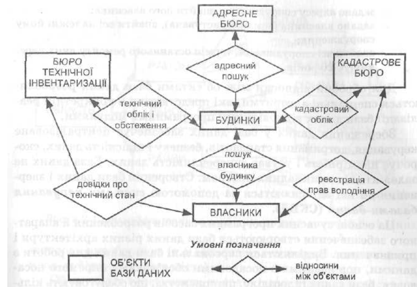
Рис. 3.1. Приклад концептуальної схеми муніципальної бази даних
