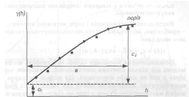
Рис. 8.4. Схематизована експериментальна варіограма перехідного типу з позначенням основних параметрів
