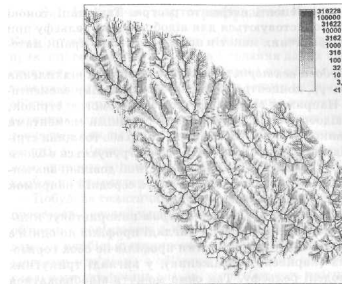
6.2. Візуалізація карти, що являє мережу елементарних водотоків, у логарифмічній шкалі
