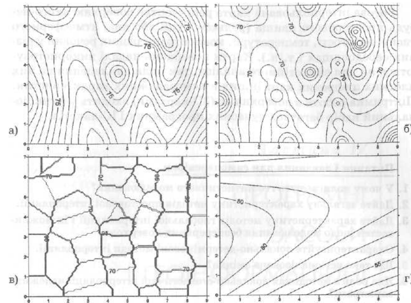
Рис. 8.6. Різні варіанти інтерполяції одного набору базових точок:
