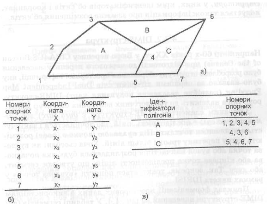
Рис 4 3 Подання картографічних даних з використанням точкової ' полігональної структури: а) формалізація вихідної карти; б) таблиця координат опорних точок; в) таблиця атрибутів полігонів
