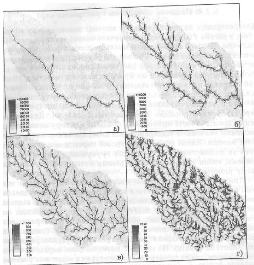
Рис. 6.1. Варіанти візуалізації карти, що являє мережу елементарних водотоків, при зміні верхнього значення відображуваного діапазону: а) до 100 000 комірок; б) до 10 000 комірок; в) до 1 000 комірок; г) до 100 комірок
