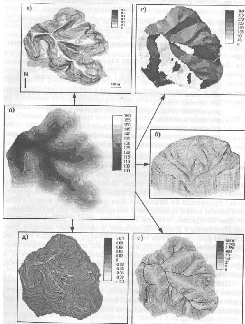
Рис. 7.9. Цифрова модель рельєфу балкового водозбору площею 0,59 км 2 у вигляді растра (а) і тривимірної блок-діаграми (б) та побудовані на її основі засобами ГІС-пакета PCRaster карти ухилів, безрозм. (в), експозицій, град, (г), поздовжньої кривизни схилів, безрозм. (д) і «вищерозміщених елементів», м 2 (е)
