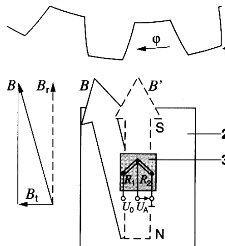
1 – зубчатий ротор (Fe); 2 – постійний магніт; 3 – датчик; B – керуюча напруженість поля з тангенційною B_t і радіальною B_r складовими ( B' – нульове положення, B_t = 0 ); R_1, R_2 – тонкоплівкові резистори (AMR); \varphi – кут повороту; U_0 – напруга живлення; U_A – вимірювана напруга
