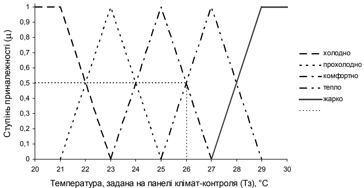
Рисунок 2.53 – Лінгвістична змінна T_z
