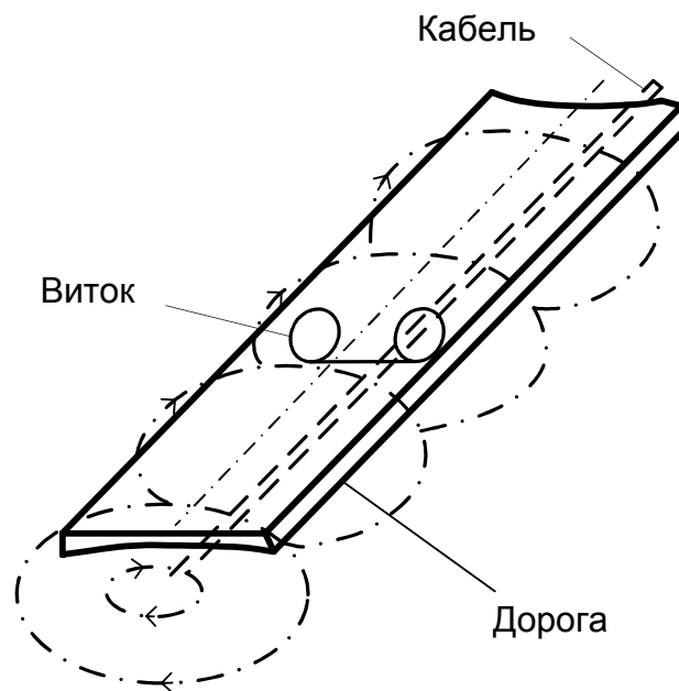
Рисунок 2.62 – Схема виявлення автомобіля на дорозі
