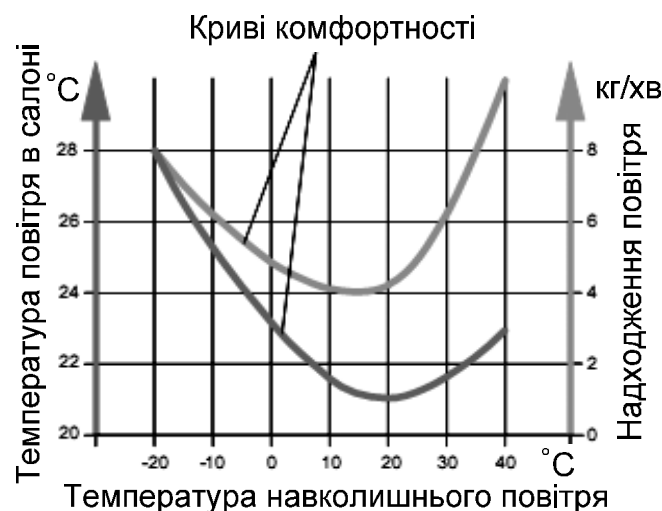
Рисунок 9.1 – Криві комфортності
