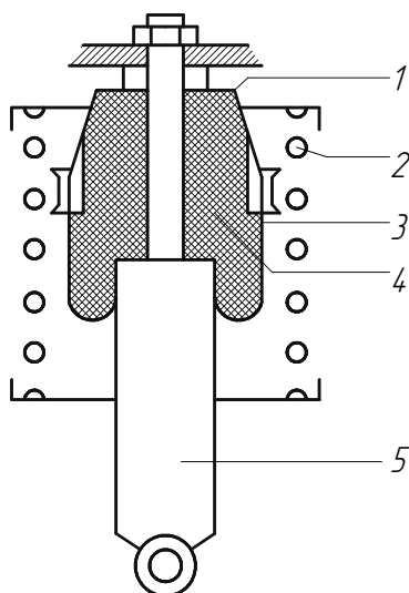
1 - повітряний штуцер; 2 - сталевая пружина; 3 - додаткова пневмопружина; 4 - газова камера; 5 - амортизатор
