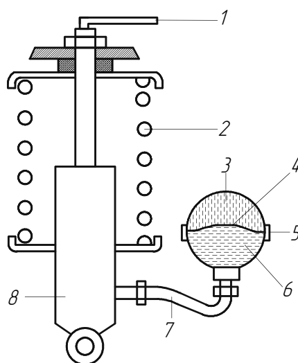
1 - подача рідини; 2 - сталевая пружина; 3 - акумулятор; 4 - газова камера; 5 - гумова діафрагма; 6 - рідина; 7 - шланг; 8 - амортизатор
