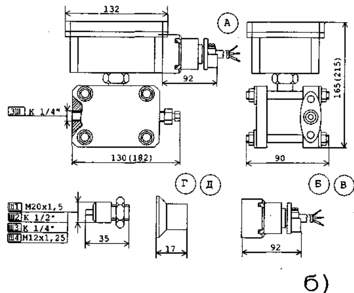
Рис. 2.31. Габаритно-монтажні розміри датчиків: а – КВАНТ ДІІ моделі 1318Т – 1339Т; б – КВАНТ ДІІ моделі 1405П – 1420П, КВАНТ ДВІ моделі 4405П – 4421П, КВАНТ ДАІ моделі 3411П – 3423П, КВАНТ ДІВІ моделі 6405П – 6423П. (У дужках вказані розміри для моделей 1405П – 1410П, 4405П – 4410П, 6405П – 6410П).
