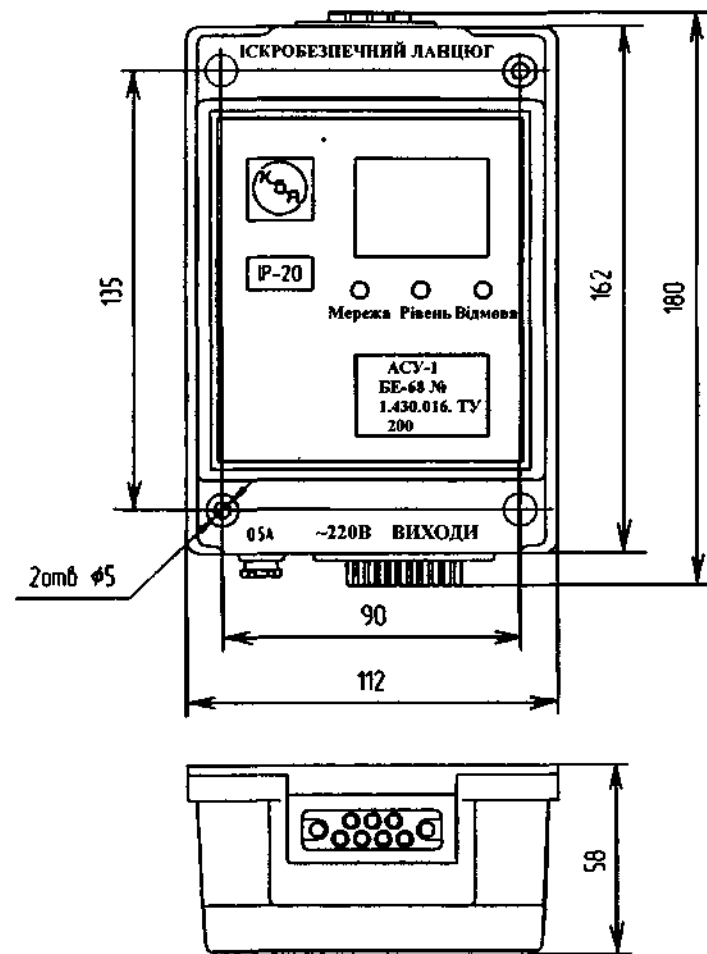
Рис. 3.23. Габаритно-установчі розміри електронному блоку БЗ-68
