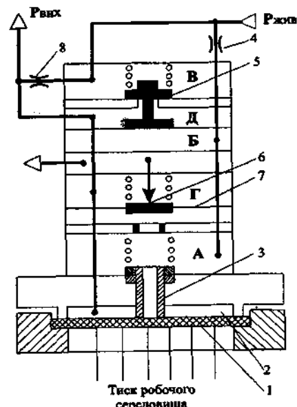
Рис. 2.7.Схема пневматична принципова повторювача тиску ПД-4М.
