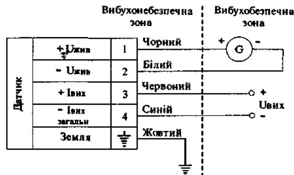
Рис. 2.30. Схема зовнішнього електричного з'єднання датчиків у звичайному та вибухозахищеному виконанні з чотирьох провідною лінією зв'язку і вихідними (U вих ) аналоговими сигналами напруги: G – блок живлення.
