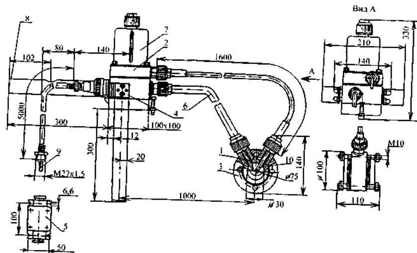
Рис. 6.62. Габаритно – монтажне креслення чутливого елемента магістрального виконання типу ДМ-5М (модифікації І – 4); 1 – електрод скляний; 2 – електрод допоміжний; 3 – корпус; 4 – коробка затискачів; 5 – коробка з'єднувальна; 6 – рукав; 7 – кожух; 8 – кронштейн; 9 – кабель; 10 – електролітичний ключ.
