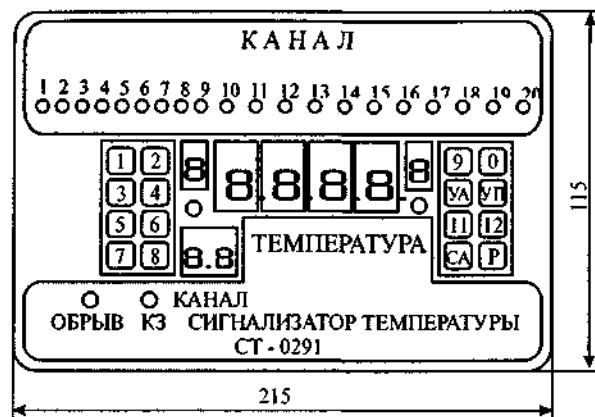
Рис. 5.10. Загальний вигляд сигналізатора СТ – 0291.
