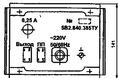
Рис. 6.38. Загальний вигляд передавального перетворювача кондуктометра КВА 4 (довжина 200 мм).
