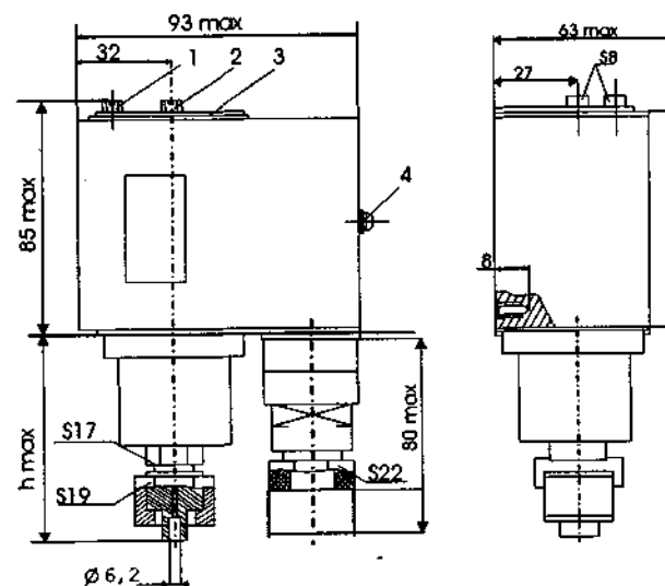
Рис. 2.15. Габаритні, з'єднувальні та монтажні розміри приладів типу ДЕМ: 1 – гвинт нагвинчування зони вороття; 2 – гвинт встановлення діапазону уставки; 3 – планка; 4 – гвинт заземлення; S – розмір під ключ.
