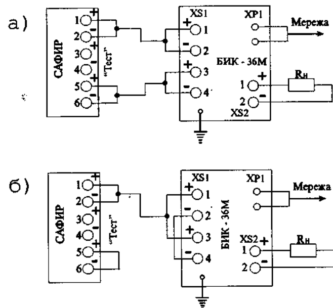
Рис.2.23. Схема зовнішніх з'єднань датчика САФІР і блоку витягання кореня БИК-36М: а) для датчика САФІР з вихідним сигналом 0 – 5 чи 4 – 20 мА і чотирьохпровідною лінією зв'язку; б) для датчика САФІР з вихідним сигналом 4 – 20 мА і двопровідною лінією зв'язку.
