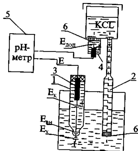
Рис. 6.60. Схема електродної вимірювальної системи.
