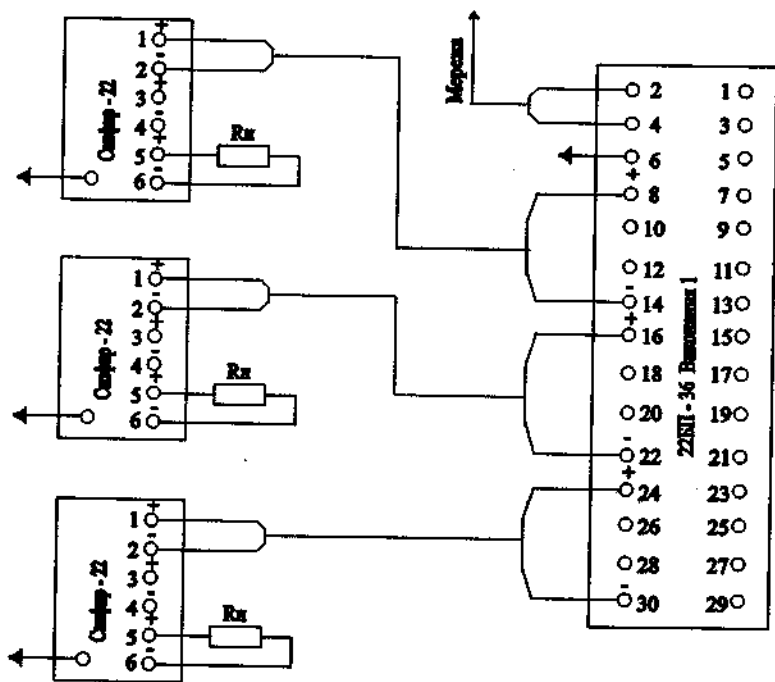
Рис.2.19. Схема зовнішніх з'єднань перетворювача “САПФІР-22” з межовими значеннями вихідного сигналу 0 – 5, 0 – 20 та 4 – 20 мА і блоку живлення 22БП-36 при підключенні навантаження R_n до перетворювача.
