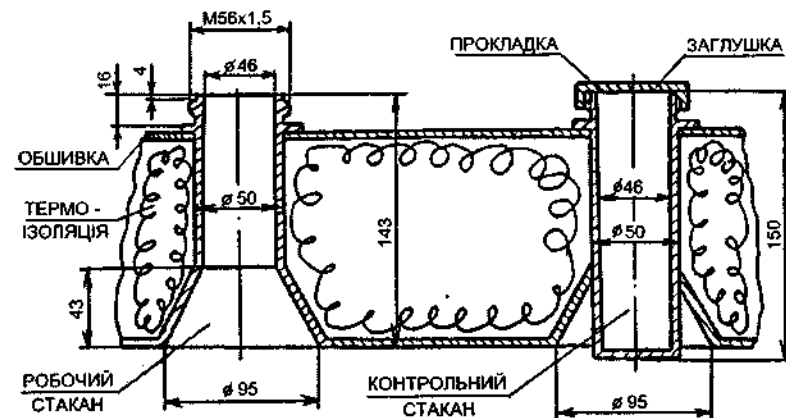
Рис.6.18. Приклад установлення робочого і контрольного стаканів сигналізаторів СТХ-7М-1, СТХ-7М-2.
