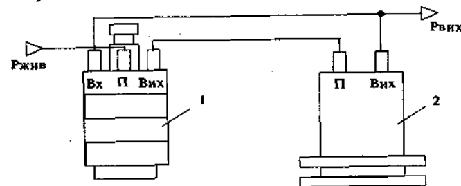
Рис. 2.8. Схема з'єднання повторювача ПД-4М(2) і стабілізатора тиску(1).
