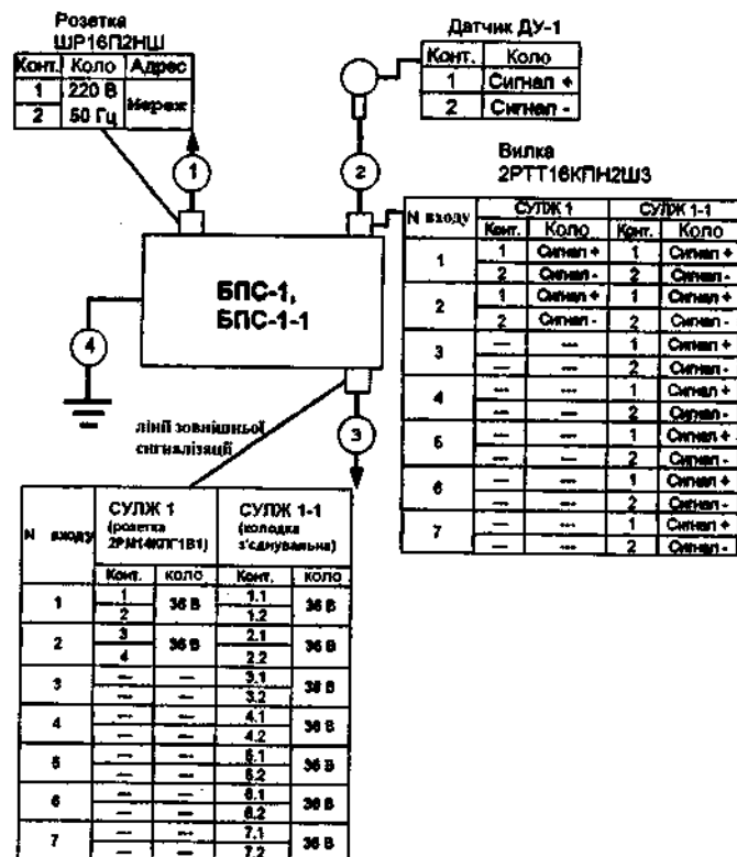
Рис. 3.15. Схема зовнішніх з'єднань сигналізаторів рівня типів СУЛЖ 1 і СУЛЖ 1-1: 1,3 – кабель КЛГУ 2х0,5 мм; 2 – кабель РК 75-4-12 або провід МГШВЭВ з перерізом не менше 0,2 мм 2 ; 4 – заземлення мідним проводом перерізом не менше 0,75 мм 2 .
