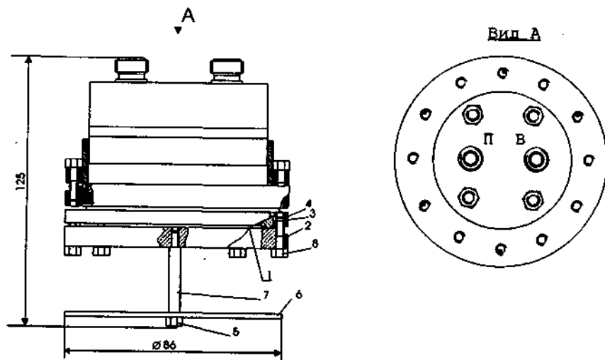
Рис. 2.9. Загальний вигляд конструкції повторювача ПД-4М зануреного монтажу: 1 – мембранний блок; 2,4 – фланець; 3 – прокладка; 5 – гайка; 6 – кришка; 7 – шток; 8 – болт.
