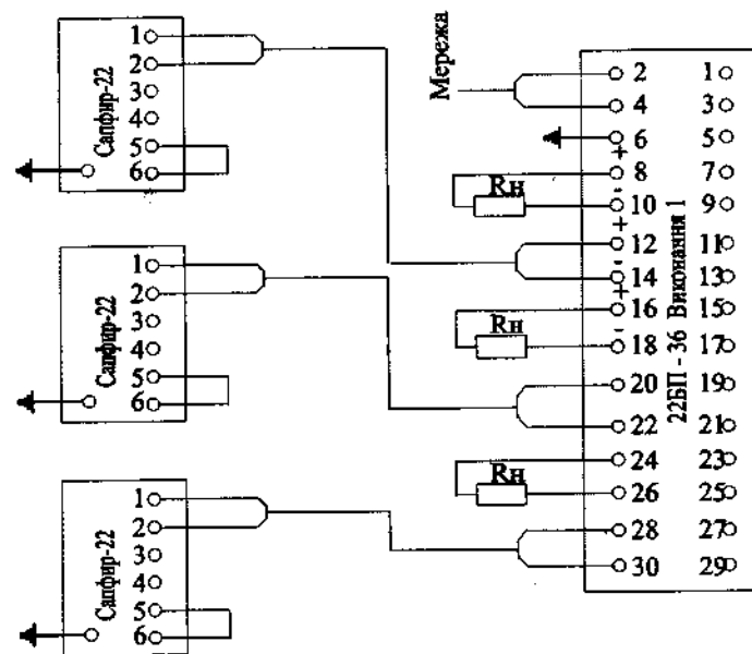
Рис.2.20. Схема зовнішніх з'єднань перетворювача “САПФІР-22” з межовими значеннями вихідного сигналу 0 – 5, 0 – 20 та 4 – 20 мА і блоку живлення 22БП-36 при підключенні навантаження R_n до блоку живлення.
