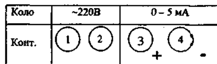
Рис.2.13 Маркування колодки зовнішніх з'єднань перетворювачів з компенсацією магнітних потоків.
