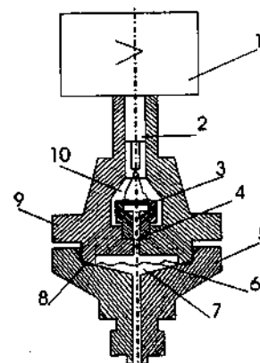
Рис. 2.16. Принципова схема перетворювача типу "Сапфир - 22ДГ".
