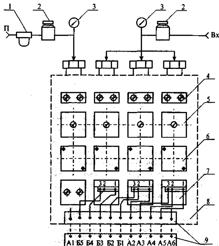
Рис. 7.6. Схема з'єднань перетворювача ППЭД-3М: 1 — фільтр повітря; 2 — стабілізатор тиску СДВ-1,6; 3 — манометр з діапазоном 0 - 0,16 МПа; 4 — постійні дроселі; 5 — пневмодатчики; 6 — компаратори; 7 — пневмоелектроперетворювачі ППЭР.4; 8 — комутаційна плата; 9 — штепсельний роз'єм.
