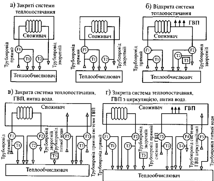
Рис.4.56. Можливі варіанти організації обліку у схемах тепло- і водопостачання: F1, T1 – датчик витрати і температури теплоносія у прямому трубопроводі системи опалення; F2, T2 – теж саме, але у зворотному трубопроводі системи опалення; F3, T3 – датчик витрати і температури гарячої води у прямому трубопроводі системи ГВП; F4, T4 – теж саме, але у зворотному трубопроводі системи ГВП; F5 – витрата питної води; T5 – температура питної води.
