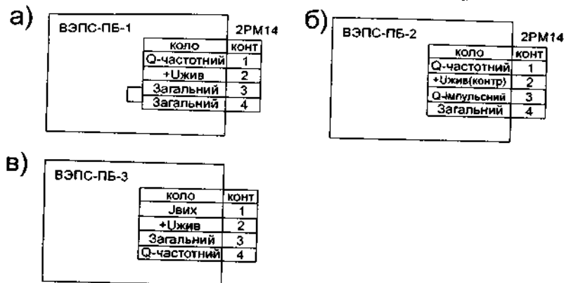
Рис. 4.55. Схема розпаювання роз'єму 2РМ14 для ВЭПС з частотним (а), імпульсним (б) і струмовим (в) виходом.
