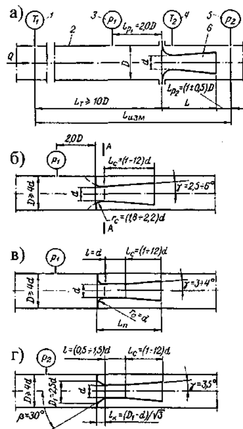
Рис.4.28. витратомір з соплом критичного стисання: а-принципова схема витратоміра; б-сопло з тороїдальною горловиною; в-сопло з циліндричною горловиною; г-сопло з прямолінійними утворючими.
