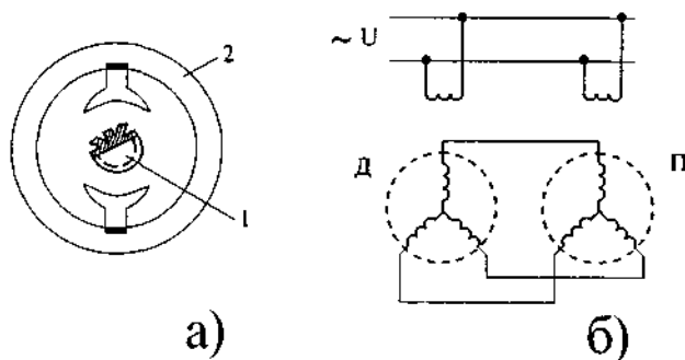
Рис. 3.3. Селесина передача: а - схема побудови; б - схема включення; 1 - ротор; 2 - статор.
