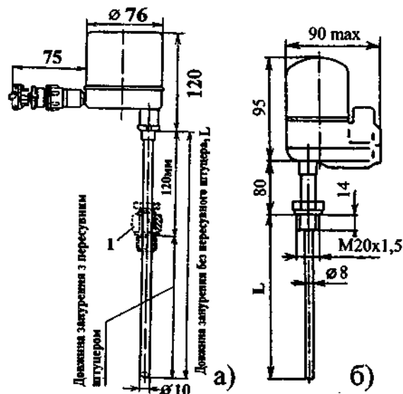
Рис.5.5. Габаритно-монтажні розміри термоперетворювачів ТХАУ-0288, 0388 (а) і ТХАУ-0289 (б); 1 – пересувний штупер або без нього.
