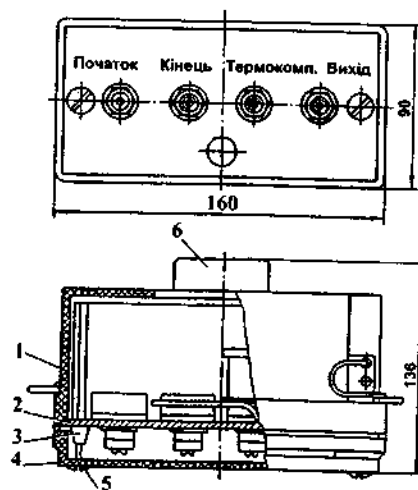
Рис. 6.53. Конструктивне оформлення вимірювального блоку концентратомірів КК-8(9).
