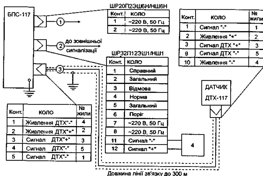
Рис. 6.20. Загальна схема електричних з'єднань сигналізатора СТХ-7М: 1 – кабель МКШ 2х0,75; 2 – кабель МКШ 10х0,75; 3 – кабель РПШЗ 6х1,5; 4 – вторинний прилад.
