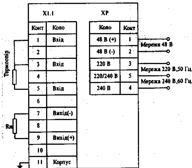
Рис. 7.2. Схема зовнішніх з'єднань перетворювача ПІ-79.
