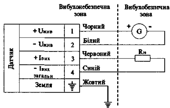
Рис. 2.29. Схема зовнішнього електричного з'єднання датчиків у вибухозахищеному виконанні з чотирьох провідною лінією зв'язку і вихідними (I вих ) аналоговими струмовими сигналами: G – блок живлення; R н – опір навантаження приймального пристрою.
