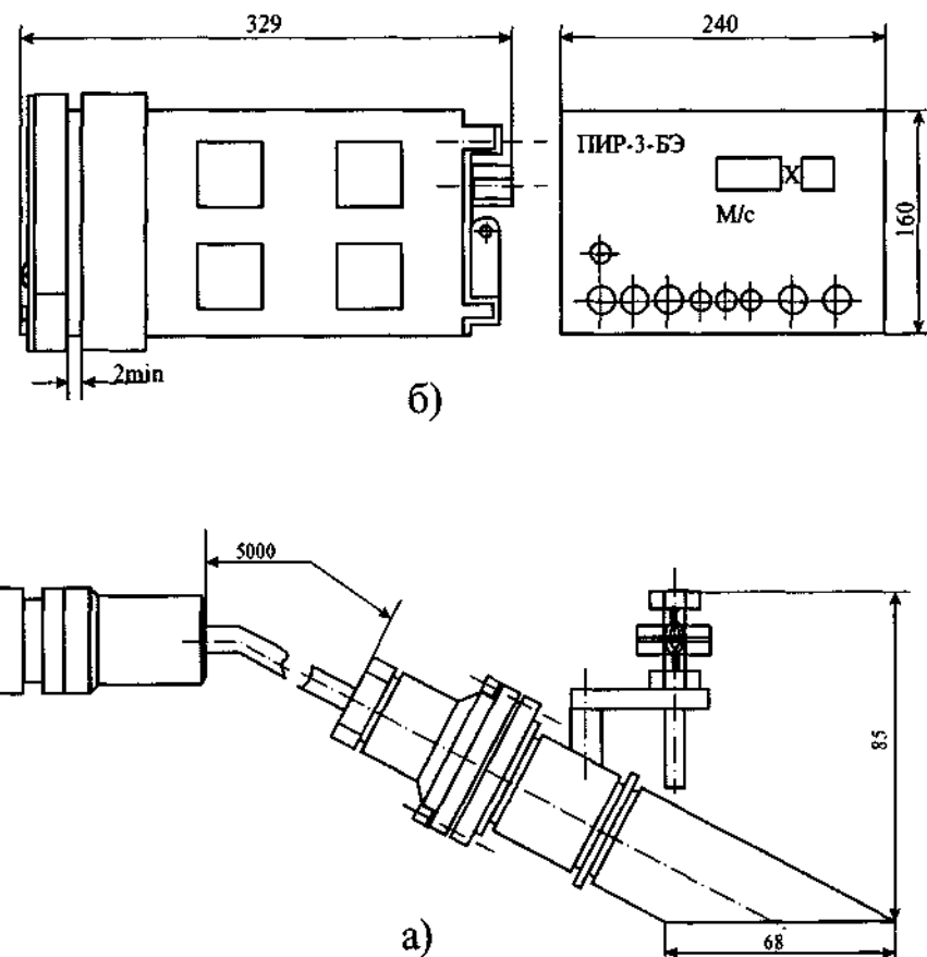
Рис. 4.34. Загальний вигляд та габаритні розміри первинного (а) і передавального (б) перетворювачів витратоміру типу ПИР.
