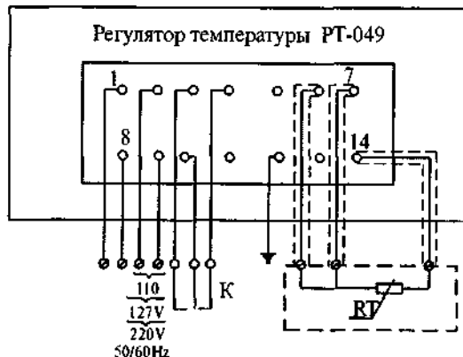
Рис. 5.14. Схема зовнішніх з'єднань регулятора РТ-049
