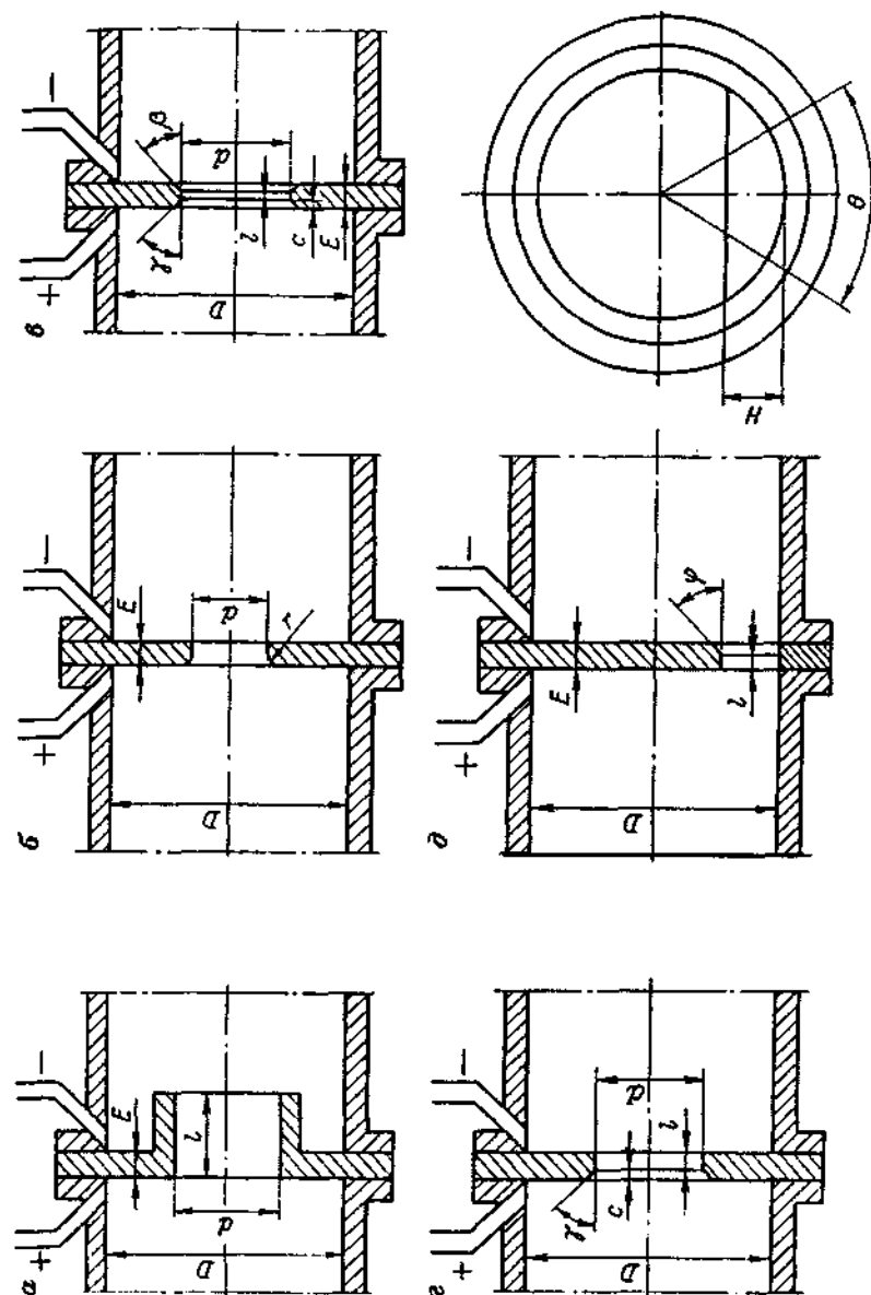
Рис. 4.26. Конструкції спеціальних звукувальних пристроїв.
