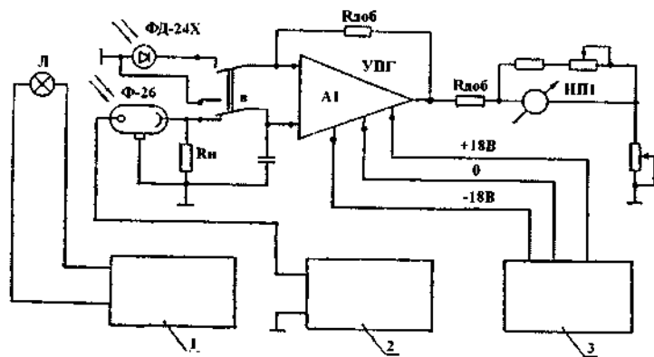
Рис.6.68. Блок-схема електрична фотокориметра.
