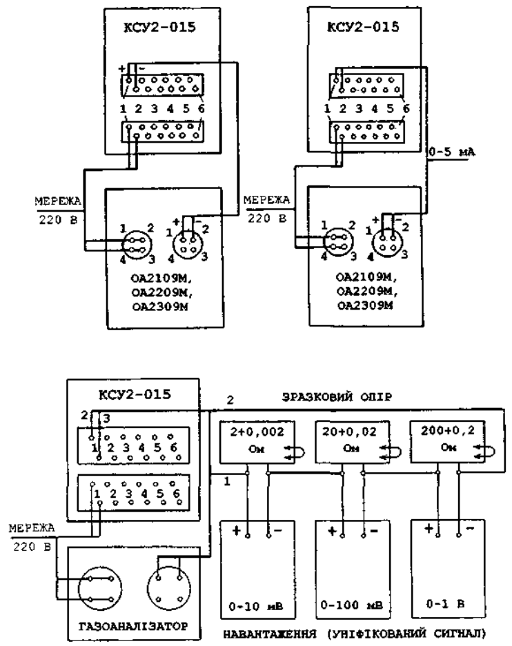
Рис.6.71. Схема електричних з'єднань газоаналізаторів ОА2109М, ОА2209М, ОА2309М: без уніфікованого вихідного сигналу для дублювання (а); з уніфікованим вихідним сигналом 0 + 5 мА (б); з уніфікованим вихідним сигналом 0 + 10, 0 + 100 і 0 + 1 В (в).
