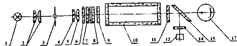
Рис.6.67. Оптична принципова схема фотоколориметра.
