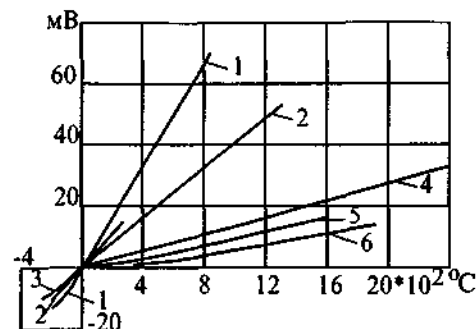
Рис.5.3. Номінальні статистичні характеристики ТЕП: 1 – ХК(Л); 2 – МК(М); 3 – ХА(К); 4 – ВР(А) – 1; 5 – ПП(С); 6 – ПР(В). (Примітка: у скобках наведено позначення ТЕП за міжнародним стандартом)
