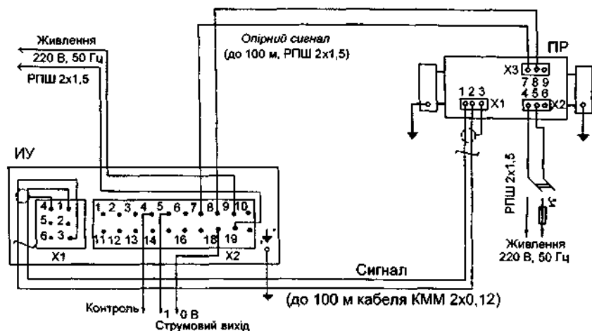
Рис.4.45. Електрична схема підключень перетворювача ІР-6М1.
