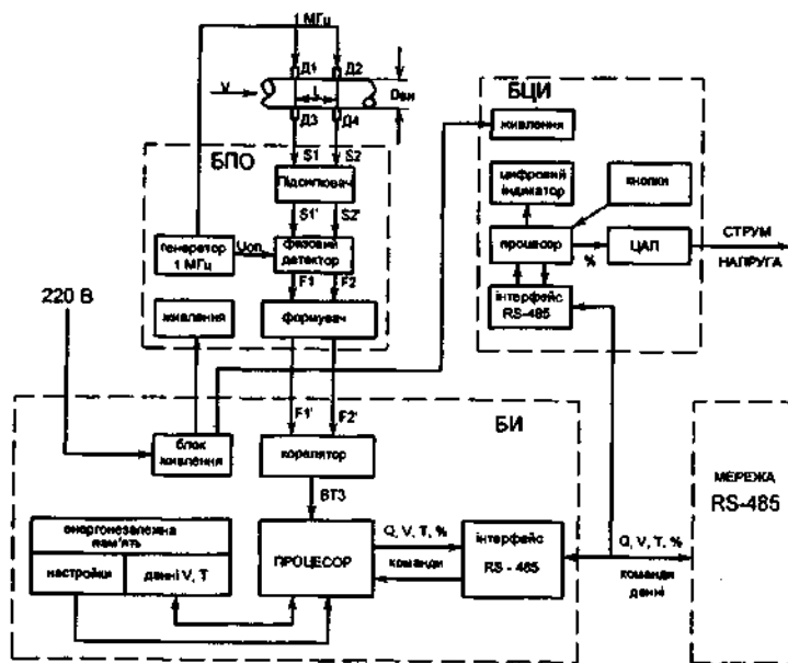
Рис.4.37. Функціональна схема витратомірного ультразвукового комплексу ІРКА: Q , V , T – параметри відповідно витрати, об'єм рідини, час наробки.
