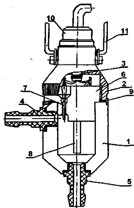
Рис. 6.40. Конструктивне оформлення чутливого елемента ЗЧ.
