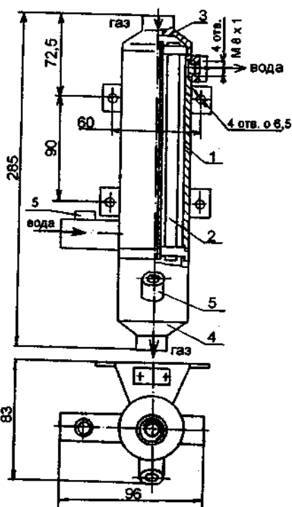
Рис. 6.34. Конструкція холодильника газу типу ХГ
