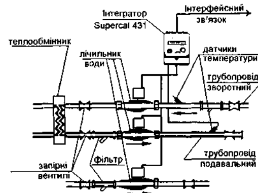
Рис. 4.59. Схема обладнання системи тепlopостачання комплектом засобів лічильника тепла SUPERCAL 431.
