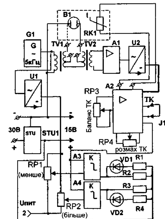
Рис. 6.42. Функціональна схема первинного перетворювача ПП.
