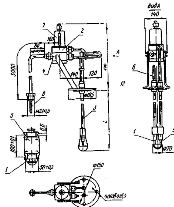
Рис.6.61. Габаритно-монтажне креслення чутливого елемента зануреного виконання типу ДПГ-4М (модифікації 1–12): 1 – електрод скляний; 2 – електрод допоміжний; 3 – корпус; 4 – коробка затискачів; 5 – коробка з'єднувальна; 6 – рукав; 7 – кожух; 8 – кабель; 9 – електролітичний ключ; L – довжина занурення.
