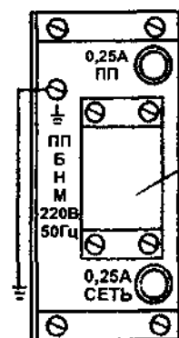
Плата ЗПС - 20 - 10
