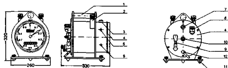
Рис. 4.5. Загальний вигляд та габаритні розміри лічильника серії TG (моделі 5–7): 1–ручка; 2–додатковий вимірювальний комплект (газовий термометр, термометр для рідини, манометр); 3–візуальний рівнемір положення установки; 4–кришка; 5–вихід імпульсного генератора; 6–кнопка вмикання; 7, 10 – штуцери виходу і входу газового потоку, що вимірюється; 8–штуцер для заповнення рідиною; 9–індикатор рівня рідини у барабані; 12–кран для зливу води; 11–опори регулювання положення лічильника.
