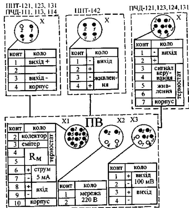
Рис. 5.20. Електрична схема зовнішніх з'єднань перетворювачів комплексу АПІР-С.
