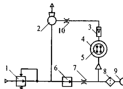
Рис.6.11. Принципова пневматична схема газового тракту датчика ДТХ-128: 1 – редуктор РДВ-5М; 2 – ежектор; 3 – ротаметр; 4 – ковпачок; 5 – блок чутливих елементів; 6 – пневмотумблер; 7, 10 – пневмодросель; 8 – фільтр; 9 – штуцер.
