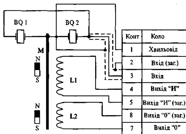
Рис.3.17. Принципова схема електромеханічного перетворювача (датчика) рівнеміра РУ-ПТ1
