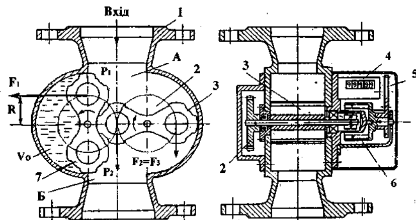
Рис. 4.6. Принципова схема ротаційного лічильника газу
