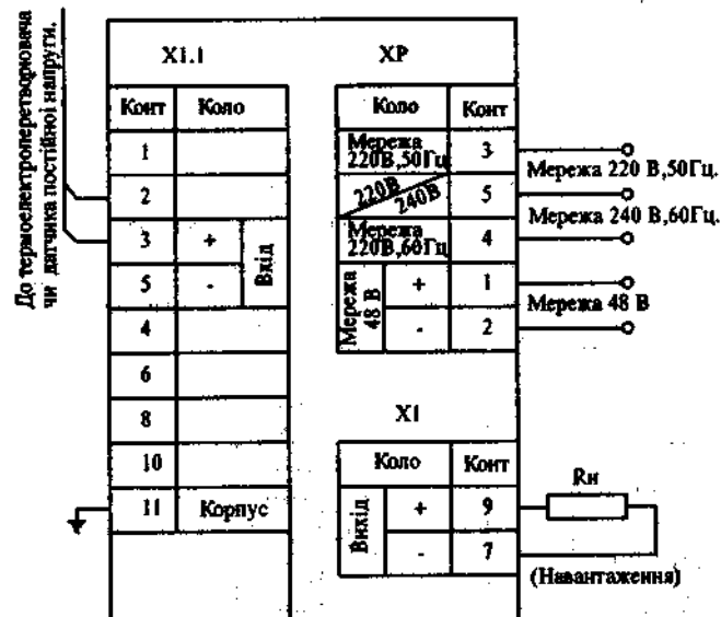
Рис. 7.1. Схема зовнішніх з'єднань перетворювача ПІ-78: XI.1 – колодка клем; ХР – вихід.
