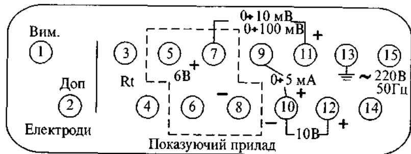
Рис.6.65. Маркування клем на кришці коробки розподільної.
