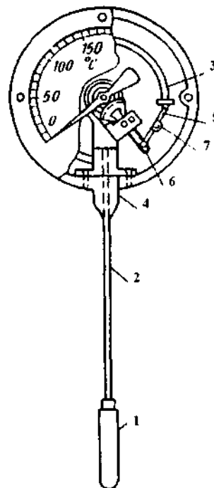
Рис.5.1. Принципова схема манометричного термометра з трубчастою пружиною: 1 – термобалон; 2 – капілярна трубка; 3 – манометрична трубка; 4 – утримувач; 5 – поводок; 6 – зубчастий сектор; 7 – біметалевий компенсатор
