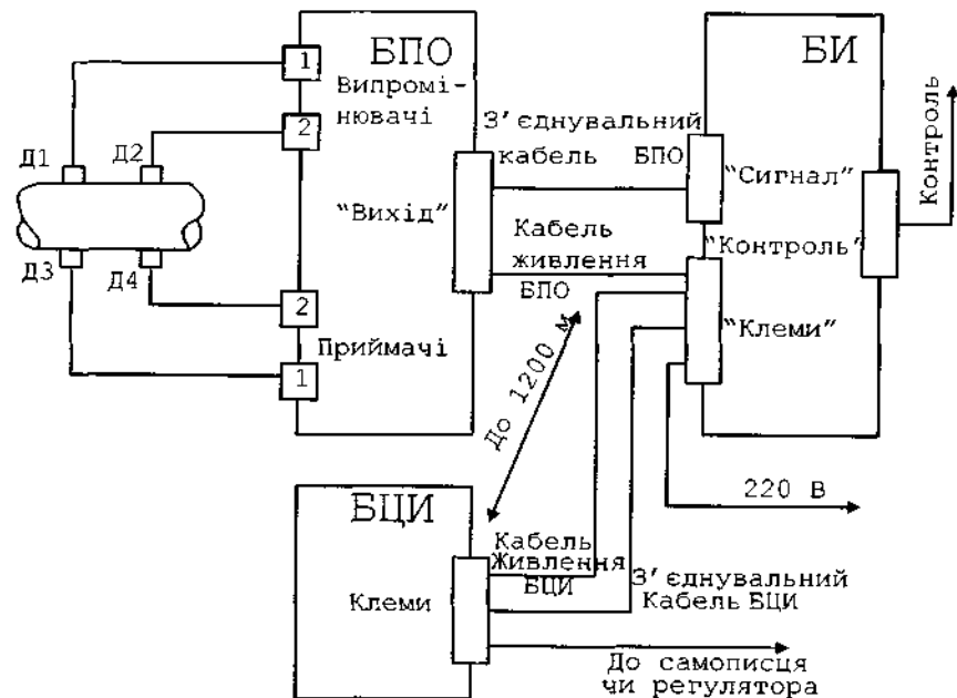
Рис.4.38. Схема зовнішніх з'єднань блоків комплексу ІРКА.
