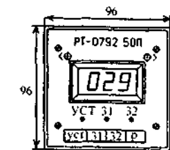
Рис.5.15. Загальний вигляд регулятора РТ-0792
