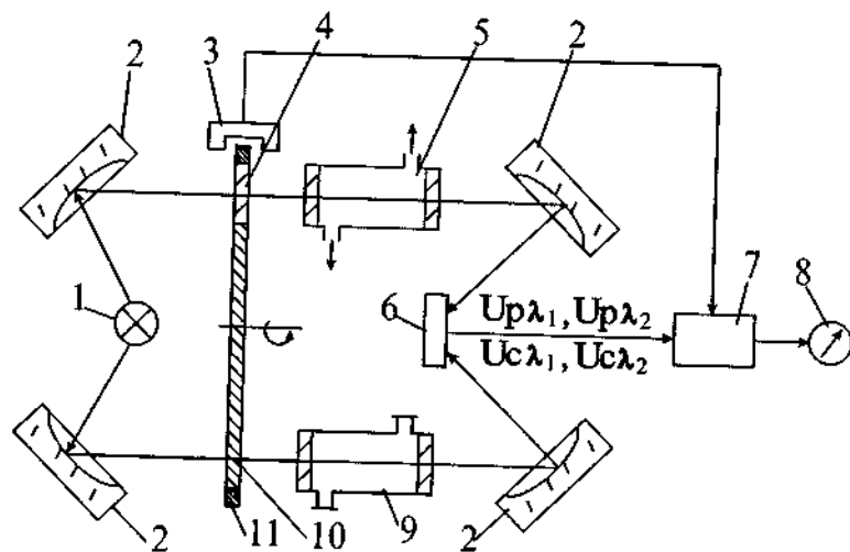
Рис. 6.66. Функціональна схема комбінованого (подвійна одноканальна двопроменева) інфрачервоного аналізатора рідини.
