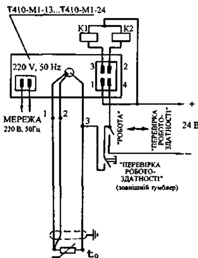
Рис.5.17. Схема зовнішніх з'єднань приладу T410-M1.
