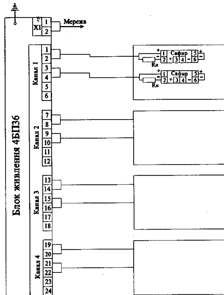
Рис. 2.25. Схема зовнішніх з'єднань датчика САΦИР з вихідним сигналом 4 – 20 мА і блоку живлення 4BP36 по двох провідній лінії зв'язку (на один канал допускається підключати не більше двох датчиків з вихідним сигналом 4 – 20 мА).
