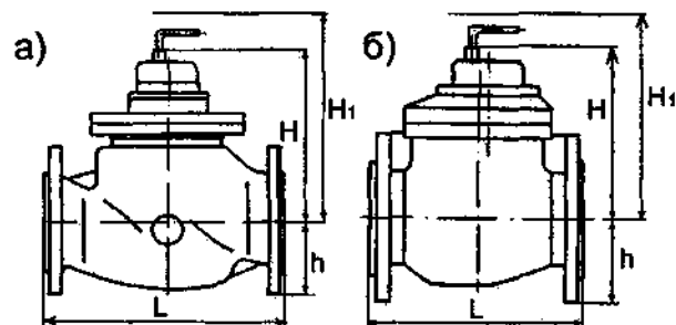
Рис.4.16. Загальний вигляд лічильників типу MP(а) і MW (б)
