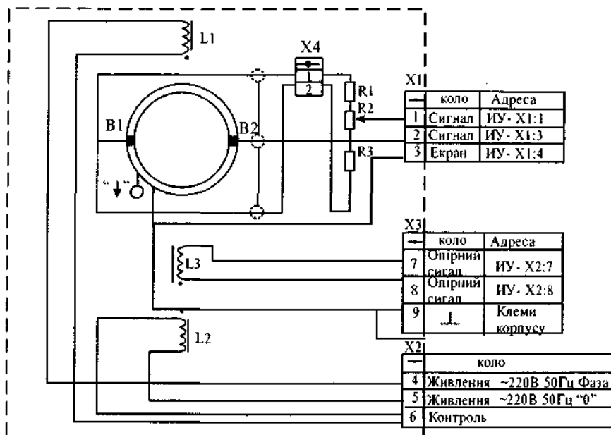
Рис.4.42. Схема електрична принципова первинного перетворювача ПР.
