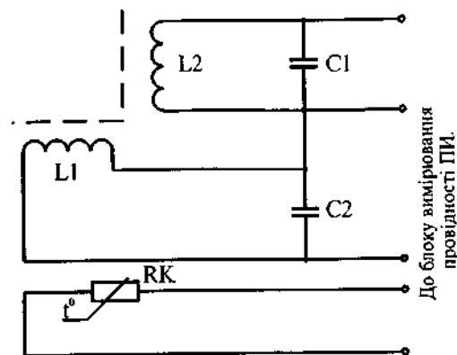
Рис. 6.56. Принципова електрична схема чутливого елемента перетворювача ПП.
