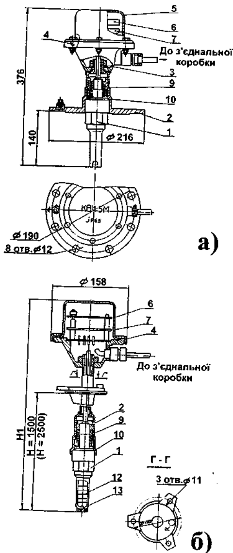
Рис. 6.55. Конструкція перетворювача вимірювального ПП проточного (а) і зануреного (б) виконань: Н1, дорівнює 1720 і 2720 мм відповідно для глибини занурення 1500 і 2500 мм.
