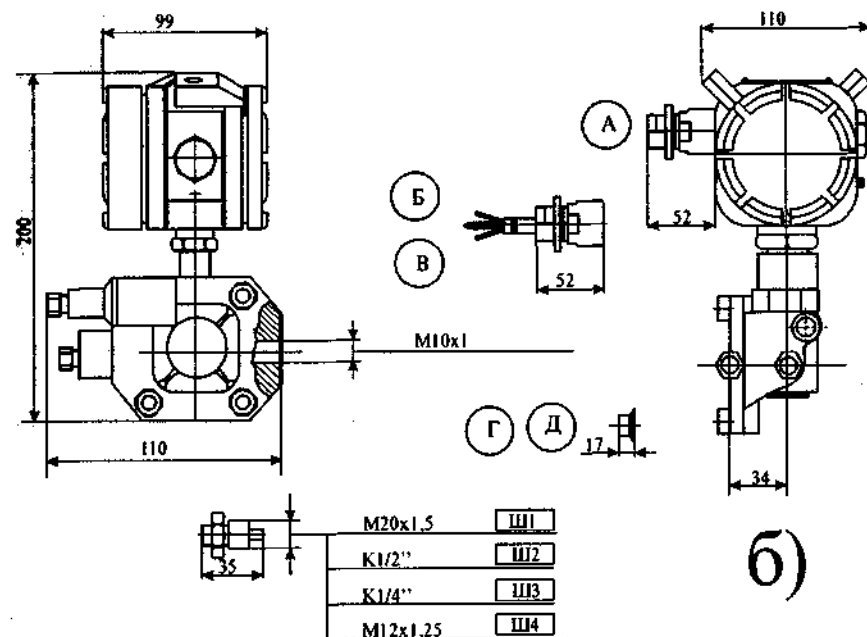
Рис. 2.32. Габаритно – монтажні розміри датчиків: а – КВАНТ ДГІ моделі 5511П – 5523П; б – КВАНТ ДДІ моделі 2509М – 2526М.
