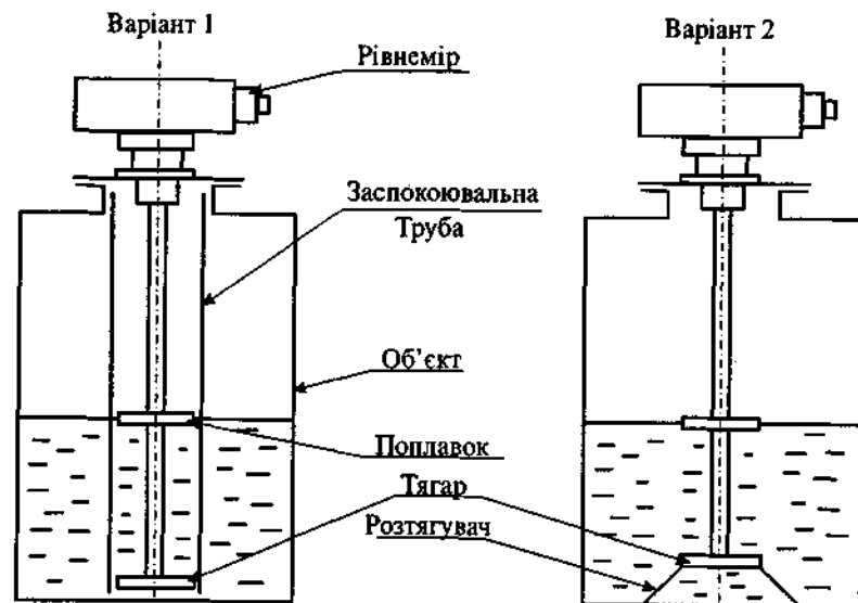
Рис. 3.20. Варіанти монтажу первинного перетворювача рівнеміра РУ-ПТ1.
