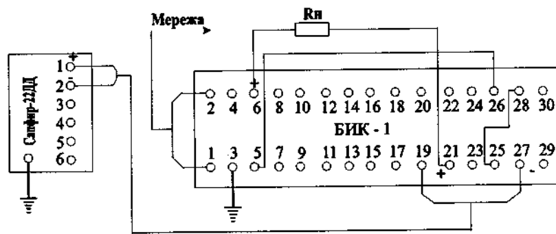
Рис. 2.21. Схема зовнішніх з'єднань перетворювача “САПФІР-22ДД” з вихідним сигналом 4 + 20 мА і блоку витягання кореня БИК-1 з вихідним сигналом 0 – 5 мА до навантаження R_n
