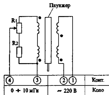
Рис.2.10. Схема електрична принципова дифманометра: 1, 2 – клеми живлення первинної обмотки змінним струмом 0.125 А для моделі ДМ-3583М і 0.32 А для моделі ДМ-3583ФМ частотою 50Гц від приладу або регулятора; 3, 4 – клеми вторинної обмотки для з'єднання з приладом або регулятором; R 1 – опір для настроювання границь вимірювання вхідних сигналів; R 2 – опір постійний.
