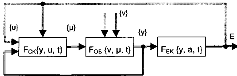
Рис. 1.1. Узагальнююча математична структура АСКТП : {y} - вихідні параметри об'єкта керування; {μ} - впливи, що регулюють чи керують; {v} - збурювальні впливи; {u} - параметри стану об'єкта, що задаються або визначаються; {a} - параметри і характеристики системи керування; FСК, FОБ, FЕК - оператори алгоритму відповідно системи керування, об'єкта та цільової функції; E - критерій економічної ефективності; t - час.
