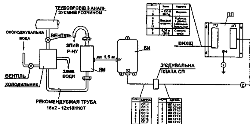
Рис.6.49. Монтажна схема солеміру типу СКВ-3: 1-мідний провід діаметром понад 2 мм; 2-кабель з'єднувальний КУПВ-7х0,36 або проводи типу МГШВ, МГШП діаметром до 7 мм.
