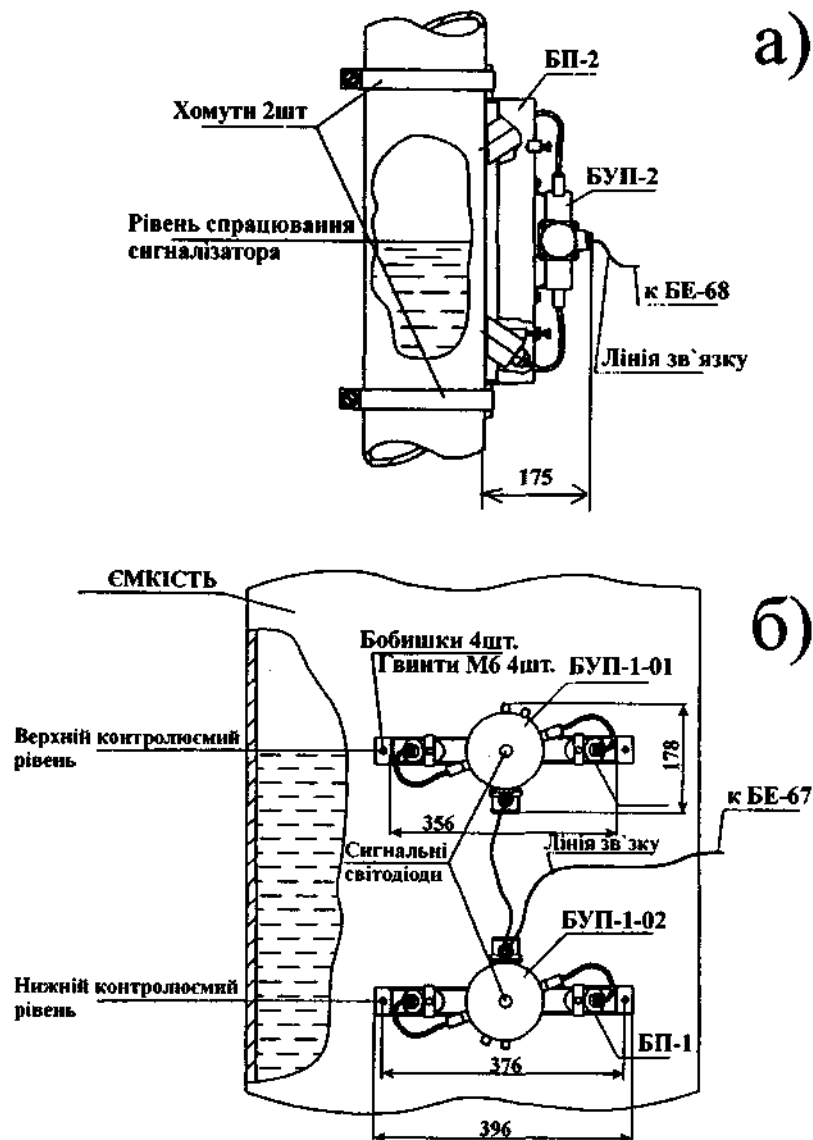
Рис.3.21 Монтаж блоків БП з блоком БУП: а – на контролюємій ділянці труби; б – на контролюємій ємкості.
