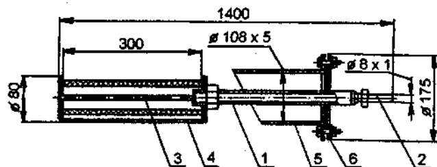
Рис. 6.33. Конструкція газозабірного пристрою ГЗУ – 2.
