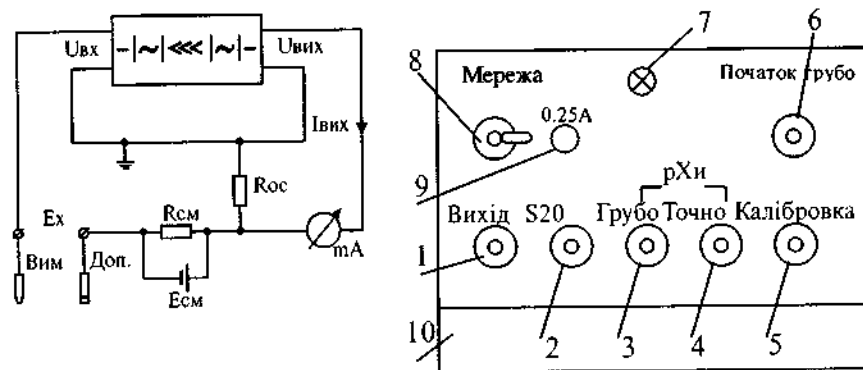
Рис. 6.64. Розміщення органів на- строювання на передній панелі перетво- рювача П-201.
