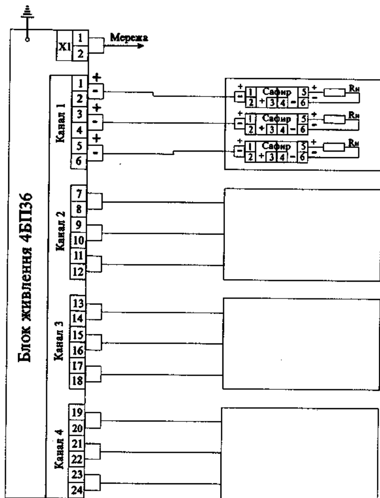
Рис. 2.24. Схема зовнішніх з'єднань датчика САΦИР з вихідними сигналами 0 – 5 та 4 – 20 мА і блоку живлення 4BP36 по чотирьох провідній лінії зв'язку (на один канал дозволяється підключати три датчики з вихідним сигналом 0 – 5 мА або два датчики з вихідним сигналом 4 – 20 мА).
