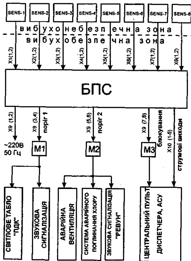
Рис. 6.28. Блок-схема підключення сигналізатора ДОЗОР-Х-Т на технологічному об'єкті.
