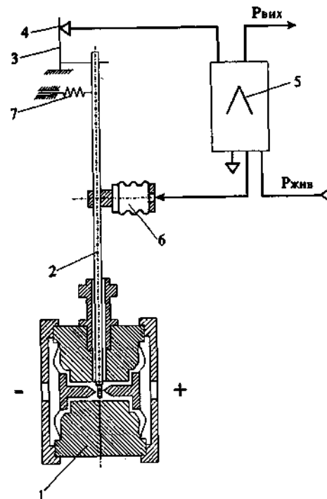
Рис.2.6 Принципова схема перетворювача різниці тисків 13ДД11: 1–двомембранний чутливий елемент; 2–важіль; 3–заслінка; 4–сопло; 5–пневмореле; 6–сильфон зворотного зв'язку; 7–пружина коректора нуля.
