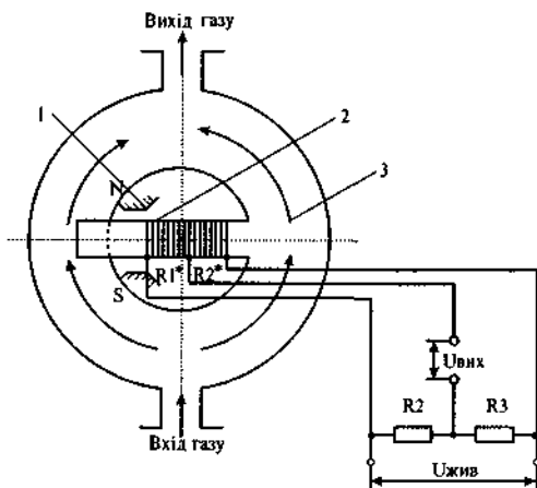
Рис. 6.1. Принципова схема перетворювача ПП-16: R_1^*, R_2^* – опори секцій чутливого елементу, R_2, R_3 – опори плеч моста; 1 – постійний магніт; 2 – чутливий елемент; 3 – кільцевий канал.
