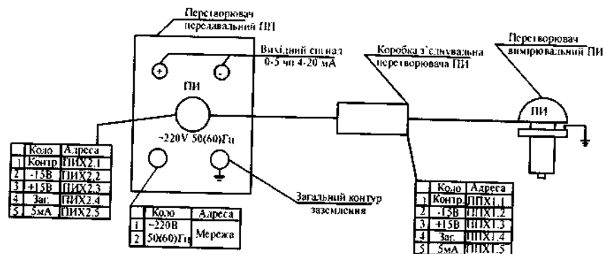
Рис.6.58. Схема з'єднань аналізатора типу KBЧ-5М.
