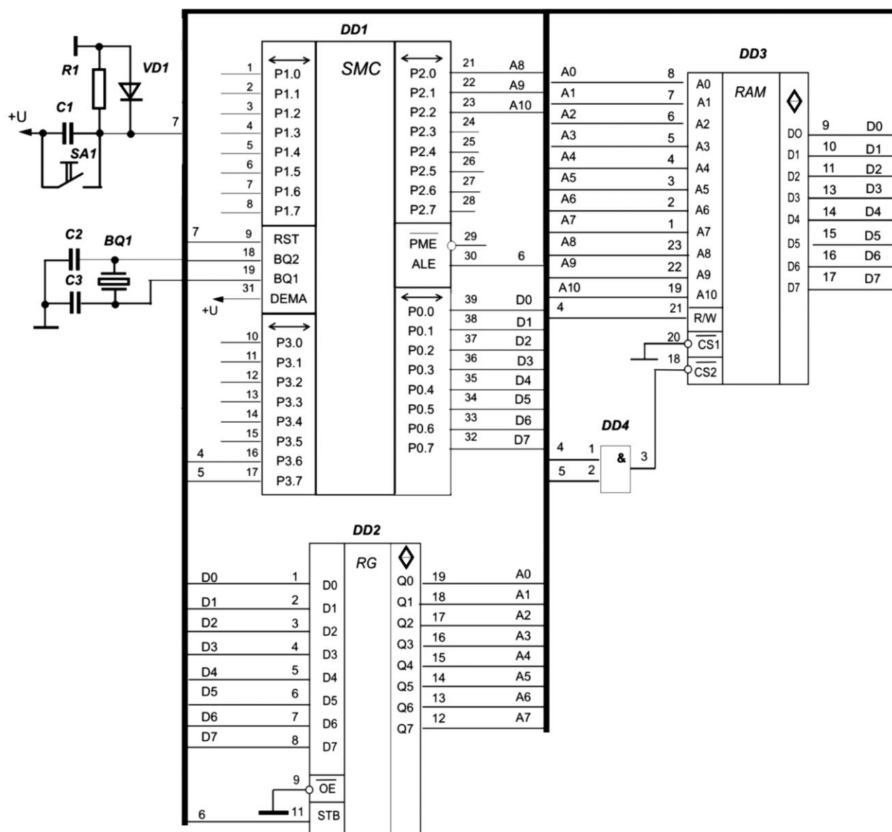
Рисунок 6. Розширення пам'яті даних для мікроЕОМ 87C51
