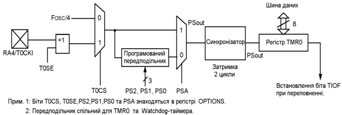
Рисунок 62. Структурна схема таймера-лічильника TMR0
