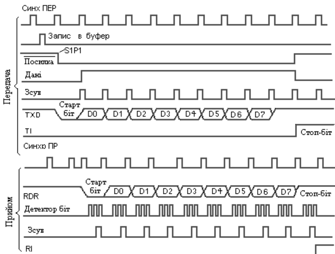
Рисунок 15. Часова діаграма роботи УАПП у режимі 1
