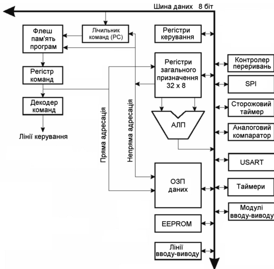
Рисунок 98. Архітектура ATmega32
