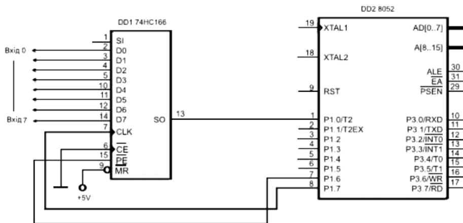
Рисунок 24. Перетворення паралельних вхідних даних у послідовний код
