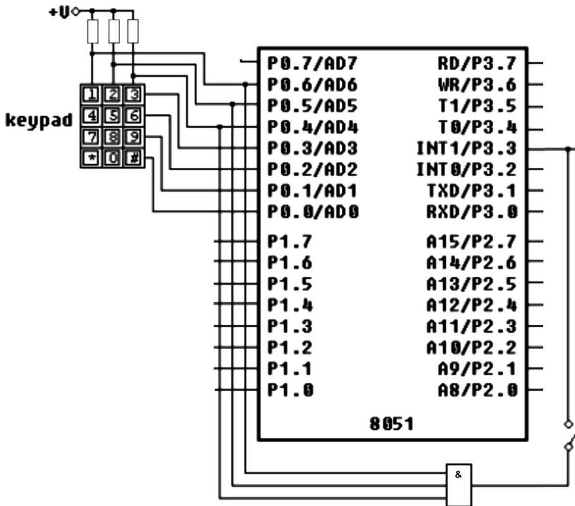
Рисунок 47. Підключення клавіатури
