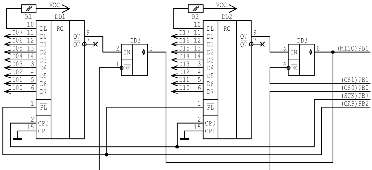
Рисунок 163. Розширення портів вводу за допомогою інтерфейсу SPI. Варіант із вибором регістра окремим сигналом
