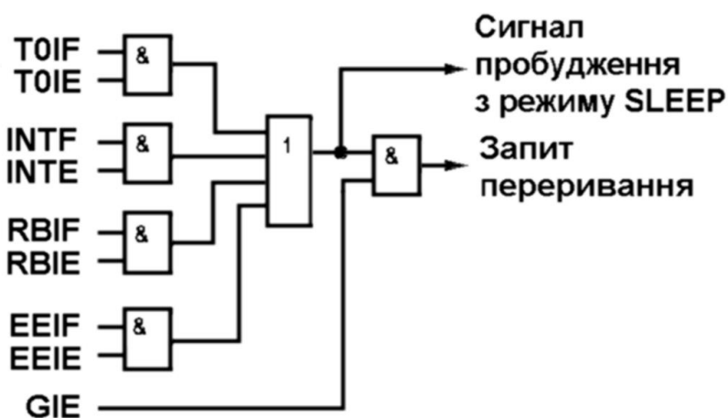
Рисунок 65. Логіка переривань мікроконтролера
