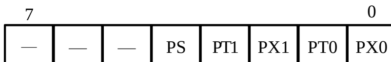
Рисунок 19. Формат регістра пріоритетів переривань IP
