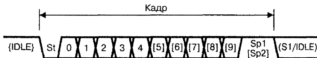
Рисунок 168. Формати кадру
