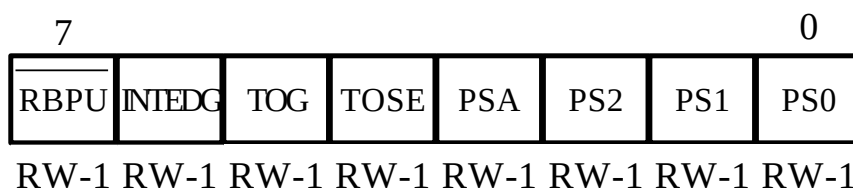
Рисунок 57. Формат регістра конфігурації OPTION
