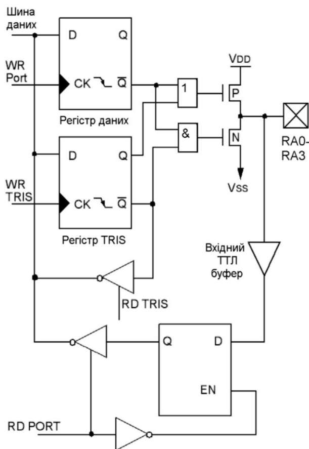
Рисунок 58. Схема ліній RA<3:0> порту A
