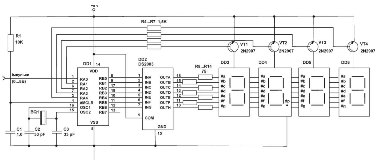
Рисунок 95. Схема лічильника на основі PIC-контролера
