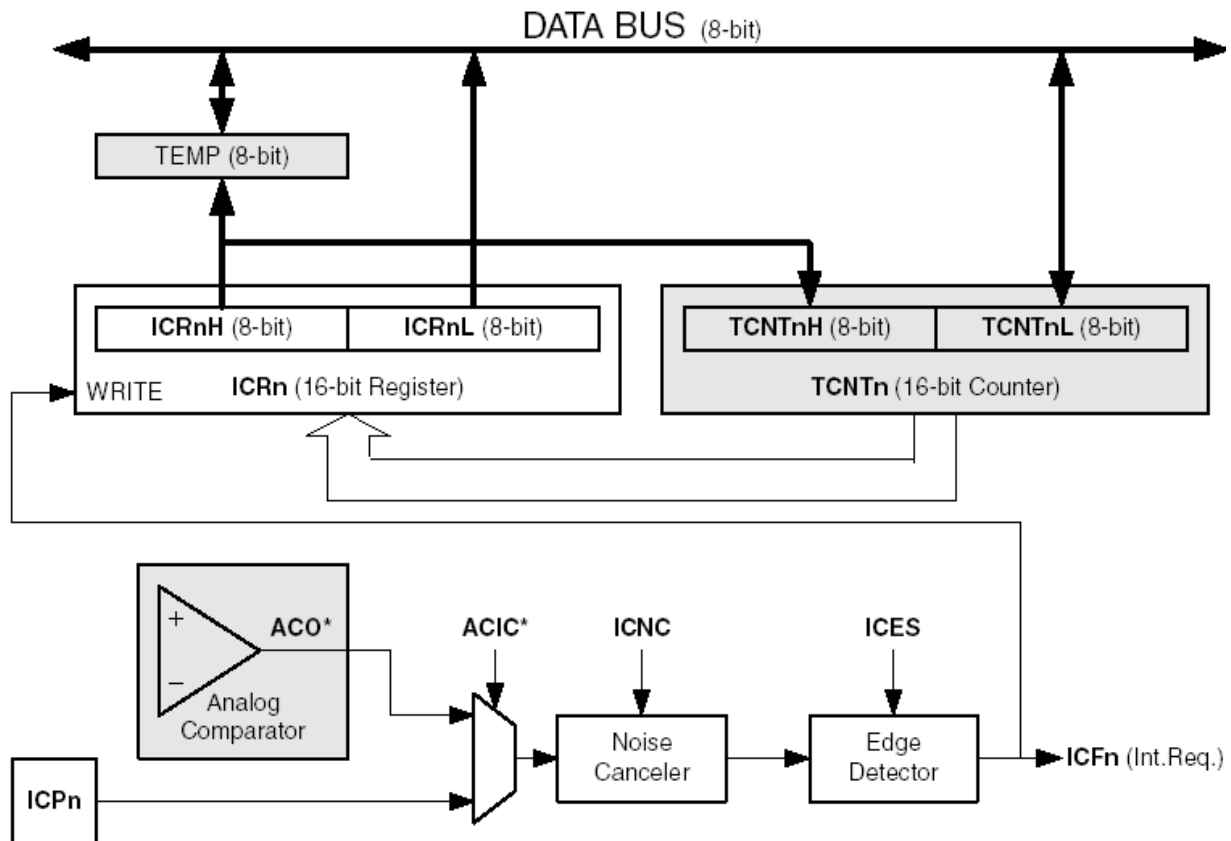
Рисунок 139. Структурна схема блока захоплення
