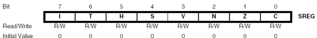
Рисунок 100. Формат регістра SREG
