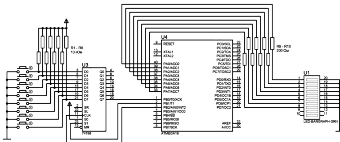
Рисунок 198. Принципова схема підключення клавіатури з використанням зсувних регістрів
