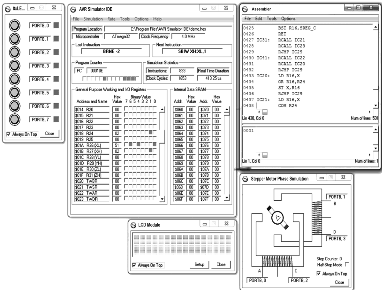
Рисунок 208. Вигляд симулятора з завантаженою програмою, вікнами: LCD Module, Stepper Motor Phase Simulation та дисплеєм 8xLED Board
