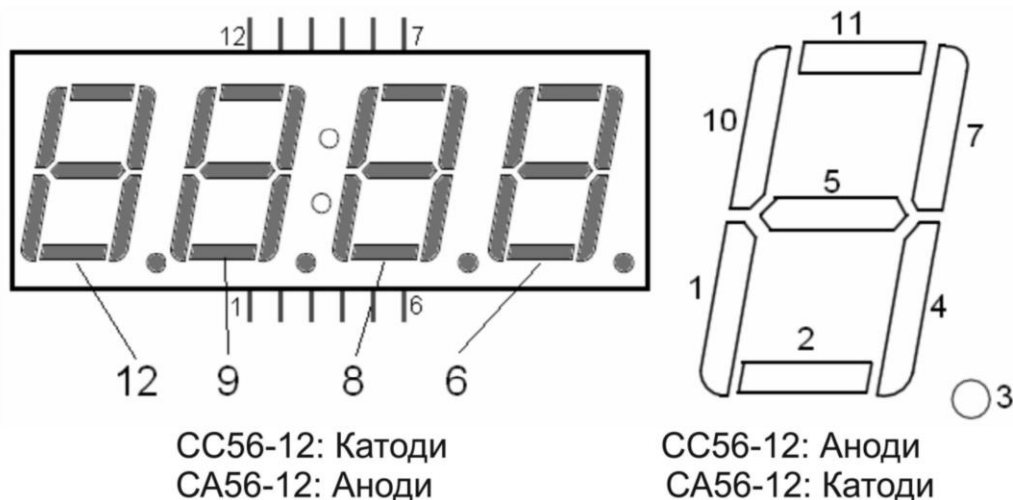
Рисунок 203. Нумерація виводів індикаторів CA56-12/CC56-12
