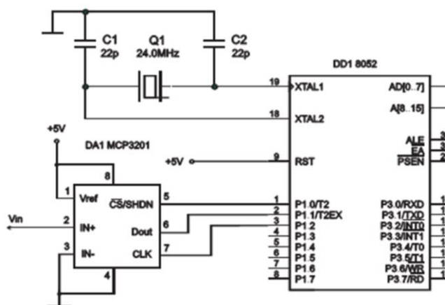
Рисунок 25. Схема опрацювання аналогового сигналу
