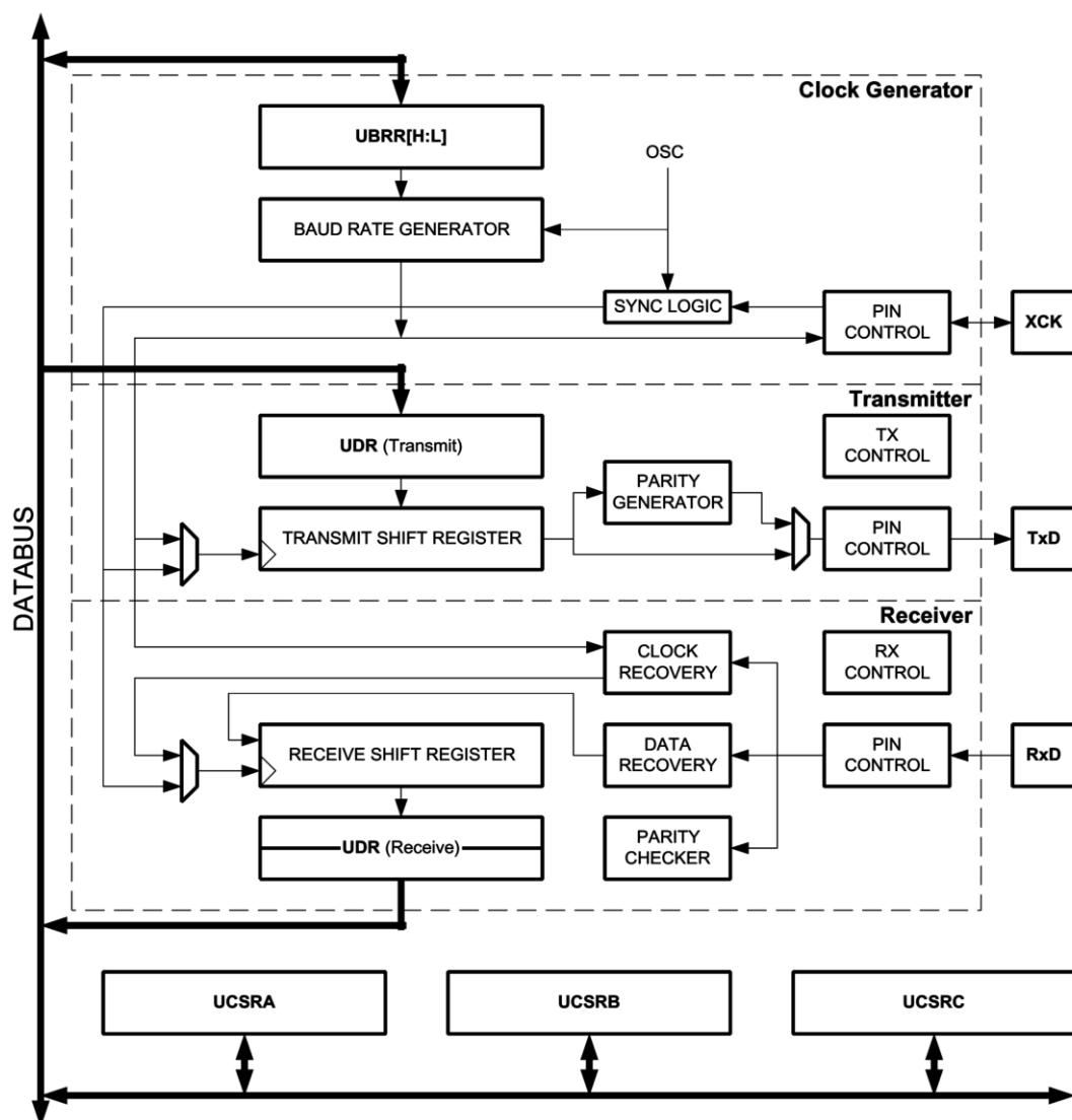
Рисунок 167. Блок-схема USART
