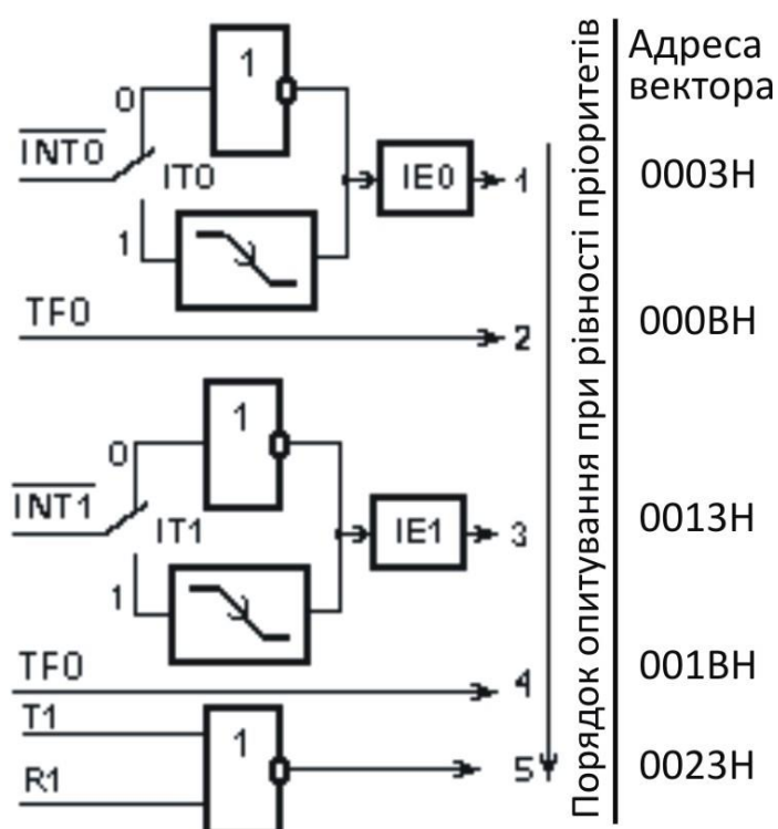
Рисунок 17. Схема переривань MCS-51
