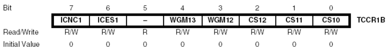
Рисунок 142. Формат регістра TCCR1B
