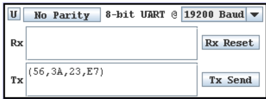
Рисунок 45. Передача даних
