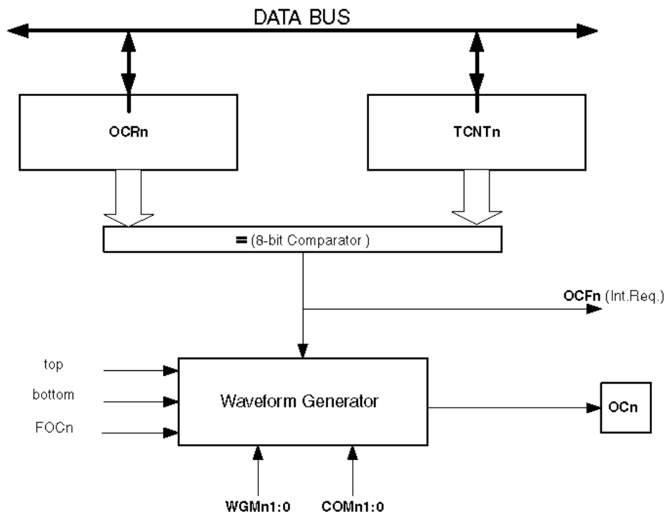
Рисунок 124. Схема порівняння 8-бітного таймера-лічильника n ( n = 0 або 2 )
