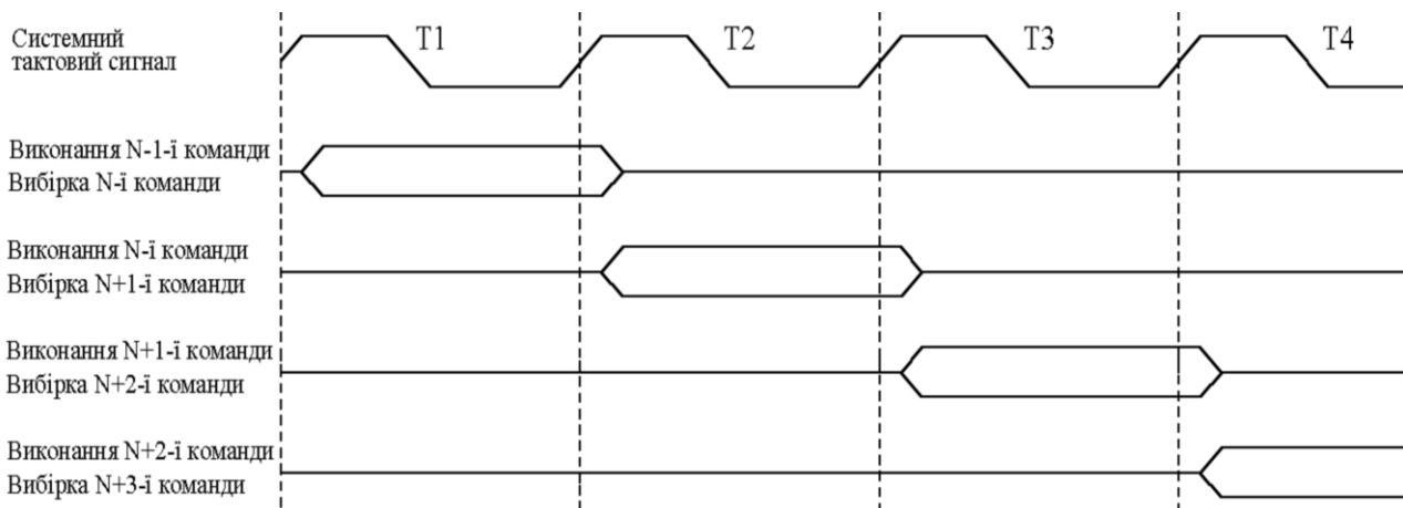
Рисунок 99. Робота конвеєра
