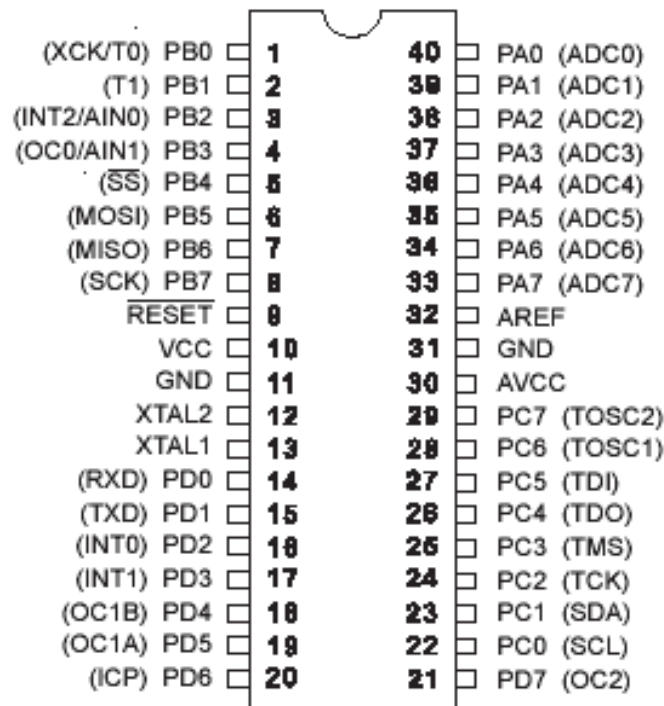
Рисунок 97. Позначення виводів мікросхеми ATmega32
