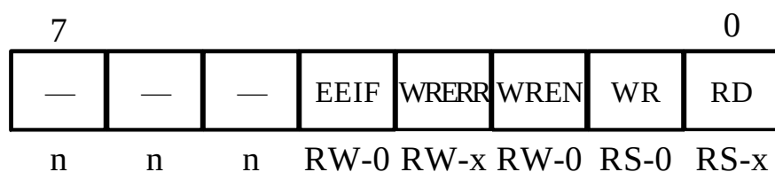
Рисунок 56. Формат регістра EECON1
