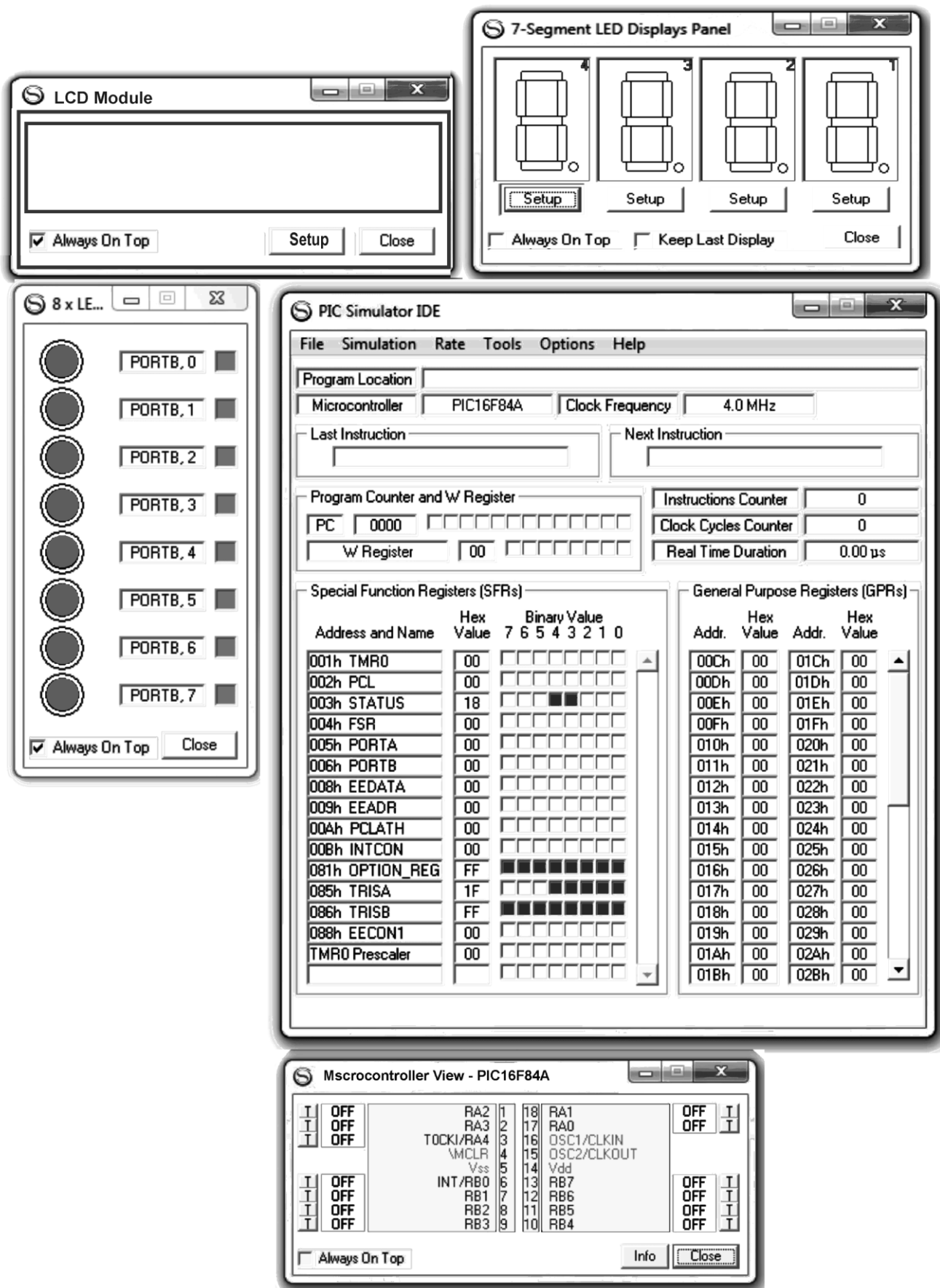
Рисунок 72. Графічне середовище програмного симулятора PIC Simulator IDE
