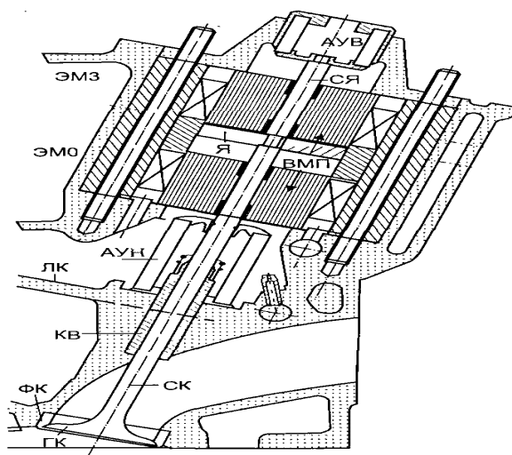
Рисунок 9.6 – Газорозподільний клапан
