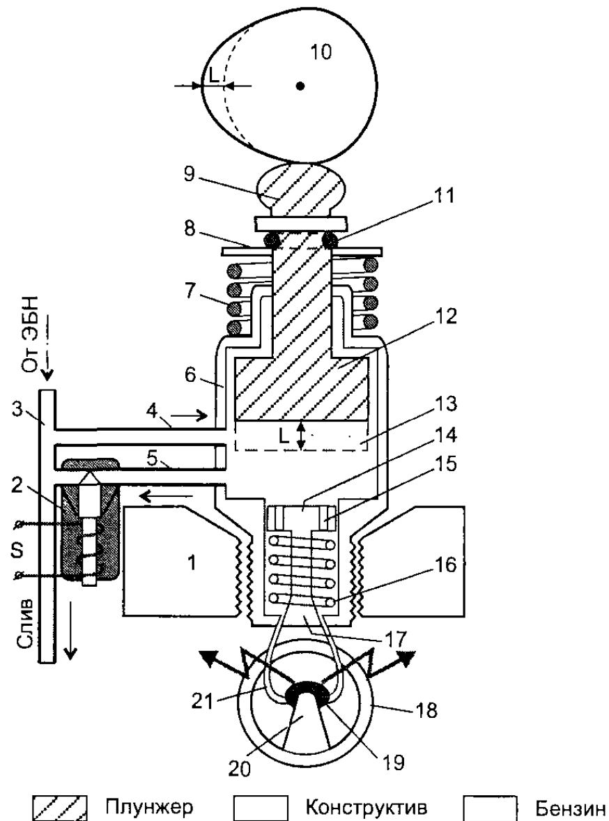
Рисунок 1.2 - Насос-форсунка системи впорскування бензину
