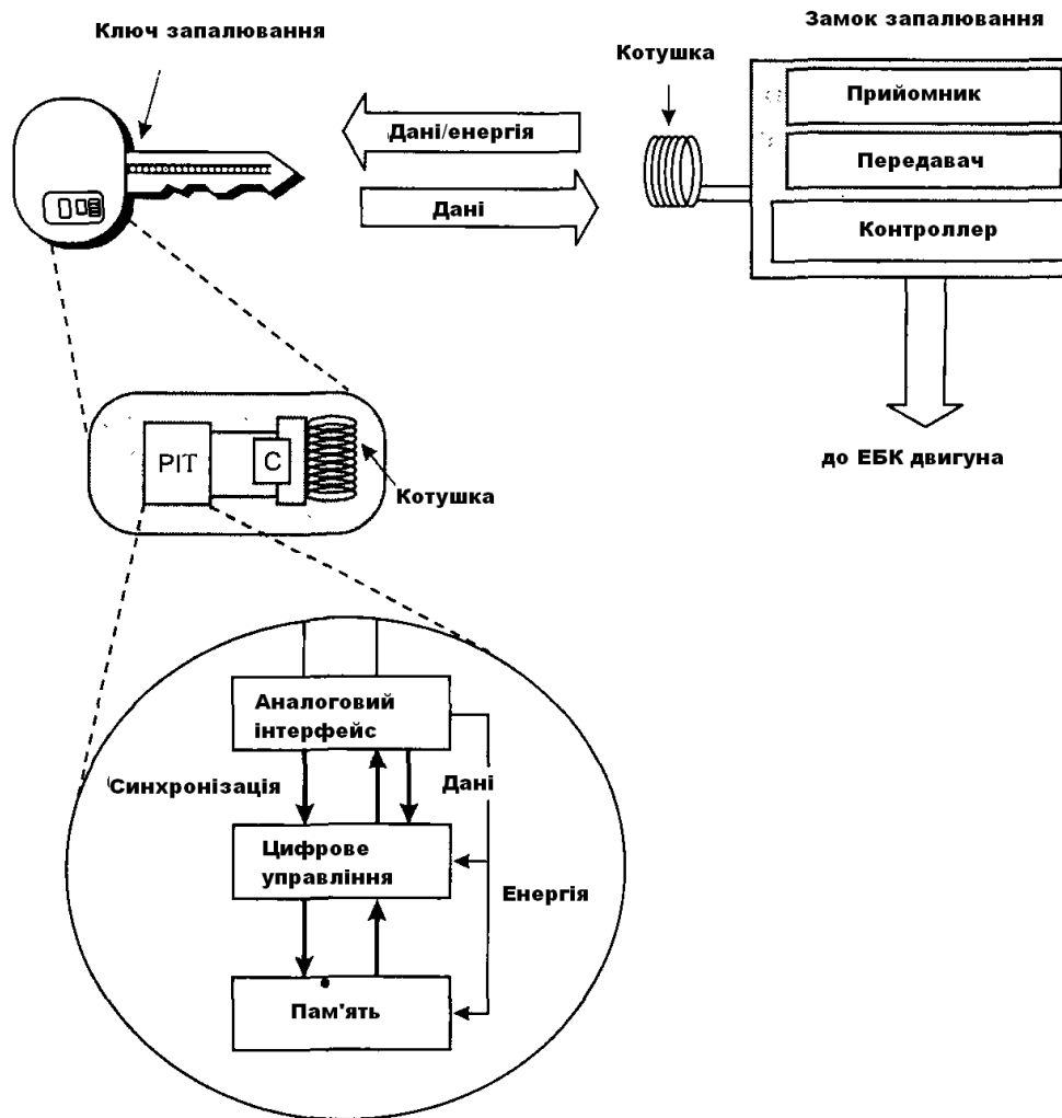
Рисунок 5.35 - Імобілізатор з транспондером
