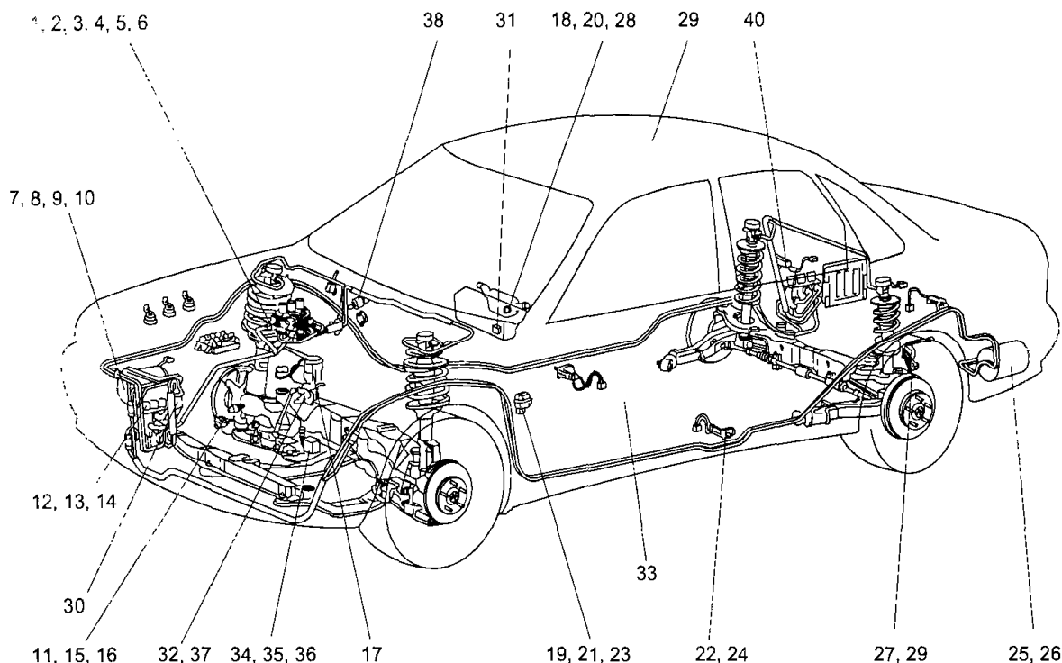
Рисунок 2.1 - Розташування датчиків на автомобілі
