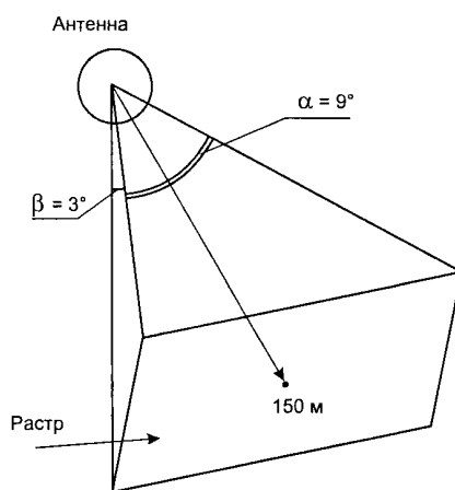
Рисунок 2.31 Растр Радіовипромінювача
