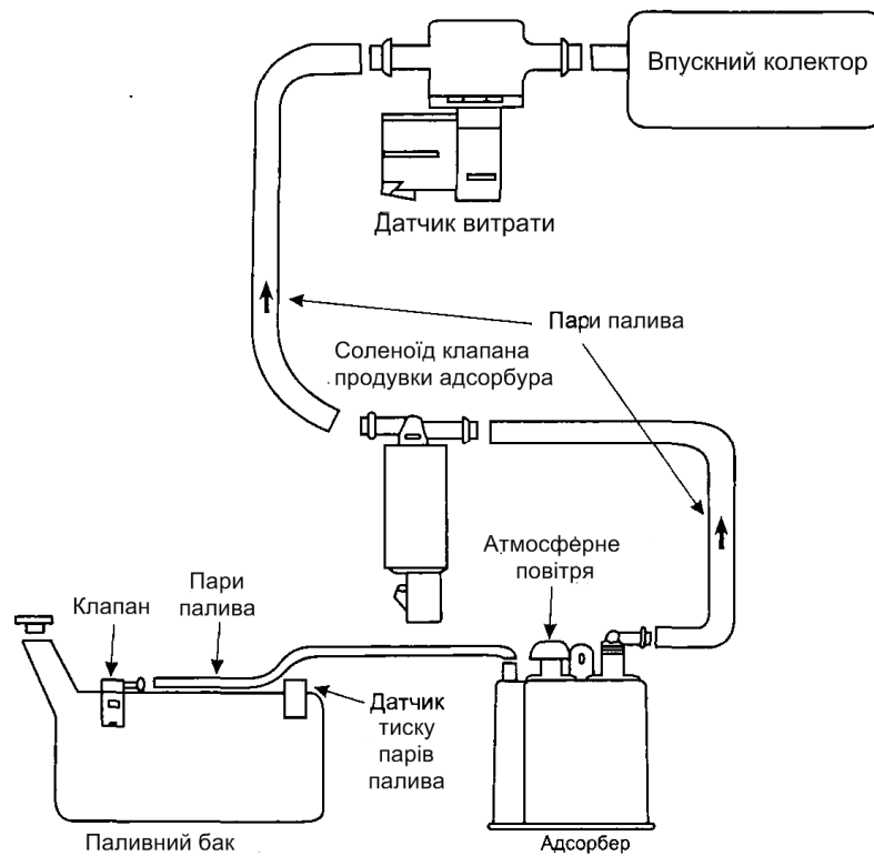
Рисунок 3.9 - Схема уловлювання парів палива на баку
