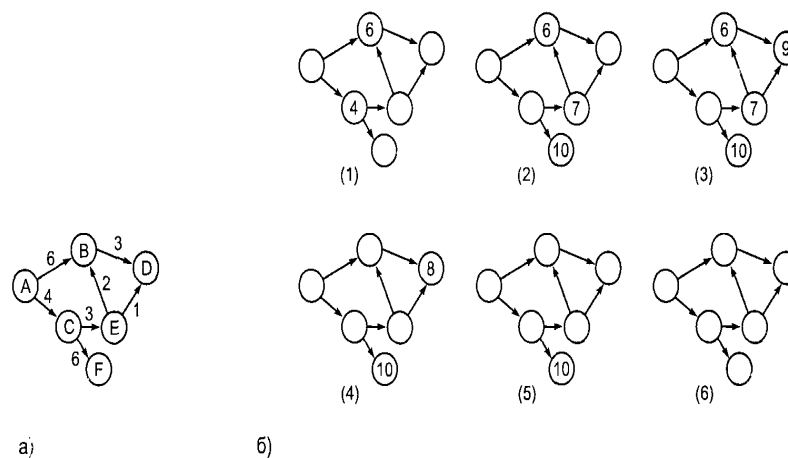
Рисунок 5.24 - Алгоритм Дейкстри
