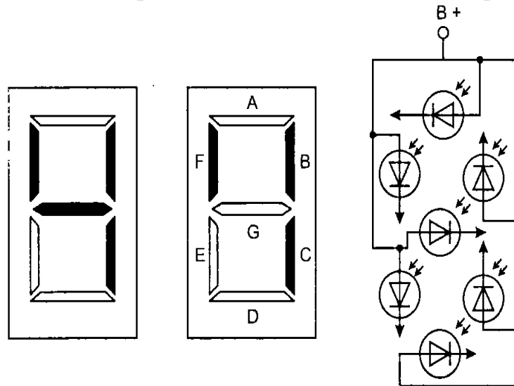
Рисунок 5.6 - Світлодіодні індикатори
