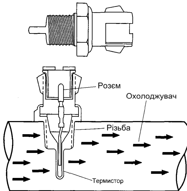
Рисунок 2.12 - Датчик температури охолоджувальної рідини
