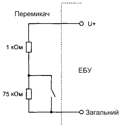
Рисунок 2.22 - Мікровимикач з можливістю діагностування
