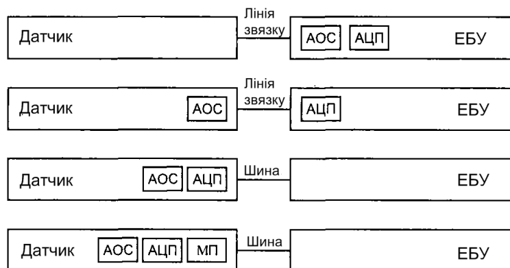
Рисунок 2.42 - Інтеграція датчиків.
