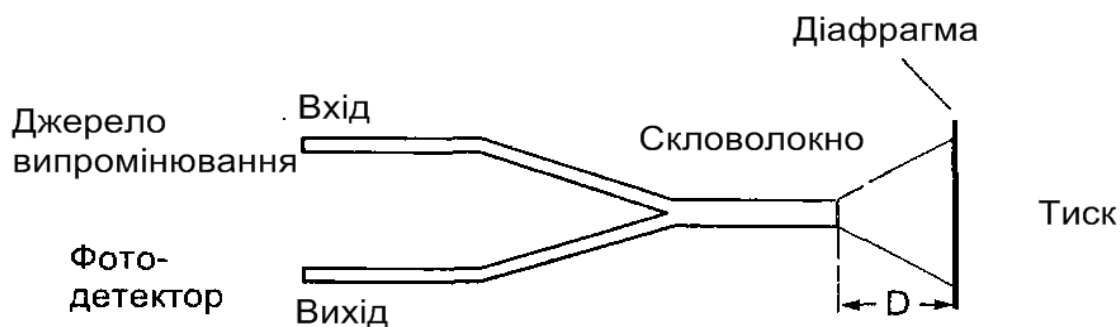
Рисунок 2.10 - Скловолокний датчик тиску
