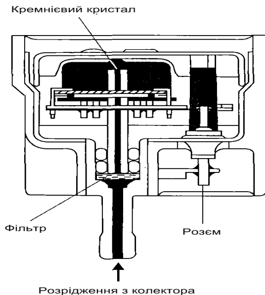
Рисунок 2.5 - Датчик розрідження у впускному трубопроводі
