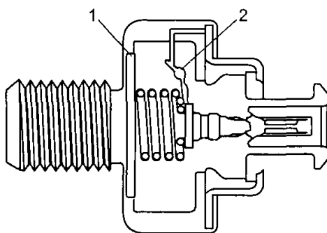
2.36 - Датчик детонації.
