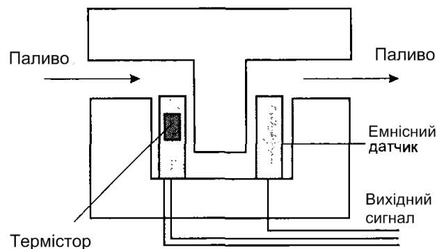
Рисунок 2.39 Датчик метанолу
