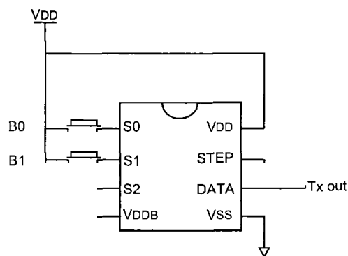
Рисунок 5.34 - Шифратор
