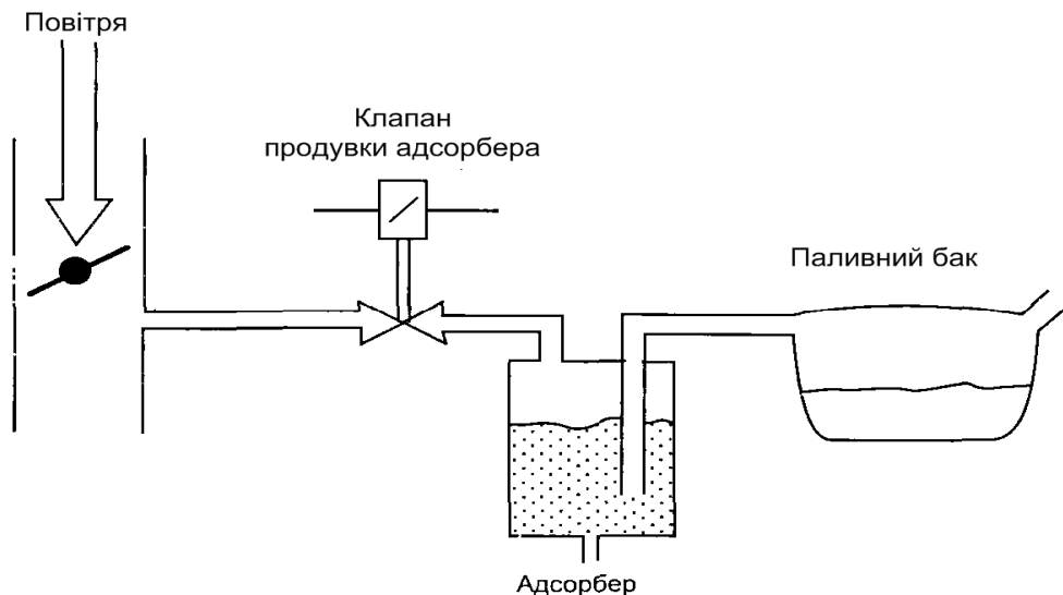
Рисунок 2.7 - Система уловлювання парів бензину
