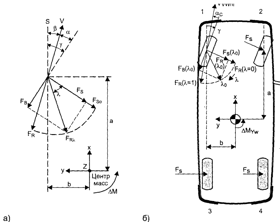
Рисунок 8.2 - СИЛИ, які діють на колеса автомобіля під час повороту
