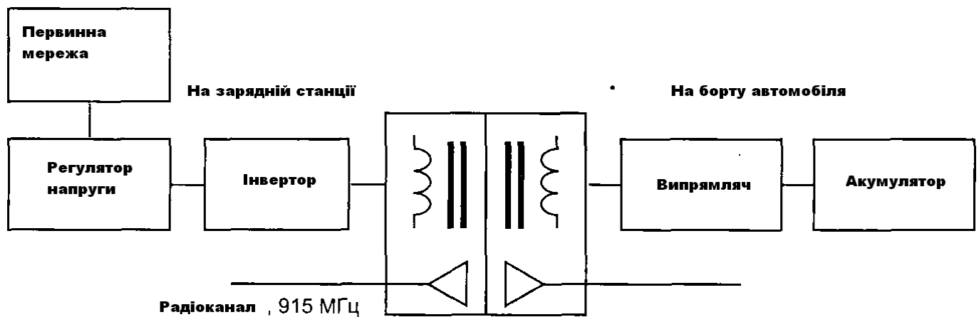
Рисунок 10.2 - Підключення з гальванічною роз'язкою
