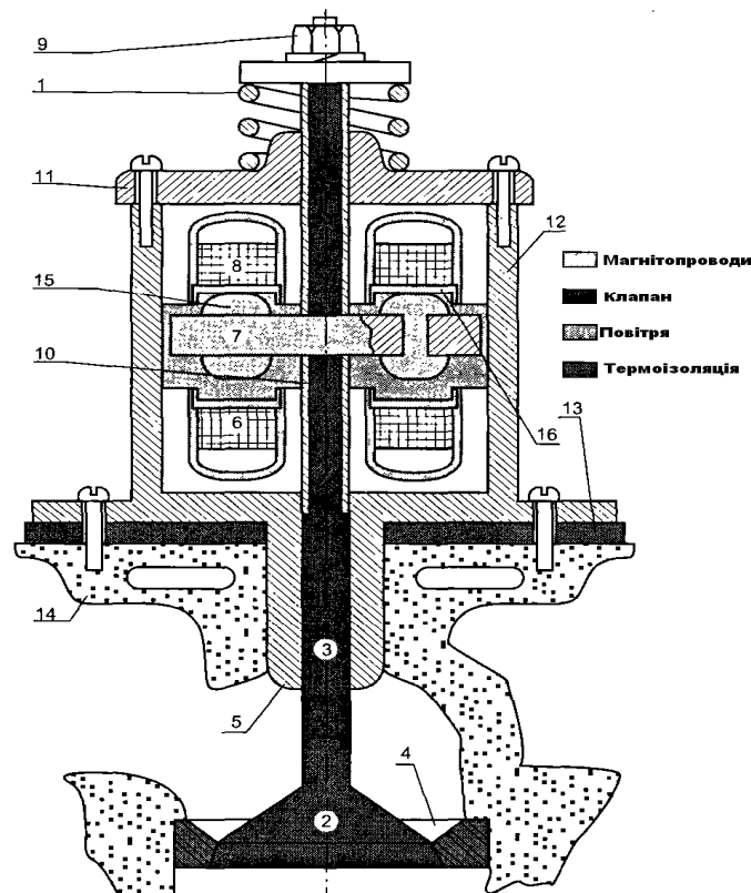
Рисунок 9.5 - Електромагнітний клапан без поворотної запірної пружини
