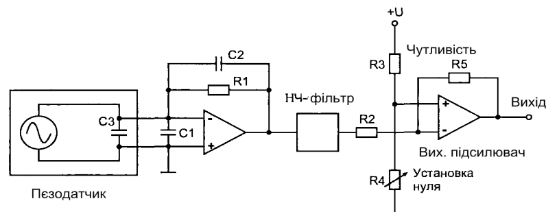
Рисунок 2.34 - Схема підсилювача-формуваця для обробки сигналу п'єзоелектричного акселерометра
