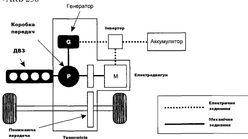
Рисунк 10.10 - Блок-схема гібридної силової установки електромобіля Toyota Prius
