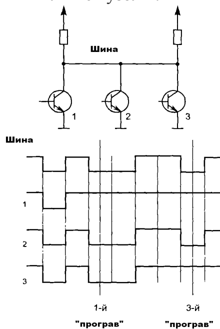
Рисунок 7.14 - Побітовий арбітраж
