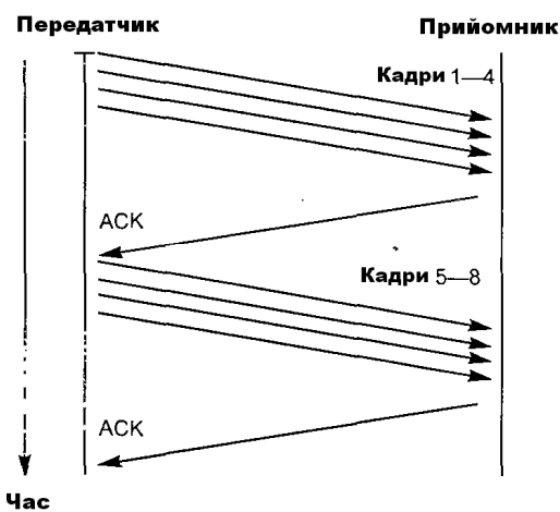
Рисунок 6.20 – Блоки кадрів
