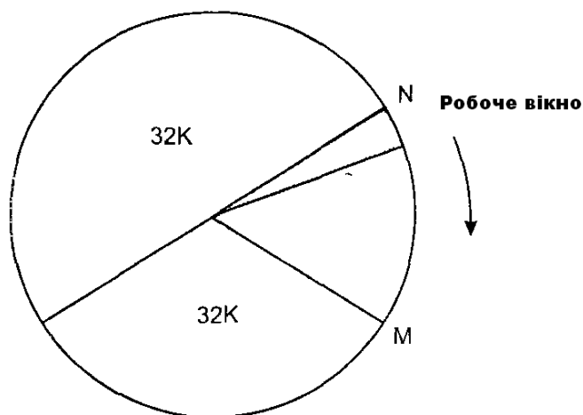
Рисунок 5.30 - Алгоритм синхронізації
