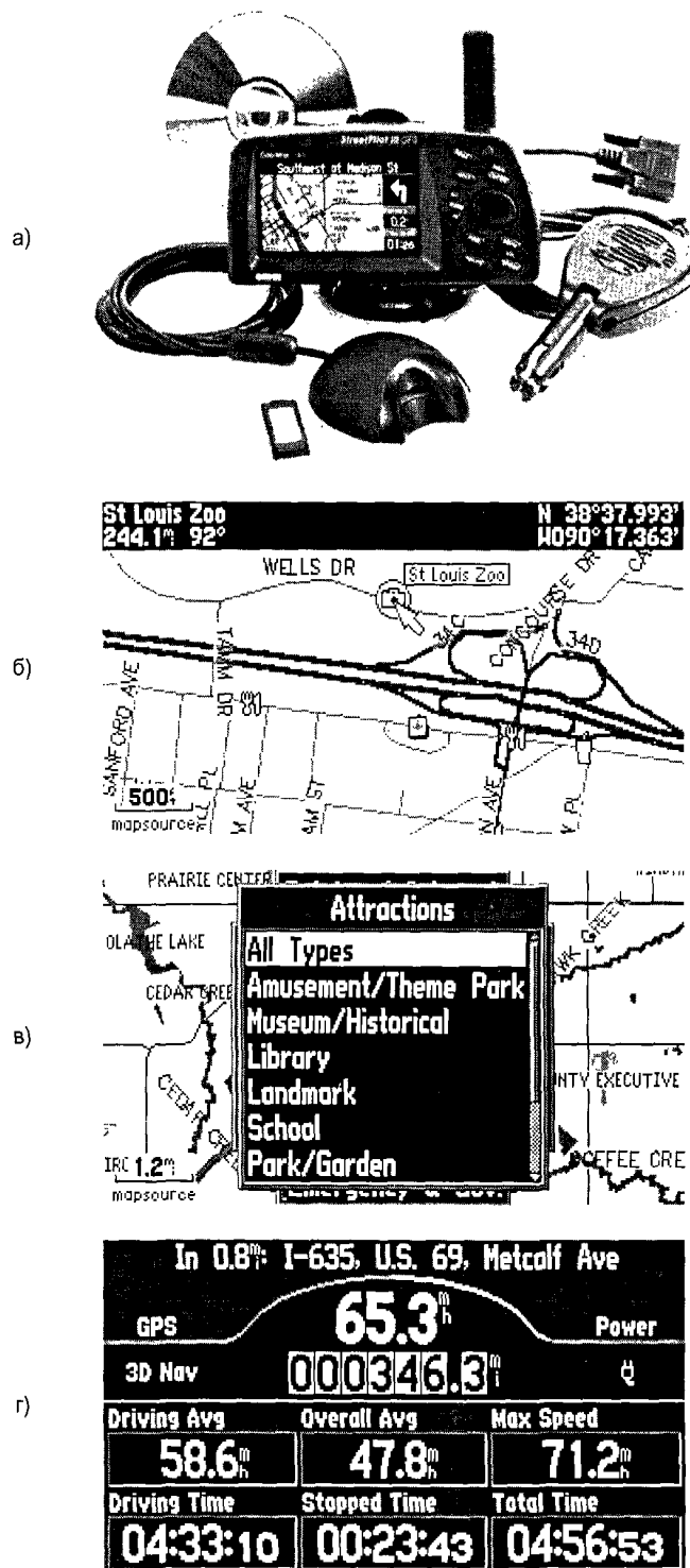
Рисунок 5.27 - Автомобільна навігаційна система Garmin StreetPilot III:
