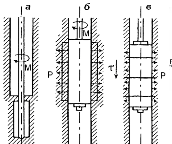
Рис. 4.4. Схема випробування ґрунтів на зріз: а – обертальний; б – кільцевий; в – поступальний
