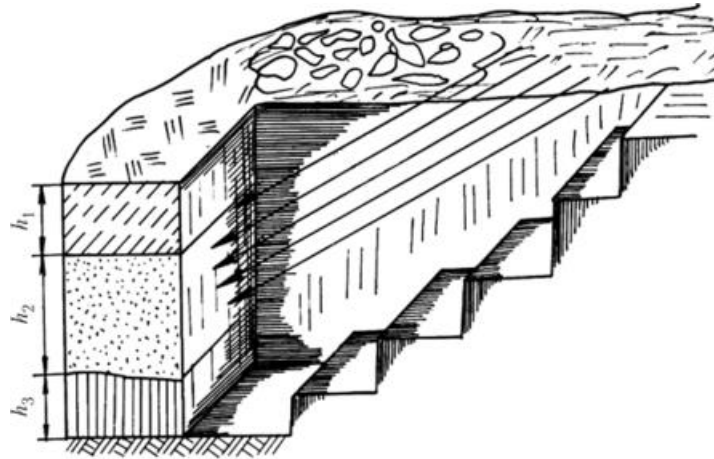
Рис. 2.2. Схема шурфу
