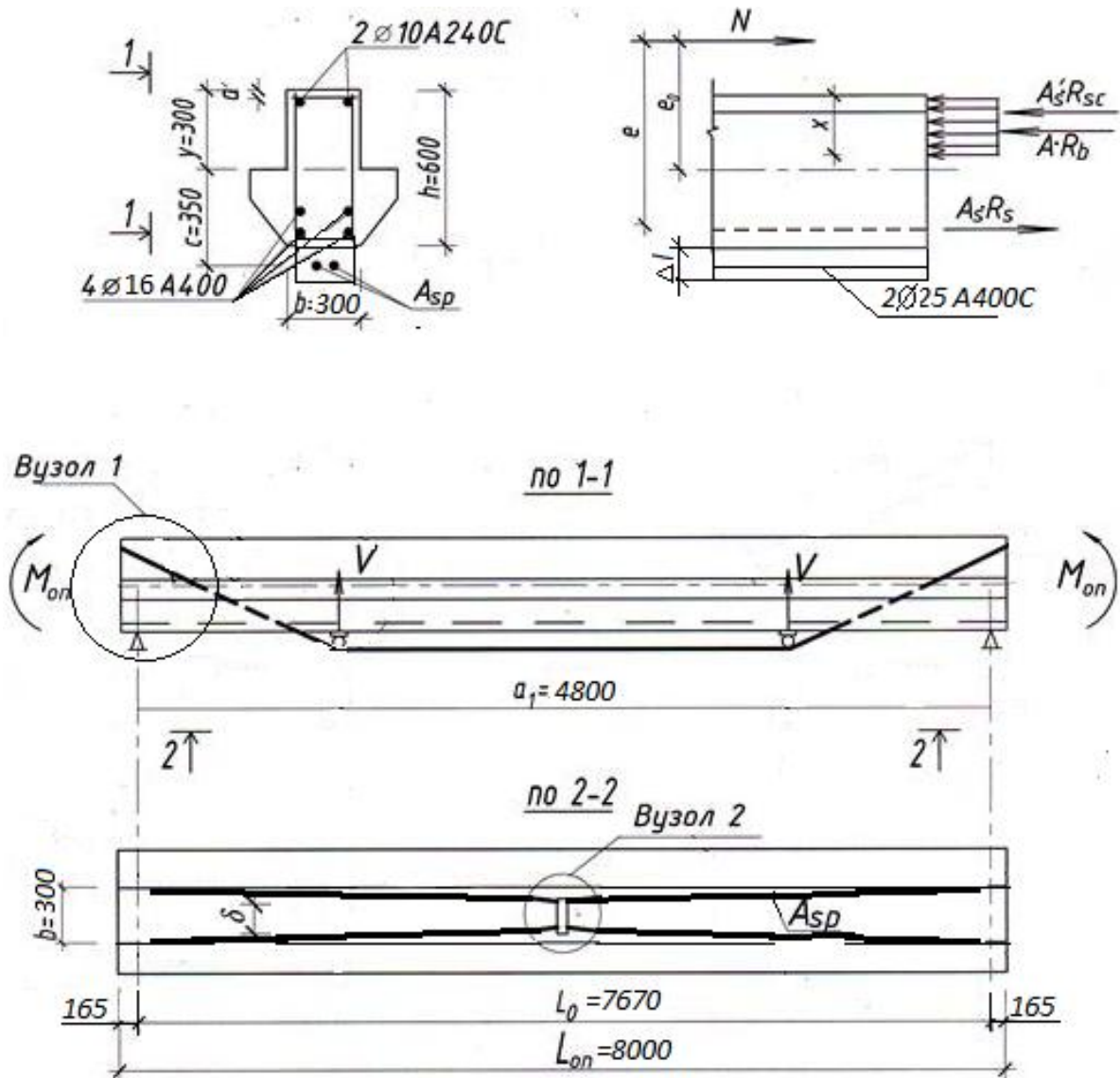
Рисунок 4.1 - Підсилення балки горизонтальною стяжкою
