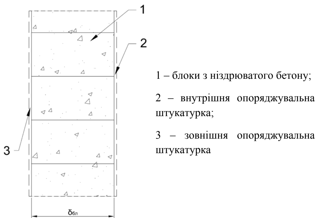
Рисунок 4.1 – Загальний вигляд конструктивного рішення зовнішньої стіни
