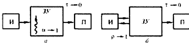
Рис. 18.3 Методи ізоляції при розташуванні джерела (И) і приймача (П) з різних боків від захисного пристрою (ЗУ): а - енергія поглинається; б - енергія відбивається
