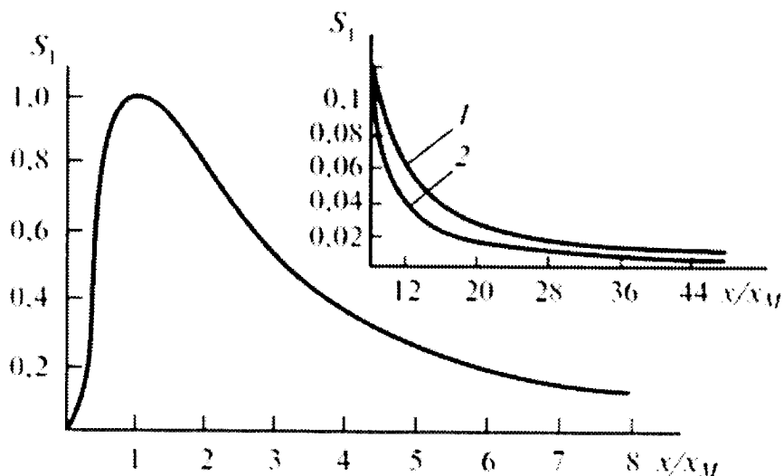
Рис. 8.4 Залежність безрозмірної величини S_1 від відношення x/x_M :
