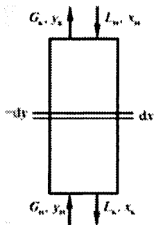
Рис. 7.3 Схема матеріальних потоків у масообмінному апараті:
