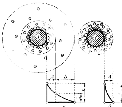
Рис. 11.1 Будова міцели:
