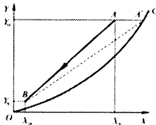
Рис. 7.4 Крива рівноваги і робоча лінія процесу абсорбції
