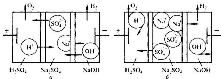
Рис. 11.9 Схеми електродіалізу з пористими діафрагмами (а) та іонітовими мембранами (б)
