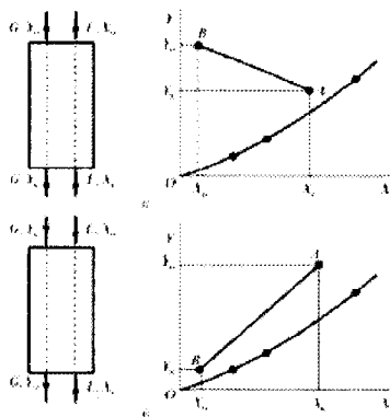
Рис. 7.5 Побудова кривої рівноваги і робочої лінії процесу абсорбції: а - прємоток руху фаз; б - протитєчїя руху фаз
