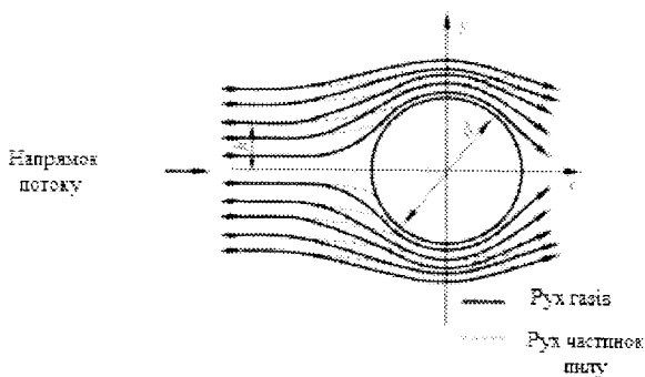
Рис. 6.5 Осадження частинок на кулі (краплі)
