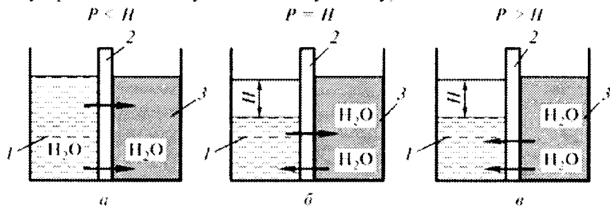
Рис. 11.6 Схеми осмосу ( H -осмотичний тиск; P - робочий тиск):
