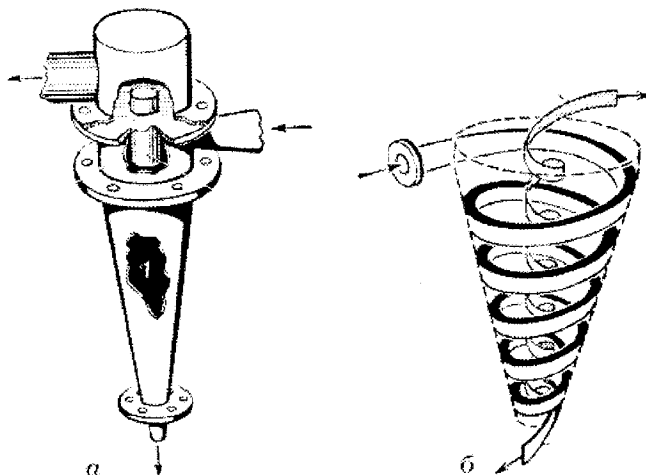
Рис. 10.2 Схема гідроциклонa а - загальний вигляд; б - схема потоків
