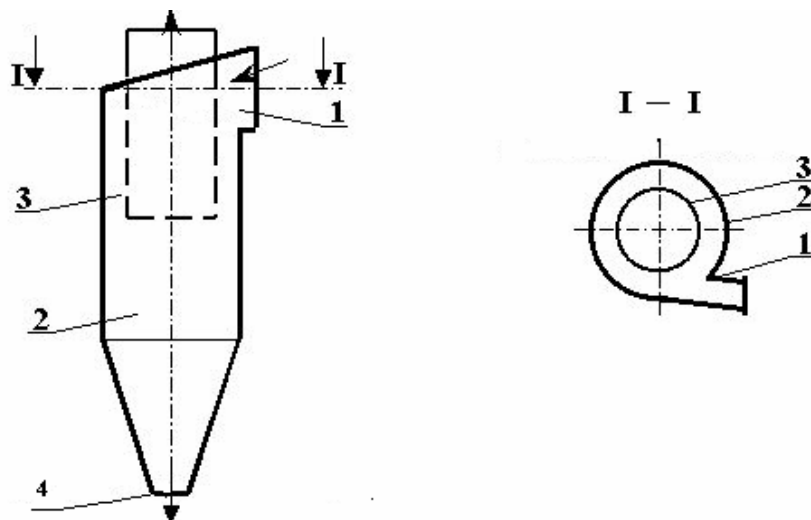
Рис. 5.2 – Схема циклону:
