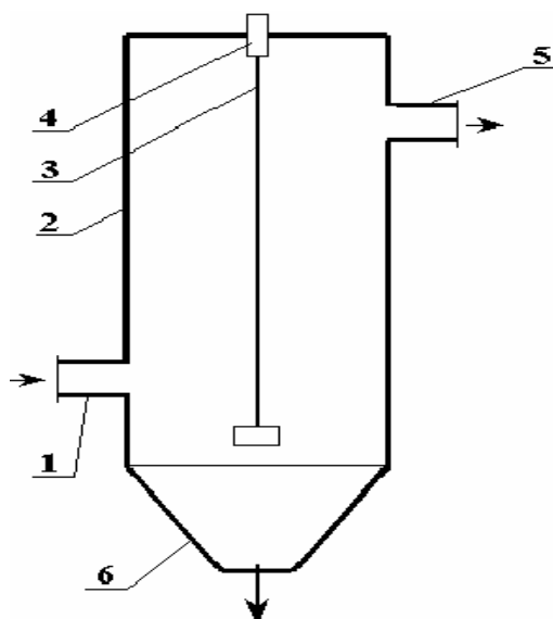
Рис. 5.3 – Схема електрофільтра:
