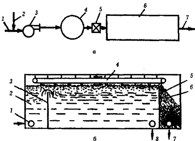
Рис. 9.3 --Напірна флотація: а – схема напірної флотаційної установки; б – схема флотовідстійника
