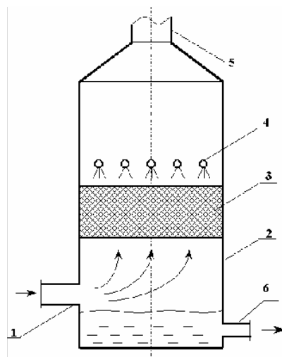
Рис. 5.6 – Схема насадочного скруббера:
