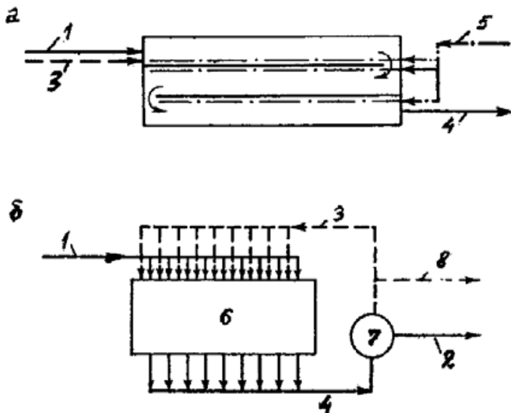
Рисунок 9.5 - Схеми аеротенків:
