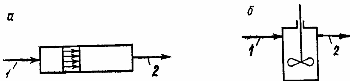
Рисунок 9.4 - Схеми роботи аеротенків:
