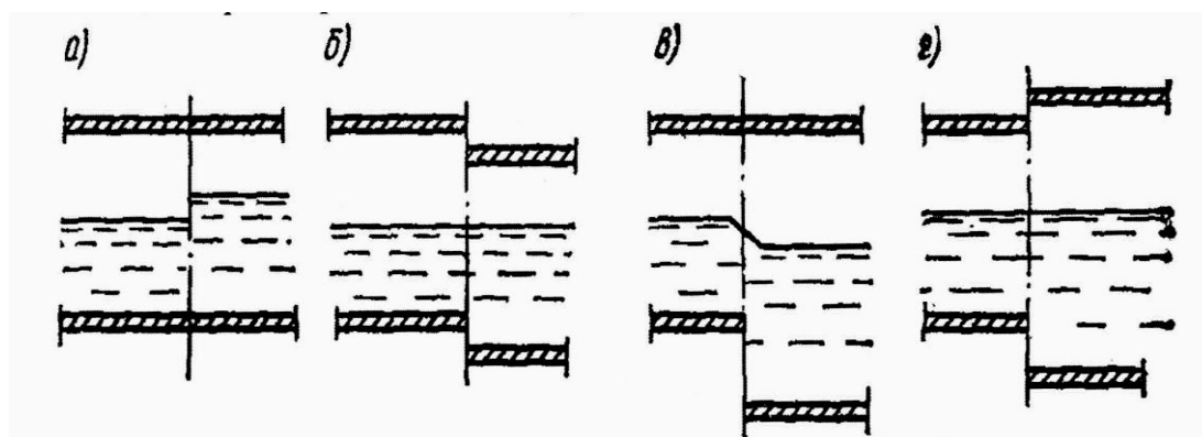
Рисунок 7.7 Схеми з'єднання каналізаційних труб
