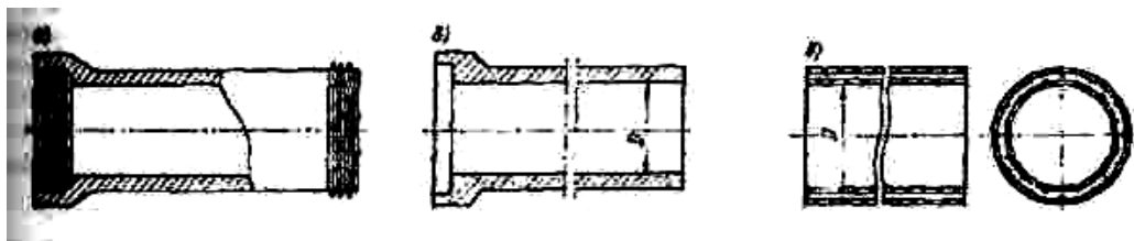
Рисунок 7.6 - Каналізаційні труби
