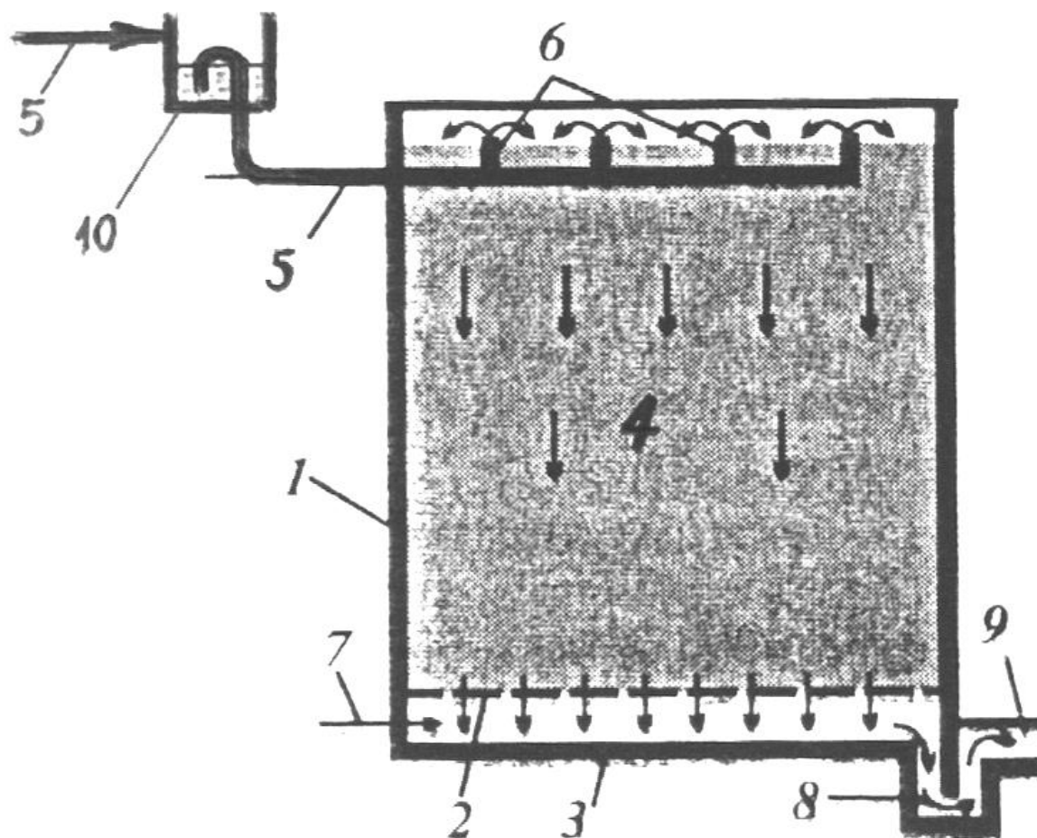
Рисунок 9.2 - Біофільтр:
