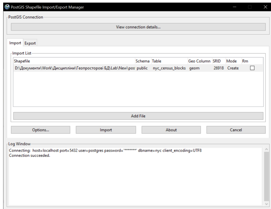
Рис. 20. Менеджер імпорту-експорту векторних даних із завантаженим файлом
