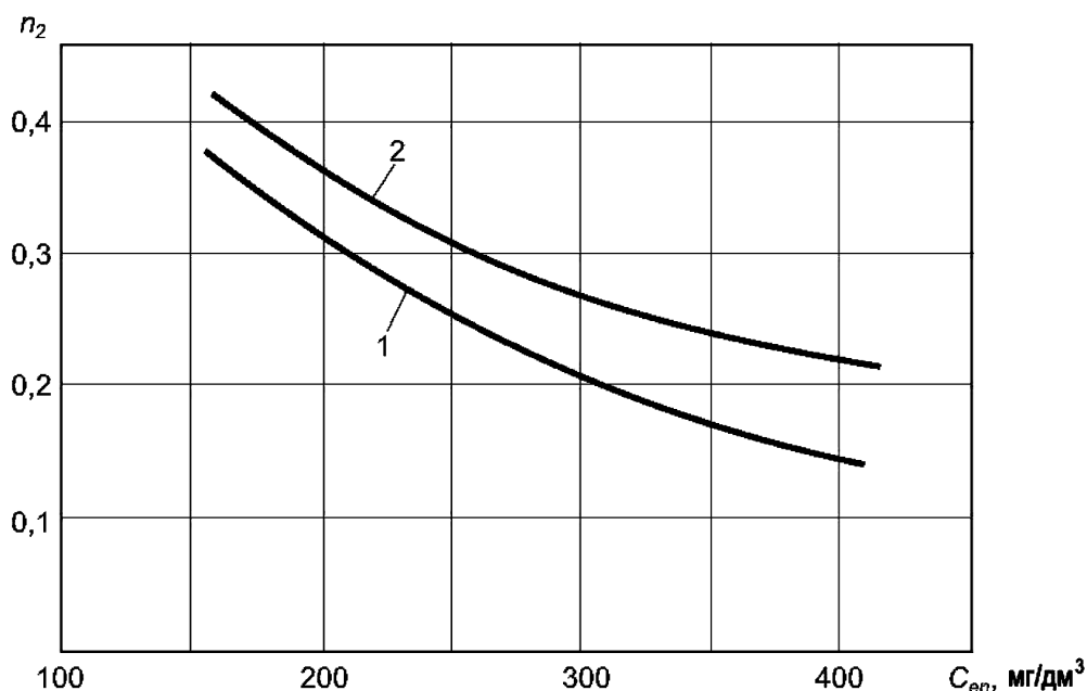
Рисунок В.1 – Залежність показника ступеня n_2 від концентрації завислих речовин C_{ен} у міських стічних водах при ефекті освітлення 50 % та 60 %
