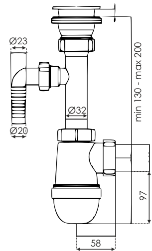
Сифон з боковим переливом
