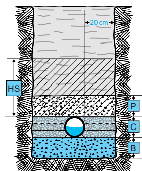
Профіль U1A
