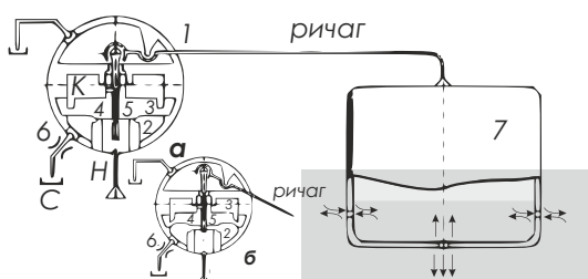
Рис. 43 - Будова поплавкового клапана: 1- корпус; 2- сопло; 3- діафрагма; 4- боковий отвір гільзи; 5- золотник з нержавіючої сталі; 6- гідродрозель; 7- поплавок; К- камера над діафрагмою; Н- напірна гідролінія; С- частина зливу
