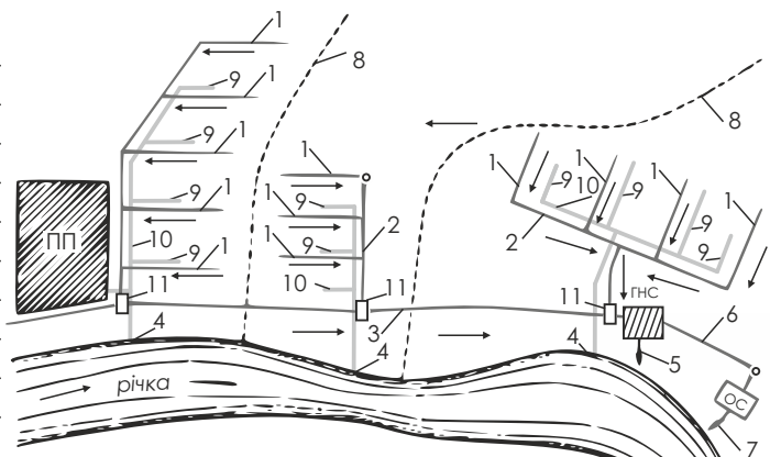
Мал. 5 - Схема напівроздільної системи водовідведення міста
