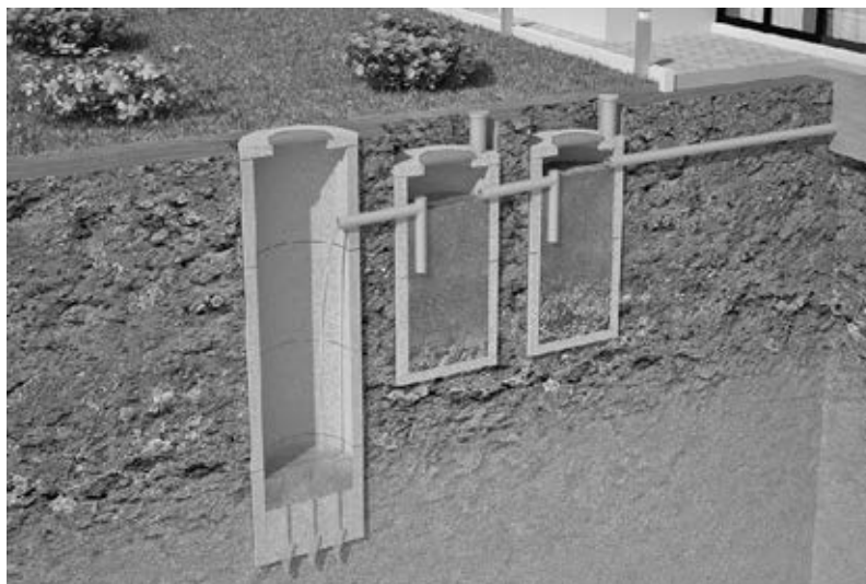
Рис. 14 – Септик
