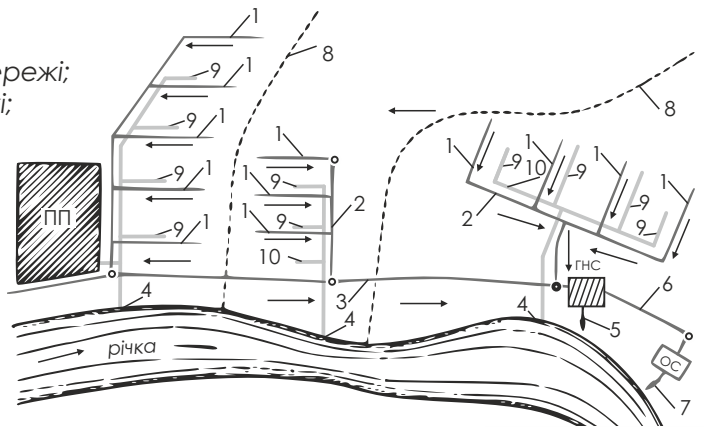
Рис. 3. - Схема повної роздільної системи водовідведення міста:
