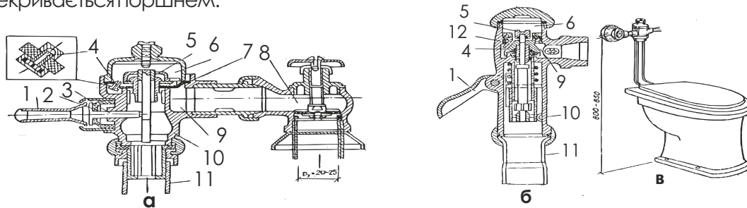
Рис. 47 - Напівавтоматичні змивні крани: а) - мембранний; б) - поршковий; в) - схема монтажу; 1-пусковий важіль; 2-гумові манжети; 3-штовхач; 4-канал; 5-клапан; 6-робоча камера; 7-мембрана; 8-вентиль; 9-вхідна камера; 10-корпус; 11-відвідна труба
