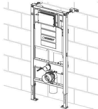
Мал. 9 - Види інсталяцій за розміщенням:
