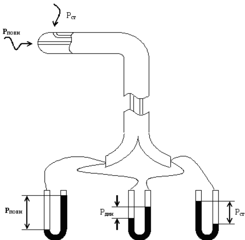
Рис.11.35. Пневмометрична трубка
