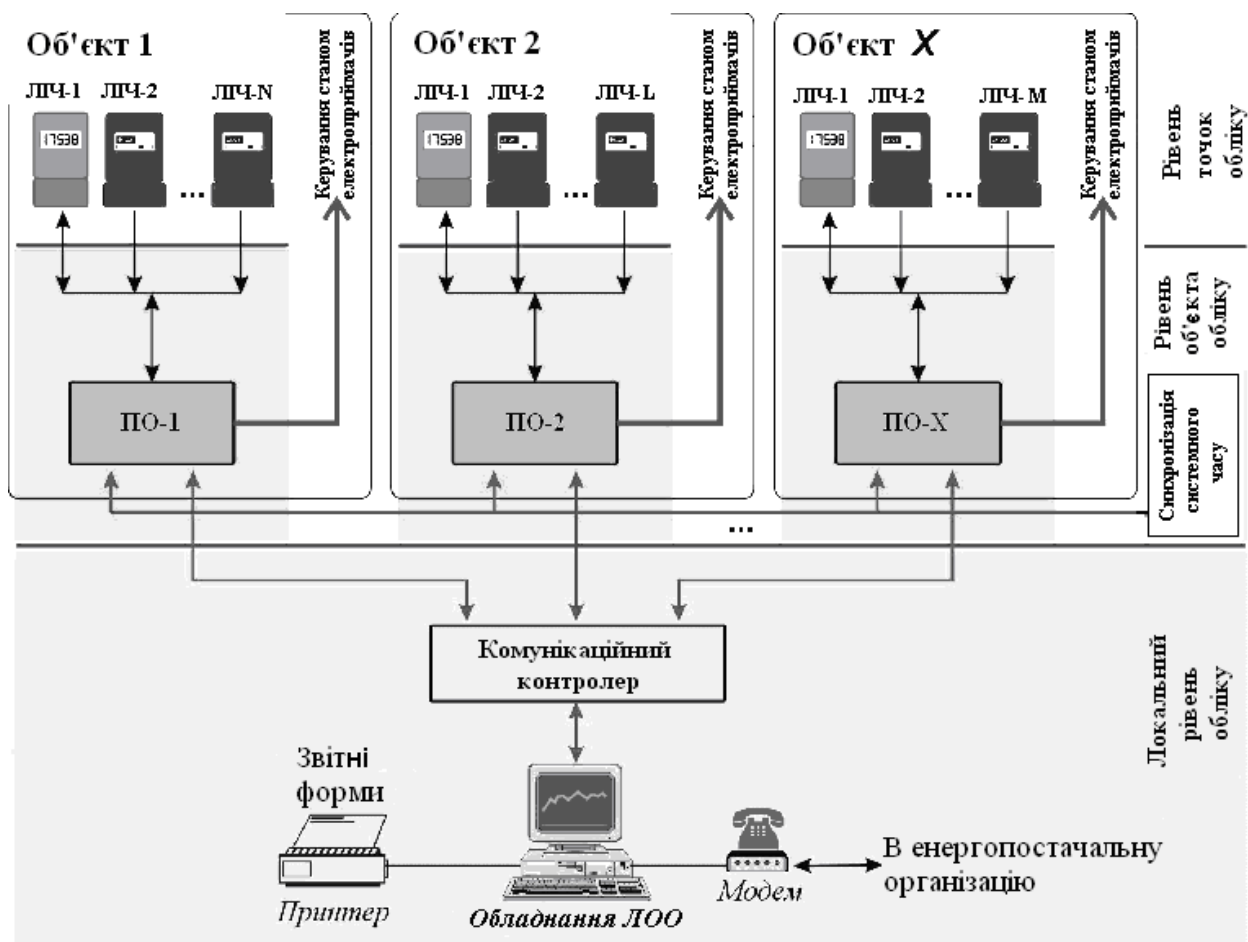
Рис. 10.9. Приклад 10.4 організації обліку споживання енергетичних ресурсів
