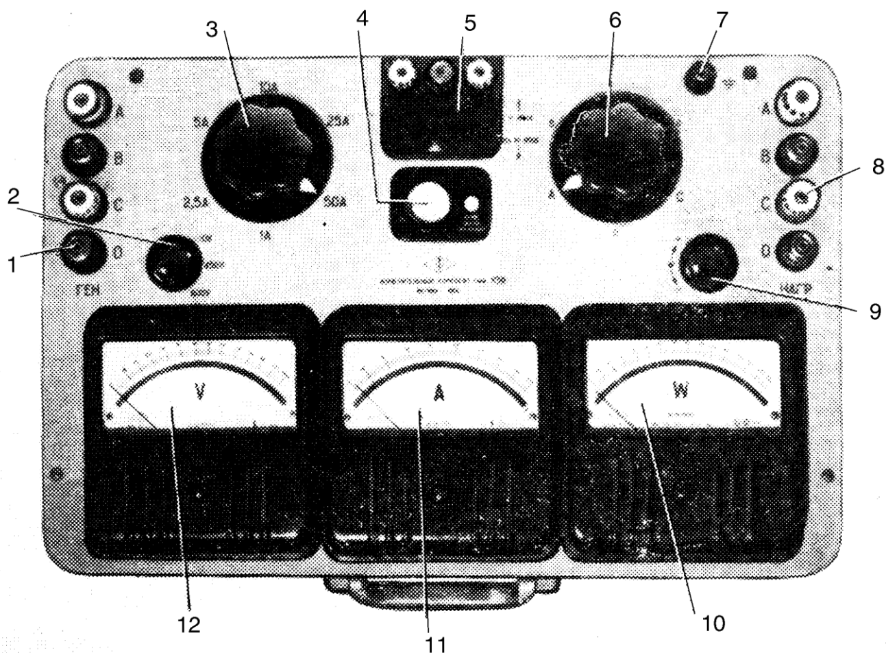
Рис. 11.3. Вимірювальний комплект К-50.
