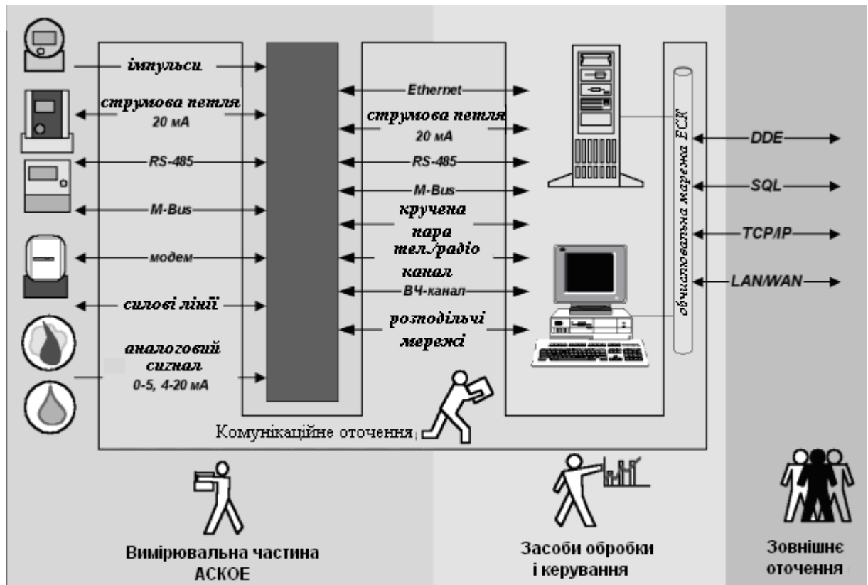
Рис. 10.4. Комунікаційна підсистема
