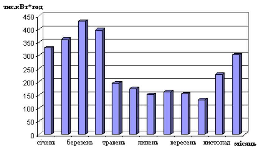
Рис. 9.3. Споживання електроенергії.
