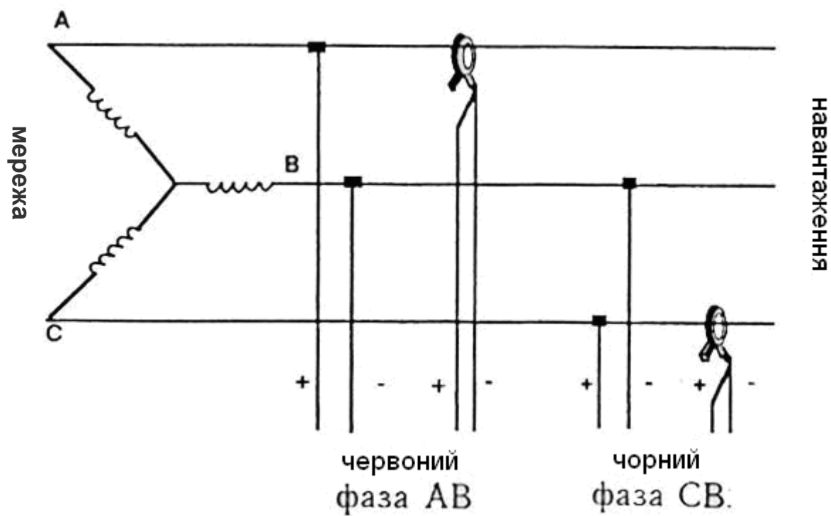
Рис. 11.9. 3-х фазне 2-х елементне приєднання (сполучення типу "зірка")
