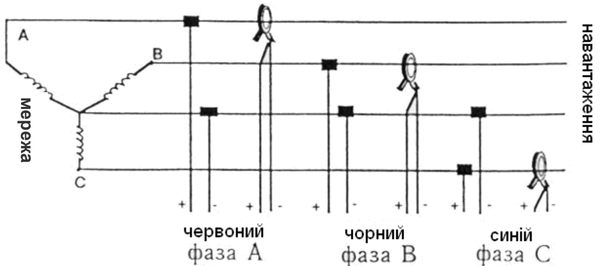
Рис. 11.7. 3-фазне 3-елементне приєднання (4 провідне сполучення "зірка")
