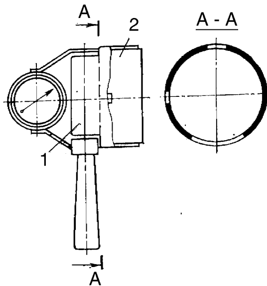
1 – анемометр, 2 - насадка
