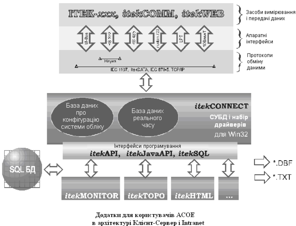
Рис. 10.5. Структура програмного забезпечення АСОЕ
