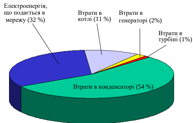
Рис. 7.4. Кругова діаграма для сучасної електростанції
