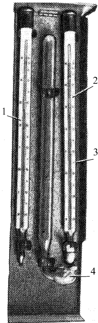
Рис. 11.37. Простий психрометр
