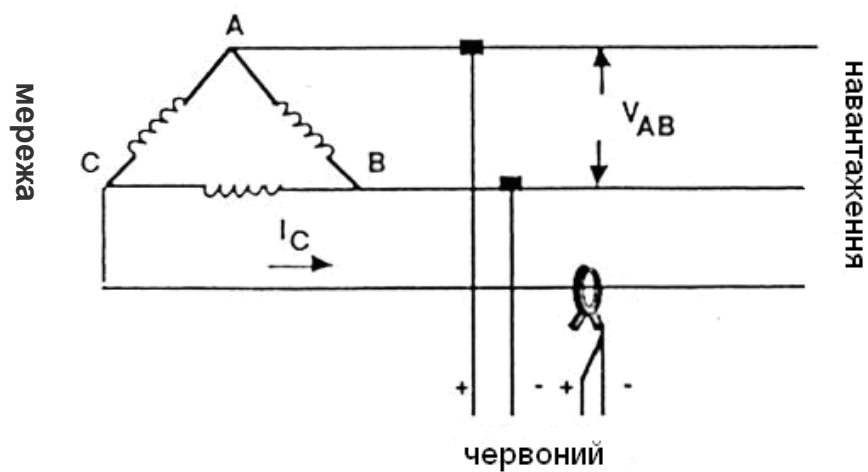
Рис. 11.12. Схема вимірювання у випадку симетричного навантаження з'єднаного в "трикутник".
