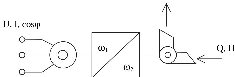
Рис. 4.1. Структурна схема вентиляційної системи
