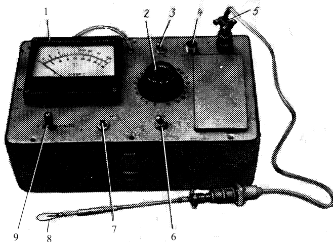
Рис. 11.29. Термоанемометр конструкції ВНИИГС.
