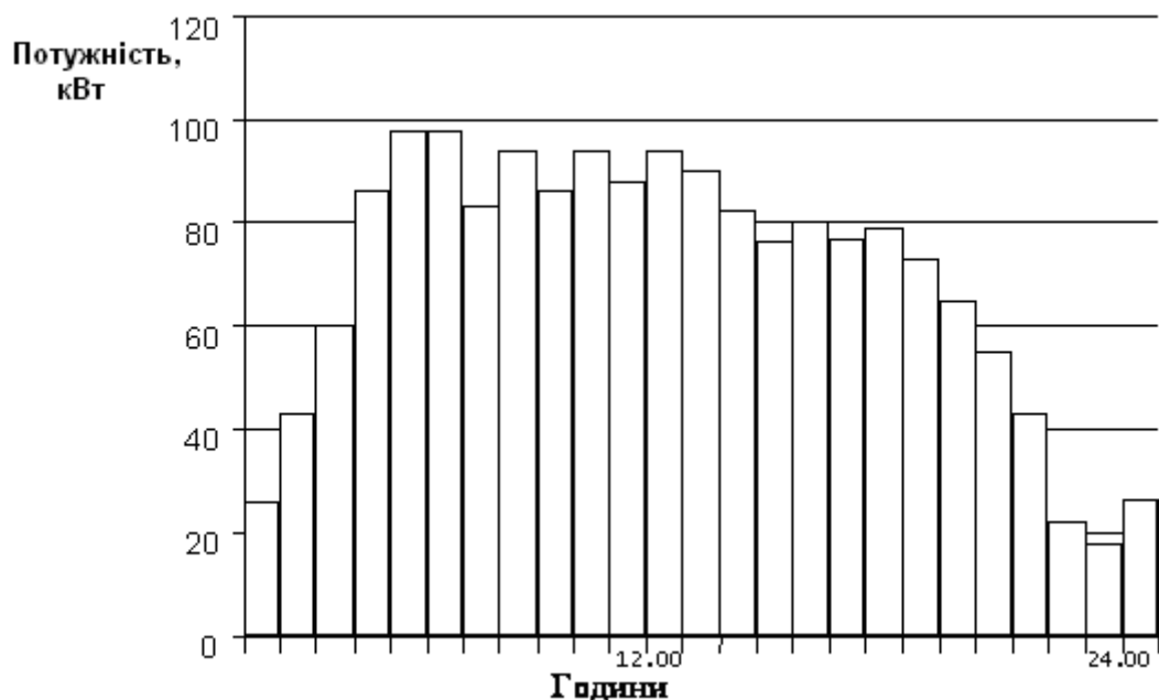
Рис. 3.2. Добовий графік навантаження
