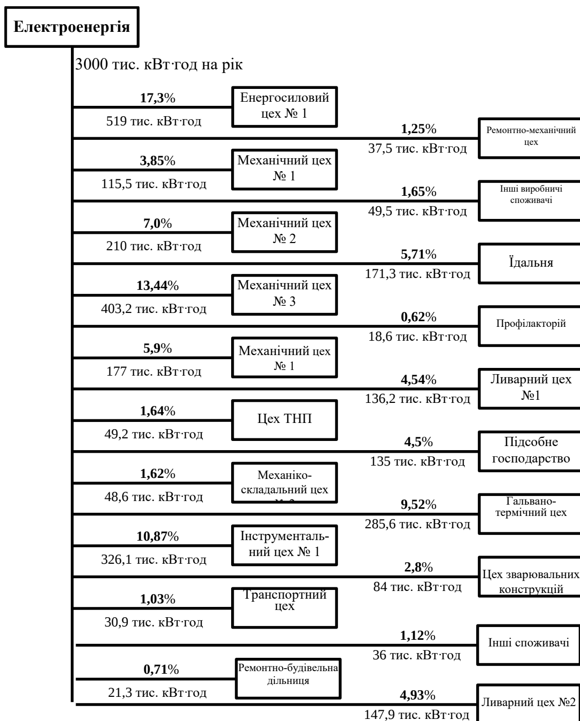
Рис. 9.8. Баланс споживання електроенергії підприємством «Молот» у 2002 р.
