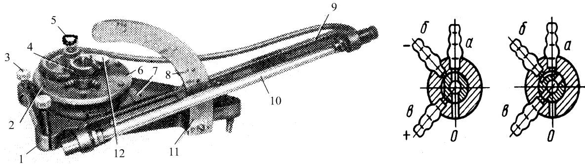
Рис. 11.34. Мікроманометр ММН
