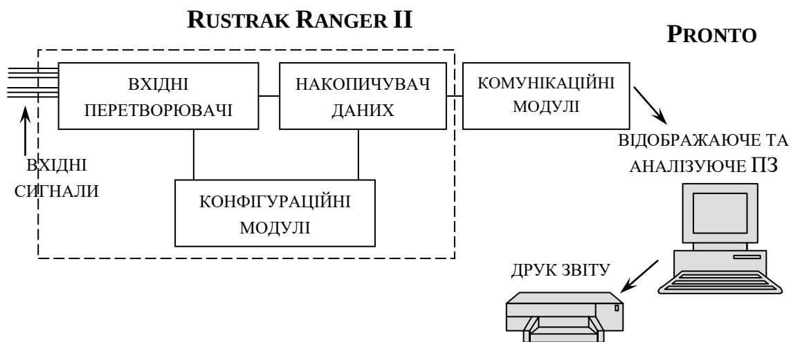
Рис. 11.6. Блок-схема комплексу Rustrak Ranger II.
