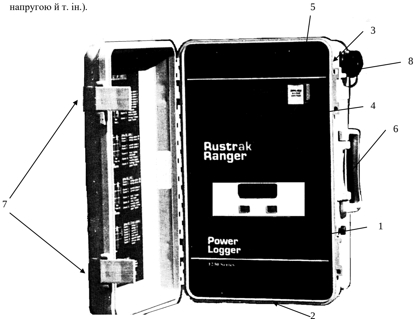
Рис. 11.5. Комплексний вимірювальний прилад Rustrak Ranger II:
