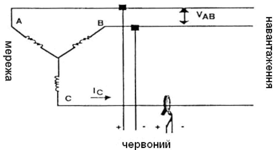
Рис. 11.11. Схема вимірювання у випадку симетричного навантаження з'єднаного в "зірку".
