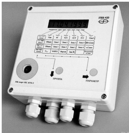
Рис. 10.3. Пристрій ІТЕК-420
