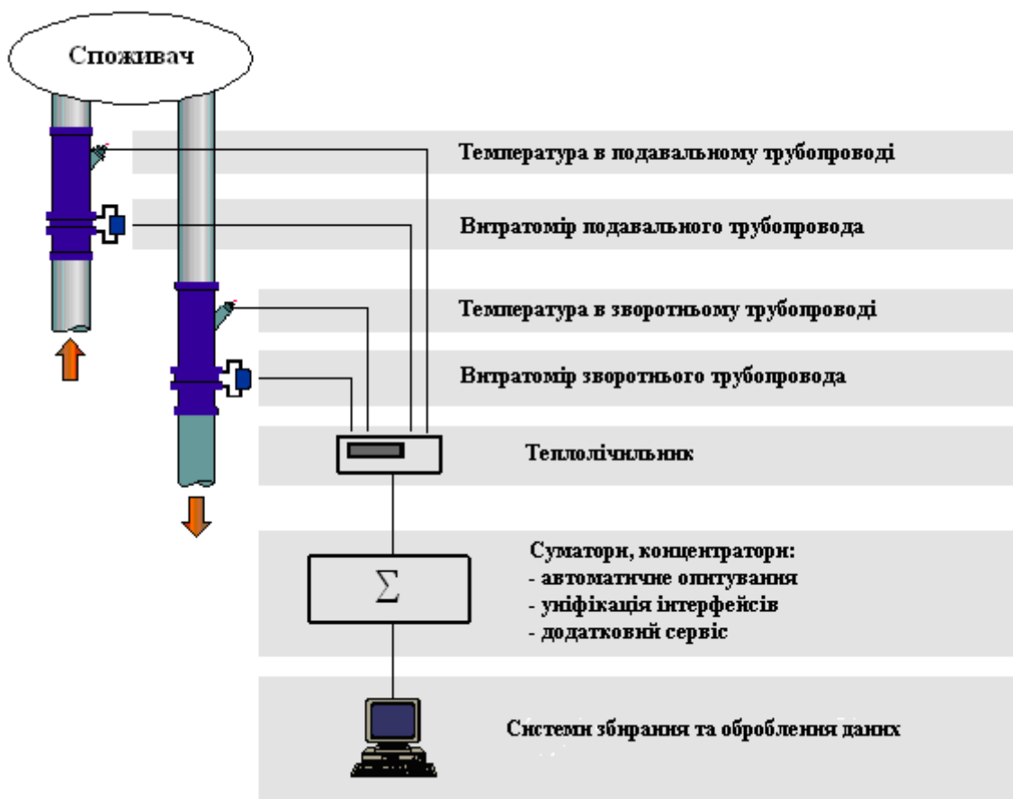
Рис. 11.41. Система збирання інформації і вимірювання теплової енергії
