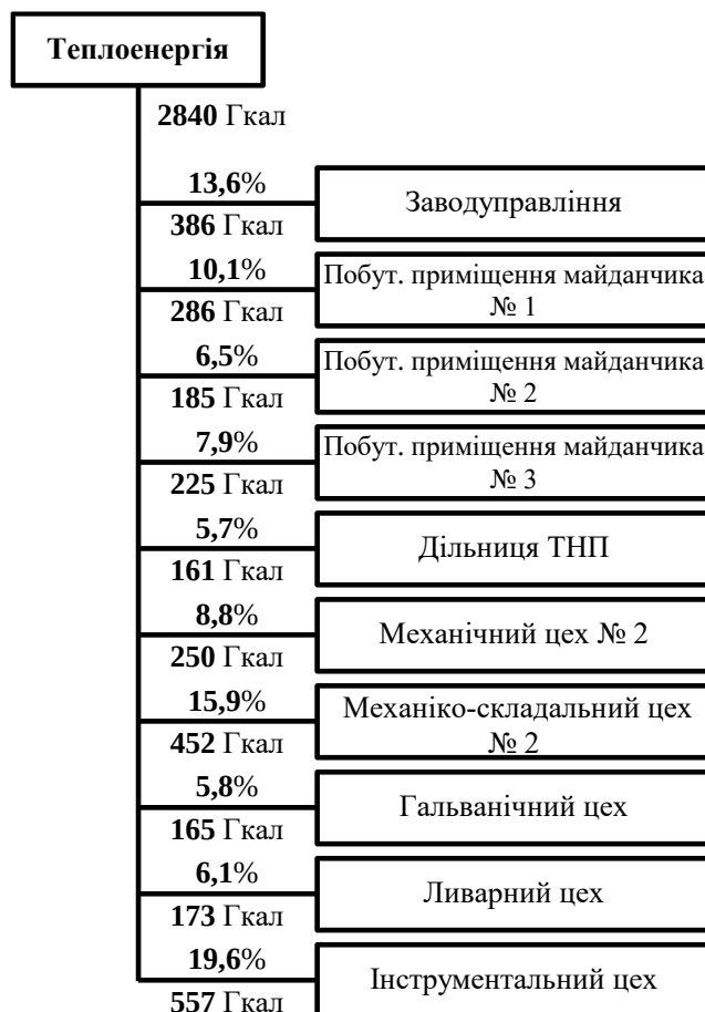
Рис. 9.11. Баланс споживання теплової енергії підприємством «Молот» у 2002 р.
