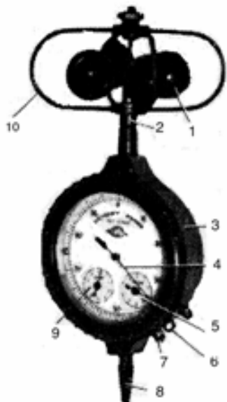
Рис. 11.26 Чашковий анемометр МС-13
