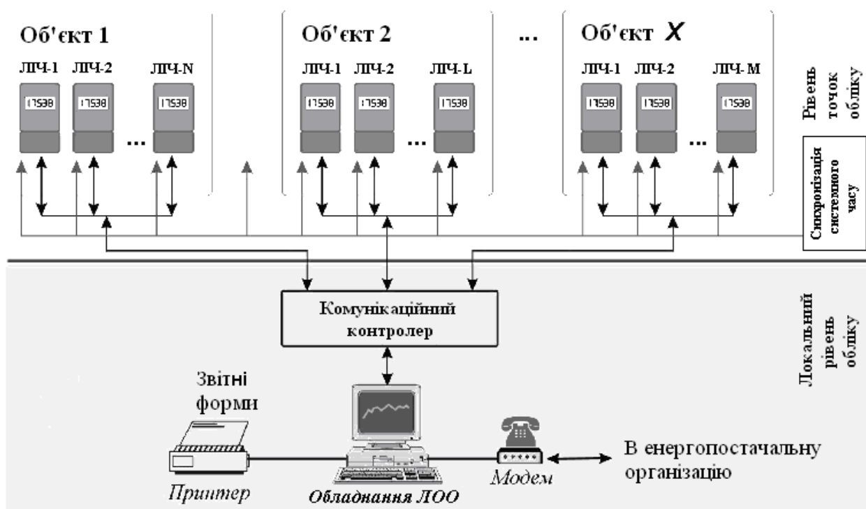
Рис. 10.8. Приклад 10.3 організації обліку споживання енергетичних ресурсів
