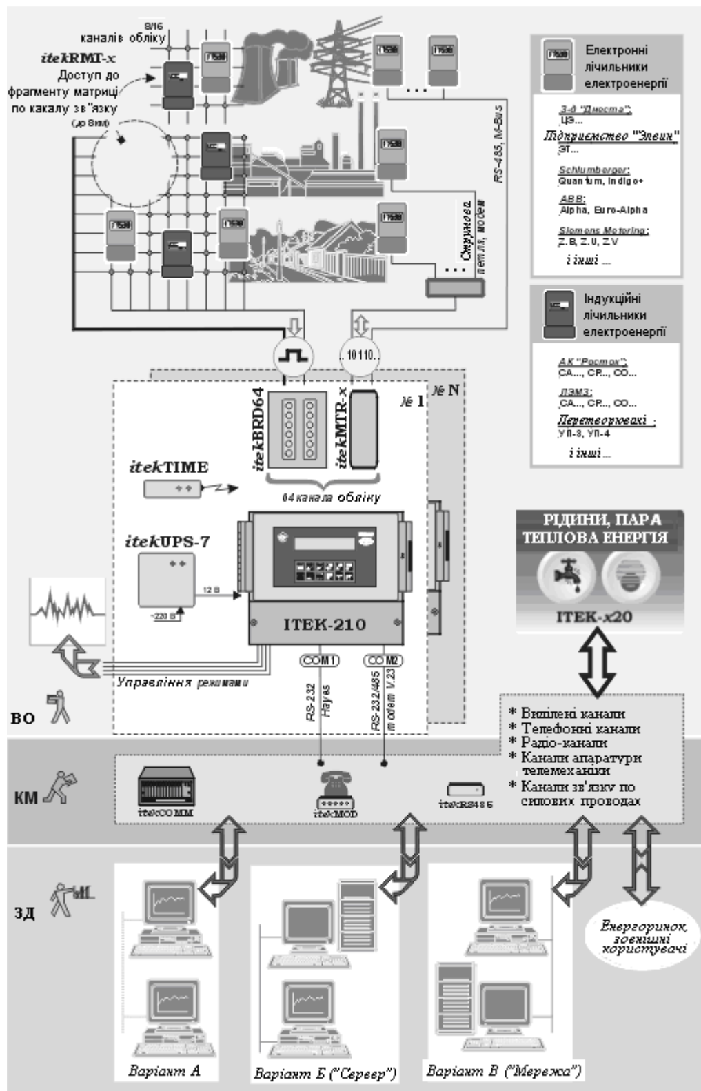
Рис. 10.1. Загальна схема організації обліку енергоресурсів
