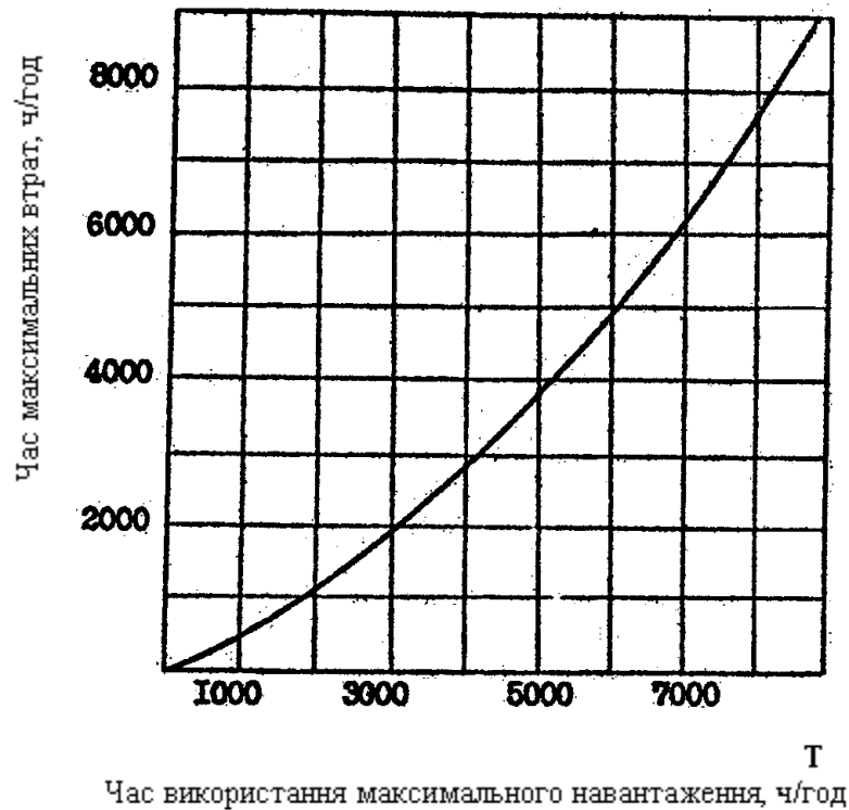
Рис. 8.7. Залежність часу максимальних втрат від часу використання максимального навантаження
