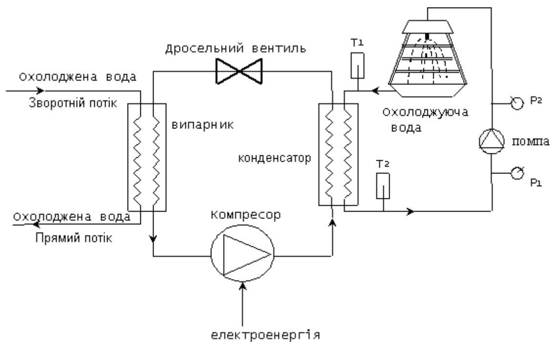
Рис. 4.2. Парокомпресійна система охолодження
