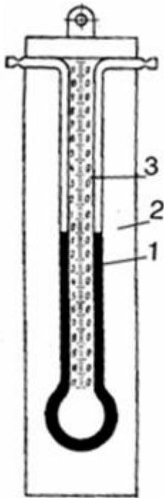
Рис 11.31 Рідинні манометри
