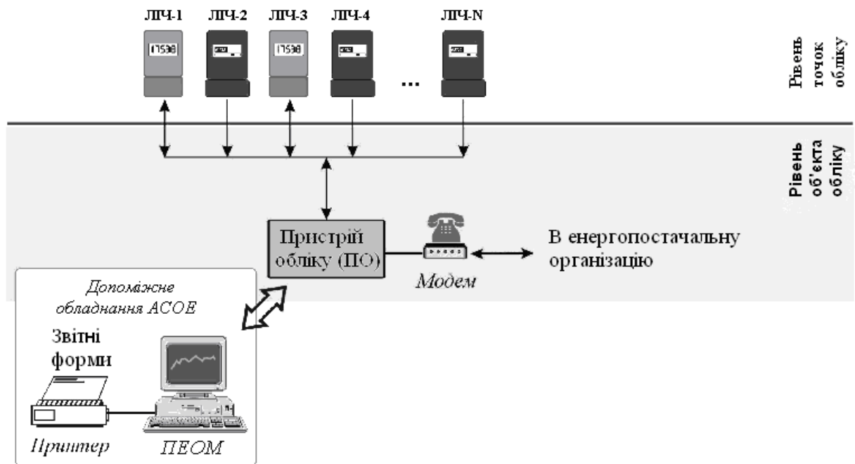
Рис. 10.7. Приклад 10.2 організації обліку споживання енергетичних ресурсів
