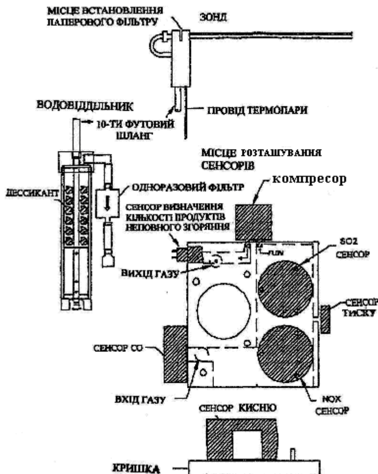
Рис. 11.38. Схема газового тракту ENERAC 2000
