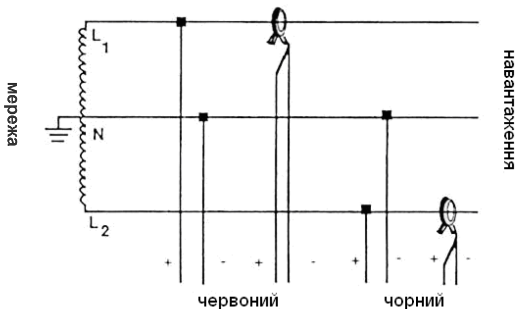
Рис. 11.10. 2-фазне 2-елементне приєднання
