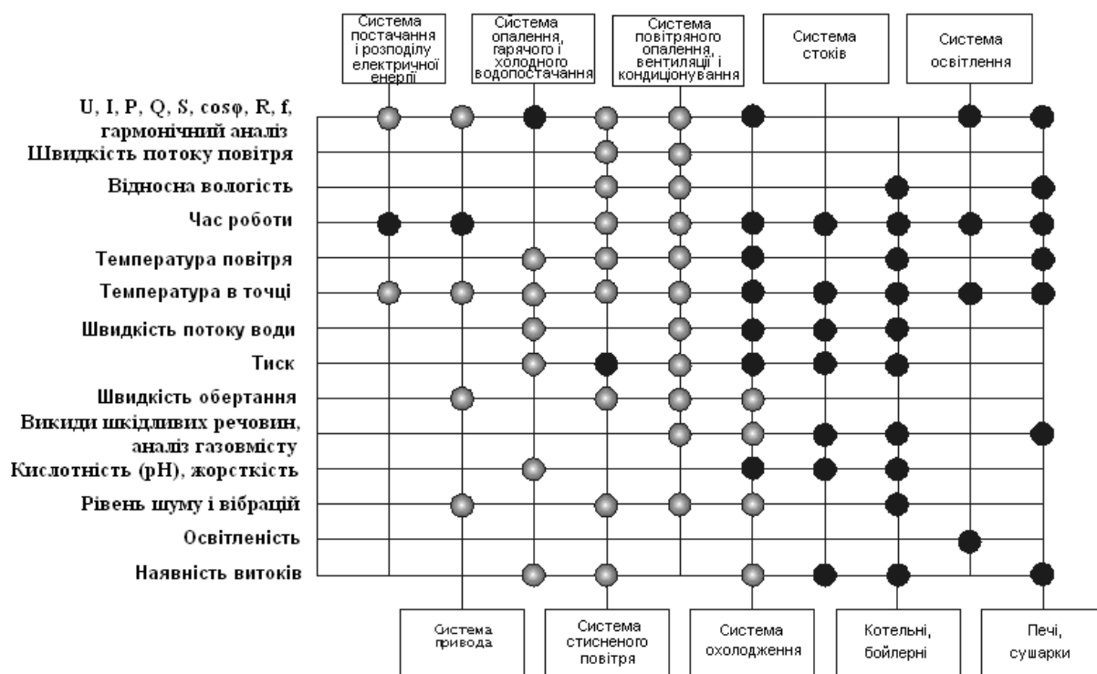
Рис. 11.1. Матриця вимірювань в енергоаудиті
