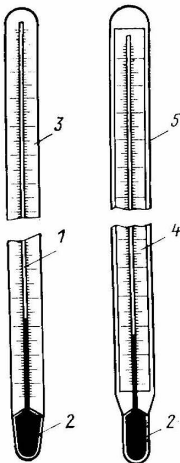
Рис. 11.13. Рідинні скляні термометри
