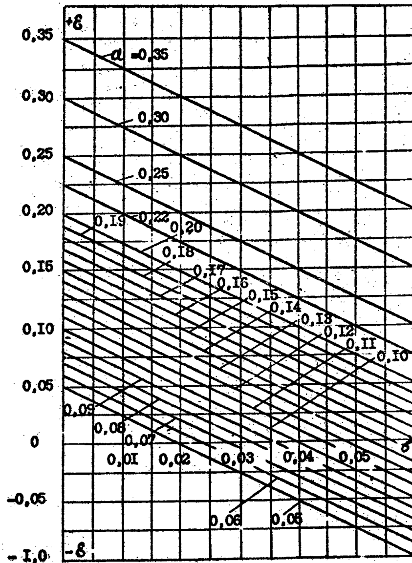
Рис. 8.5. Діаграма визначення ефективності обмежувачів неробочого ходу
