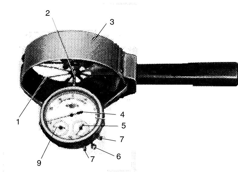
Рис. 11.25. Крильчатий анеометр АСО-3
