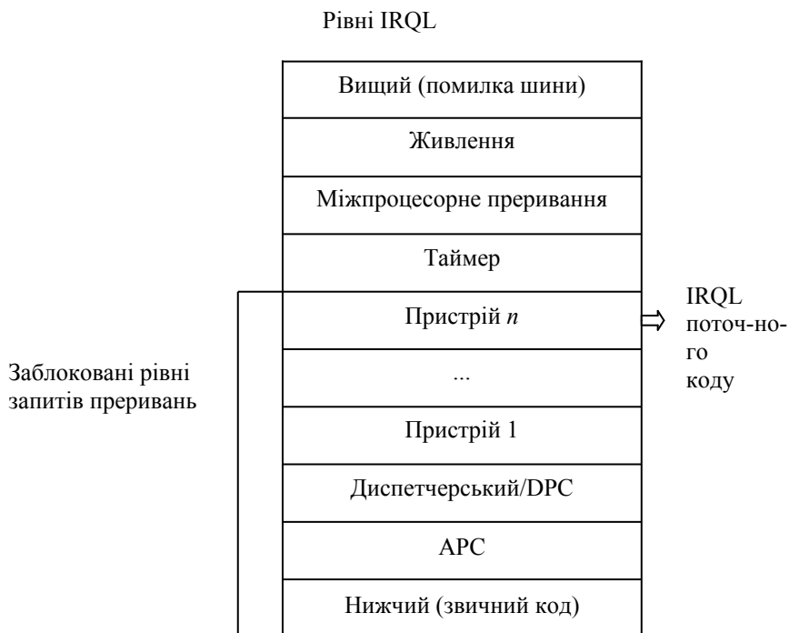
Рис. 2.11. Диспетчеризація переривань у Windows NT
