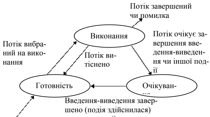
Рис. 2.1. Граф станів потоку в багатозадачному середовищі
