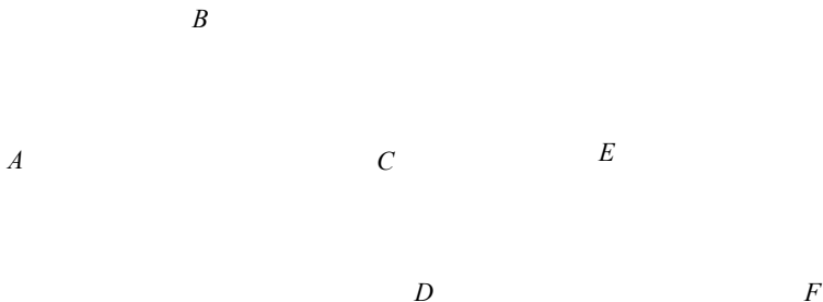
Рис. 3.19. Випадкова зв'язність
