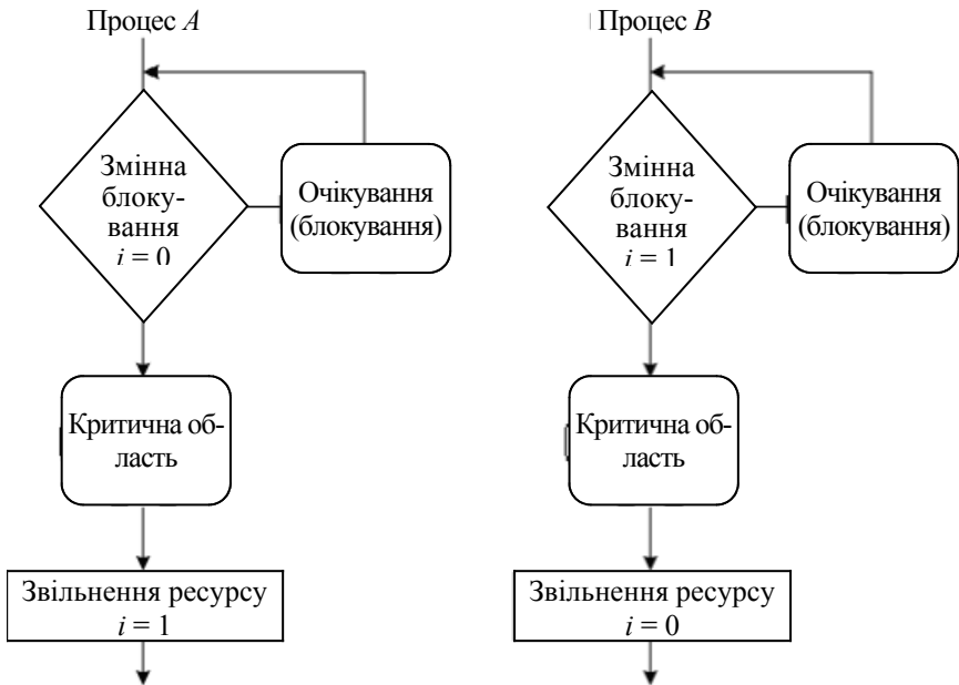
Рис.2.28. Чітке чергування
