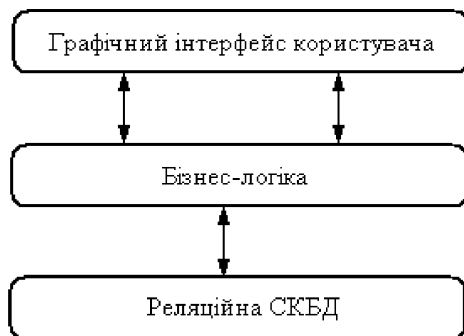
Рис. 3.10. Трирівнева модель
