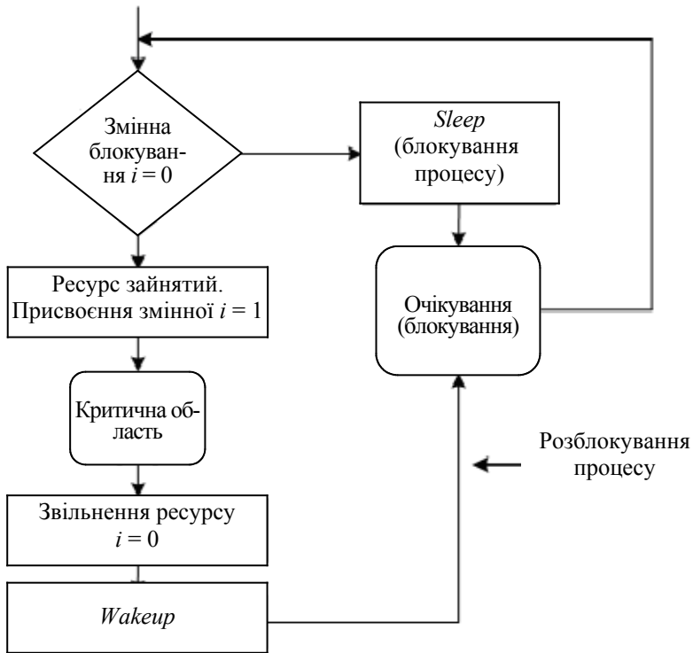
Рис. 2.29. Застосування примітивів
