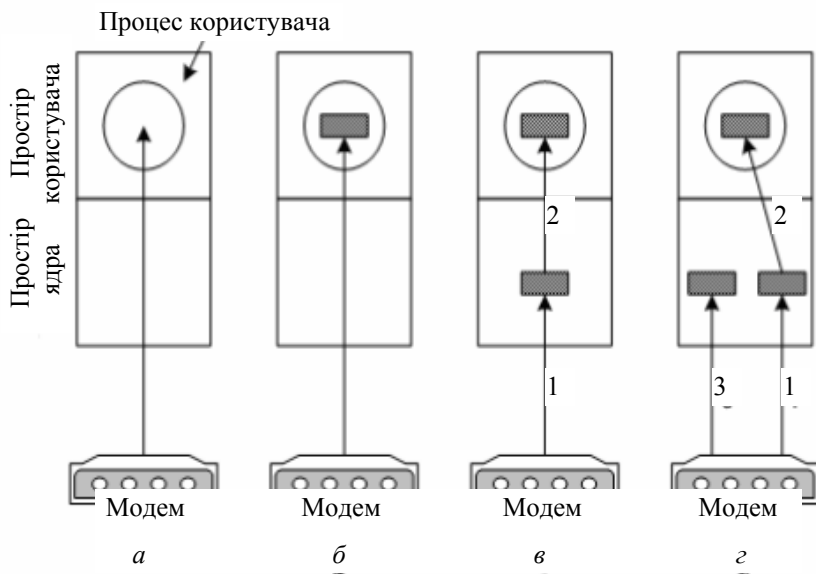
Рис. 2.38. Приклади буферизації
