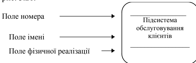
Рис. 3.26. Процес
