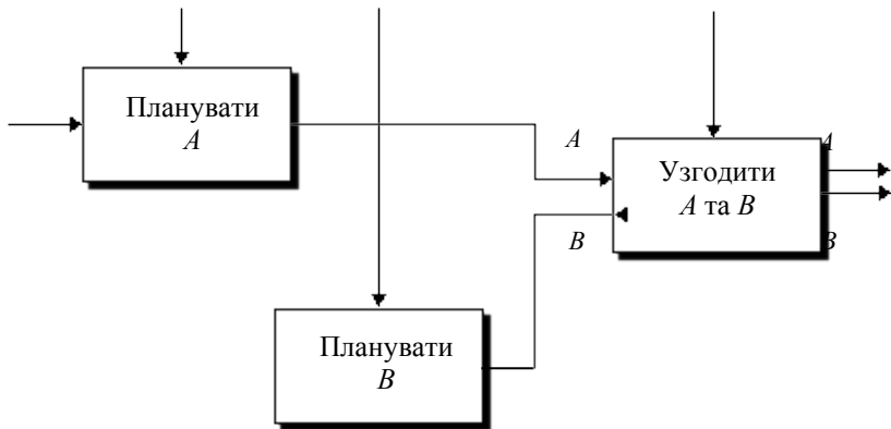
Рис. 3.20. Процедурна зв'язність
