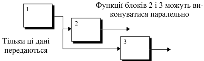
Рис. 3.14. Одночасне виконання
