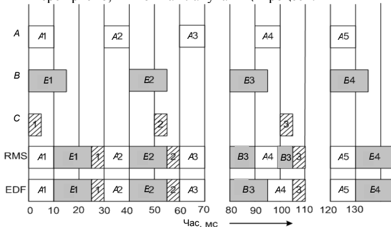
Рис. 2.21. Статичний алгоритм планування RMS
