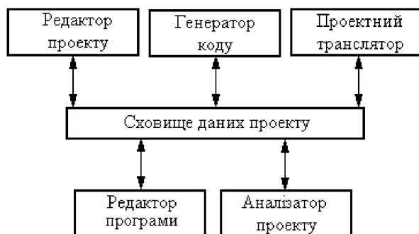
Рис. 3.8. Модель сховища даних
