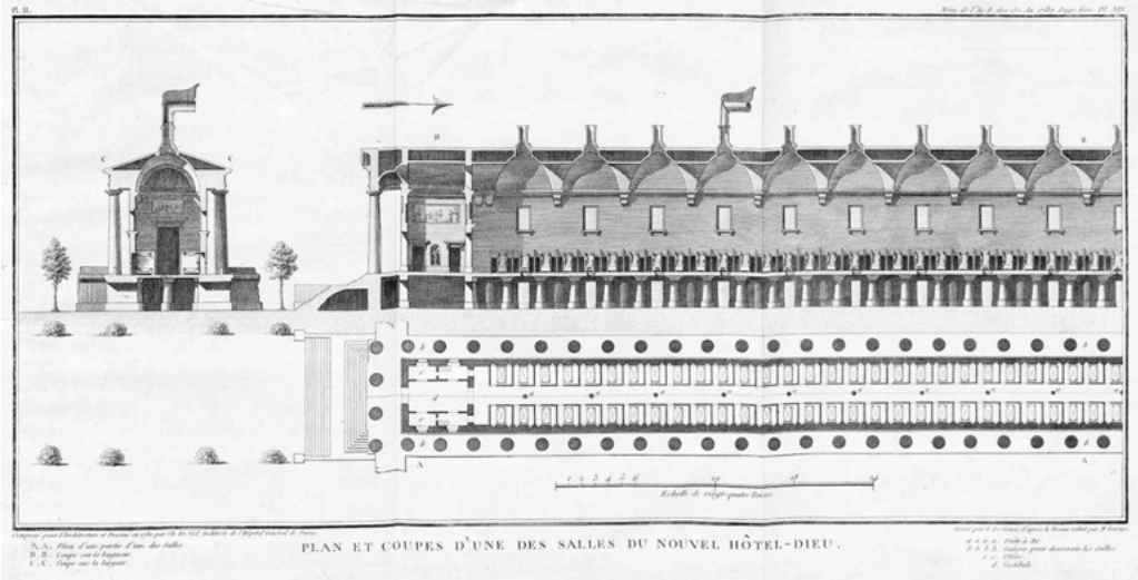
11 "[U]ne veritable machine à traiter des malades": hospital ward by Jean-Baptiste Le Roy, 1786
