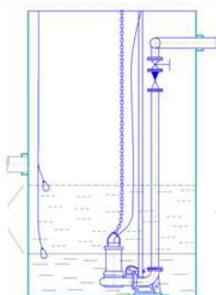
Застосування однорівневих поплавків
