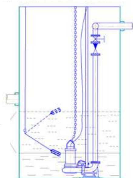
Застосування дворівневих поплавків
