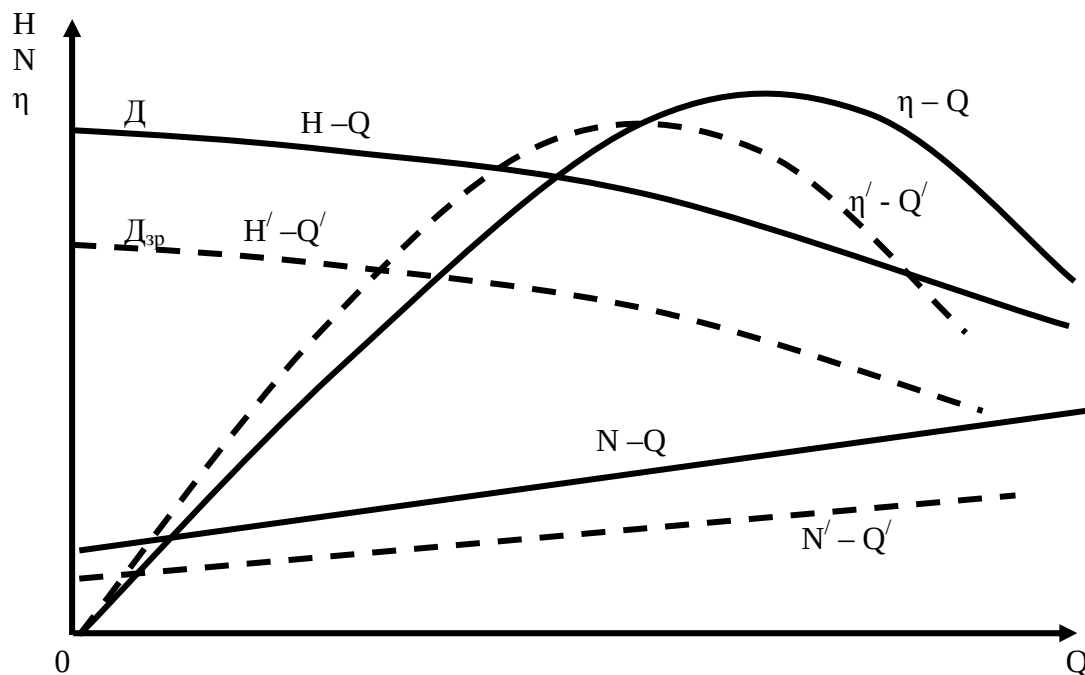
Рисунок 1.15 – Зміна характеристик насоса під час зрізання діаметра робочого колеса
