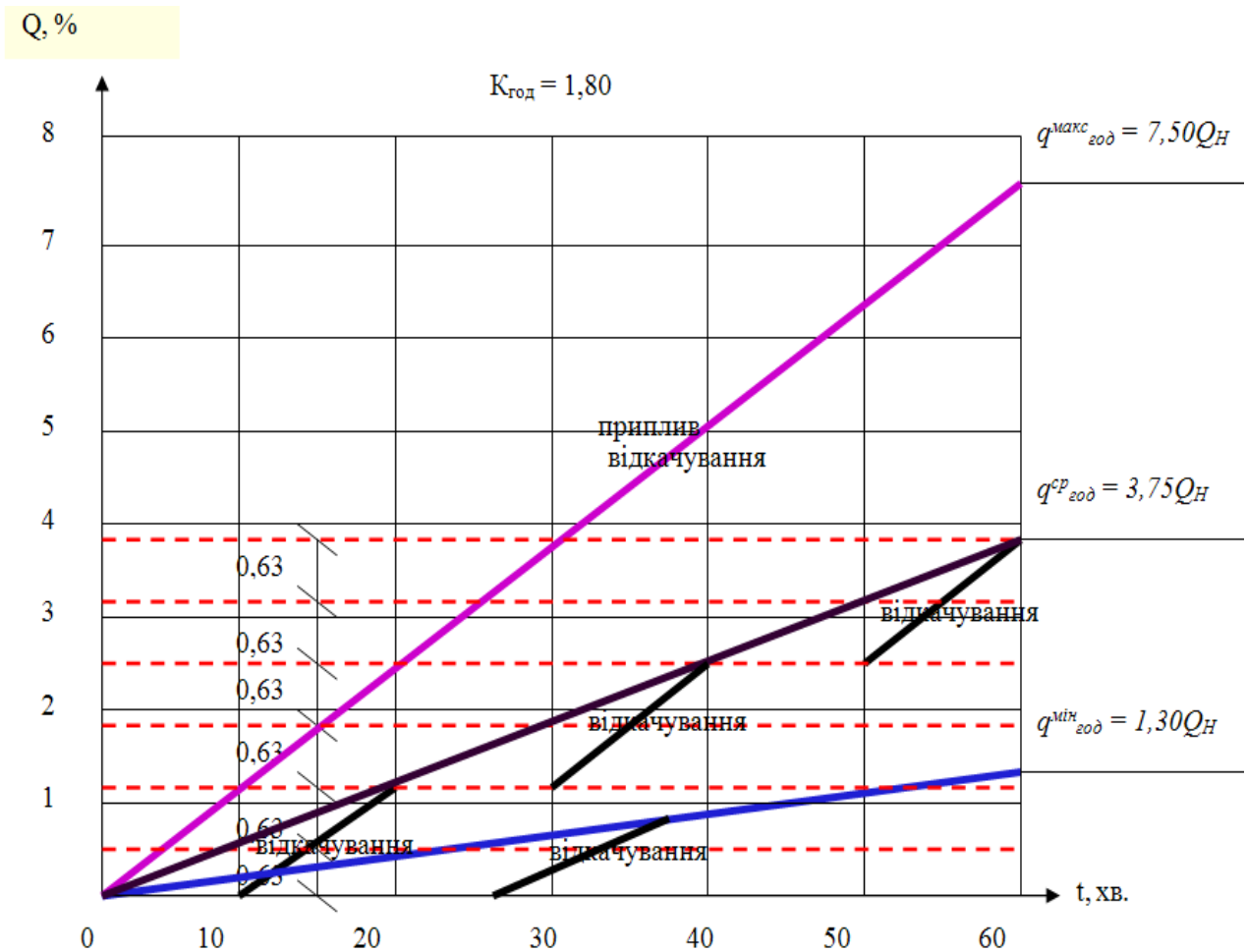
Рисунок 3.2 – Погодинні графіки припливу і відкачування стічних вод для K_{\text{год}} = 1,8
