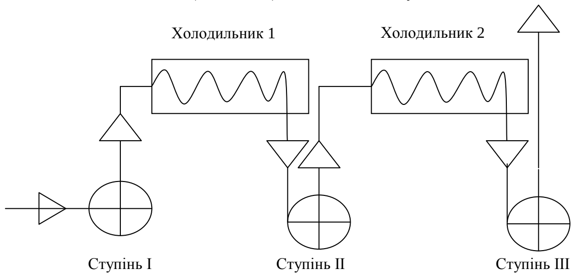
Рисунок 4.5 – Трьохступенева компресорна установка з охолодженням кожного ступеня
