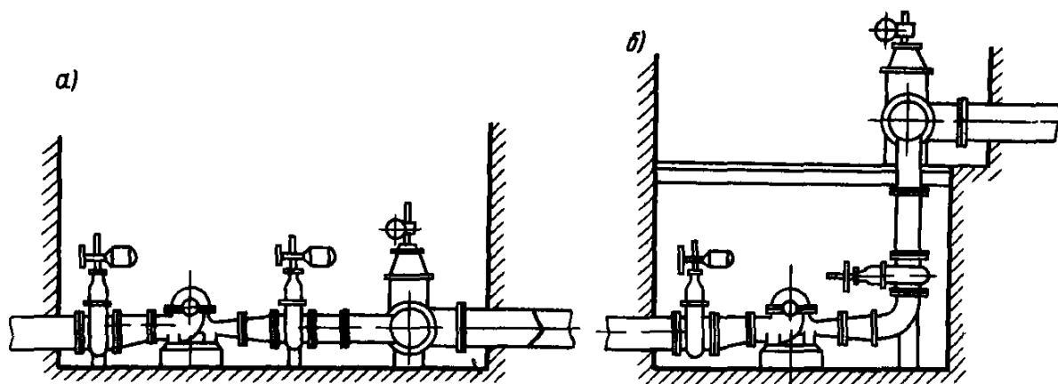
Рисунок 2.34 – Горизонтальне й вертикальне компоновання напірних внутрішньостанційних трубопроводів
