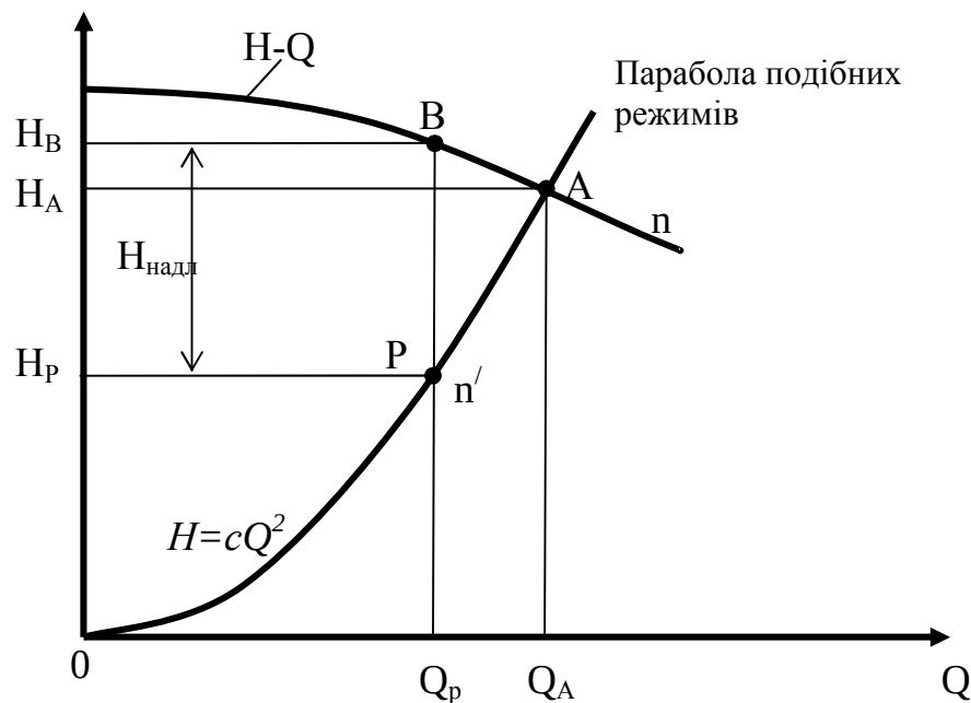
Рисунок 1.9 – Зміна головної характеристики насоса під час зміни кількості обертів робочого колеса
