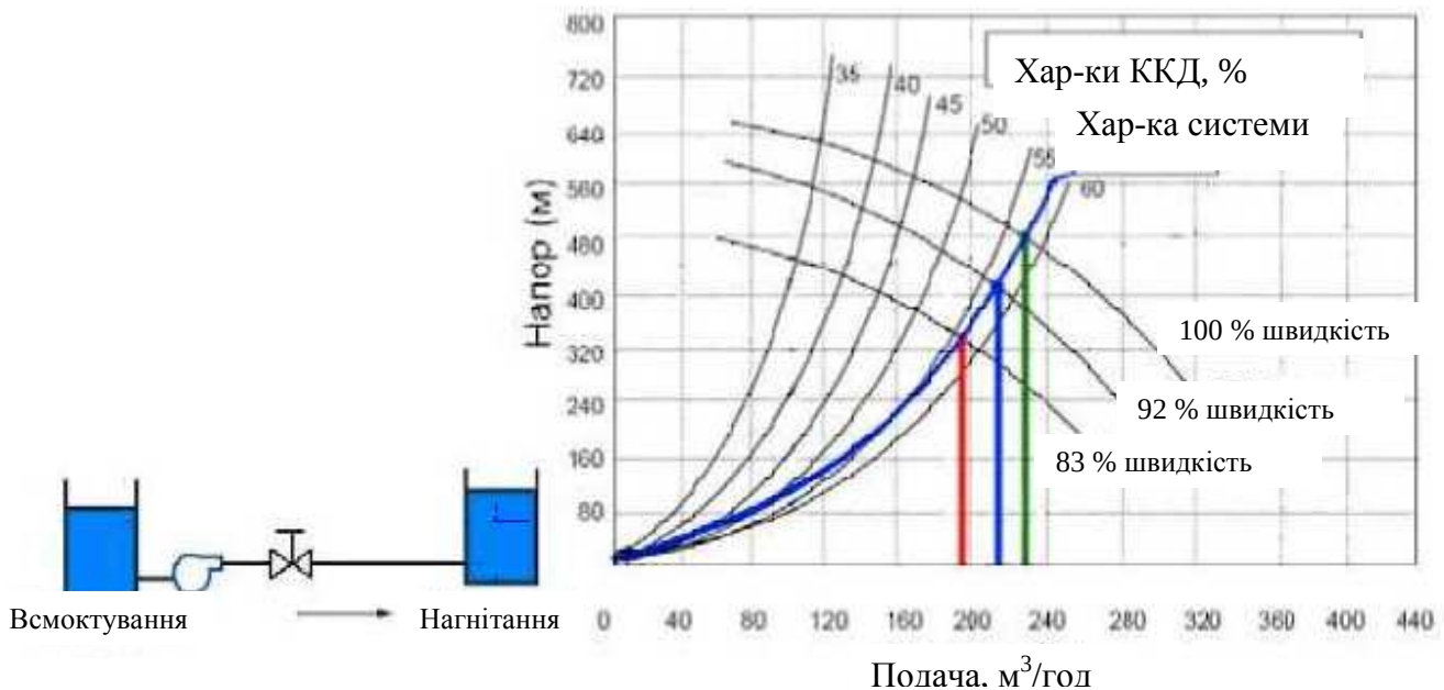
Рисунок 1.13 – Схема впливу роботи насоса з частотним регулюванням на мережу з переважними втратами на тертя
