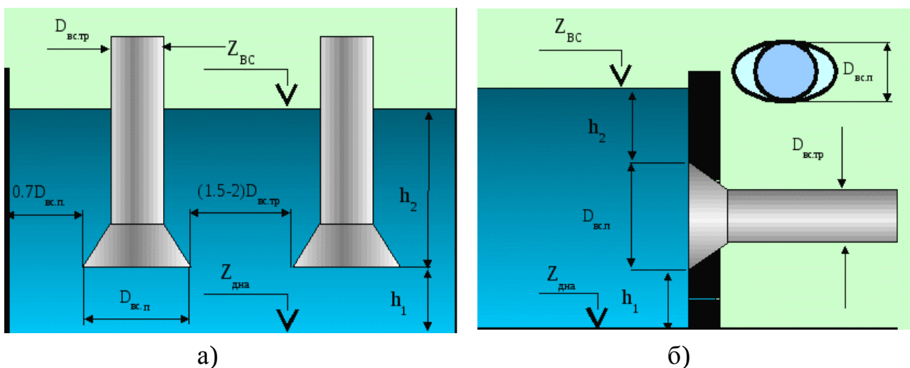
Рисунок 2.4. – Схеми розміщення усмоктувальних труб у камері:
