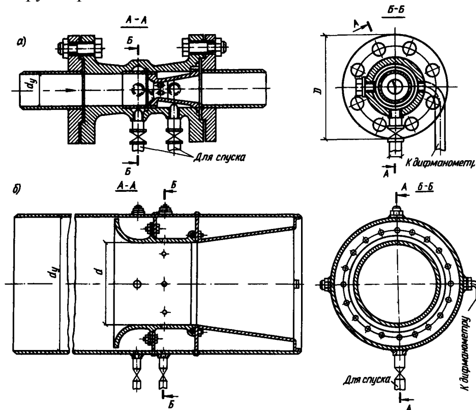
Рисунок 2.45 – Сопла Вентурі
