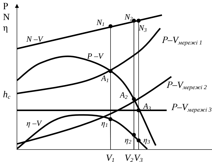
Рисунок 4.9 – Характеристика роботи мережі (повітропроводу)
