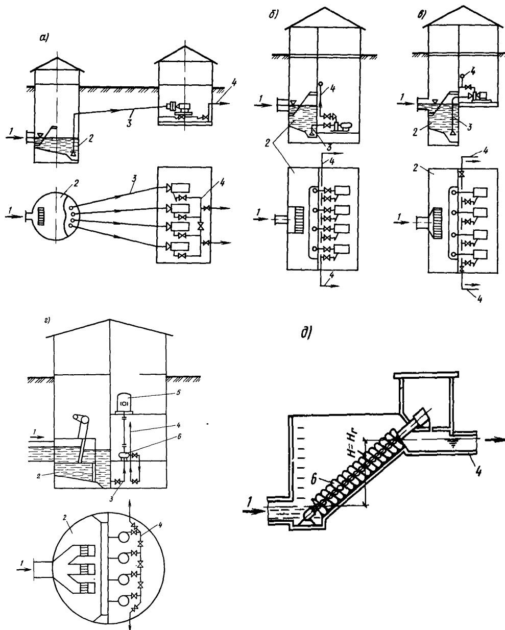
Рисунок 3.1 – Схеми каналізаційних насосних станцій:
