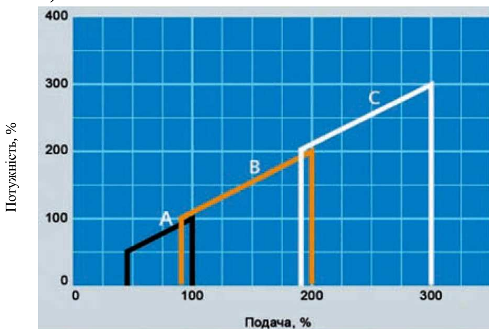
Рисунок 4.12 – Каскадне регулювання роботи повітрорудовок
