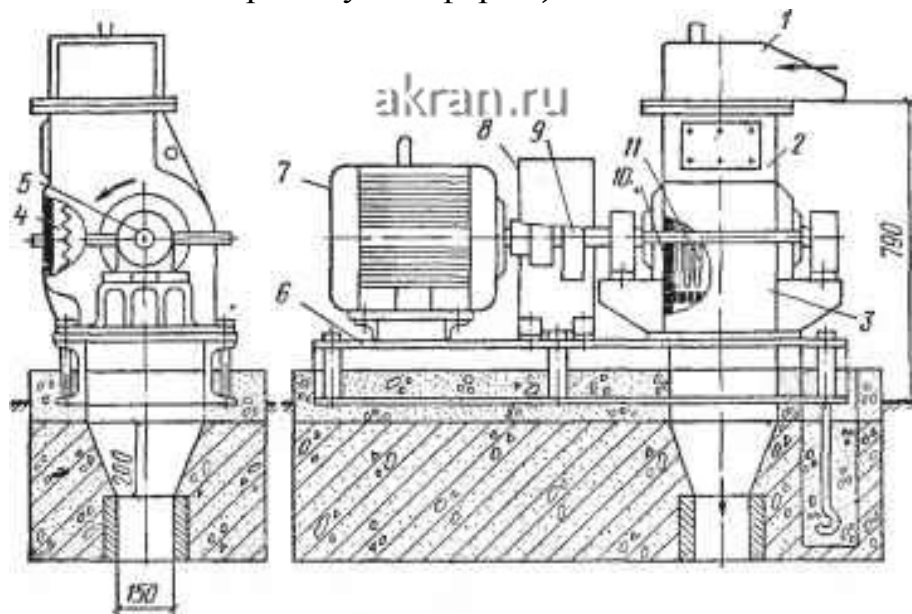
Рисунок 3.5 – Дробарка молоткова:
