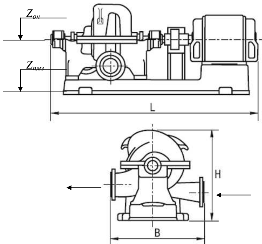
Рисунок 2.32 – Схема для визначення габаратних розмірів насосного агрегата та основних позначок у машинному залі насосної станції
