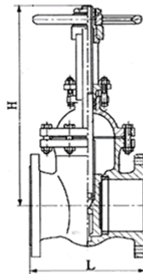
Рисунок 2.36 – Засувка паралельна дводискова чавунна
