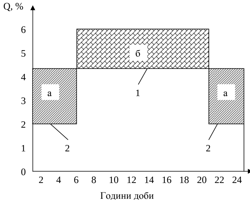
Рисунок 2. 19 – Сумісний графік роботи насосних станцій першого та другого підйому
