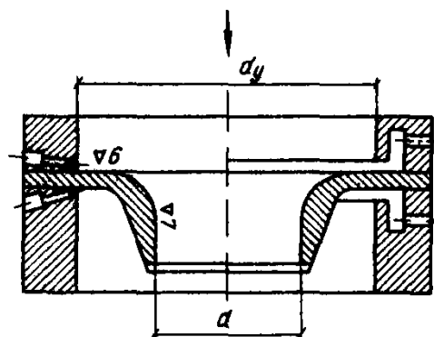
Рисунок 2.46 – Сопло нормальне
