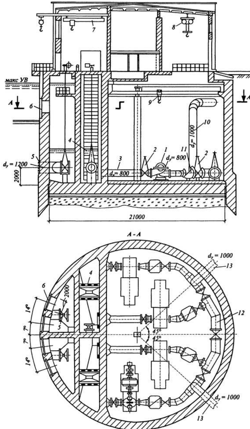
Рисунок 2.11 – Насосна станція з комбінованим водозабором:
