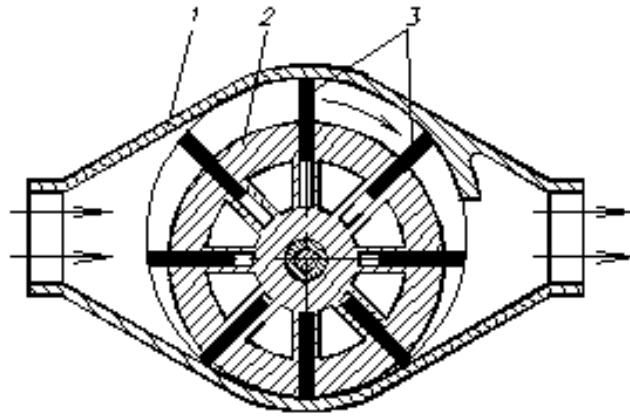
Рисунок 4.6 – Схема шибєрного (пластинчатого) компресора: 1 – корпус; 2 – ротор; 3 – пластини
