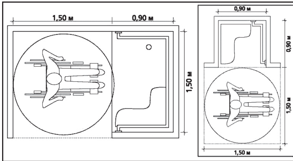
Рис. 36: Мінімальні розміри душової kabini
