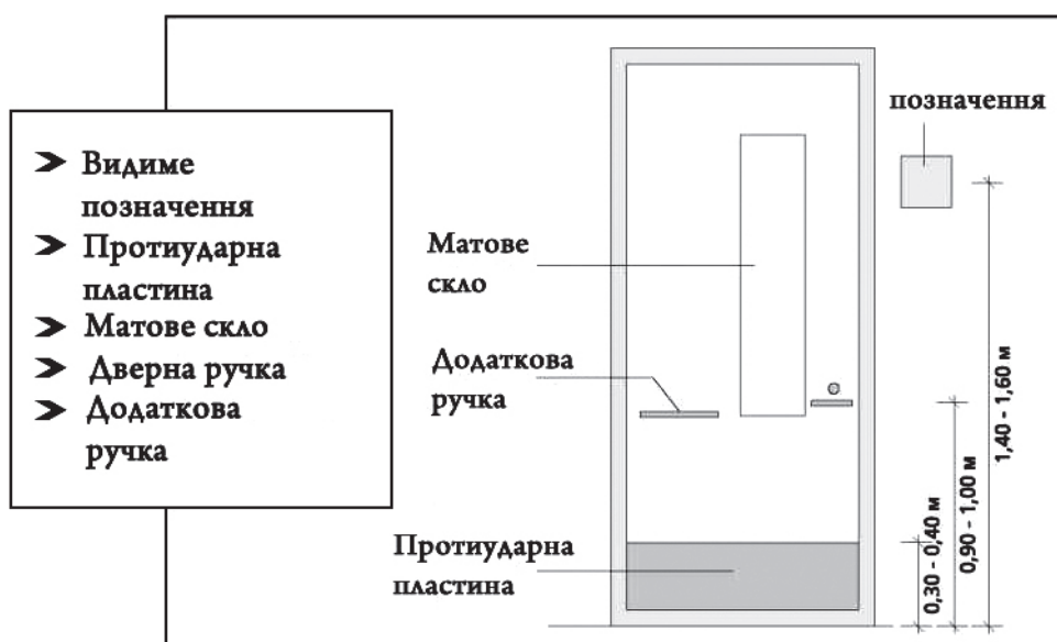
Рис. 22: Характеристика доступної двері
