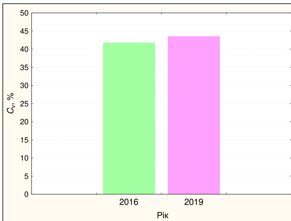
Рис. 3.3. Гістограма розподілу коефіцієнта варіації середньої тривалості перебування туристів у колективних засобах розміщення по регіонах України
