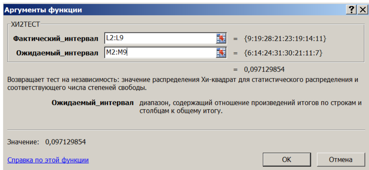
Рис. 7.24. Приклад заповнення робочих полів функції ХИ2ТЕСТ()
