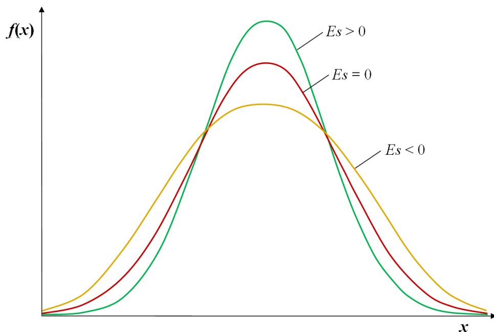
Рис. 4.5. Криві розподілу з різним ступенем крутості (ексцесом)
