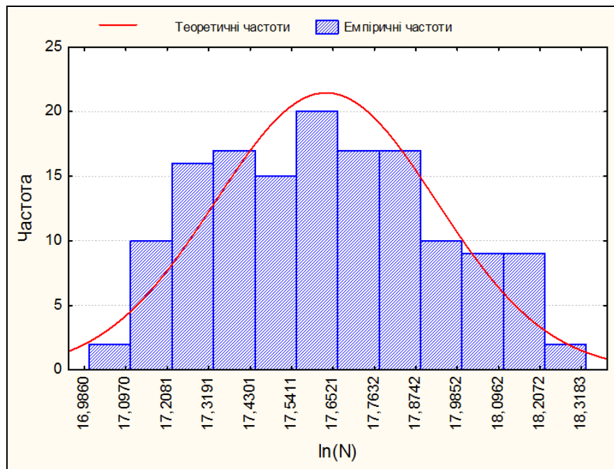
Рис. 4.8. Гістограма розподілу \ln(N) частотного
